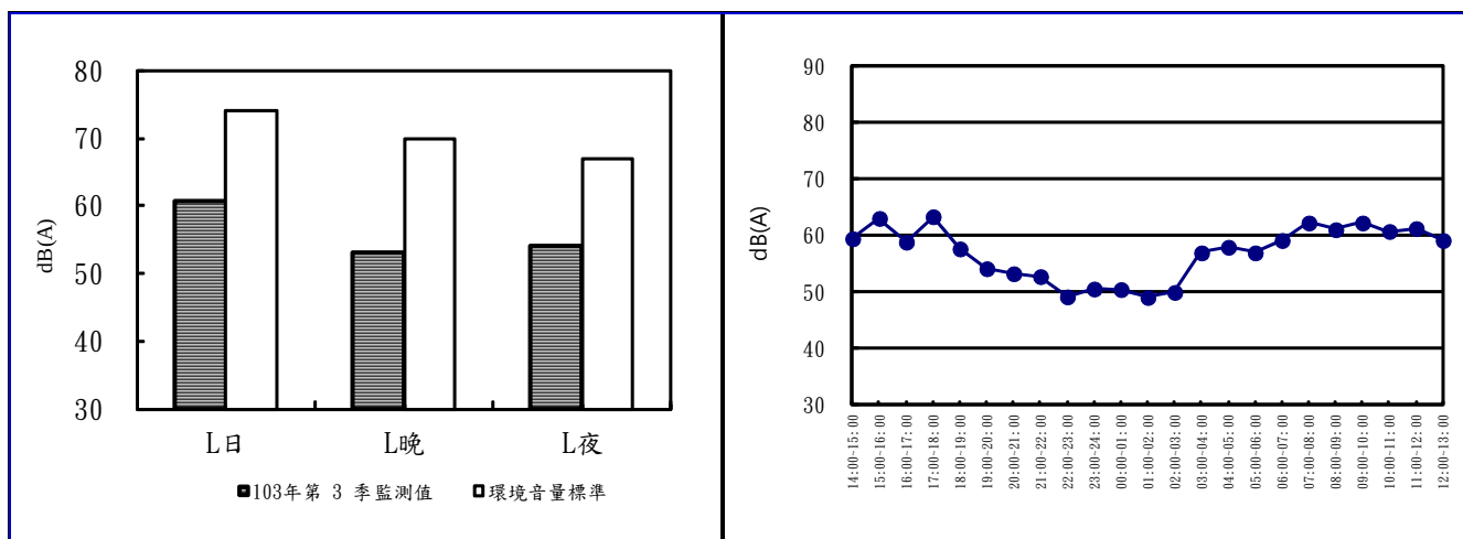
圖2.2-1 安西府 103 年第 4 季噪音監測成果分析圖及逐時變化圖
