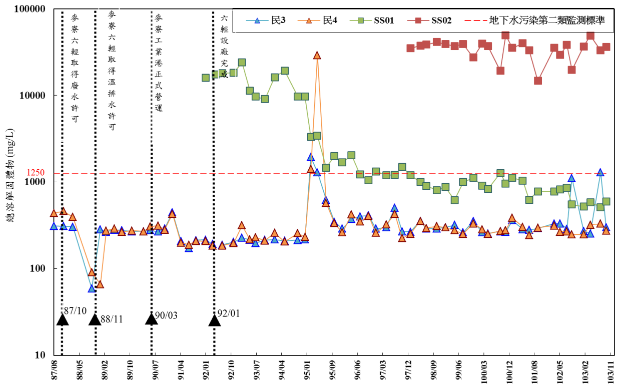
圖 3.1.6-5 總溶解固體物歷年濃度測值變化
