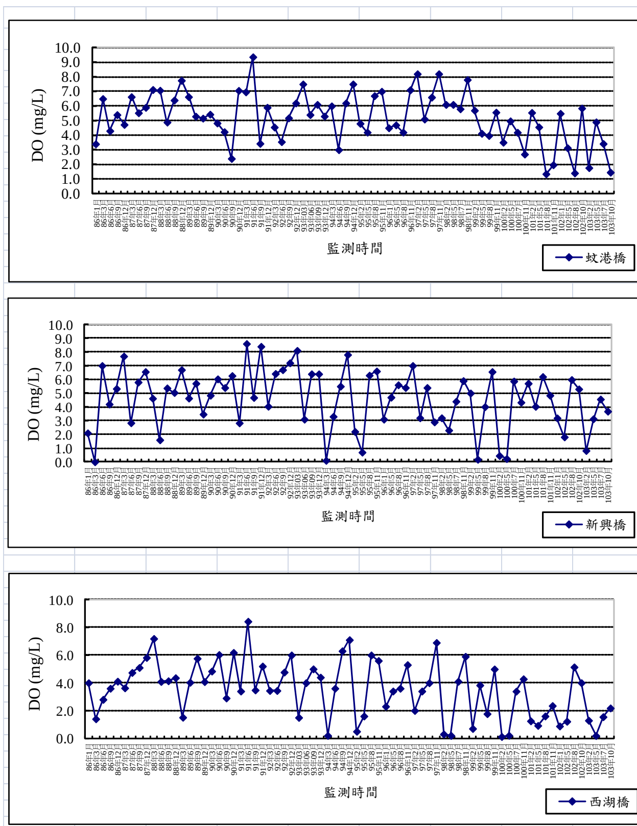
圖 3.1.7-2 陸域水質歷次溶氧比較分析圖
