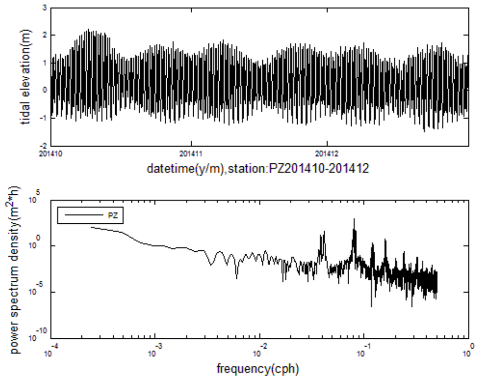
圖 2.13-4 PZ 測站 2014 年 10~12 月實測潮位頻譜與逐時變化圖
