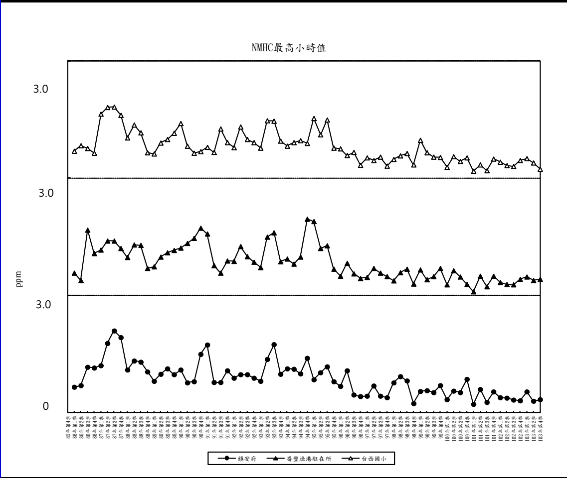
圖3.1.1-6本計畫歷次NMHC最高小時值監測結果分析圖
