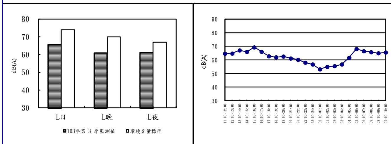
圖2.2-3 崙豐國小 103 年第 4 季噪音監測成果分析圖及逐時變化圖
