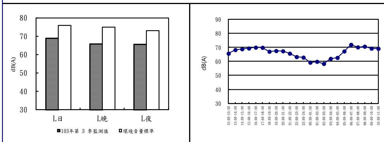
圖2.2-2 海豐橋 103年第 4 季噪音監測成果分析圖及逐時變化圖
