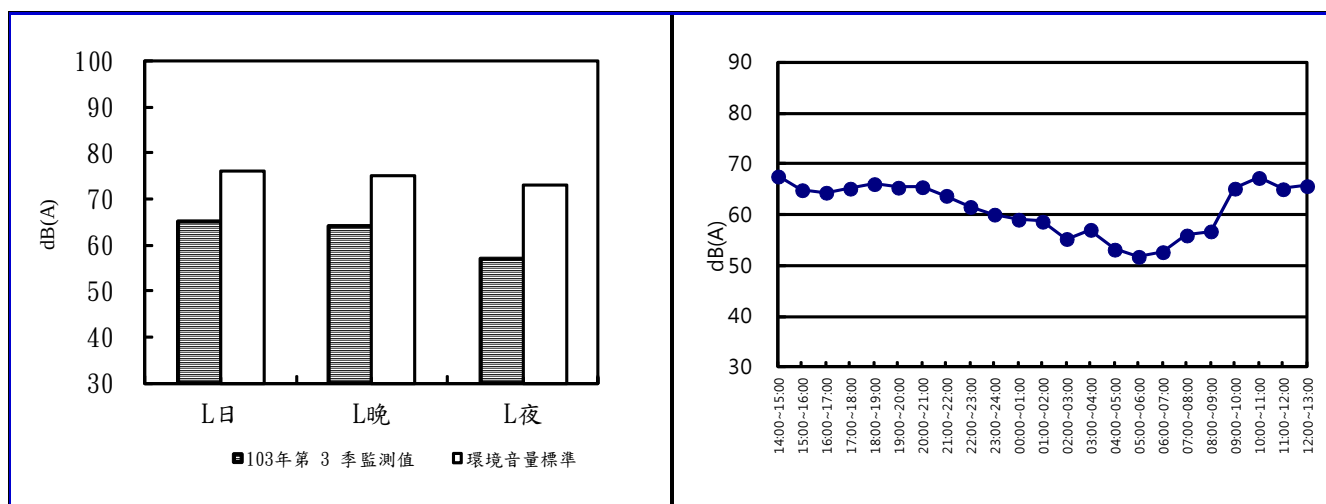
圖2.2-4 海口橋 103 年第 4 季噪音監測成果分析圖及逐時變化圖
