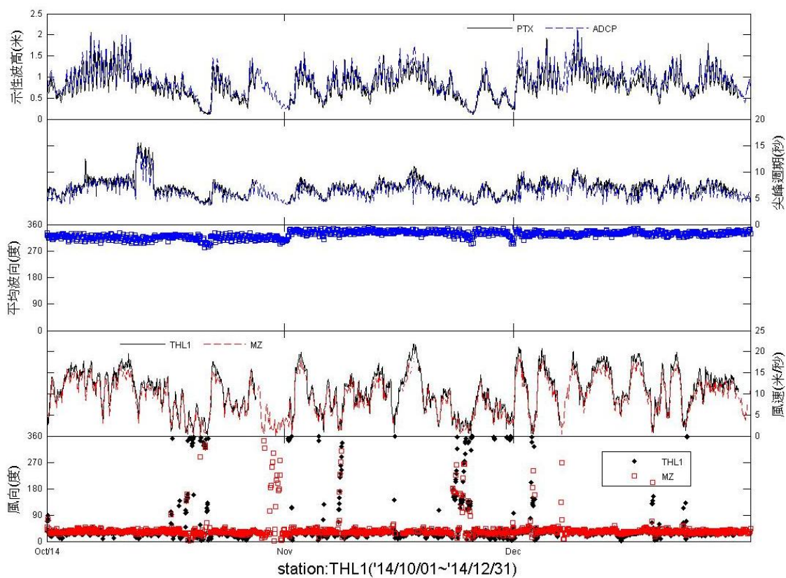
圖 2.13-6 THL1 測站 2014 年 10 月~12 月波浪與風速風向時序列
