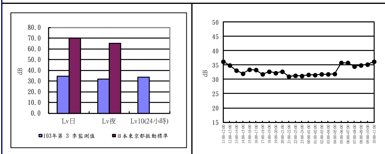
圖2.3-2 海豐橋 103 年第 4 季振動監測成果分析圖及逐時變化圖
