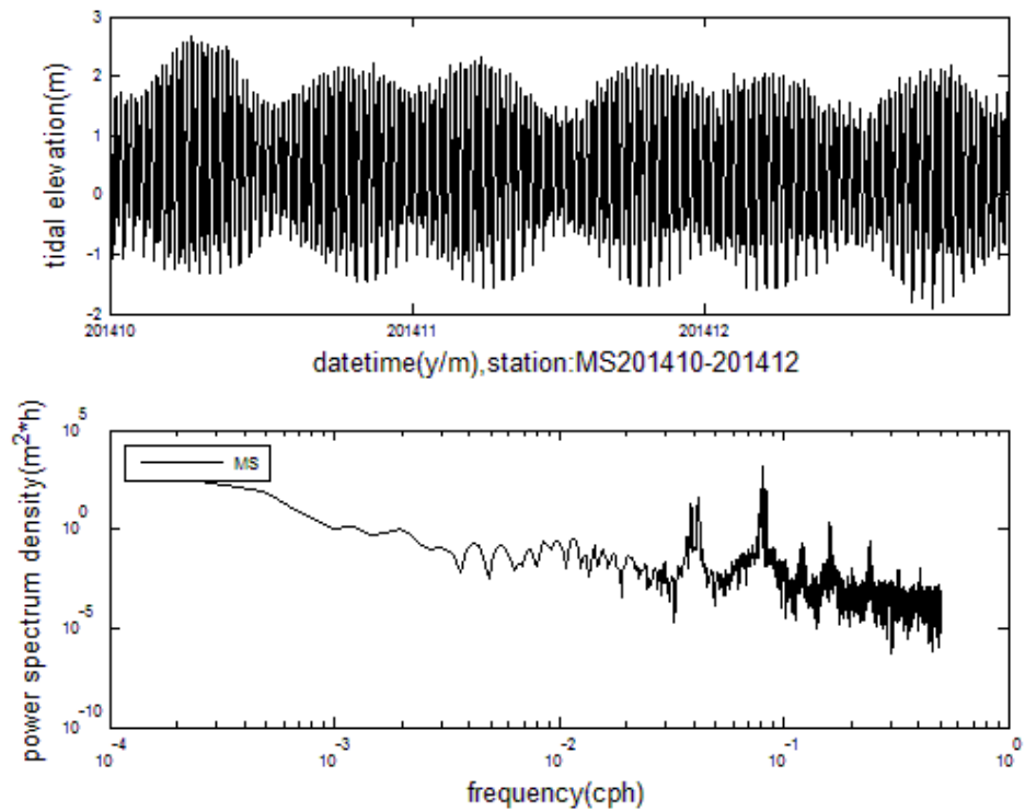
圖 2.13-3 MS 測站 2014 年 10~12 月實測潮位頻譜與逐時變化圖
