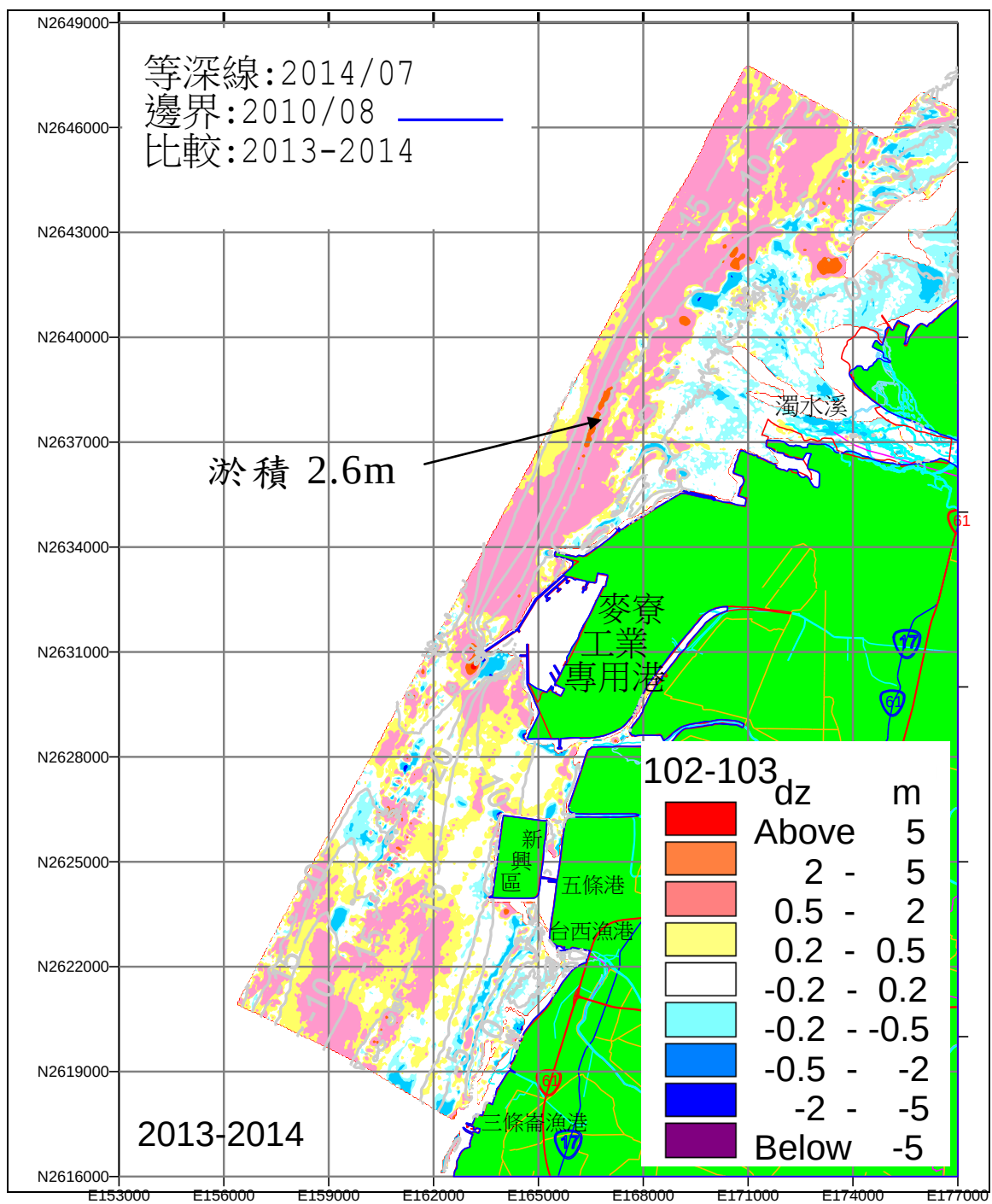
圖 2.12-2 本區地形測量變動量計算圖(2012~2014)
