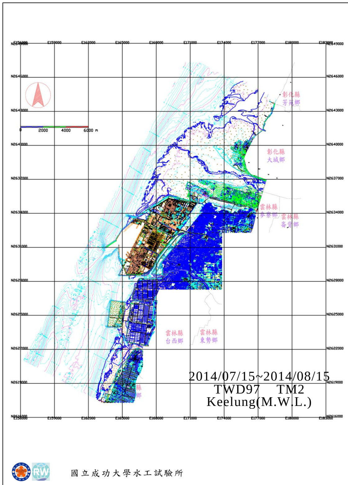
圖 2.12-1 本區海域 2014 年海域地形圖
