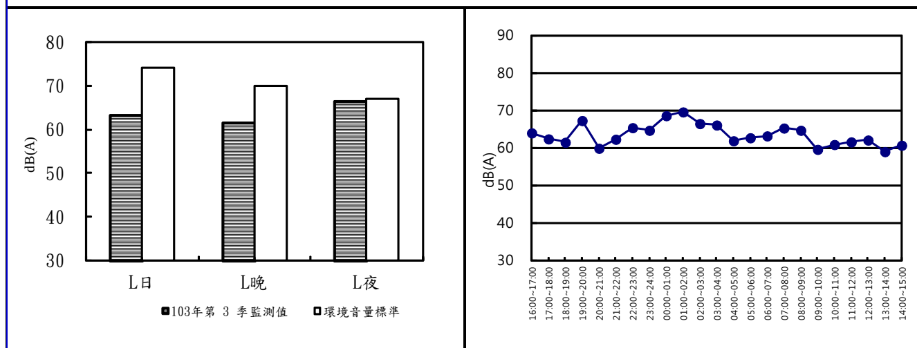
圖2.2-5 五條港出入管制站 103 年第 4 季噪音監測成果分析圖及逐時變化圖
