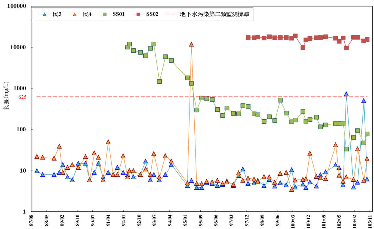
圖 2.6.2-6 氯鹽歷年濃度測值變化
