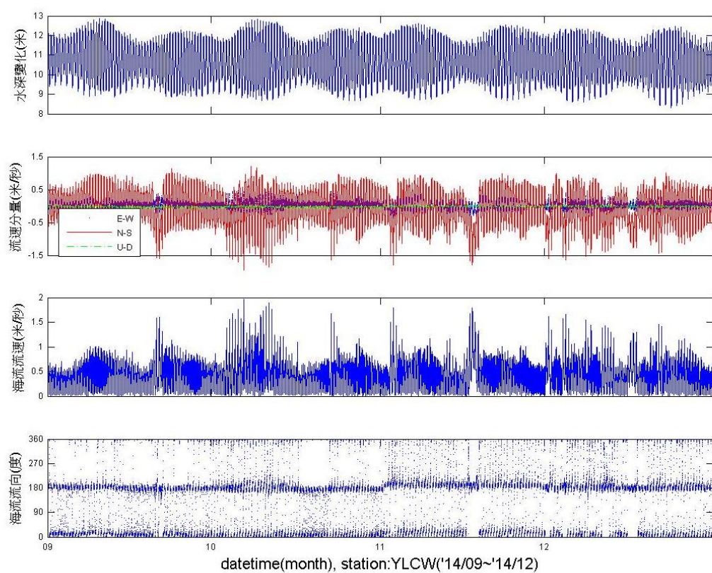
圖 2.13-10 YLCW 測站 2014 年 10 月~12 月海流分量與流速流向時序列
