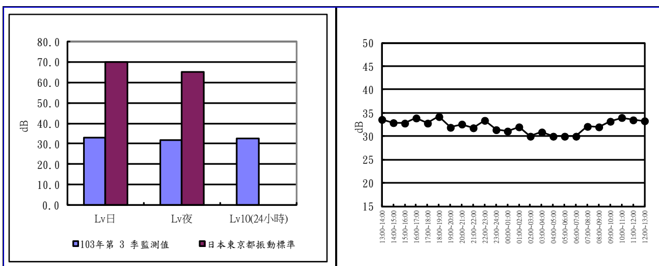
圖2.3-4 海口橋 103 年第 4 季振動監測成果分析圖及逐時變化圖
