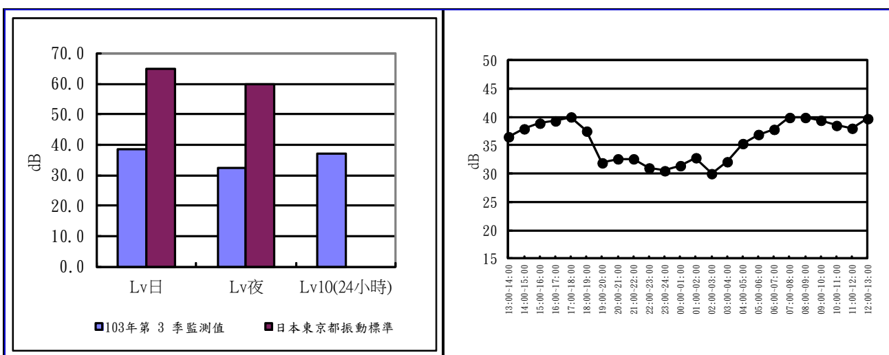
圖2.3-1 安西府 103 年第 4 季振動監測成果分析圖及逐時變化圖
