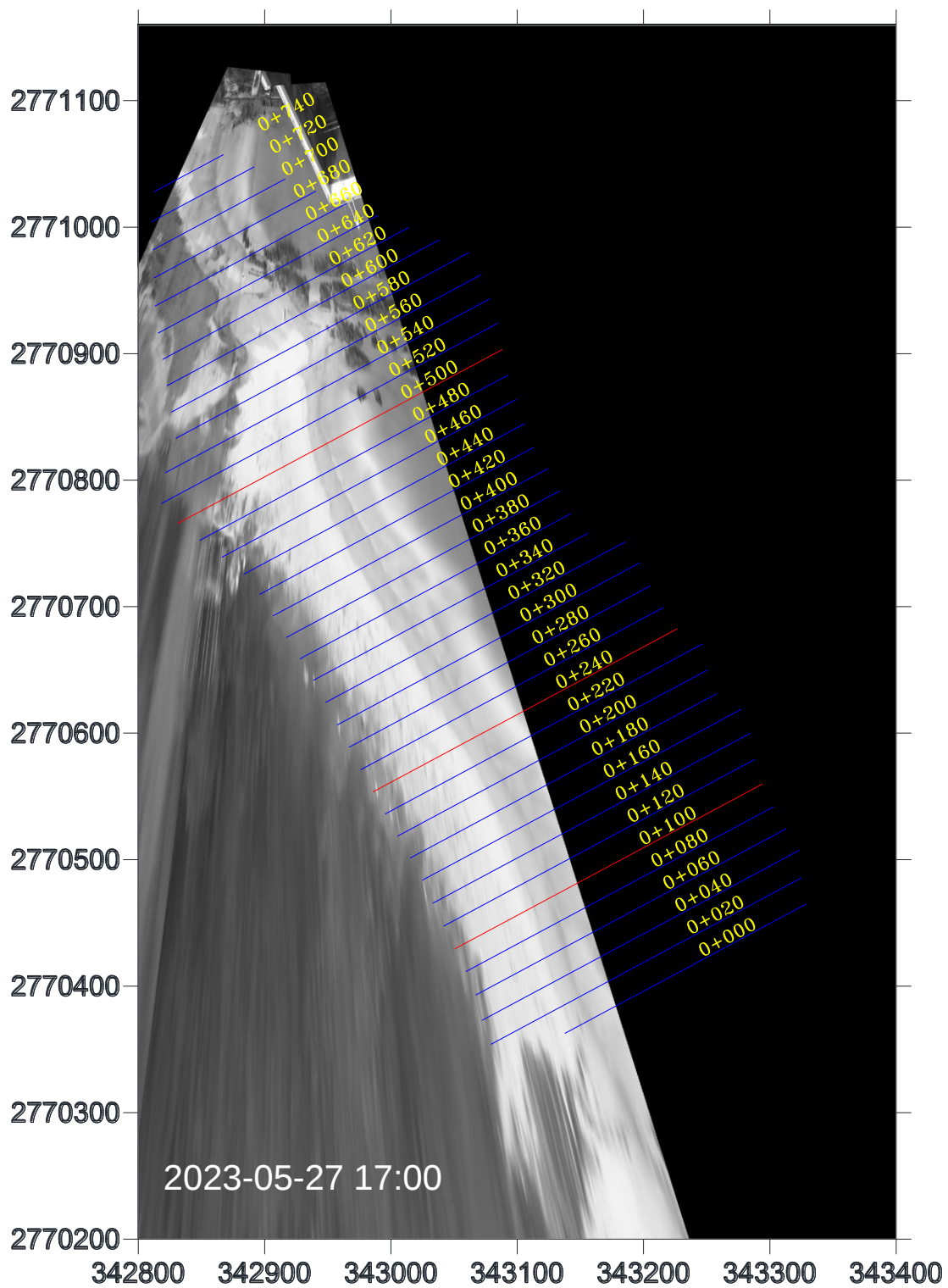
圖 4-14 鹽寮海岸地形影像全景圖(2023/05/27 17:00)
