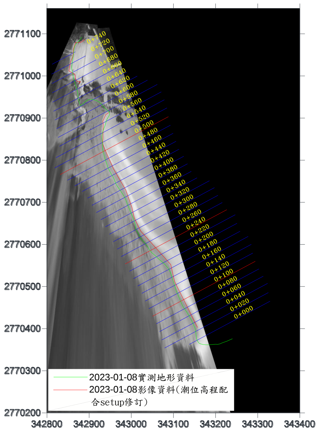
圖 3-24 水位線分析結果圖(2023/01/08)
