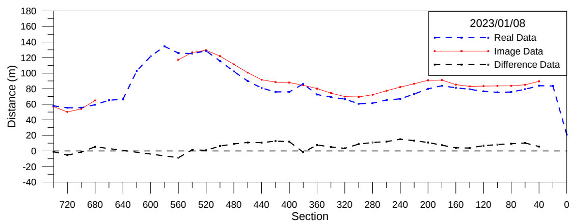
圖 3-25 海岸線分析比較圖(2023/01/08)
