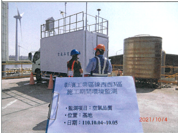
空氣品質：基地 (110.10.04~05)
