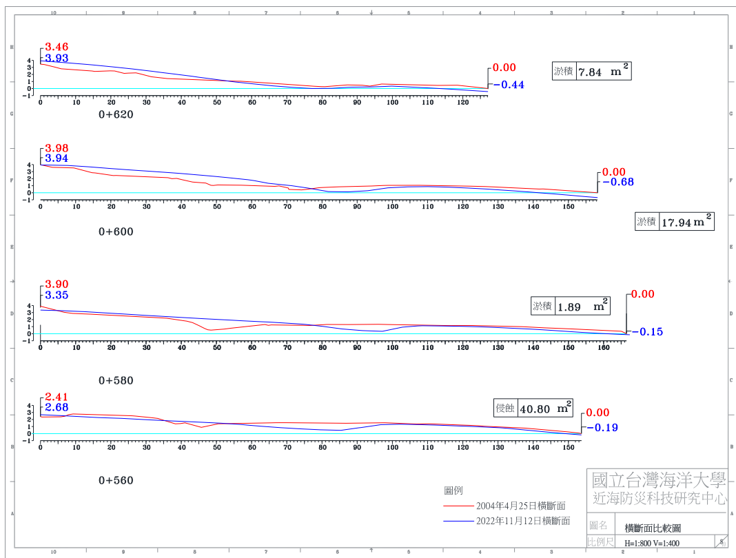
圖 4-4(c) 2022 年 11 月 12 日 A 監測區橫斷面比較圖
