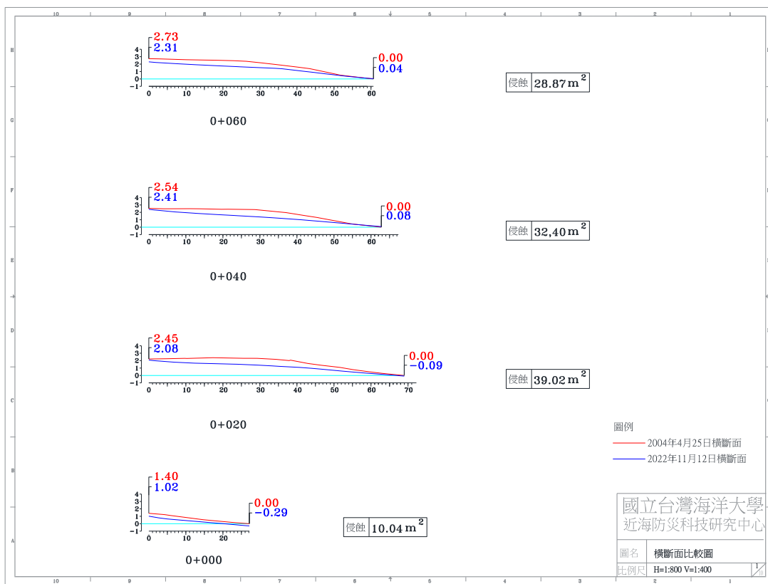
圖 4-4(j) 2022 年 11 月 12 日 A 監測區橫斷面比較圖
