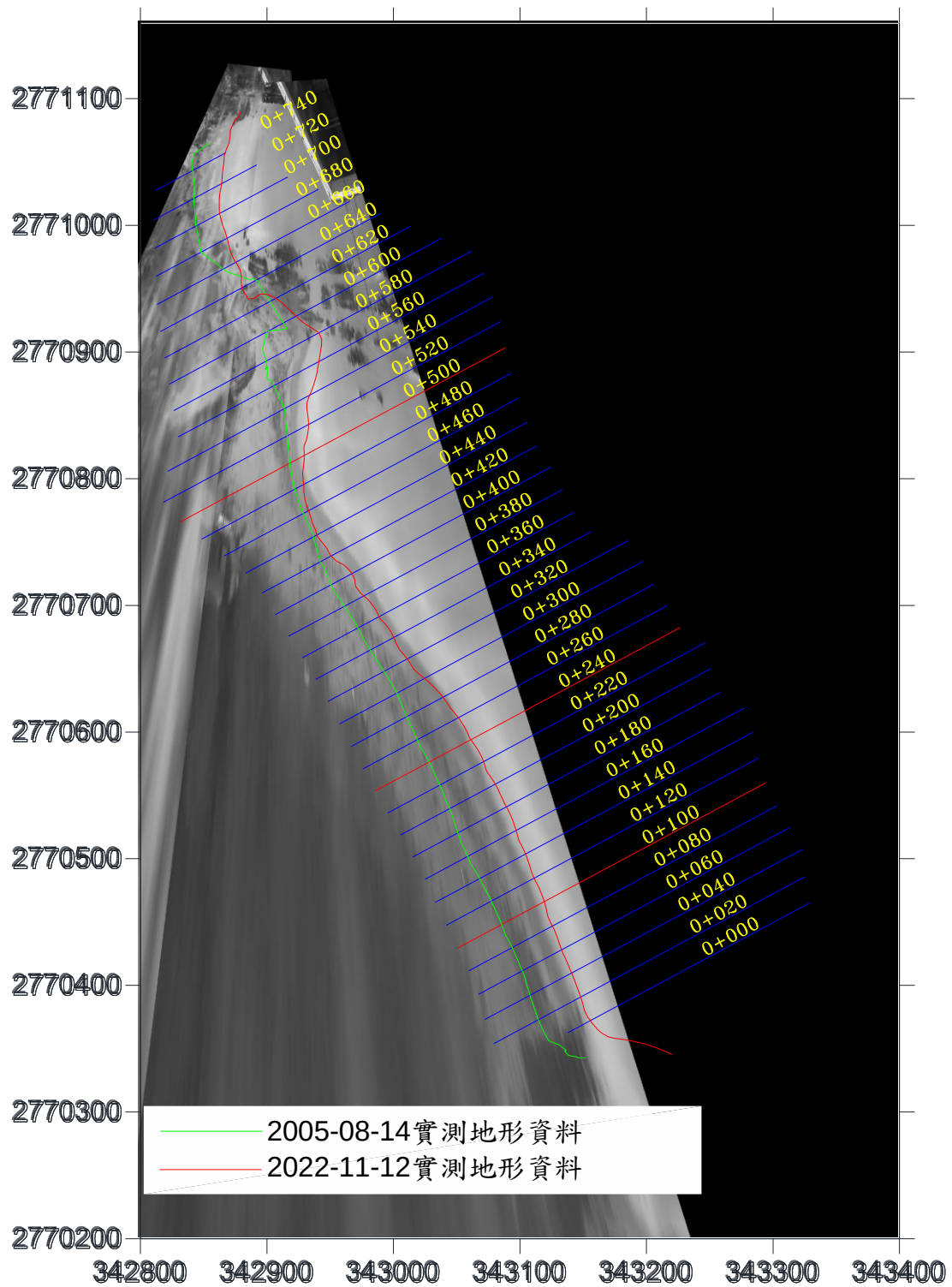
圖 4-22 長期實測 0 m 灘線比對平面示意圖(2022/11/12)
