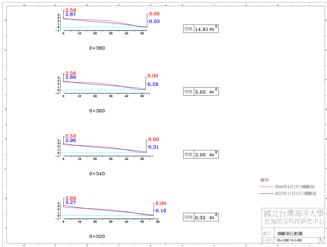
圖 4-4(f) 2022 年 11 月 12 日 A 監測區橫斷面比較圖
