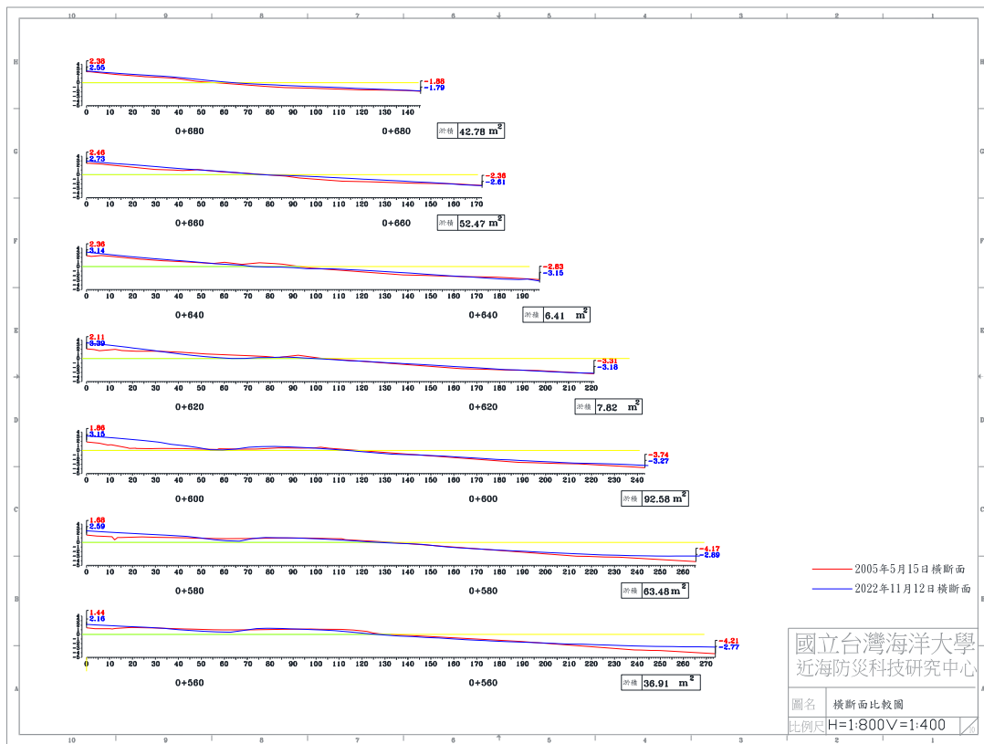
圖 4-5(b) 2022 年 11 月 12 日 B 監測區橫斷面比較圖
