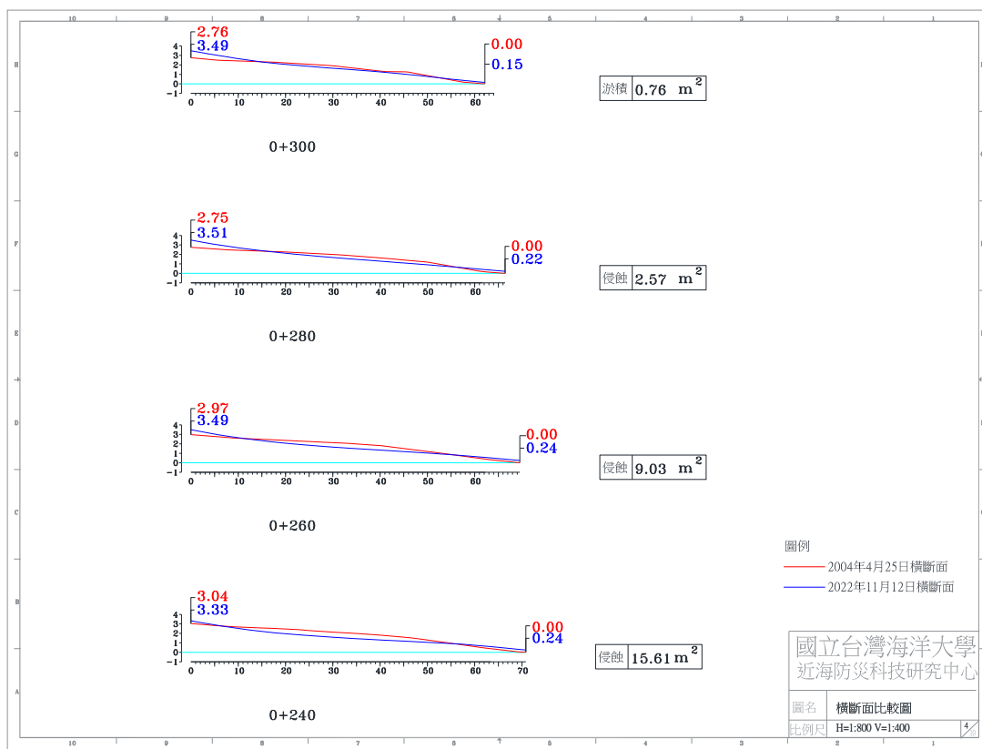
圖 4-4(g) 2022 年 11 月 12 日 A 監測區橫斷面比較圖
