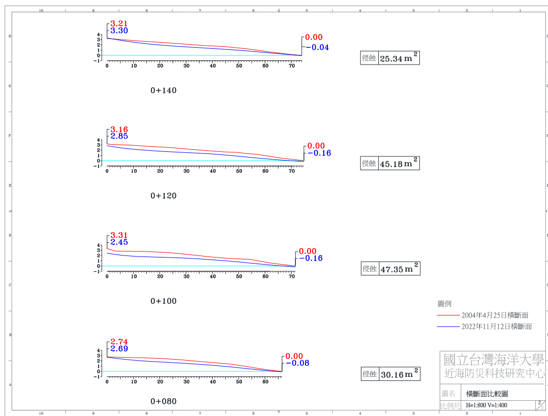
圖 4-4(i) 2022 年 11 月 12 日 A 監測區橫斷面比較圖
