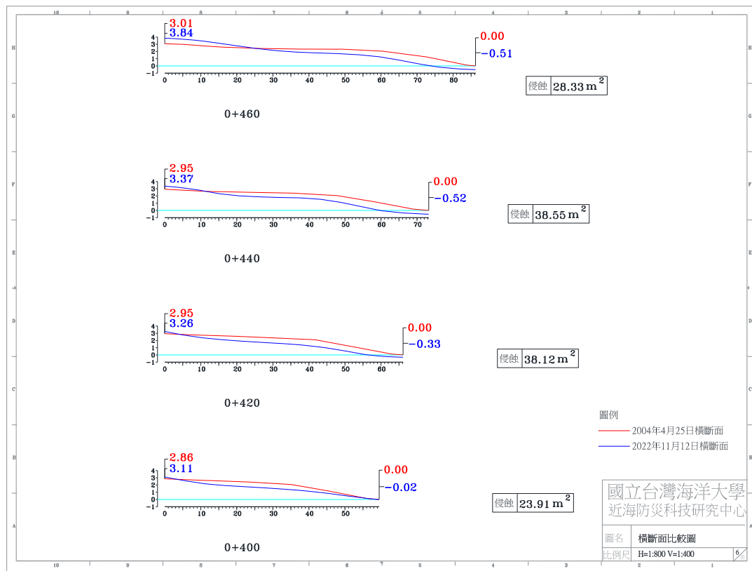
圖 4-4(e) 2022 年 11 月 12 日 A 監測區橫斷面比較圖
