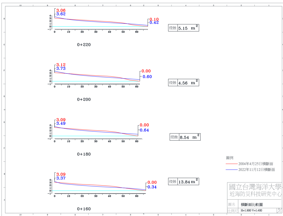
圖 4-4(h) 2022 年 11 月 12 日 A 監測區橫斷面比較圖
