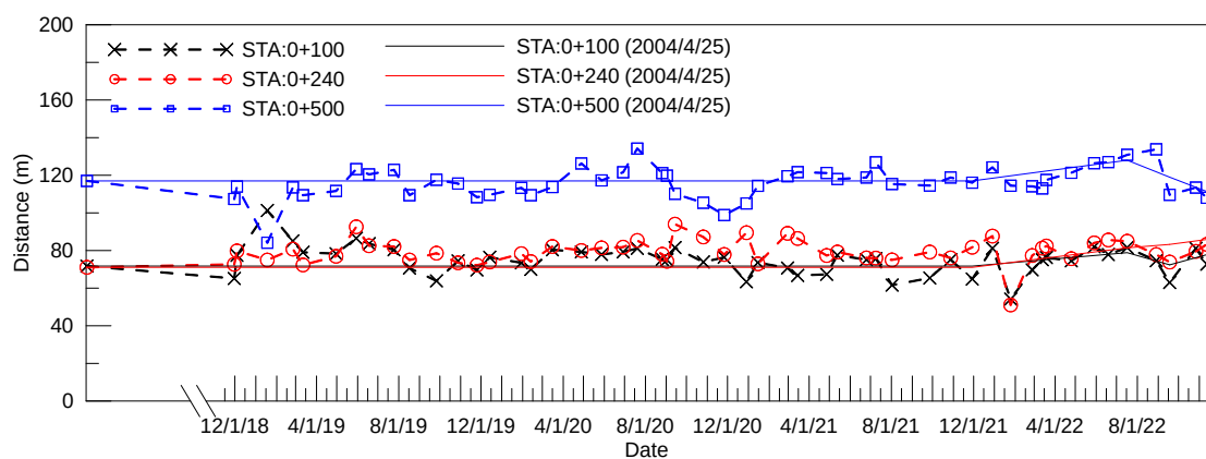
圖 4-21 岸線斷面沙灘寬度變化圖(2022/11/12)
