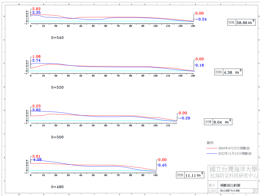
圖 4-4(d) 2022 年 11 月 12 日 A 監測區橫斷面比較圖
