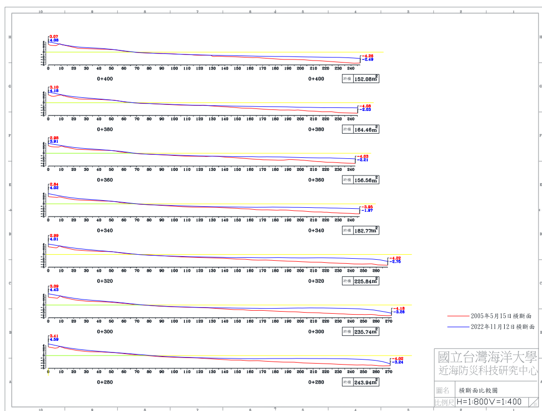
圖 4-5(d) 2022 年 11 月 12 日 B 監測區橫斷面比較圖
