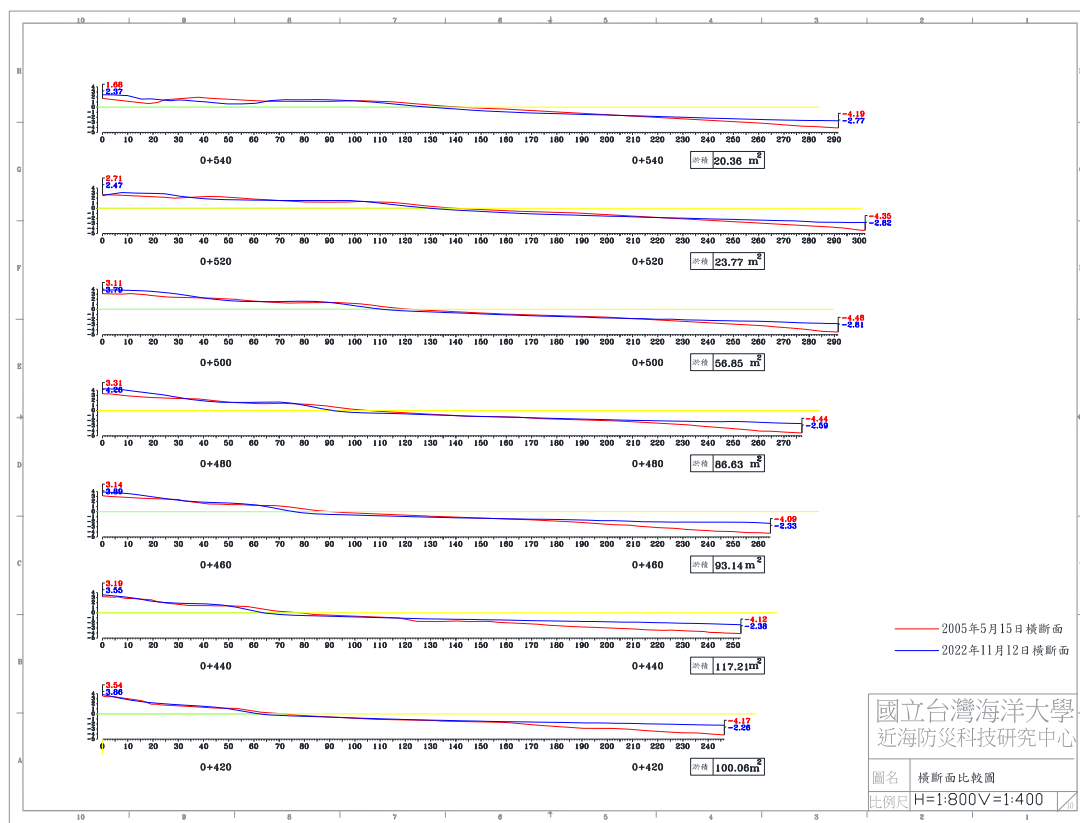
圖 4-5(c) 2022 年 11 月 12 日 B 監測區橫斷面比較圖
