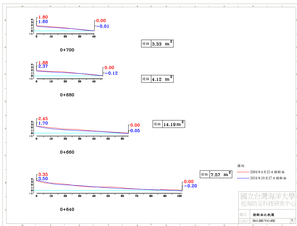
圖 4-4(b) 2016 年 10 月 27 日 A 監測區橫断面比較圖
