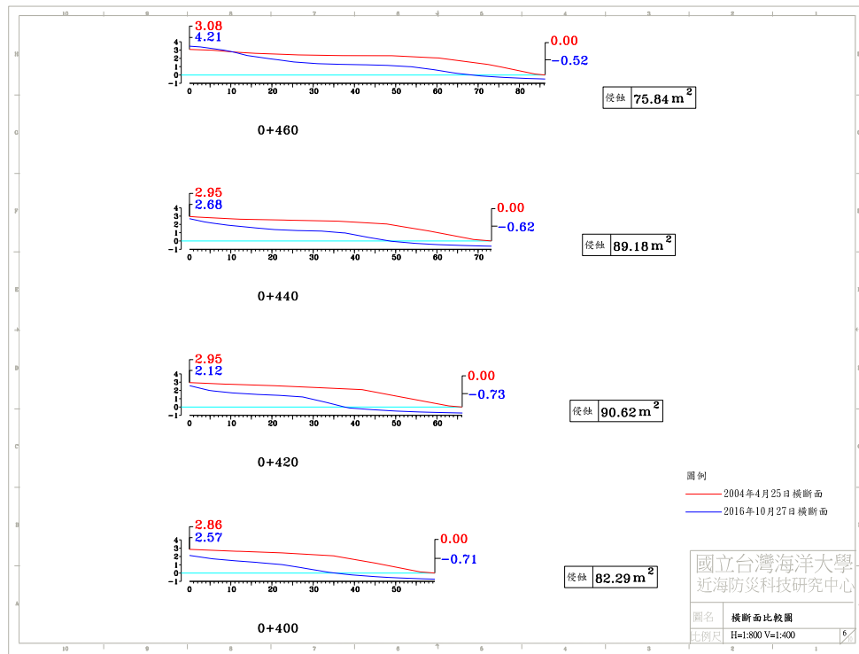
圖 4-4(e) 2016 年 10 月 27 日 A 監測區橫断面比較圖
