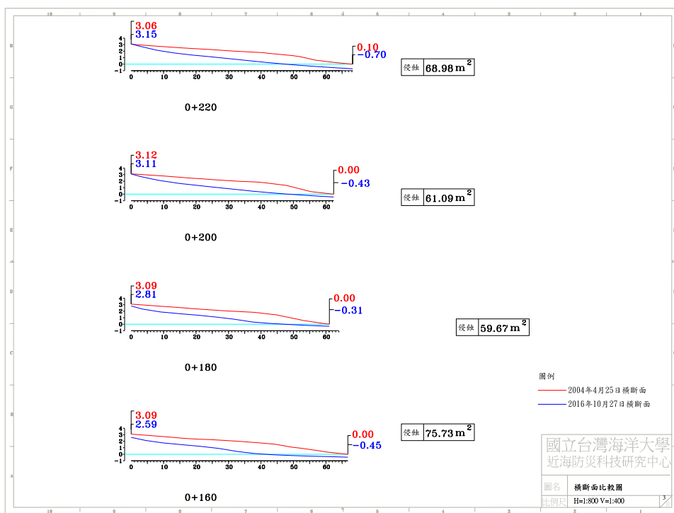
圖 4-4(h) 2016 年 10 月 27 日 A 監測區橫断面比較圖
