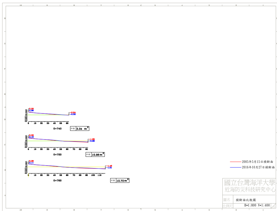
圖 4-5(a) 2016 年 10 月 27 日 B 監測區橫斷面比較圖
