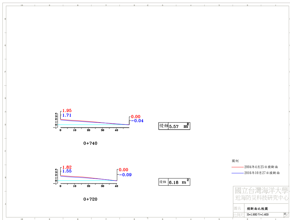
圖 4-4(a) 2016 年 10 月 27 日 A 監測區橫断面比較圖
