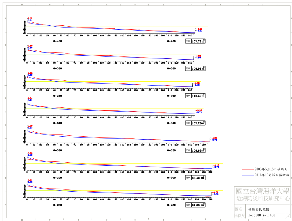
圖 4-5(d) 2016 年 10 月 27 日 B 監測區橫斷面比較圖
