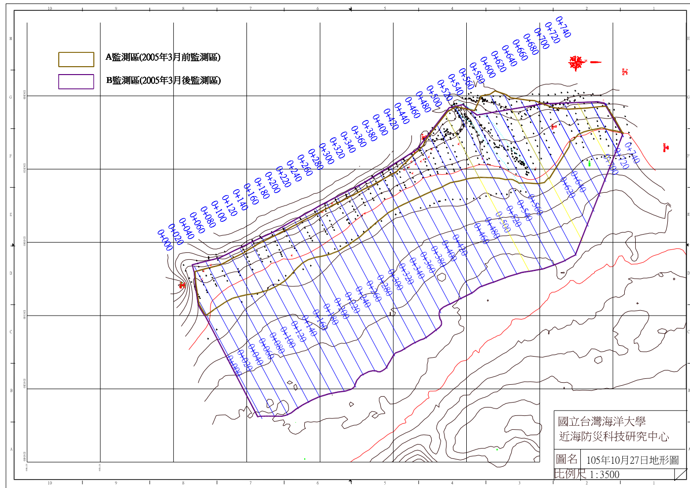
圖 4-1 2016 年 10 月 27 日監測地形圖
