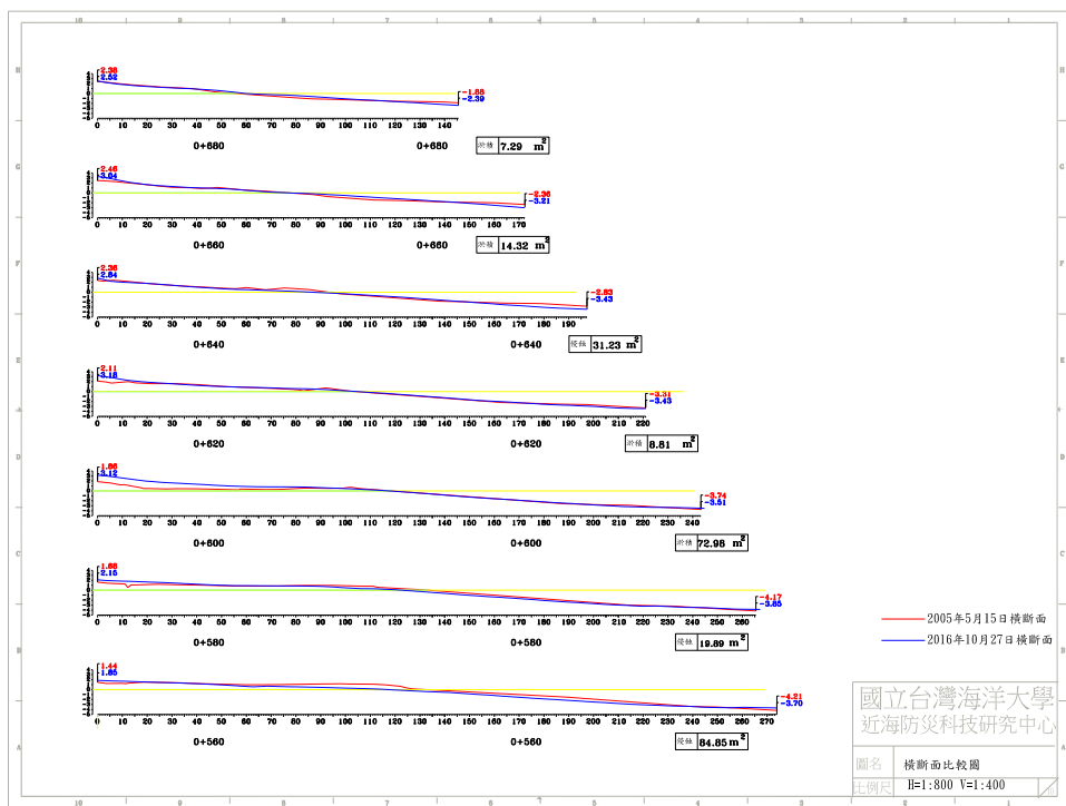
圖 4-5(b) 2016 年 10 月 27 日 B 監測區橫斷面比較圖
