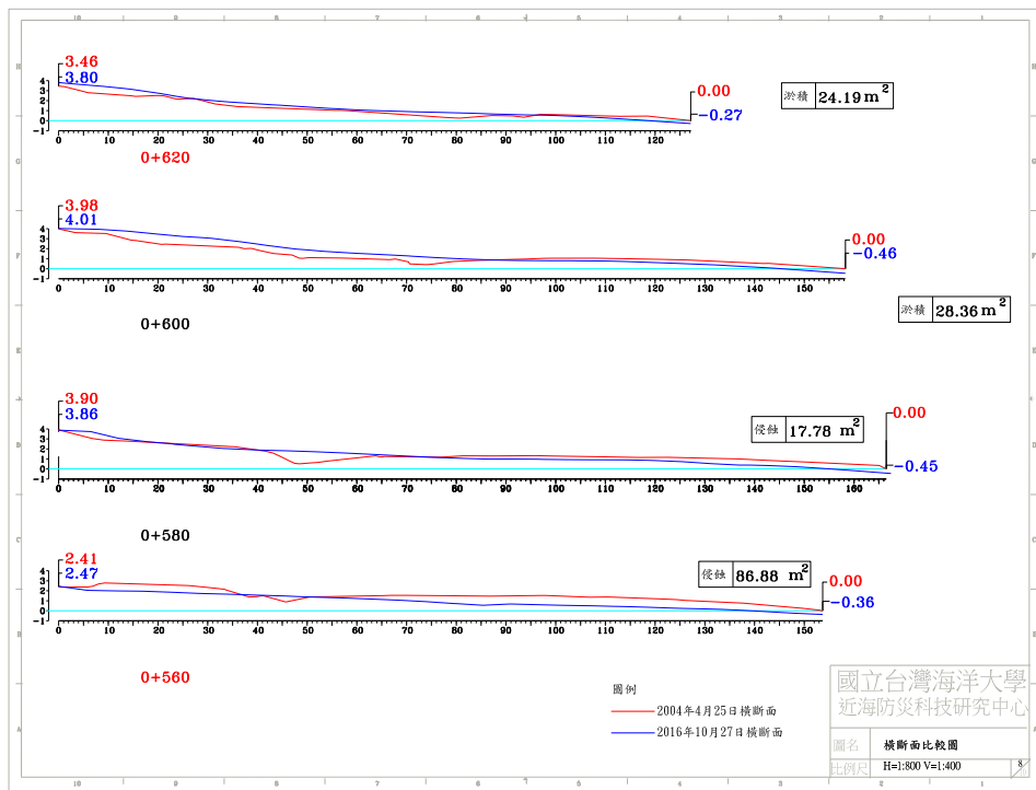
圖 4-4(c) 2016 年 10 月 27 日 A 監測區橫斷面比較圖
