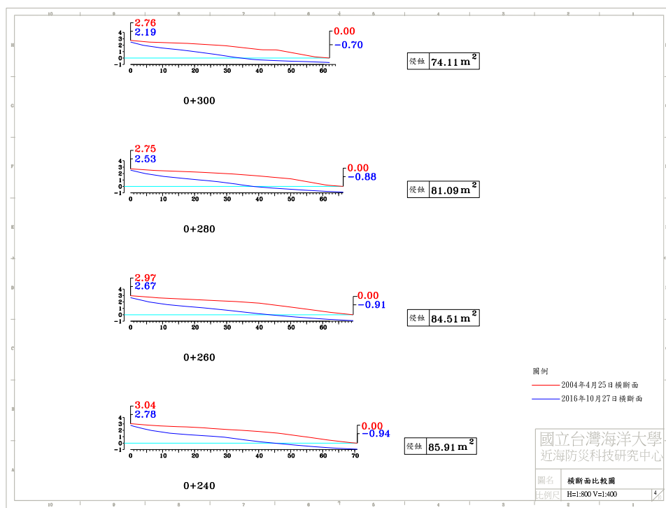
圖 4-4(g) 2016 年 10 月 27 日 A 監測區橫断面比較圖
