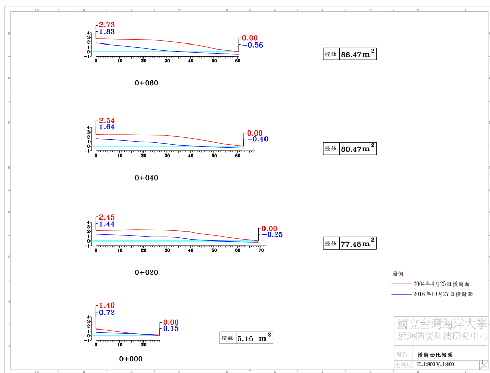
圖 4-4(j) 2016 年 10 月 27 日 A 監測區橫断面比較圖
