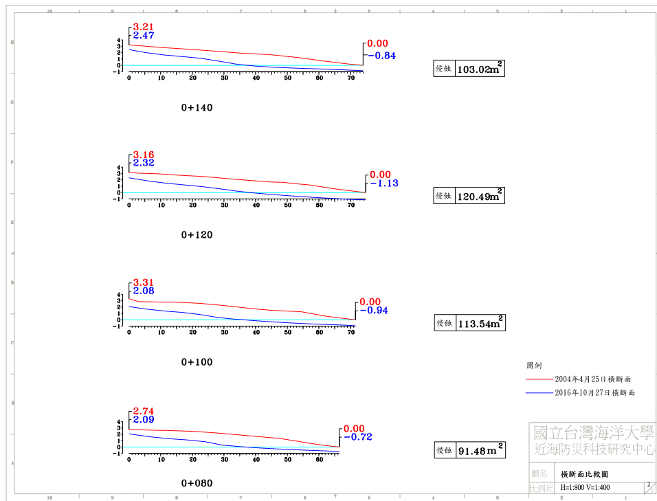
圖 4-4(i) 2016 年 10 月 27 日 A 監測區橫断面比較圖
