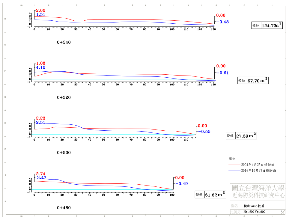
圖 4-4(d) 2016 年 10 月 27 日 A 監測區橫斷面比較圖
