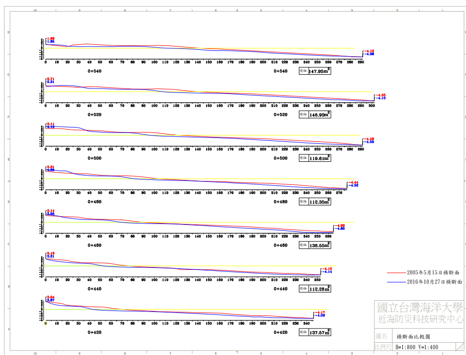
圖 4-5(c) 2016 年 10 月 27 日 B 監測區橫斷面比較圖
