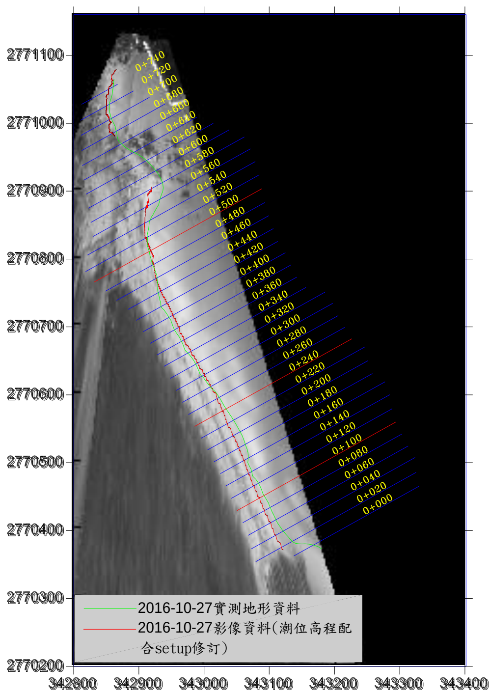
圖 3-22 水位線分析結果圖(2016/10/27)
