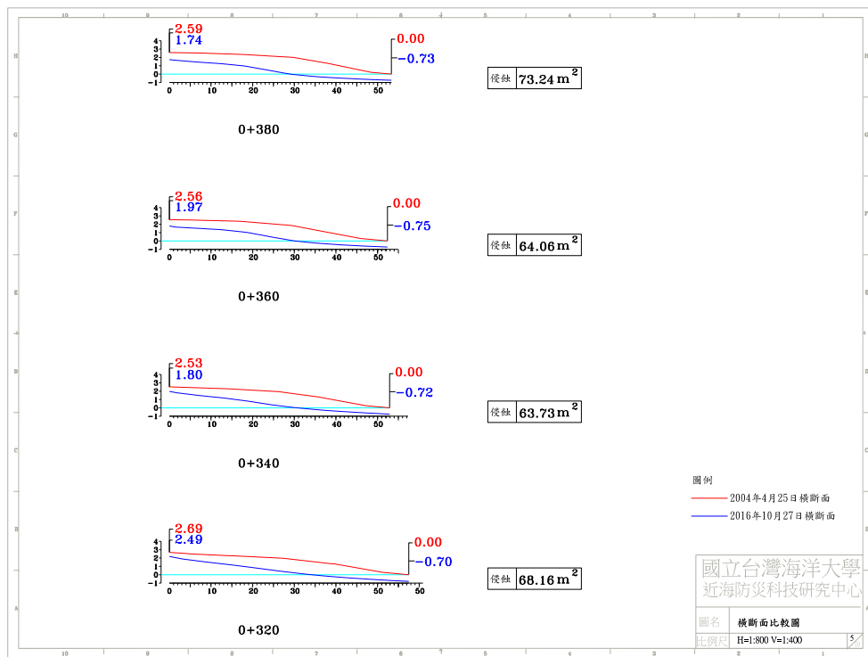
圖 4-4(f) 2016 年 10 月 27 日 A 監測區橫断面比較圖
