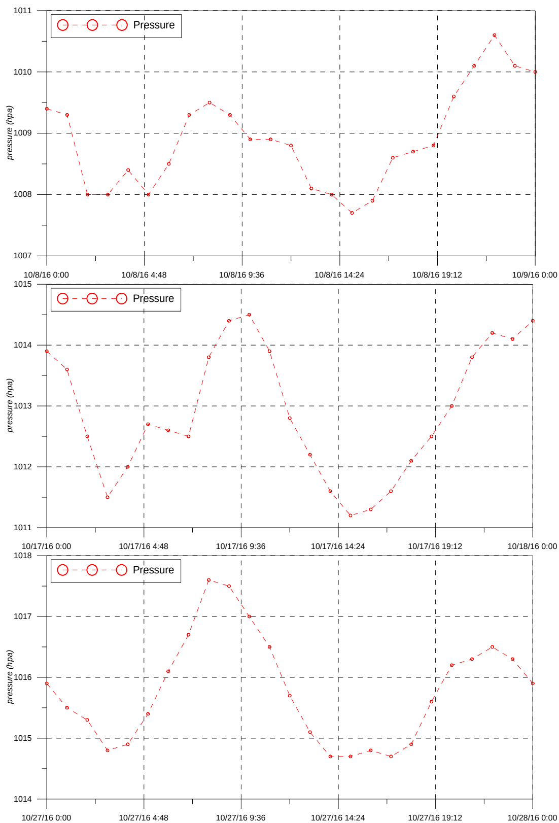
圖 2-5 壓力時序列變化圖
