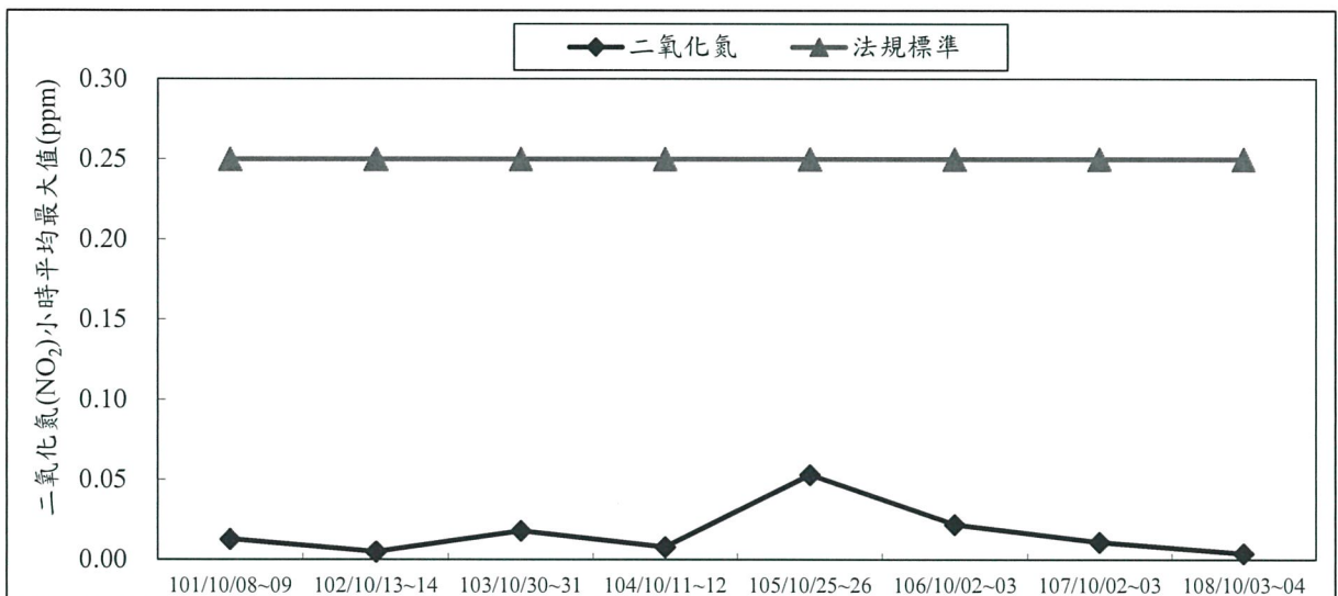
圖 3.1-4 歷年同期二氧化氮( \text{NO}_2 )小時平均最大值監測成果彙整
