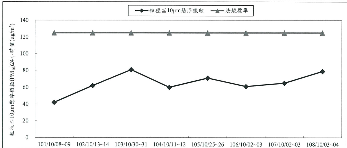
圖 3.1-3 歷年同期粒徑 \leq 10\mu\text{m} 之懸浮微粒( \text{PM}_{10} )日平均值監測成果彙整
