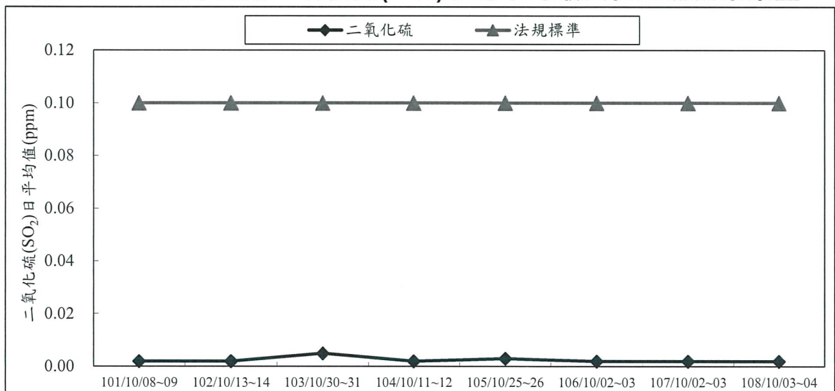
圖 3.1-5 歷年同期二氧化硫( \text{SO}_2 )日平均值監測成果彙整
