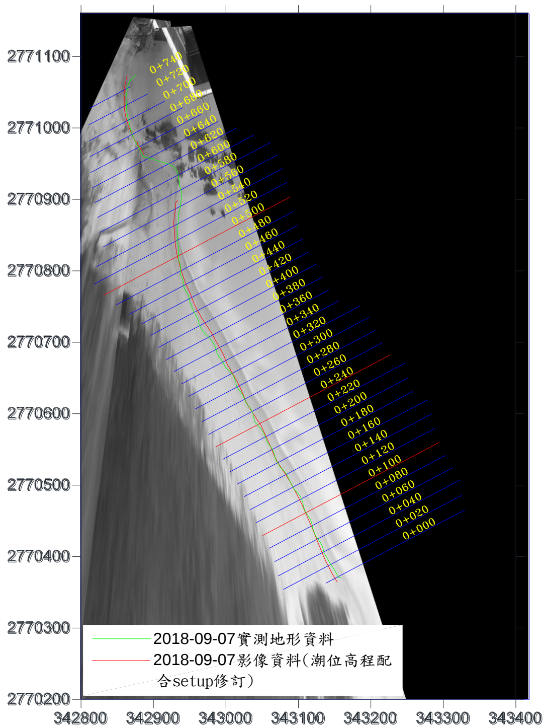
圖 3-22 水位線分析結果圖(2018/9/07)
