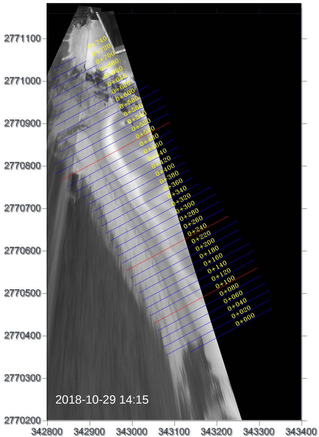
圖 4-14 鹽寮海岸地形影像全景圖(2018/10/29 14:15)
