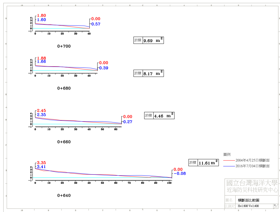
圖 4-4(b) 2016 年 7 月 4 日 A 監測區橫斷面比較圖
