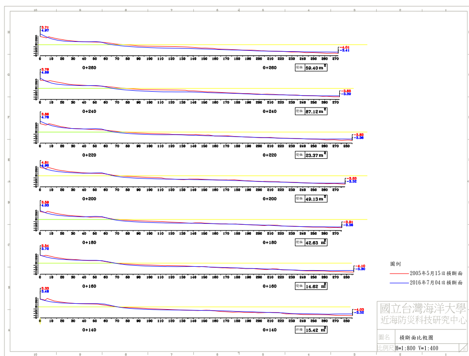
圖 4-5(e) 2016 年 7 月 4 日 B 監測區橫斷面比較圖
