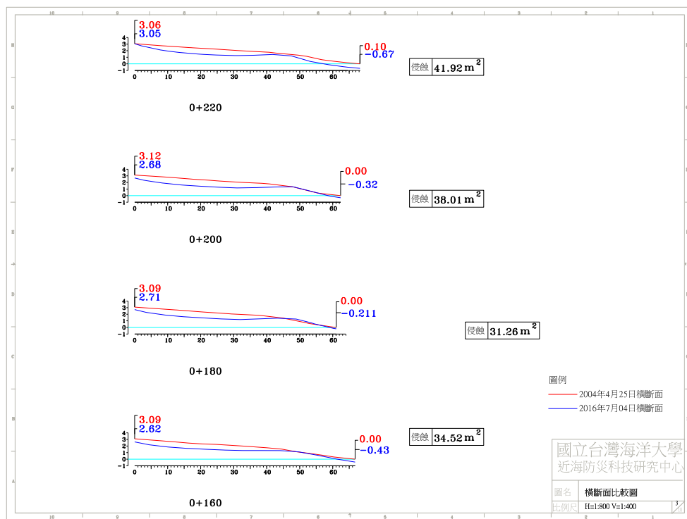
圖 4-4(h) 2016 年 7 月 4 日 A 監測區橫斷面比較圖
