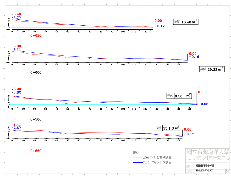
圖 4-4(c) 2016 年 7 月 4 日 A 監測區橫斷面比較圖
