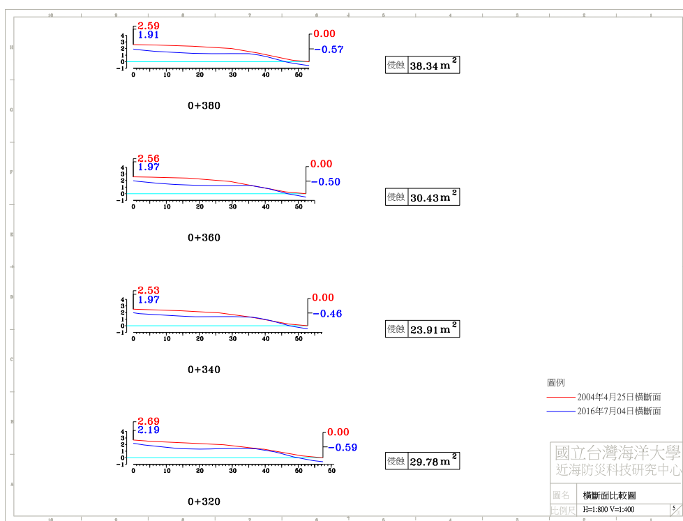
圖 4-4(f) 2016 年 7 月 4 日 A 監測區橫斷面比較圖
