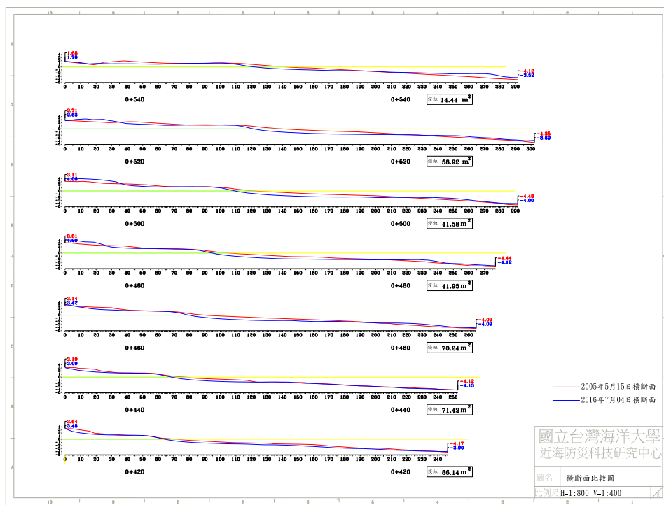
圖 4-5(c) 2016 年 7 月 4 日 B 監測區橫斷面比較圖
