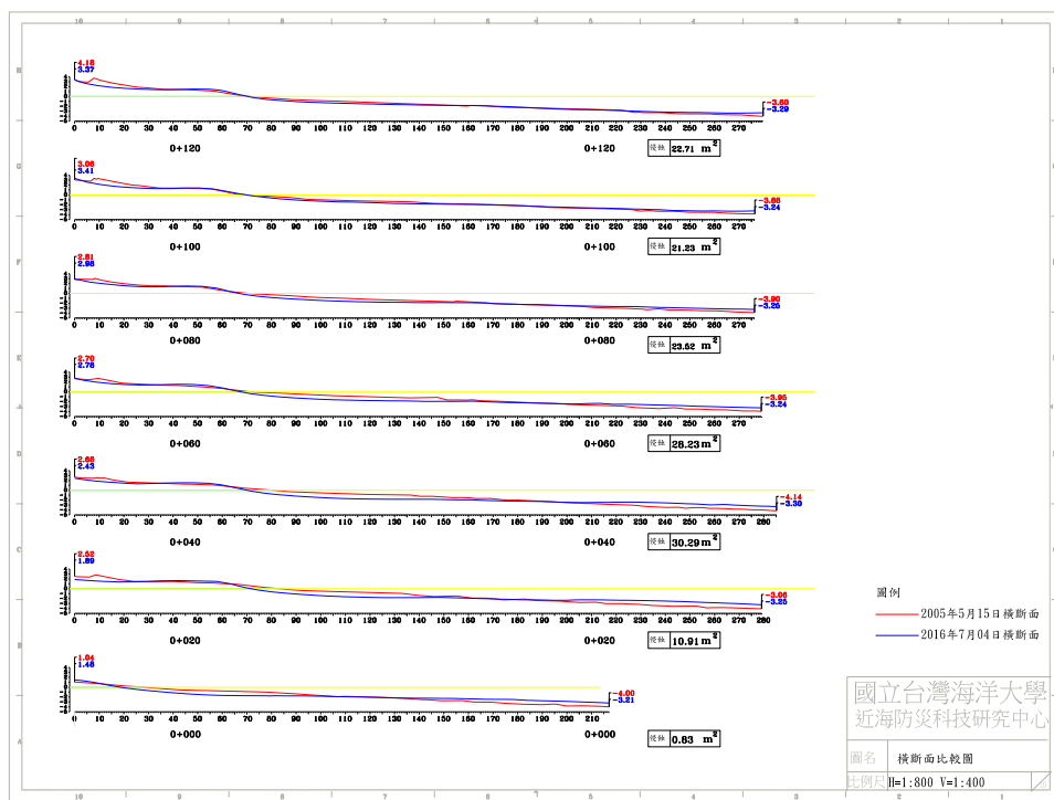
圖 4-5(f) 2016 年 7 月 4 日 B 監測區橫斷面比較圖
