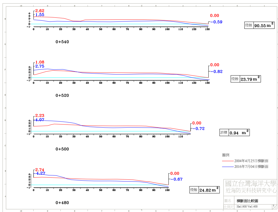
圖 4-4(d) 2016 年 7 月 4 日 A 監測區橫斷面比較圖
