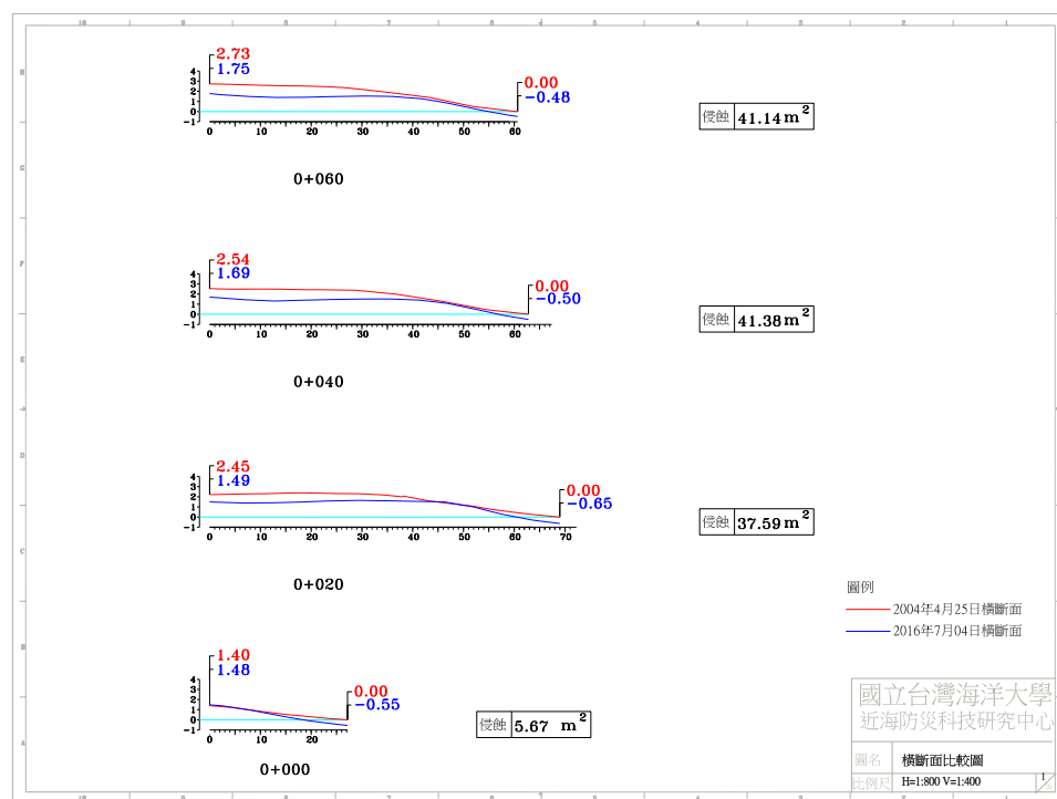
圖 4-4(j) 2016 年 7 月 4 日 A 監測區橫斷面比較圖
