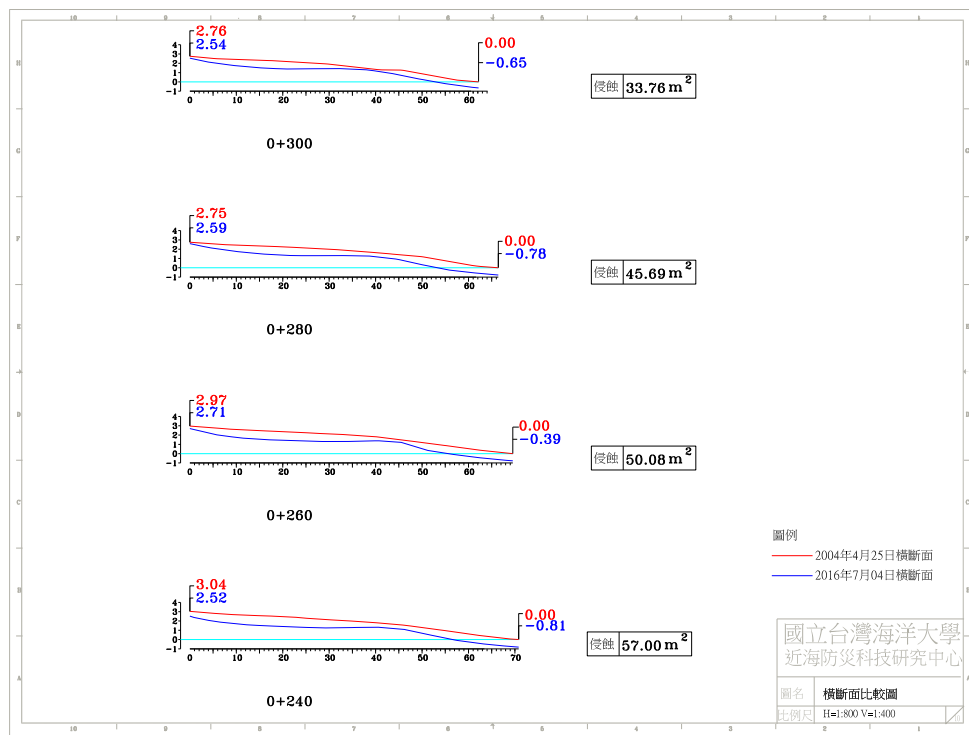
圖 4-4(g) 2016 年 7 月 4 日 A 監測區橫斷面比較圖
