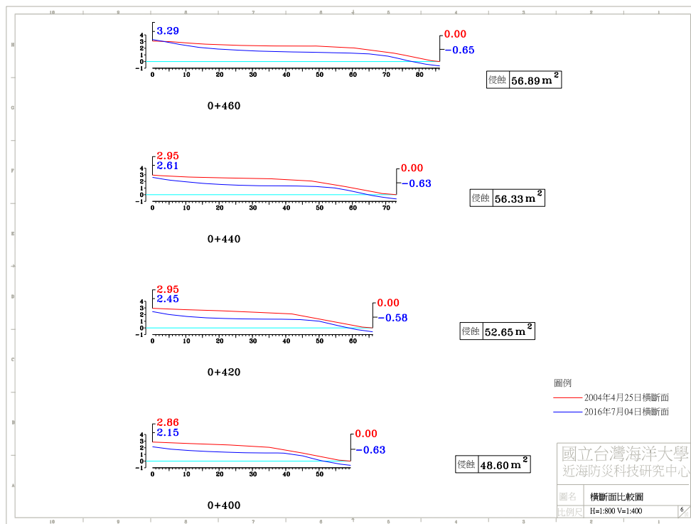
圖 4-4(e) 2016 年 7 月 4 日 A 監測區橫斷面比較圖
