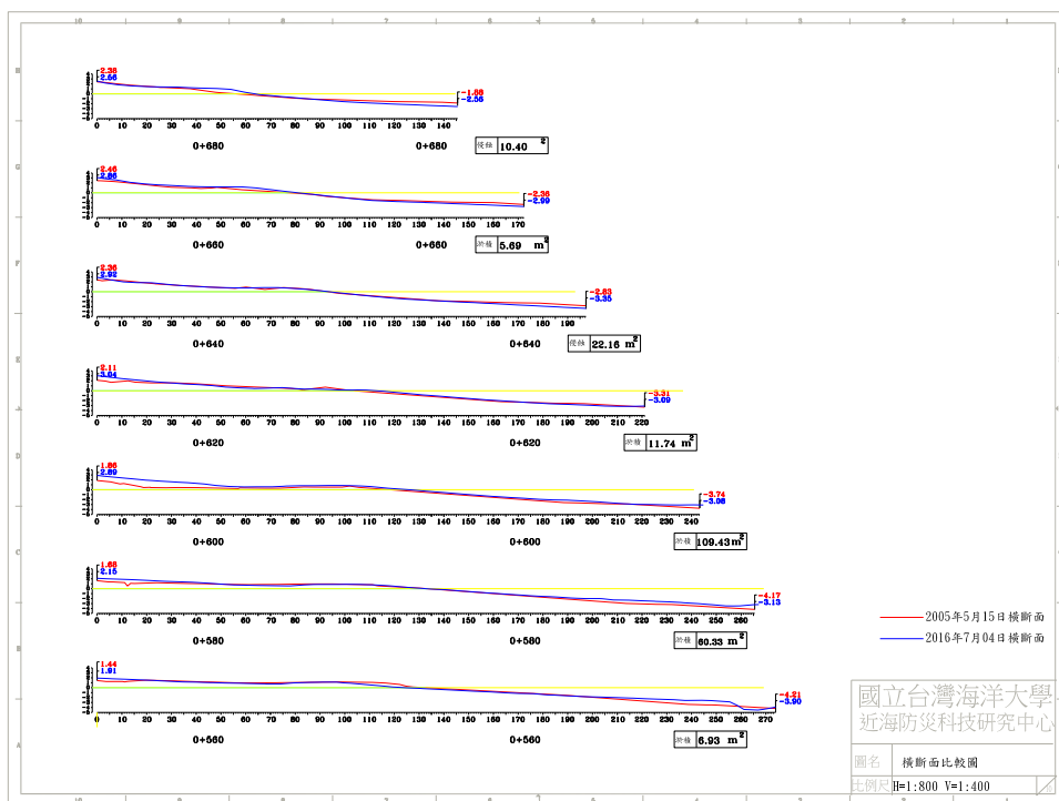
圖 4-5(b) 2016 年 7 月 4 日 B 監測區橫断面比較圖
