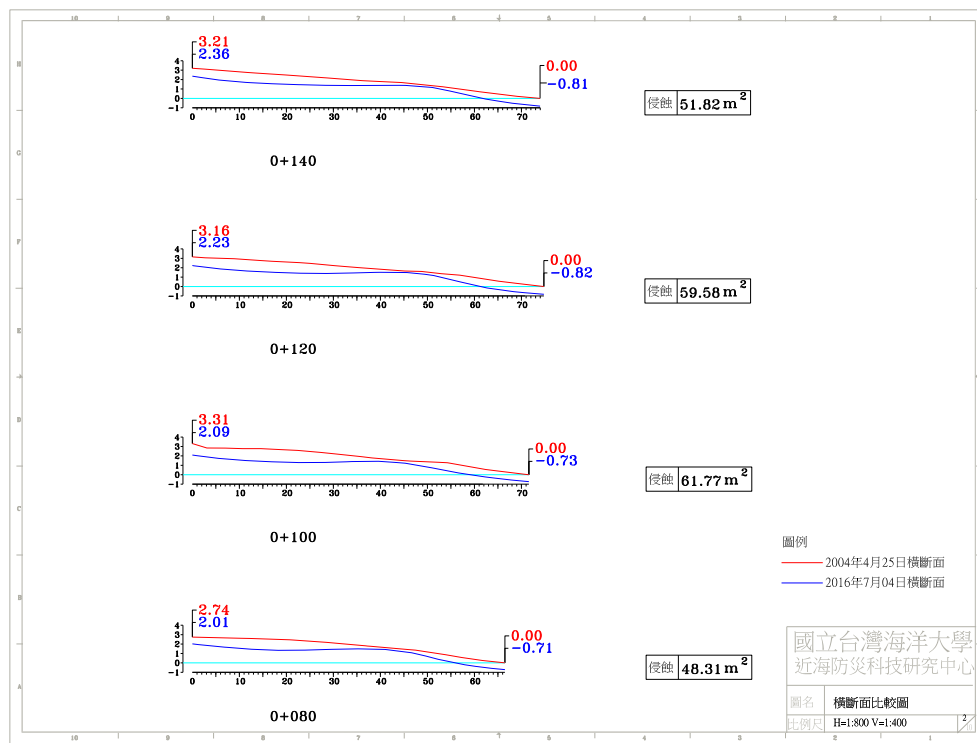
圖 4-4(i) 2016 年 7 月 4 日 A 監測區橫斷面比較圖
