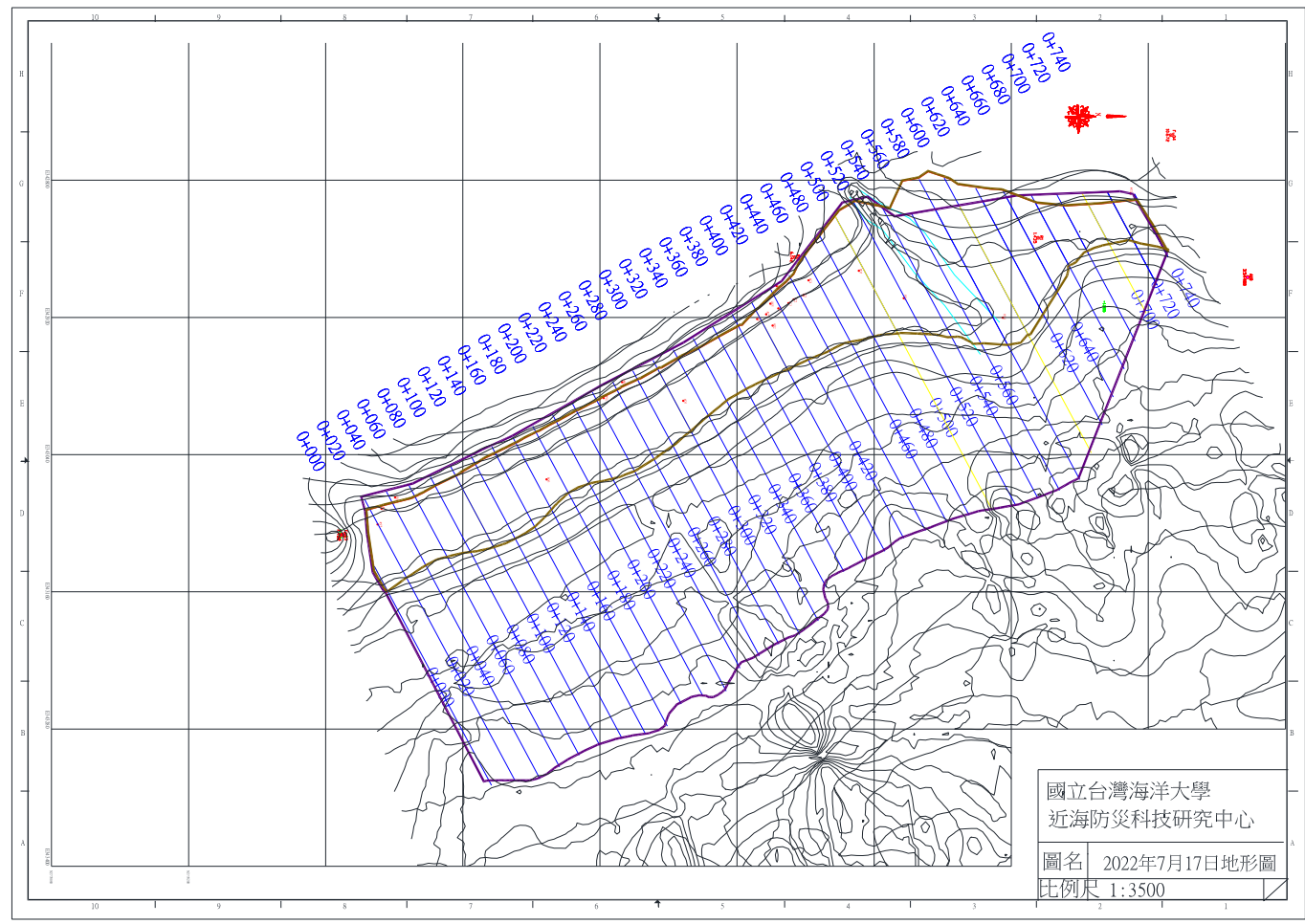
圖 4-1 2022 年 7 月 17 日監測地形
