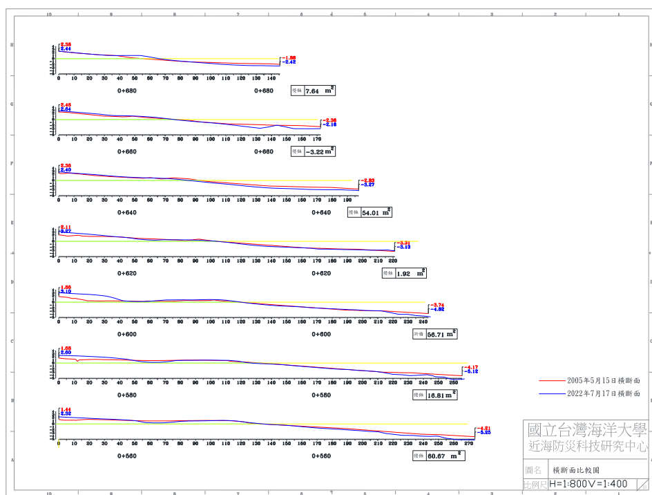
圖 4-5(b) 2022 年 7 月 17 日 B 監測區橫斷面比較圖
