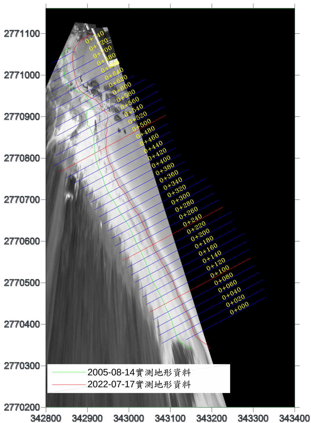
圖 4-22 長期實測 0 m 灘線比對平面示意圖(2022/07/17)
