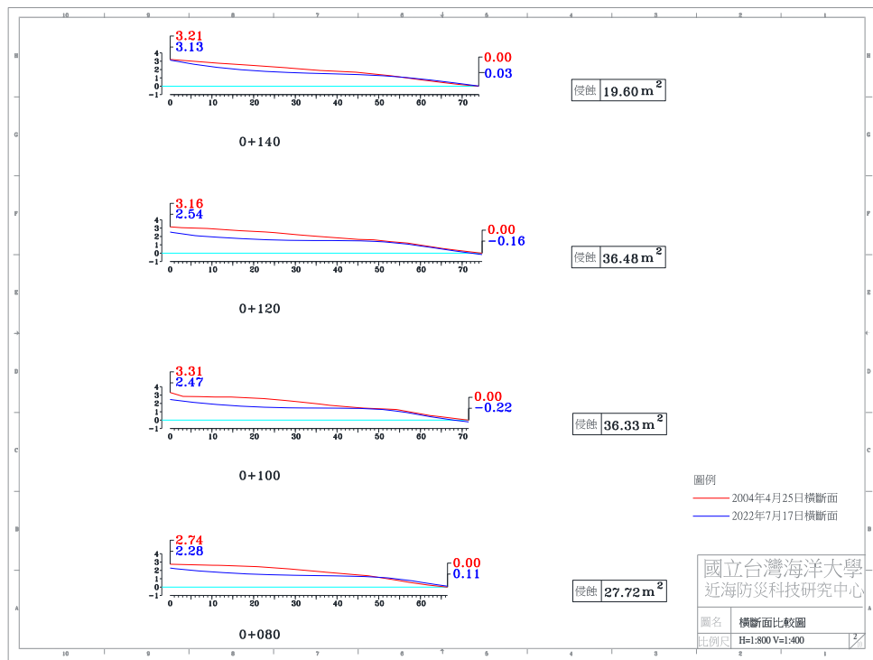
圖 4-4(i) 2022 年 7 月 17 日 A 監測區橫斷面比較圖
