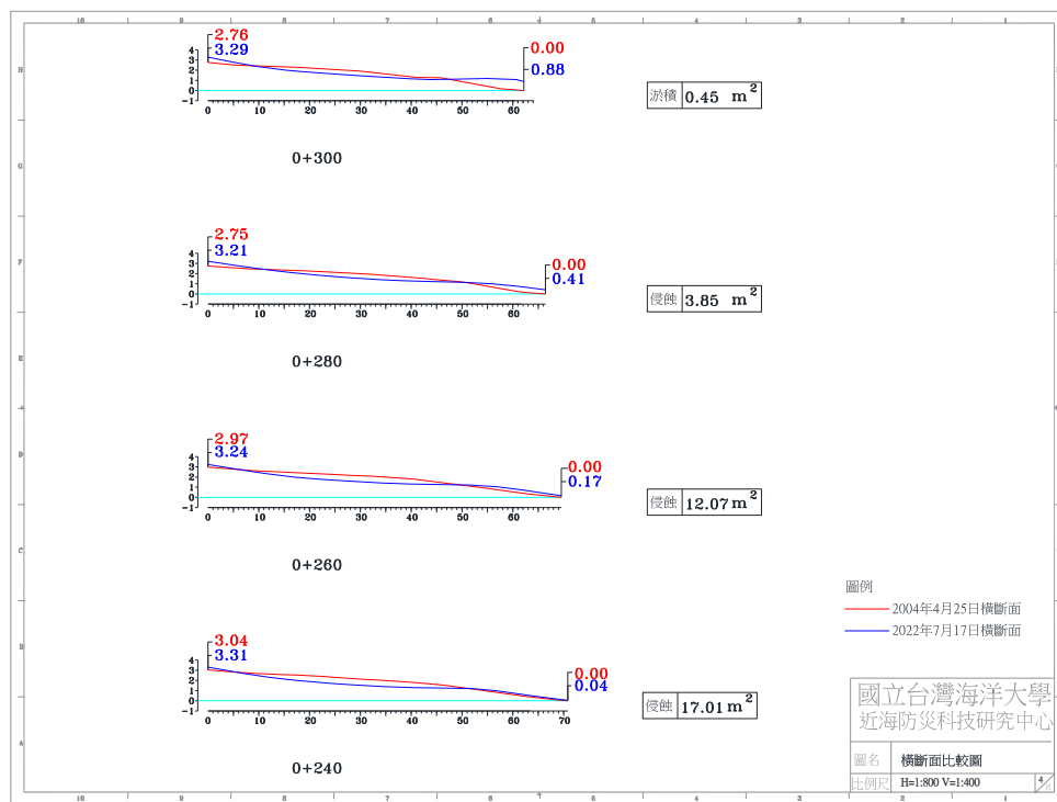
圖 4-4(g) 2022 年 7 月 17 日 A 監測區橫斷面比較圖
