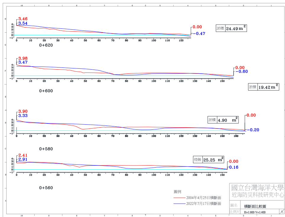
圖 4-4(c) 2022 年 7 月 17 日 A 監測區橫斷面比較圖
