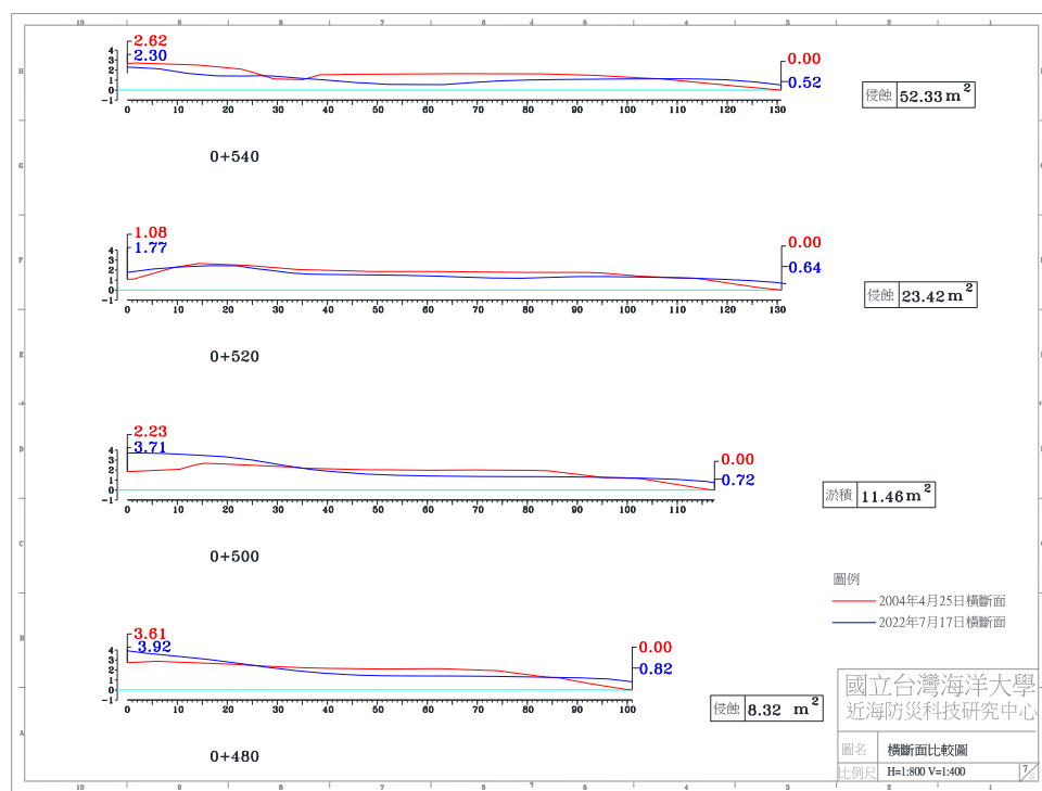
圖 4-4(d) 2022 年 7 月 17 日 A 監測區橫斷面比較圖
