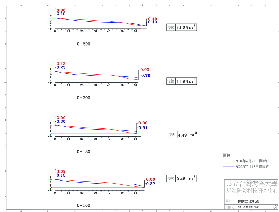
圖 4-4(h) 2022 年 7 月 17 日 A 監測區橫斷面比較圖
