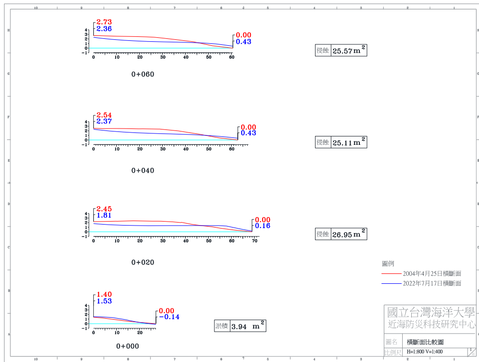
圖 4-4(j) 2022 年 7 月 17 日 A 監測區橫斷面比較圖
