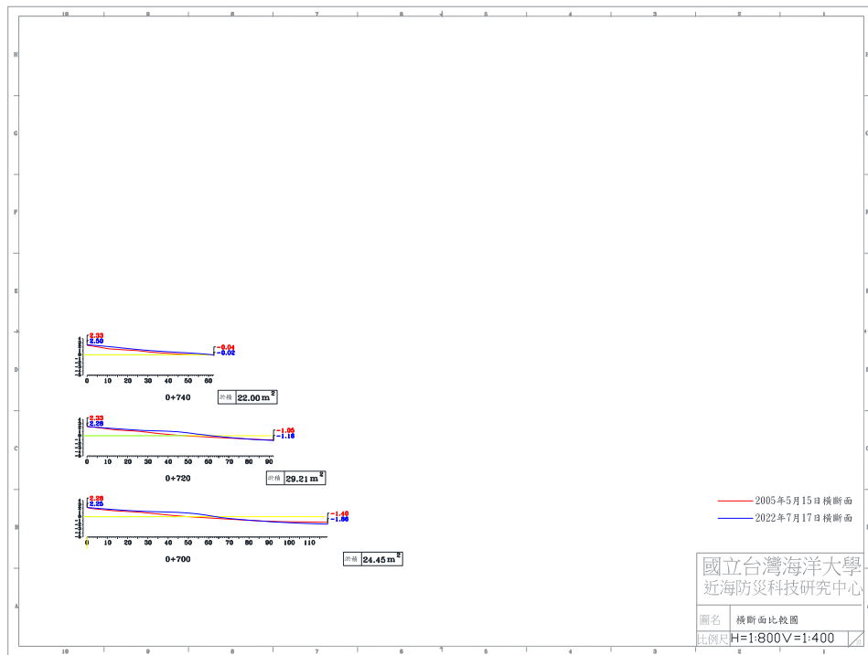
圖 4-5(a) 2022 年 7 月 17 日 B 監測區橫斷面比較圖
