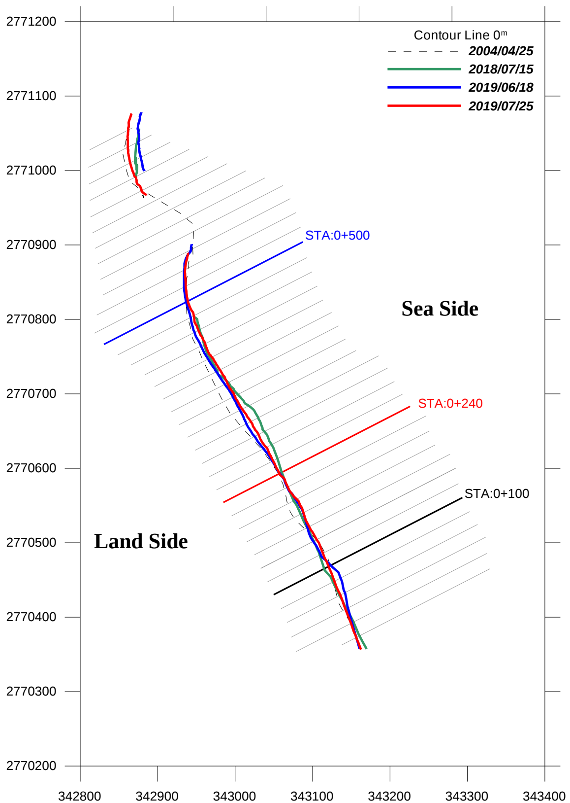
圖 4-20 鹽寮海岸線變遷分析比較圖
