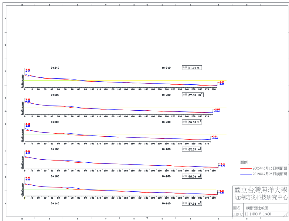
圖 4-5(e) 2019 年 7 月 25 日 B 監測區橫斷面比較圖
