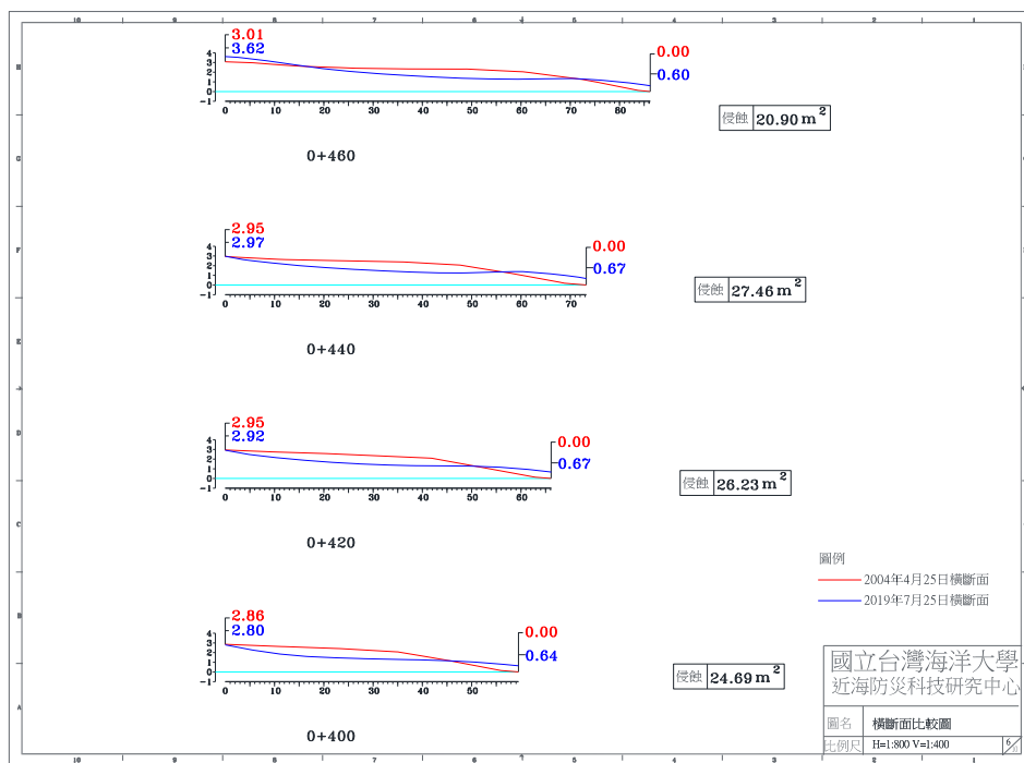
圖 4-4(e) 2019 年 7 月 25 日 A 監測區橫斷面比較圖
