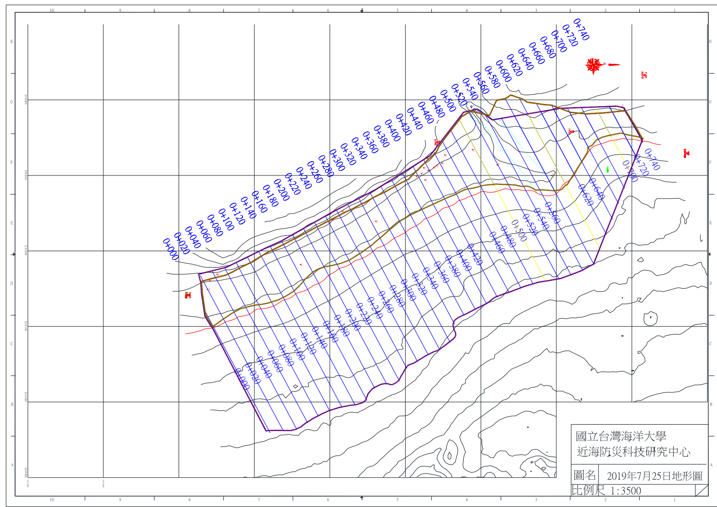
圖 4-1 2019 年 7 月 25 日監測地形圖
