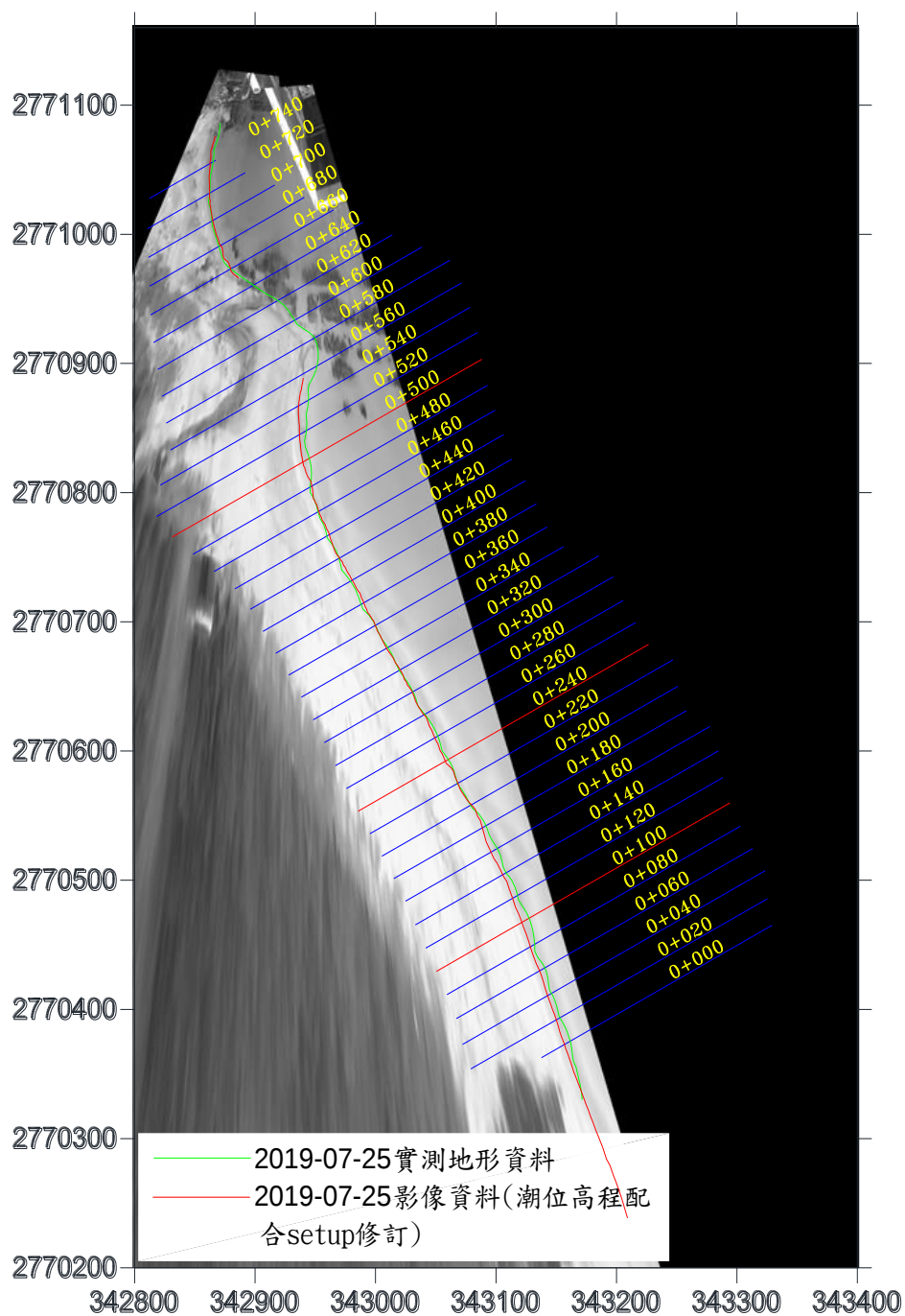
圖 3-22 水位線分析結果圖(2019/07/25)
