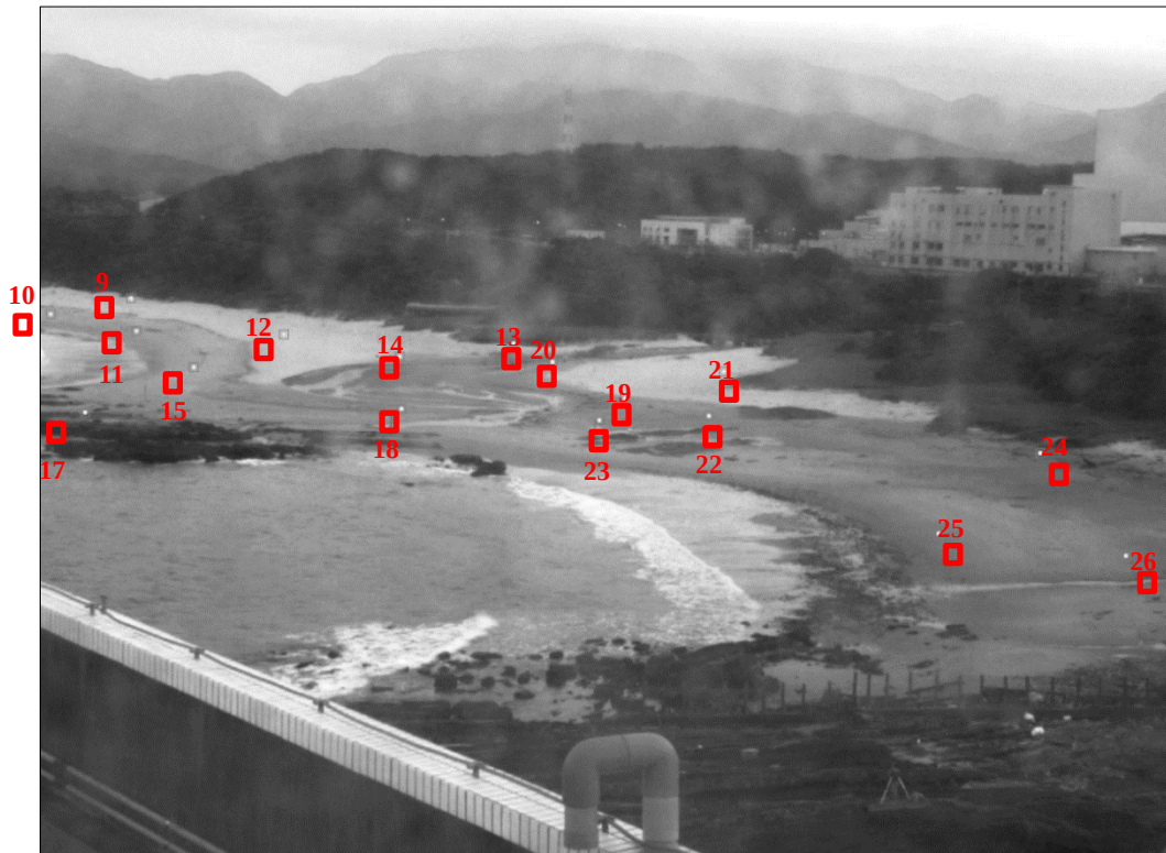
圖 3-21 視角 1(Cam1)地面控制點位置分佈圖例
