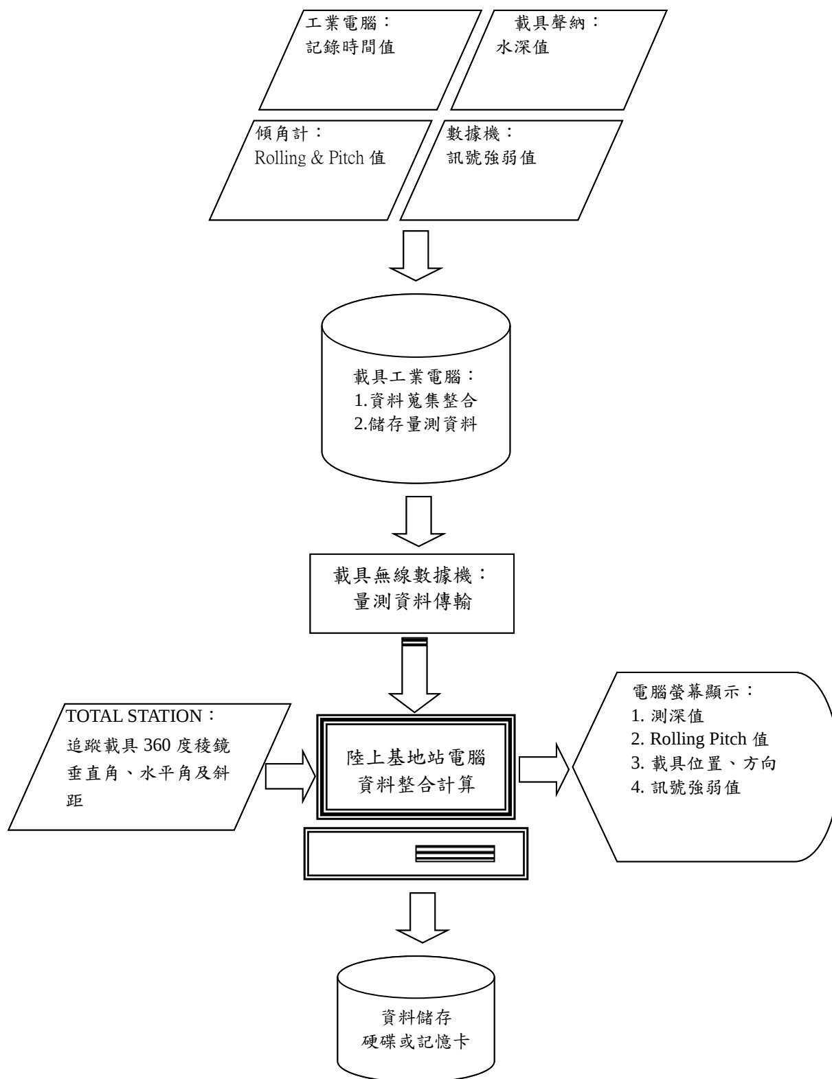
圖 3-4 量測系統資料處理流程圖
