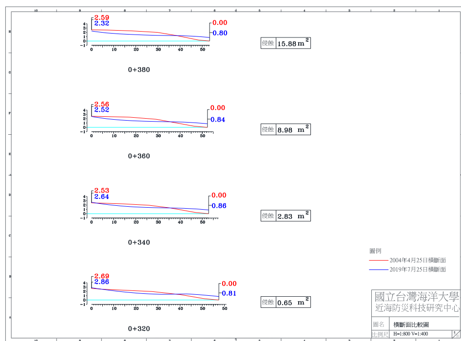
圖 4-4(f) 2019 年 7 月 25 日 A 監測區橫斷面比較圖
