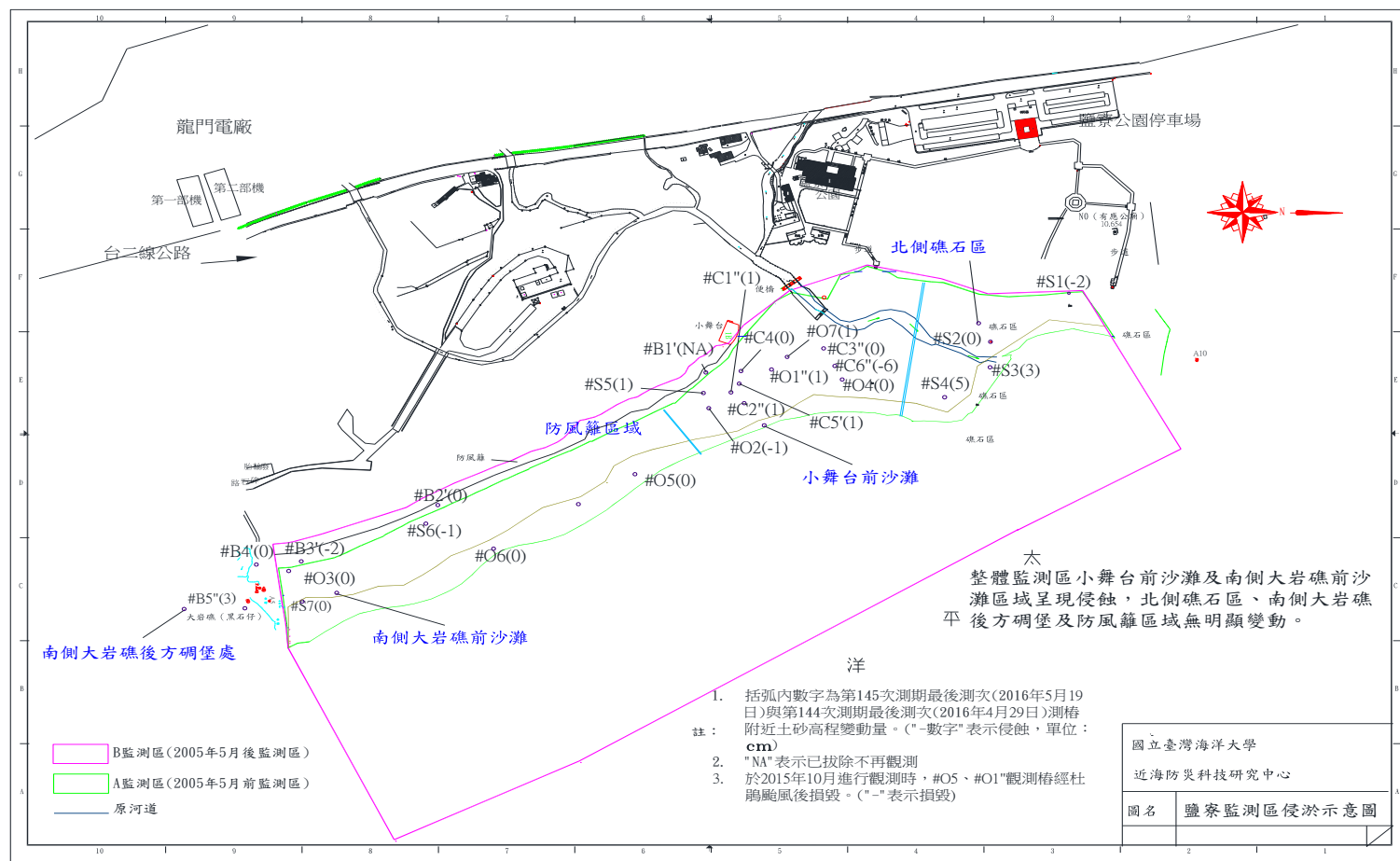
圖 1-1 鹽寮海岸短期性養灘監測各區域土砂高程變化圖
