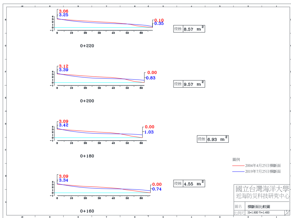
圖 4-4(h) 2019 年 7 月 25 日 A 監測區橫斷面比較圖
