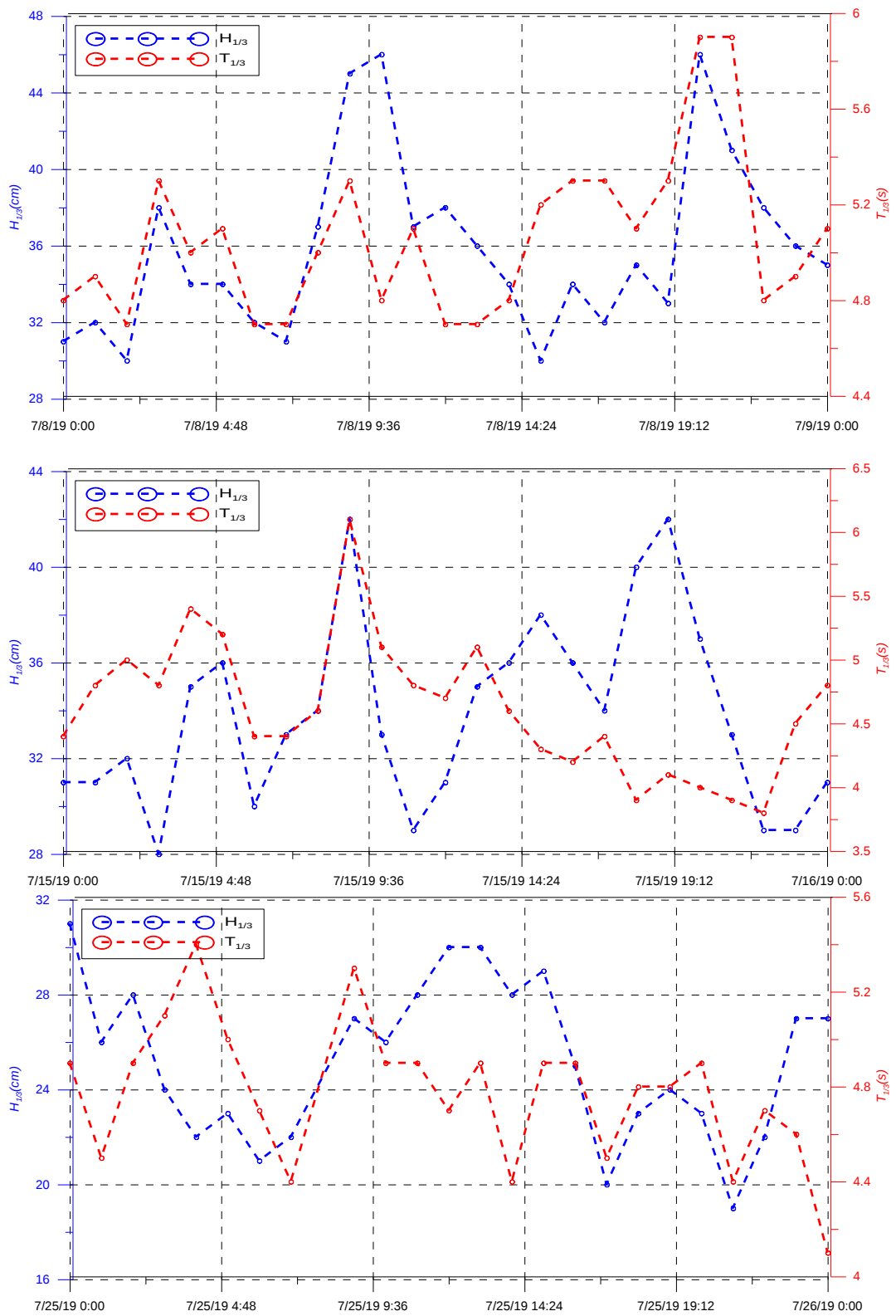
圖 2-3 波浪時序列變化圖
