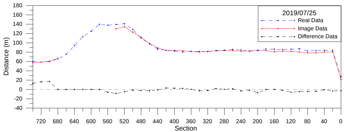
圖 3-23 海岸線分析比較圖(2019/7/25)
