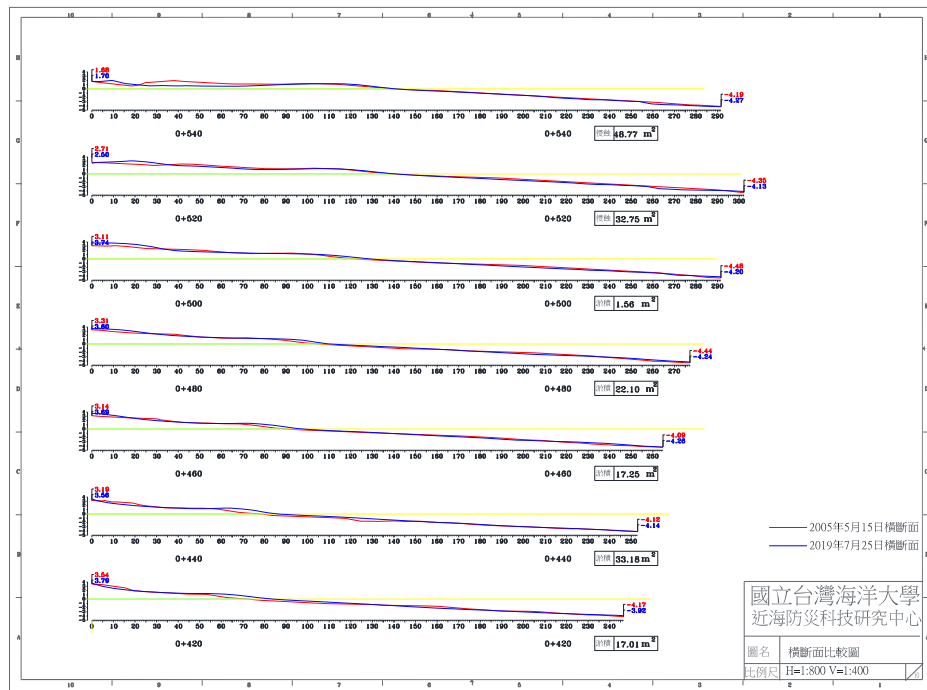
圖 4-5(c) 2019 年 7 月 25 日 B 監測區橫斷面比較圖
