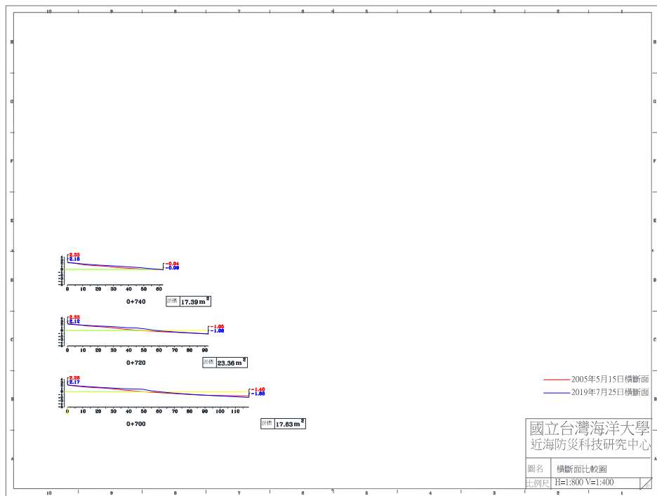
圖 4-5(a) 2019 年 7 月 25 日 B 監測區橫斷面比較圖
