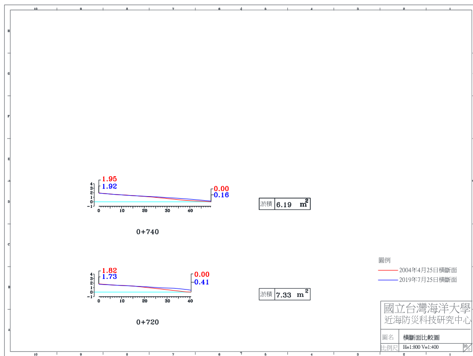
圖 4-4(a) 2019 年 7 月 25 日 A 監測區橫斷面比較圖
