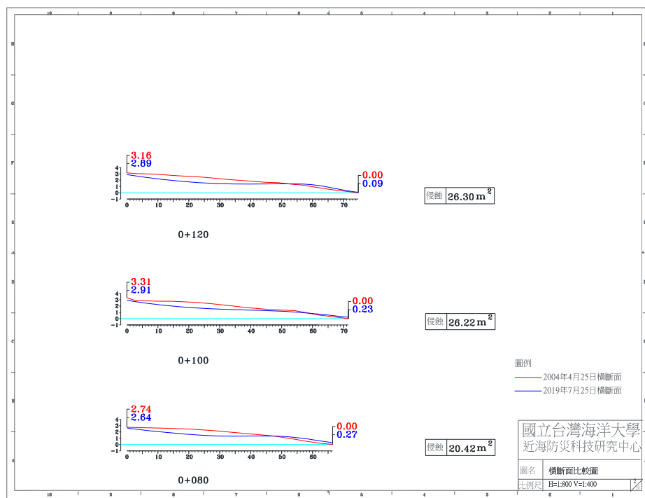
圖 4-4(i) 2019 年 7 月 25 日 A 監測區橫斷面比較圖
