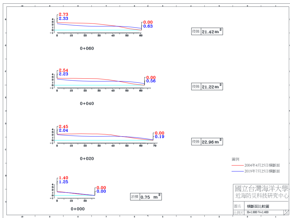
圖 4-4(j) 2019 年 7 月 25 日 A 監測區橫斷面比較圖
