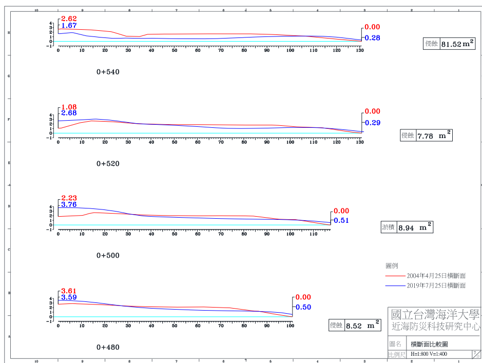
圖 4-4(d) 2019 年 7 月 25 日 A 監測區橫斷面比較圖
