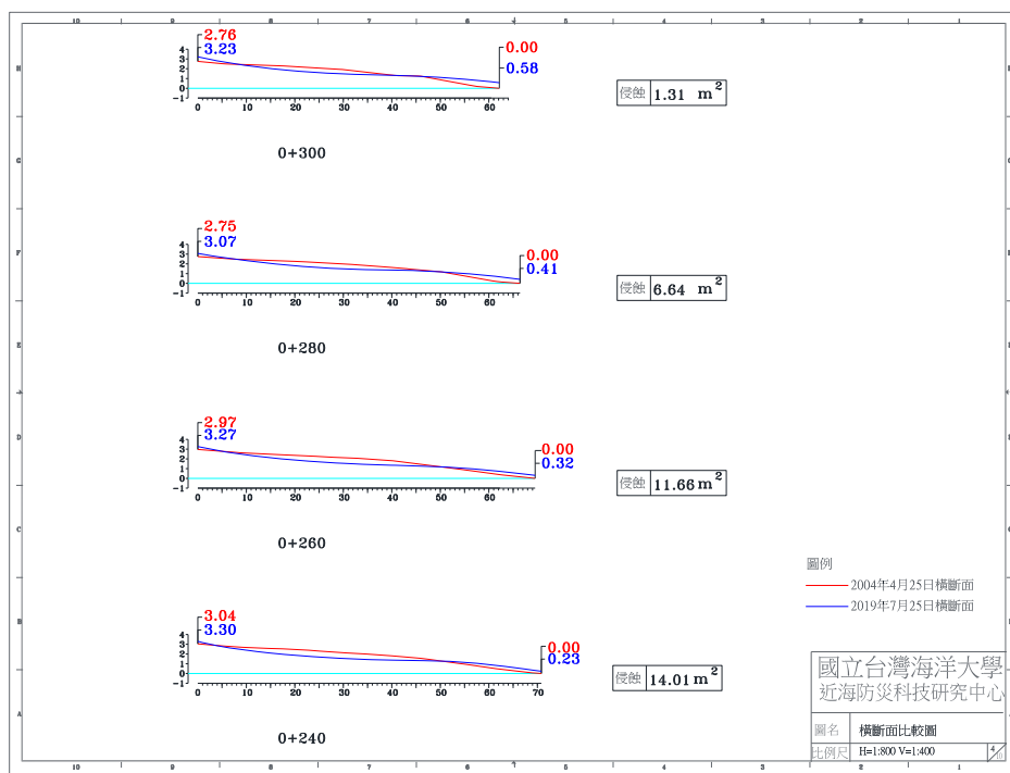
圖 4-4(g) 2019 年 7 月 25 日 A 監測區橫斷面比較圖
