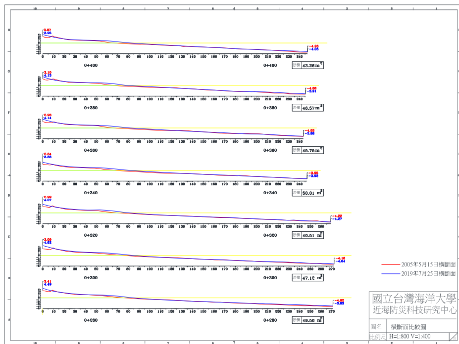
圖 4-5(d) 2019 年 7 月 25 日 B 監測區橫斷面比較圖
