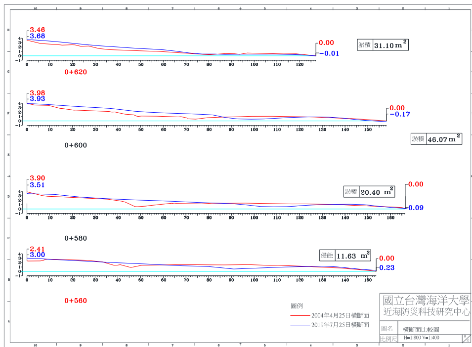
圖 4-4(c) 2019 年 7 月 25 日 A 監測區橫斷面比較圖
