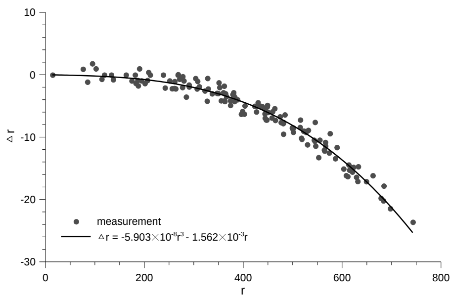
圖 3-19 攝影鏡頭編號 Cam2 之徑向扭曲迴歸結果圖
