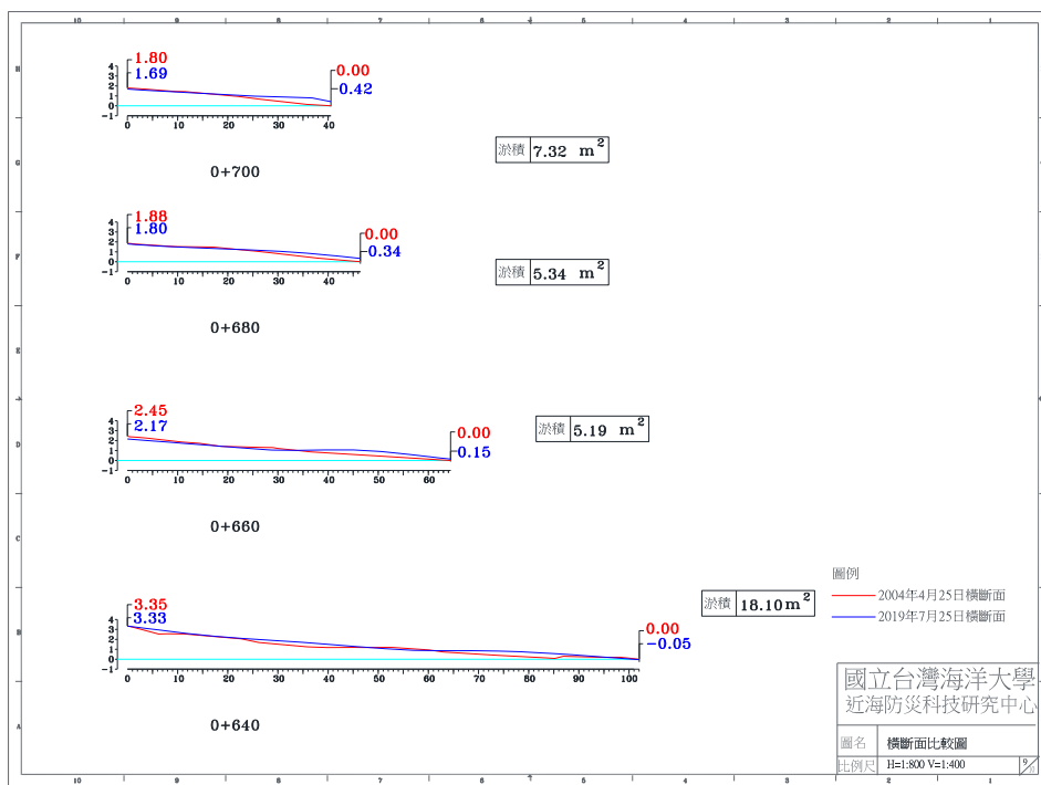
圖 4-4(b) 2019 年 7 月 25 日 A 監測區橫斷面比較圖
