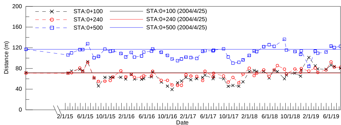
圖 4-21 岸線斷面沙灘寬度變化圖(斷面編號：0+100、0+240、0+500)
