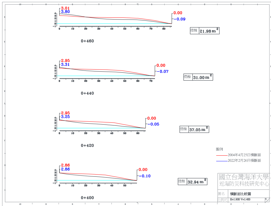
圖 4-4(e) 2022 年 2 月 26 日 A 監測區橫斷面比較圖
