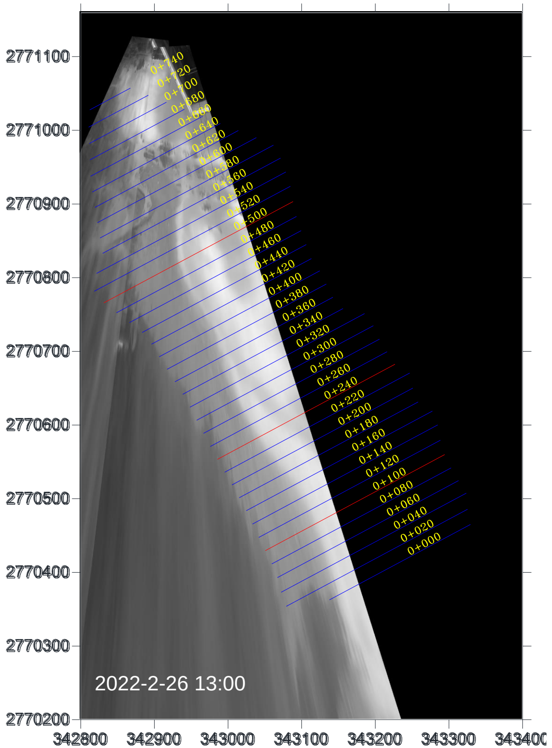
圖 4-19 鹽寮海岸地形影像全景圖(2022/02/26 13:00)
