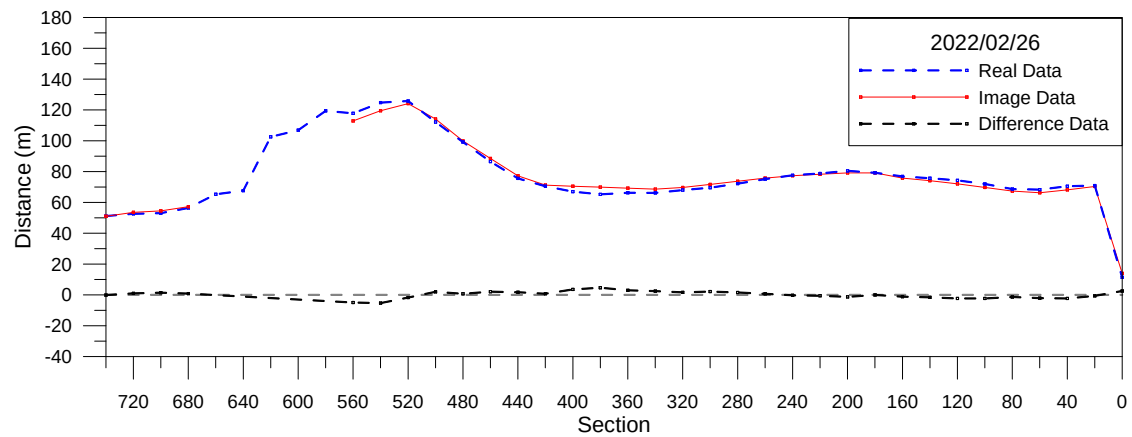
圖 3-23 海岸線分析比較圖(2022/02/26)
