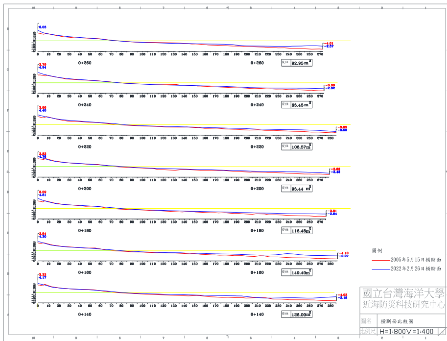
圖 4-5(e) 2022 年 2 月 26 日 B 監測區橫断面比較圖
