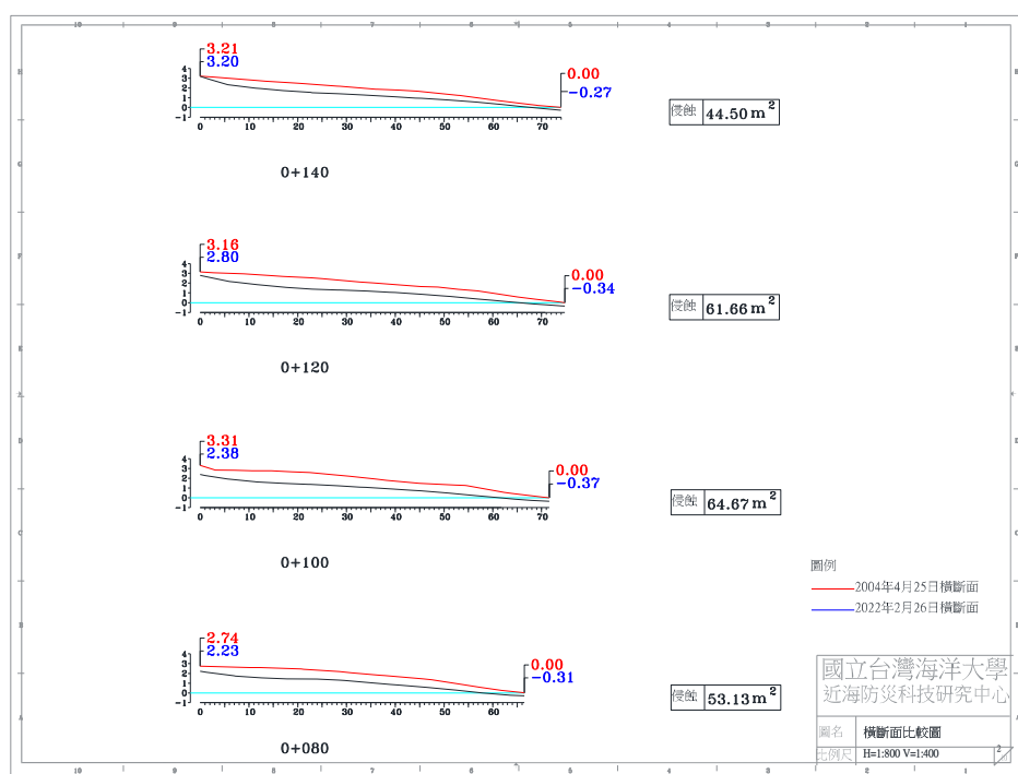
圖 4-4(i) 2022 年 2 月 26 日 A 監測區橫斷面比較圖
