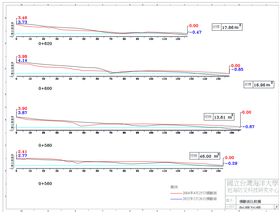
圖 4-4(c) 2022 年 2 月 26 日 A 監測區橫斷面比較圖
