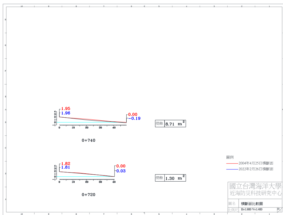
圖 4-4(a) 2022 年 2 月 26 日 A 監測區橫斷面比較圖
