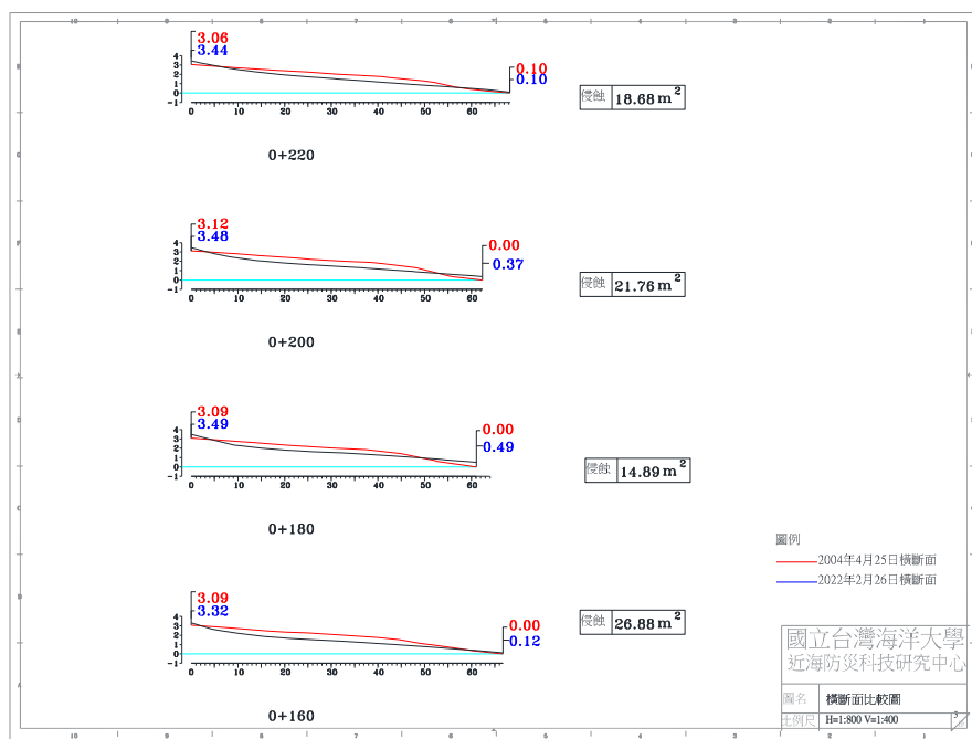
圖 4-4(h) 2022 年 2 月 26 日 A 監測區橫斷面比較圖
