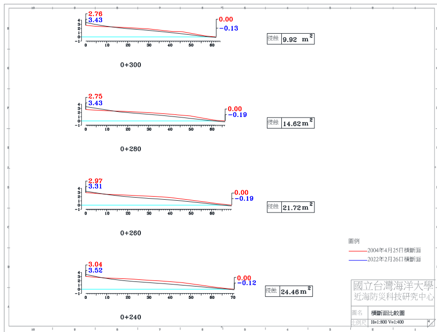
圖 4-4(g) 2022 年 2 月 26 日 A 監測區橫斷面比較圖
