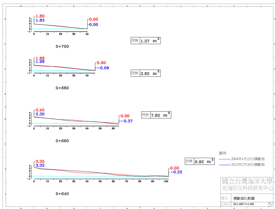
圖 4-4(b) 2022 年 2 月 26 日 A 監測區橫斷面比較圖
