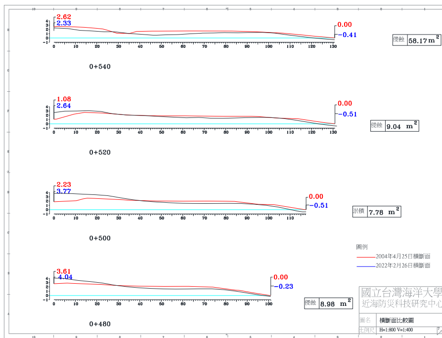
圖 4-4(d) 2022 年 2 月 26 日 A 監測區橫斷面比較圖
