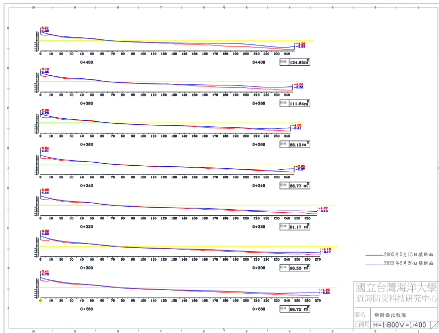
圖 4-5(d) 2022 年 2 月 26 日 B 監測區橫斷面比較圖
