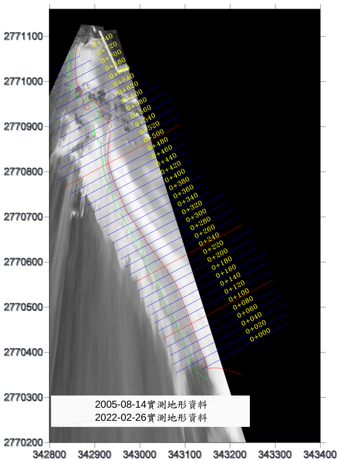
圖 4-22 實測地形水位線分析結果圖(2022/02/26)
