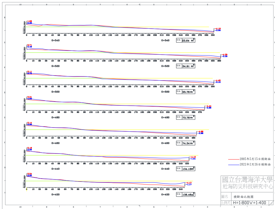
圖 4-5(c) 2022 年 2 月 26 日 B 監測區橫斷面比較圖
