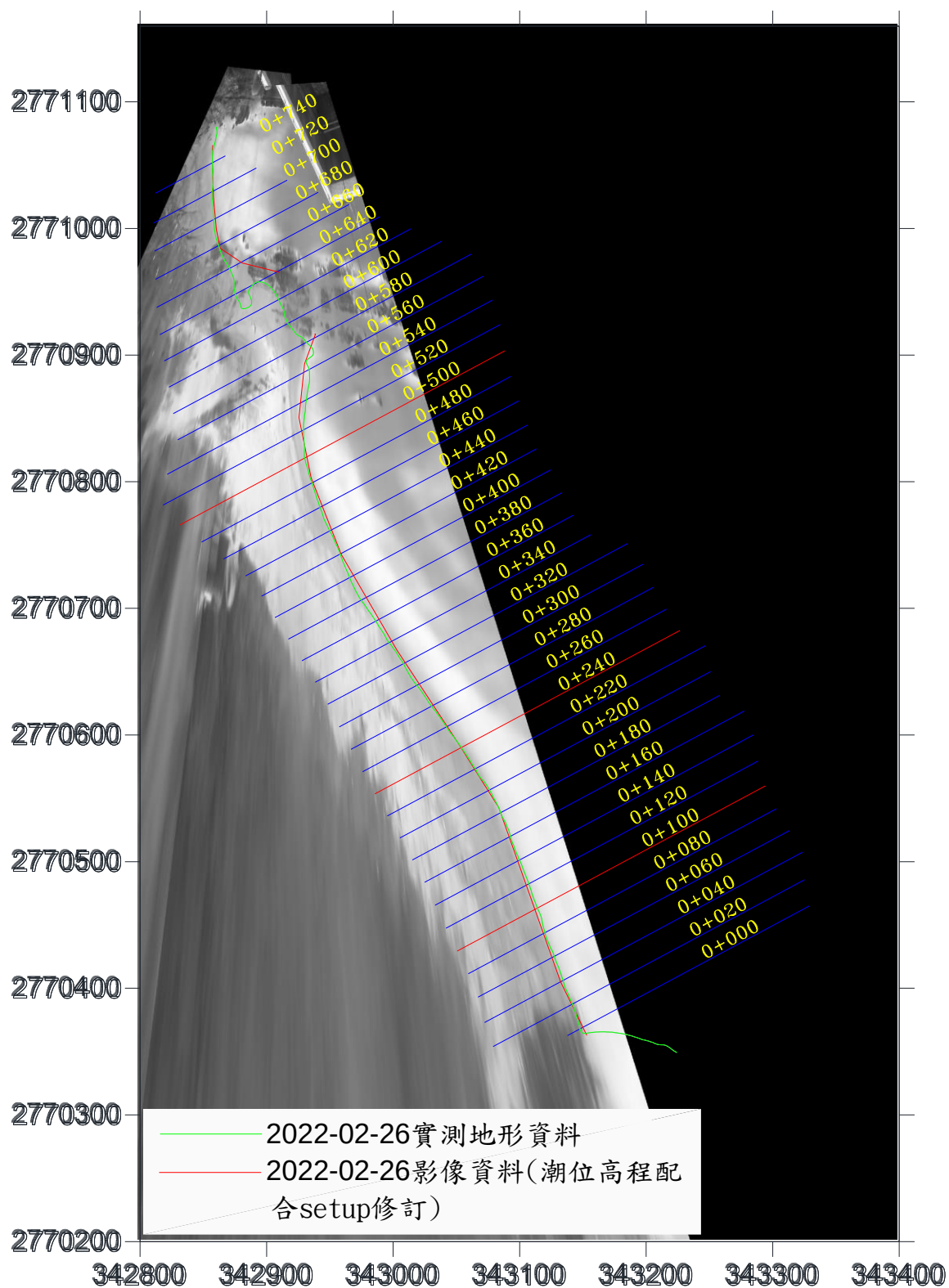
圖 3-22 水位線分析結果圖(2022/02/26)
