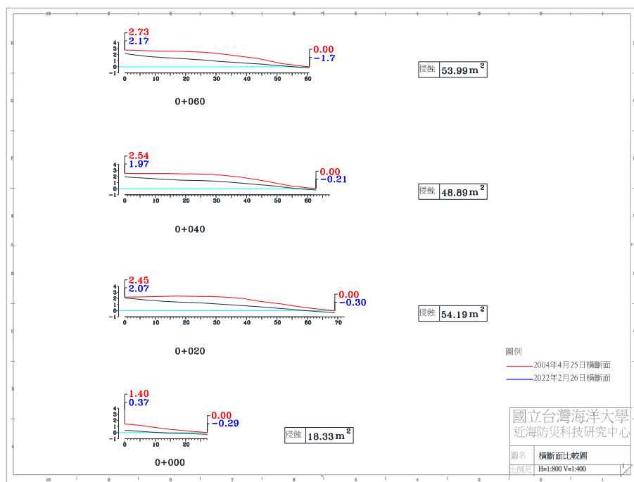
圖 4-4(j) 2022 年 2 月 26 日 A 監測區橫斷面比較圖
