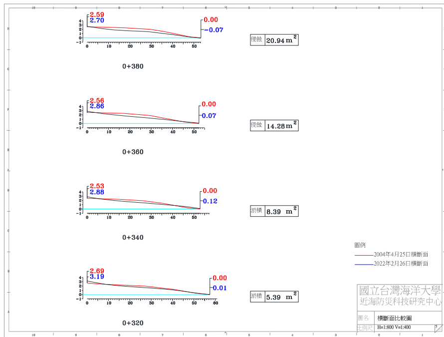
圖 4-4(f) 2022 年 2 月 26 日 A 監測區橫斷面比較圖
