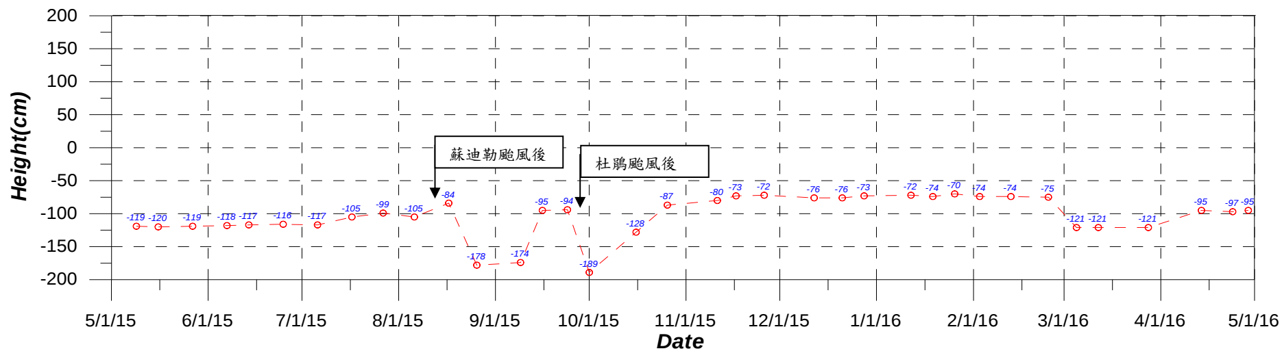
監測區 #06' 樁觀測紀錄圖 (#06 重新放置後更名為 #06')
