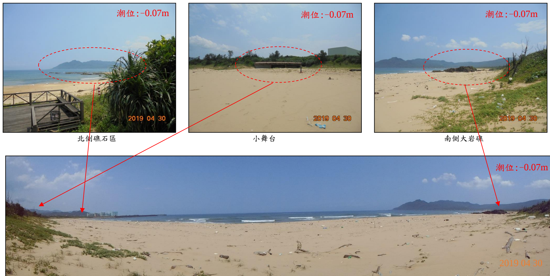
圖 3-6 鹽寮海岸短期性養灘區地形地貌圖(2019/4/30)
