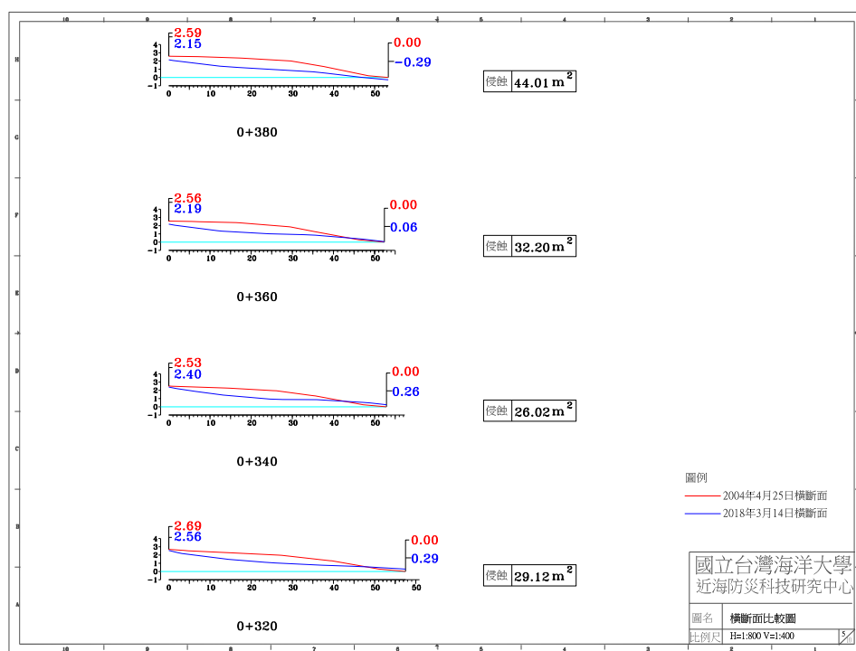
圖 4-4(f) 2018 年 3 月 14 日 A 監測區橫斷面比較圖
