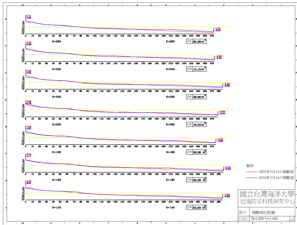
圖 4-5(e) 2018 年 3 月 14 日 B 監測區橫斷面比較圖
