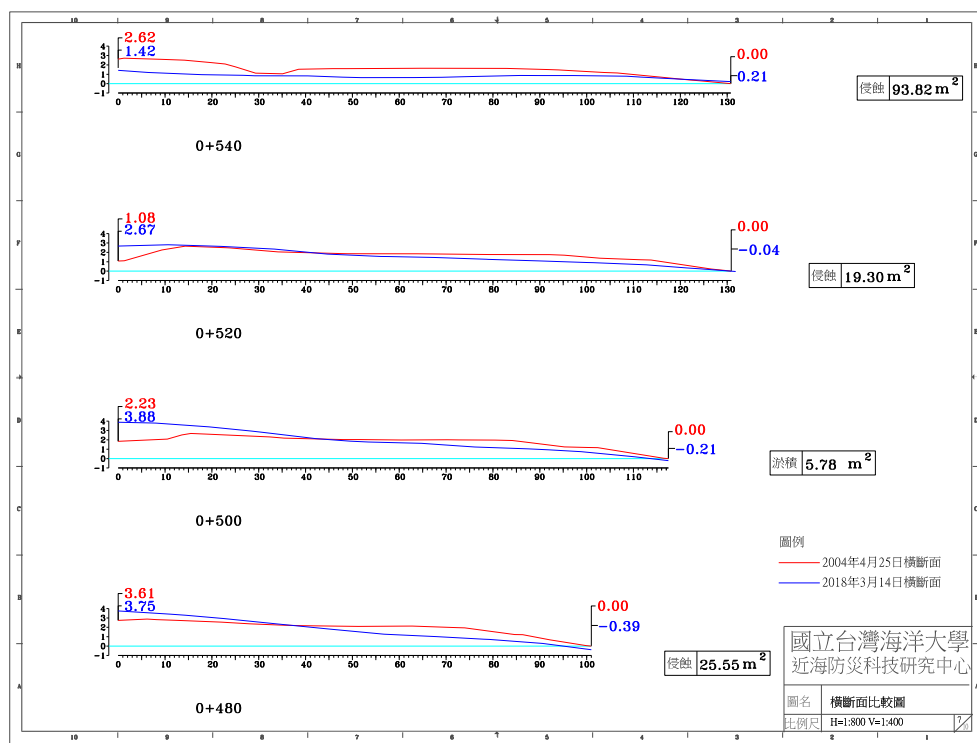
圖 4-4(d) 2018 年 3 月 14 日 A 監測區橫斷面比較圖
