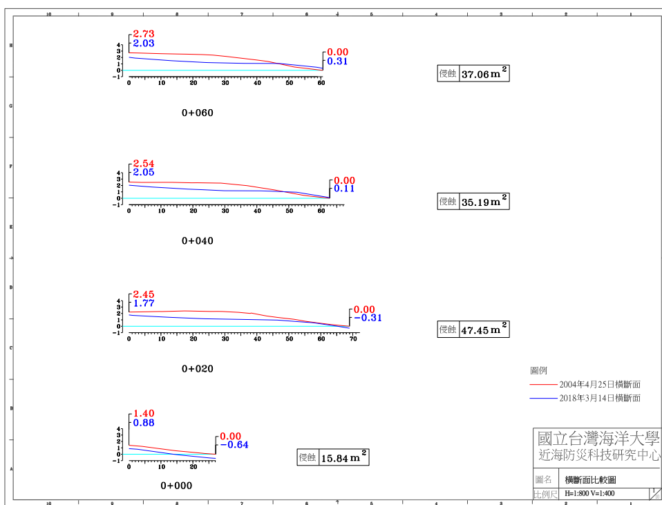
圖 4-4(j) 2018 年 3 月 14 日 A 監測區橫斷面比較圖
