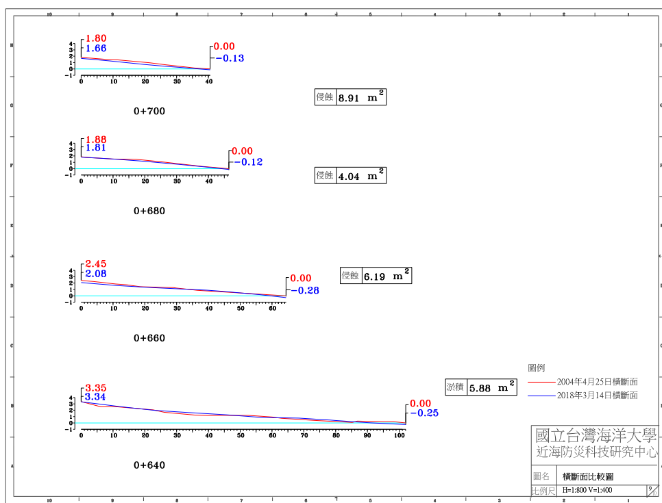
圖 4-4(b) 2018 年 3 月 14 日 A 監測區橫斷面比較圖
