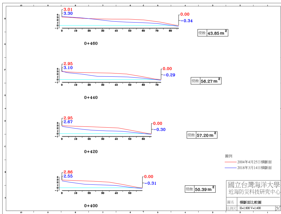
圖 4-4(e) 2018 年 3 月 14 日 A 監測區橫斷面比較圖
