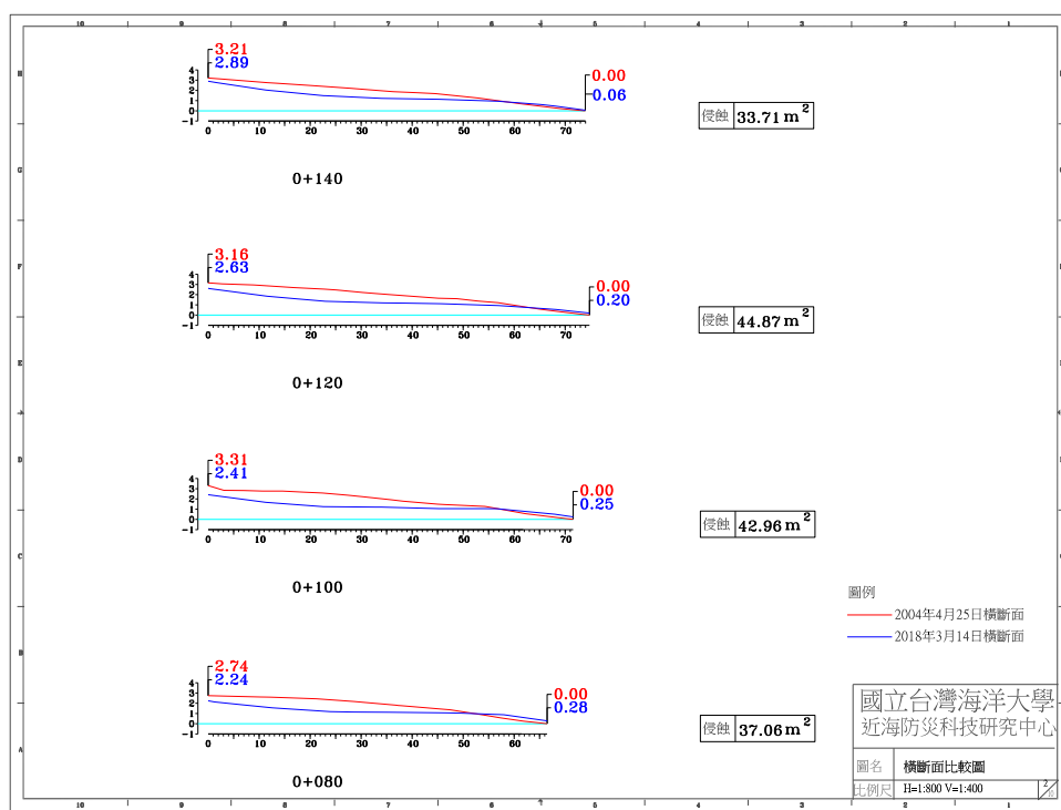
圖 4-4(i) 2018 年 3 月 14 日 A 監測區橫斷面比較圖
