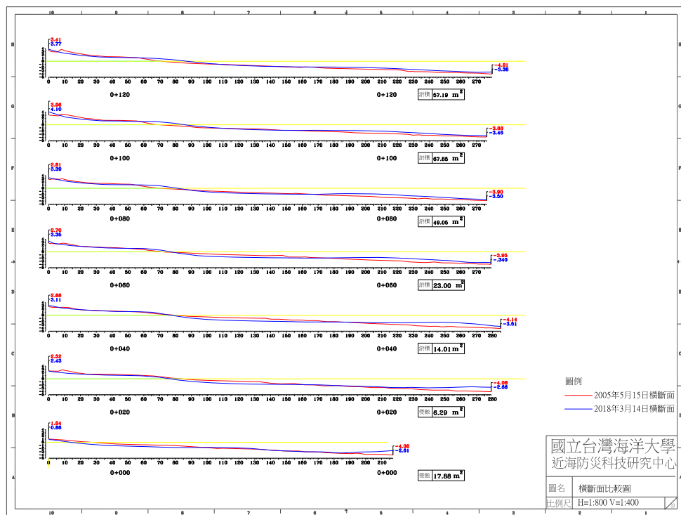
圖 4-5(f) 2018 年 3 月 14 日 B 監測區橫斷面比較圖
