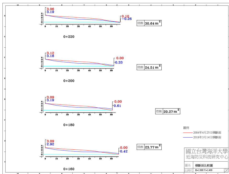
圖 4-4(h) 2018 年 3 月 14 日 A 監測區橫斷面比較圖
