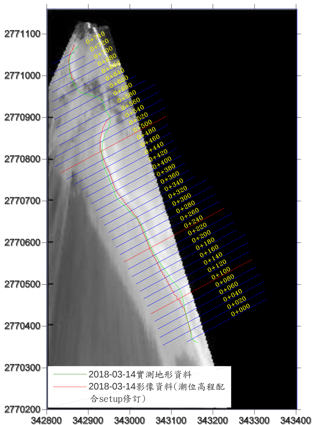
圖 3-22 水位線分析結果圖(2018/3/14)
