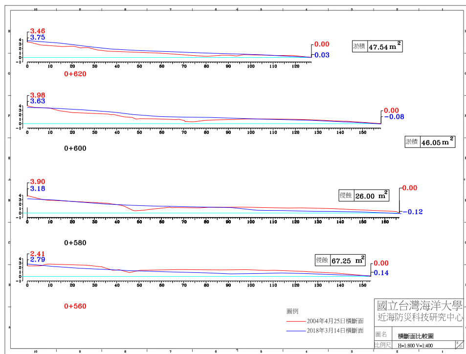
圖 4-4(c) 2018 年 3 月 14 日 A 監測區橫斷面比較圖
