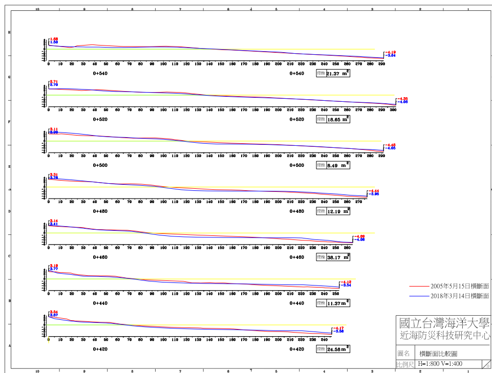
圖 4-5(c) 2018 年 3 月 14 日 B 監測區橫斷面比較圖
