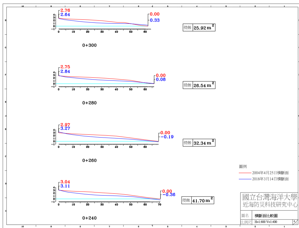
圖 4-4(g) 2018 年 3 月 14 日 A 監測區橫斷面比較圖
