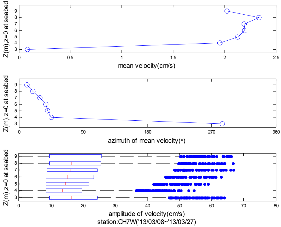
附錄 III.11 圖-7 CH7W 分層平均流速、平均流向剖面及流速振幅鬚盒圖
