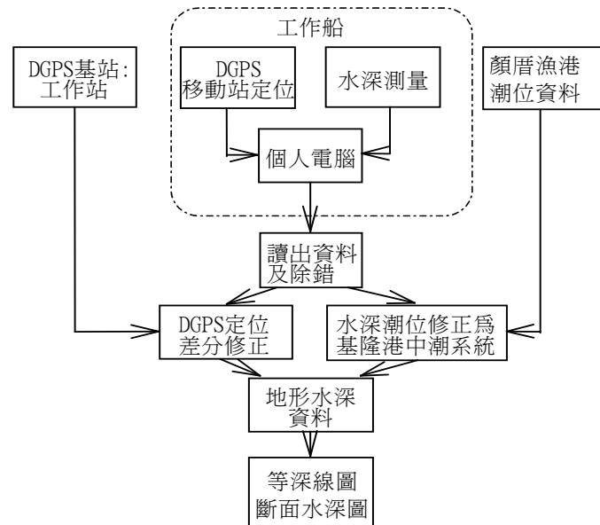
附圖 II-7 水深測量與資料處理流程
