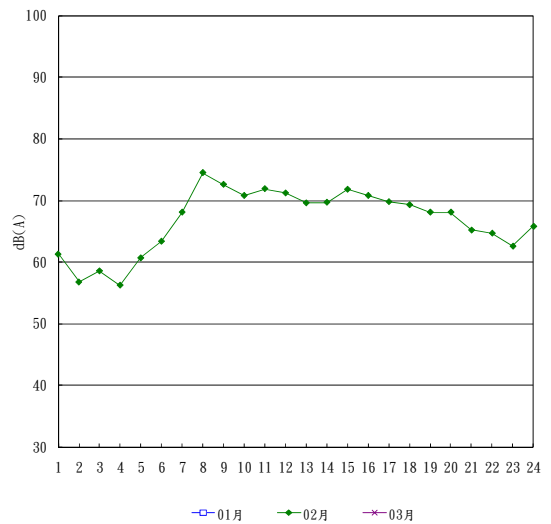
圖 2.2-8 5號連絡道路路口本季噪音測值逐時變化圖
