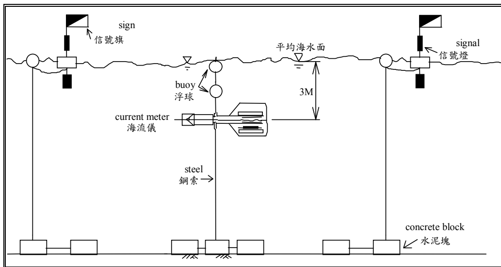
附圖II-8 海流儀與錨碇系統組合圖
