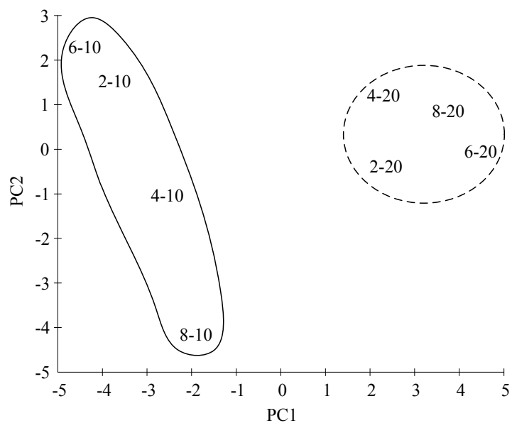
圖 2.10.2-3 民國 102 年 3 月彰濱工業區附近海域各測站浮游動物群聚分析圖(圖中第一個數字代表測站，第二個數字代表深度)
