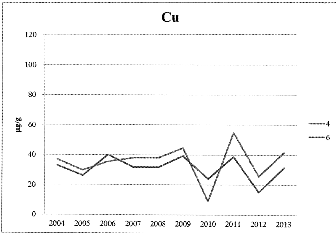
附錄 III.10-2 圖 17 2004~2013 年第一季測站 4 及 6 漁舟蜆螺體內銅含量之測 站比較圖
