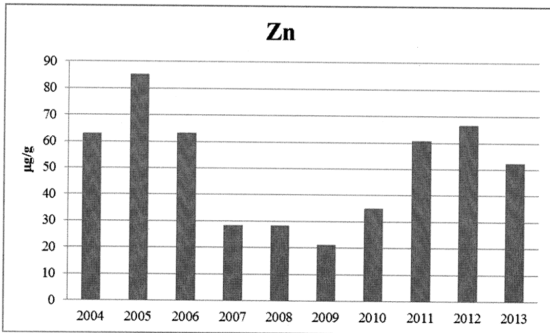
附錄 III.10-2 圖 12 2004 至 2013 年三月漁舟蜆螺體內鋅含量之年度比較圖
