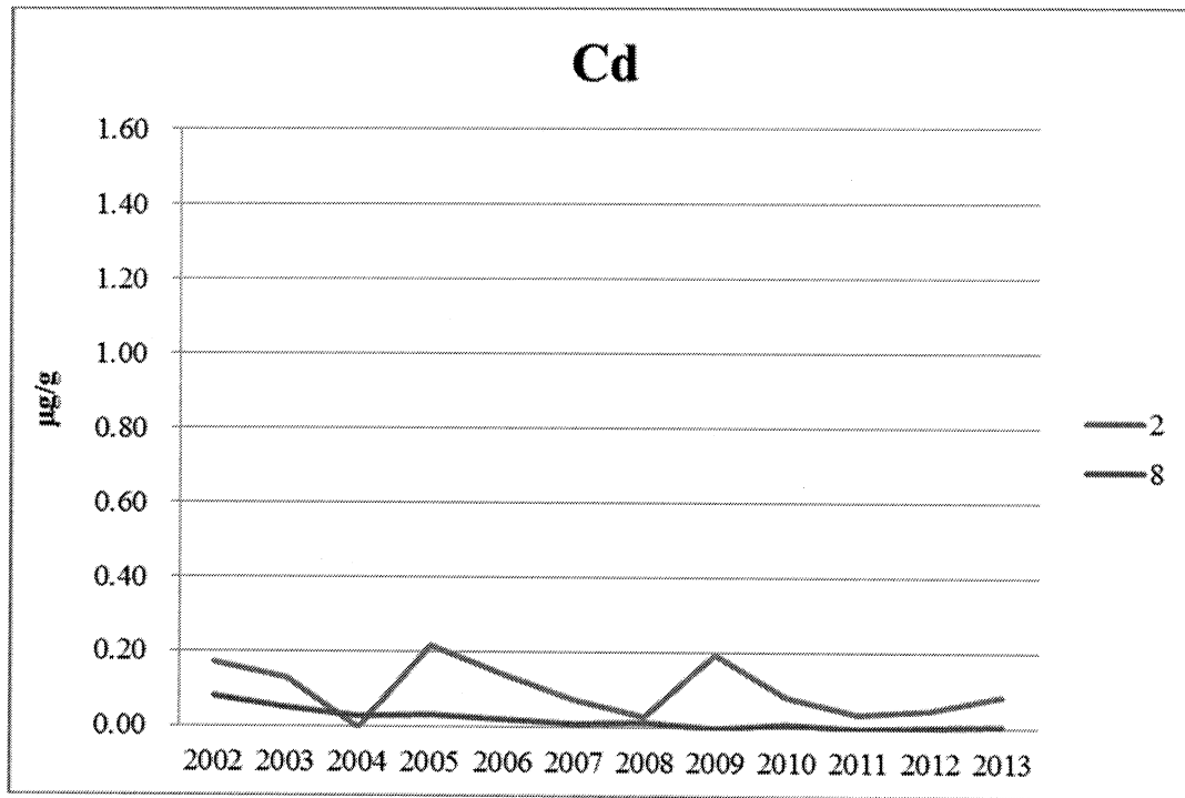
附錄 III.10-2 圖 15 2002~2013 年測站 2 及 8 第一季短指和尚蟹體內鎘含量之測站比較圖
