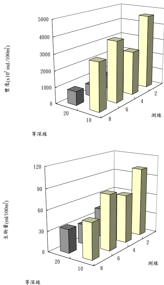
圖 2.10.2-1 民國 102 年 3 月彰化濱海工業區附近海域浮游動物之豐度及生物量分布圖
