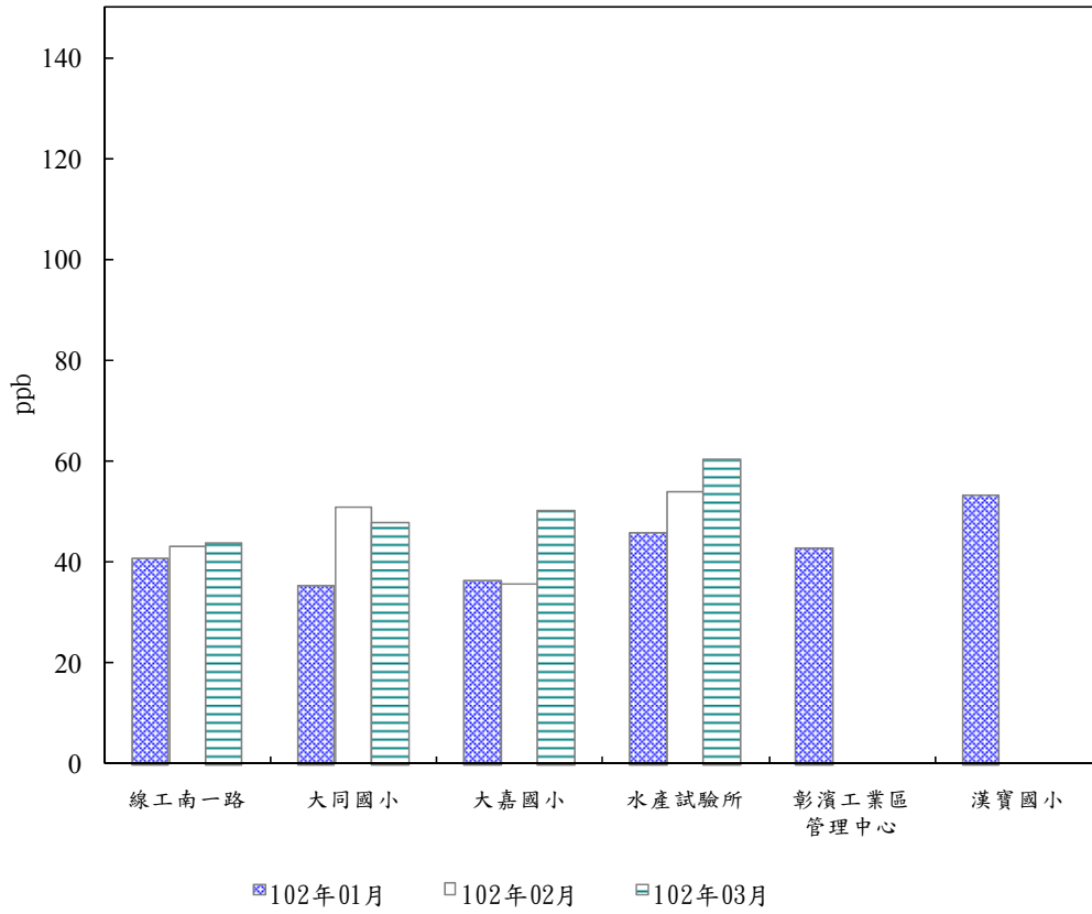
圖 2.1-7 本季各測站 O 3 最高小時值監測結果比較分析圖
