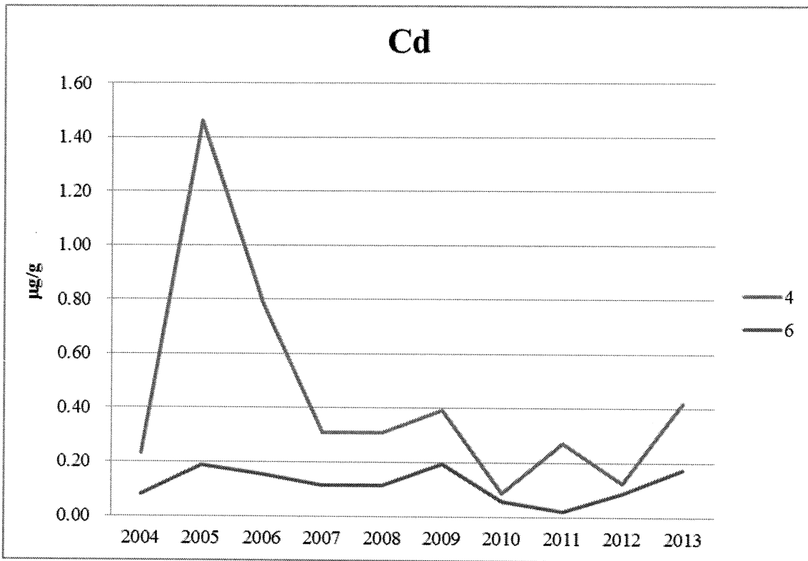
附錄 III.10-2 圖 19 2004~2013 年第一季測站 4 及 6 漁舟蜆螺體內鎘含量之測 站比較圖
