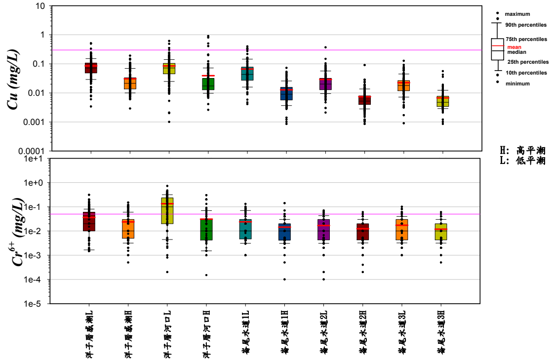
彰濱近岸水質 (河川: 1992 ~ 2012; 水道: 2000 ~ 2012)
