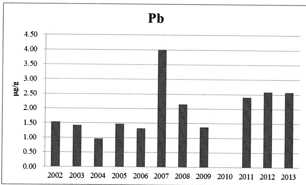
附錄 III.10-2 圖 6 2002 至 2013 年三月短指和尚蟹體內鉛含量之年度比較圖
