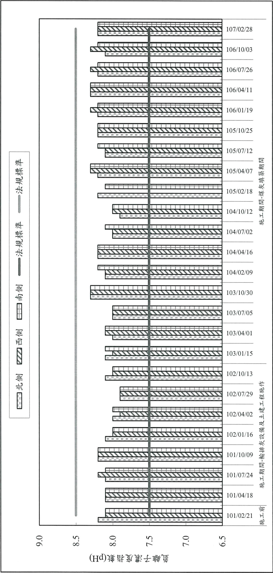
註：乙類海域環境標準之氫離子濃度指數(pH)標準值為 7.5~8.5。 圖 2.2-6 歷季各測站氫離子濃度指數(pH)監測成果彙整
