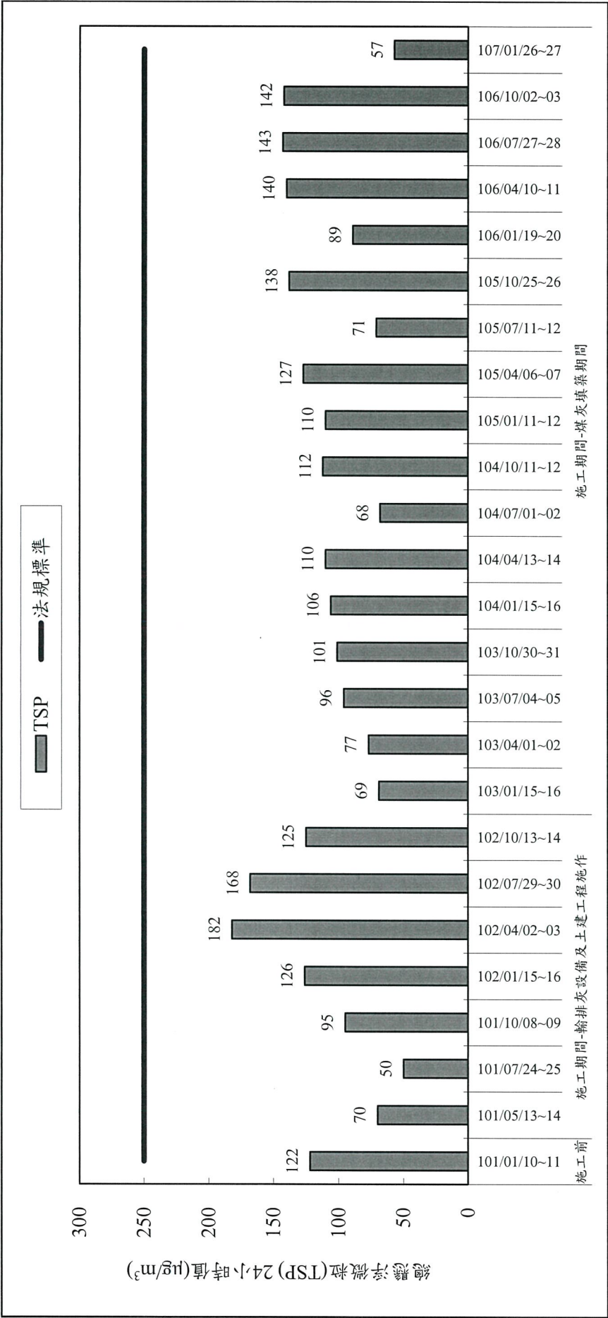
圖 2.1-1 歷季總懸浮微粒(TSP)24 小時值監測成果彙整
