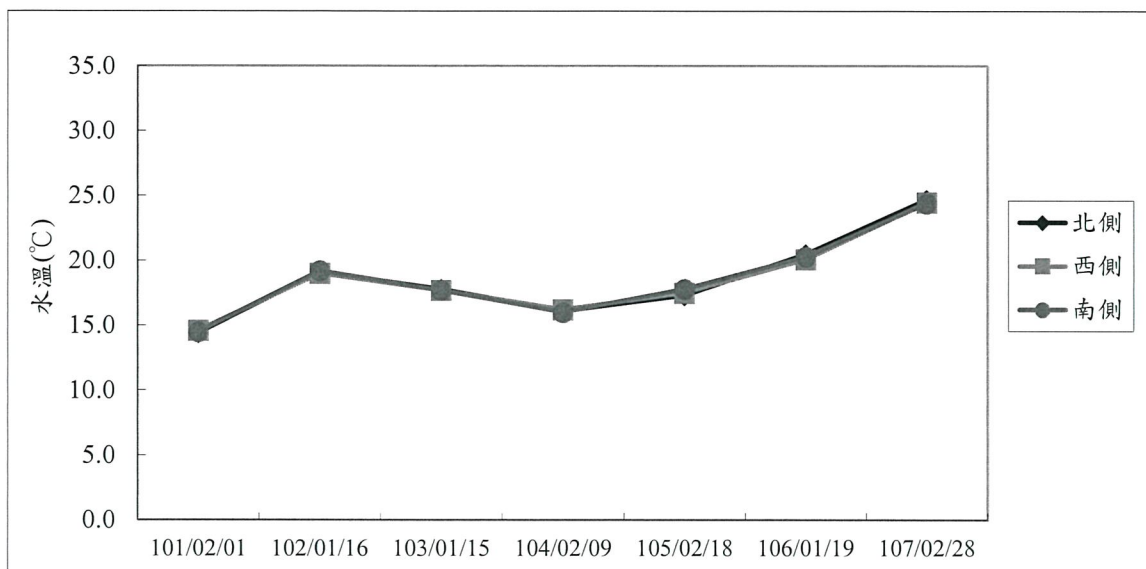
圖 3.1-9 歷年同期各測站水温監測成果彙整
