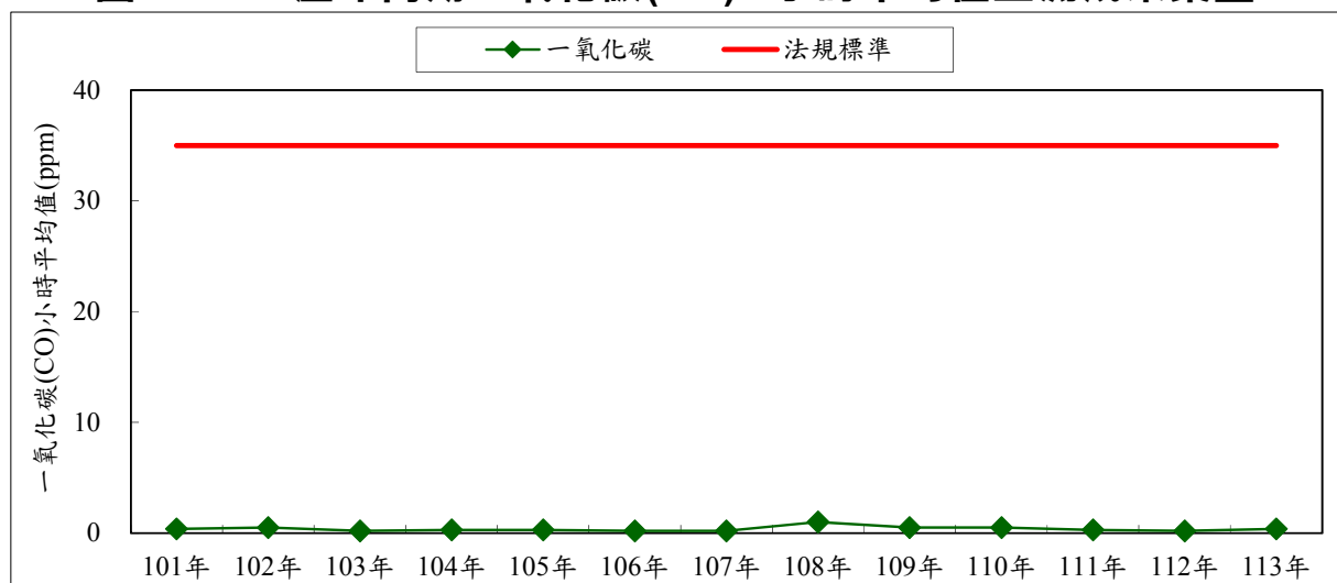
圖 3.1-8 歷年同期一氧化碳(CO)小時平均值監測成果彙整
