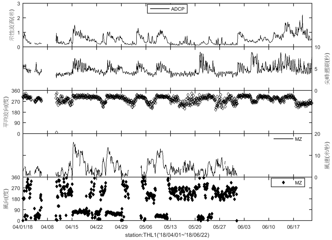
圖 2.13-6 THL1 測站 2018 年 4~6 月波浪與風速風向時序列
