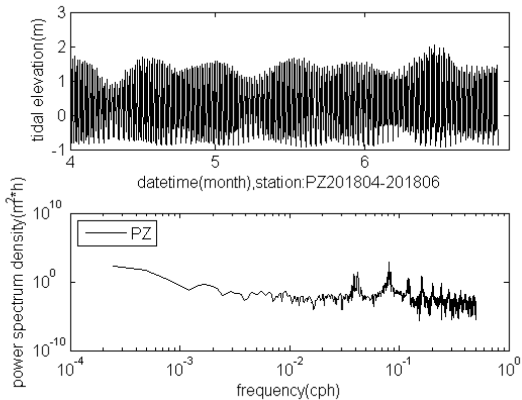
圖 2.13-4 PZ 測站 2018 年 4~6 月實測潮位頻譜與逐時變化圖
