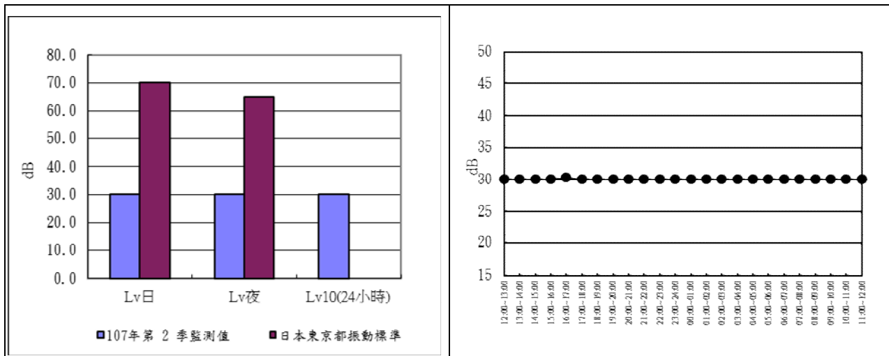
圖 2.3-4 海口橋 107 年度第 2 季振動監測成果分析圖及逐時變化圖
