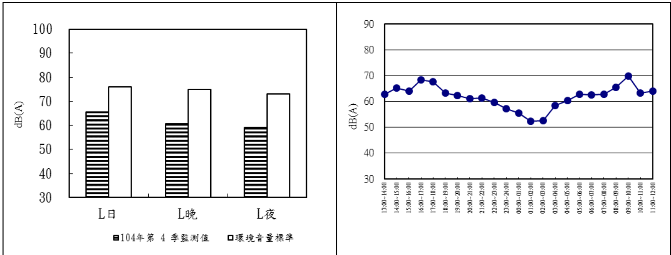
圖 2.2-4 海口橋 107 年第 2 季噪音監測成果分析圖及逐時變化圖
