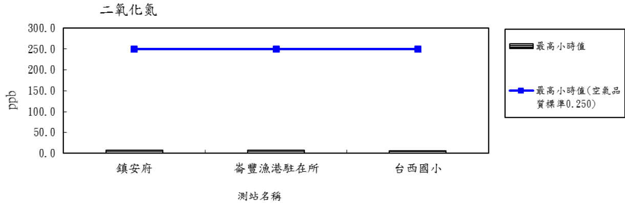
圖 2.1-4 107 年度第 2 季各測站二氧化氮(NO 2 )最高小時值比較分析圖
