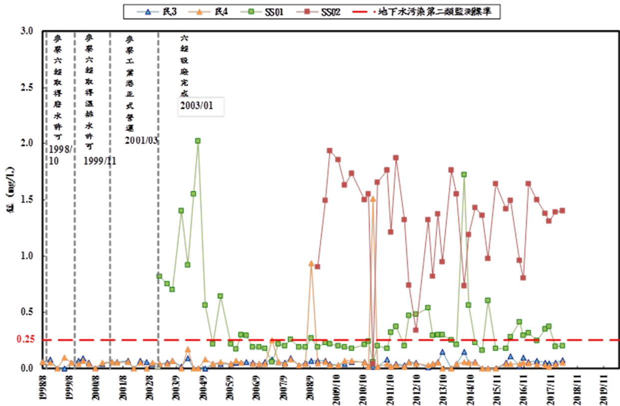
圖 3.1.6-6 錳歷年濃度測值變化
