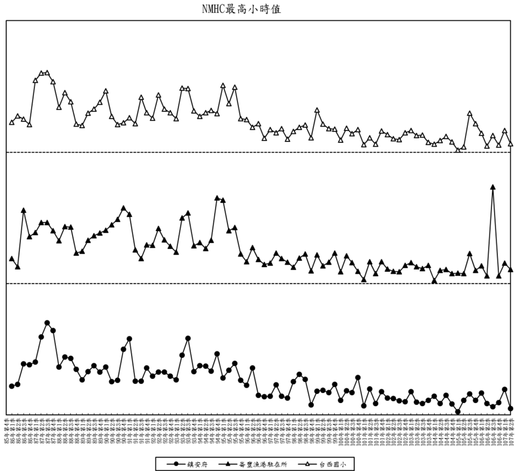
圖 3.1.1-6 本計畫歷次非甲烷碳氫化合物(NMHC)最高小時值監測結果分析圖
