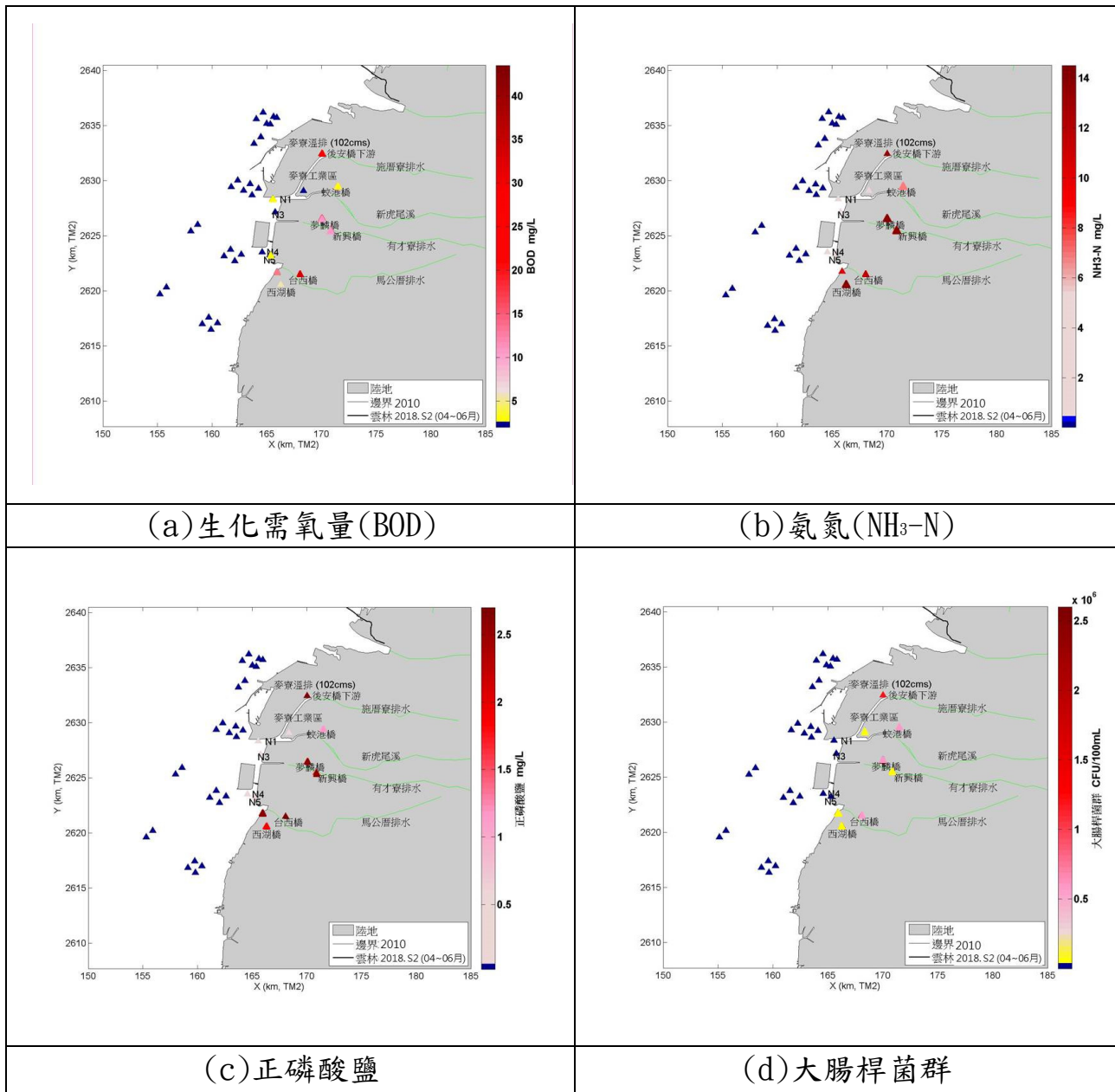
圖 2.8-1 雲林沿海水質污染特性之空間分布
