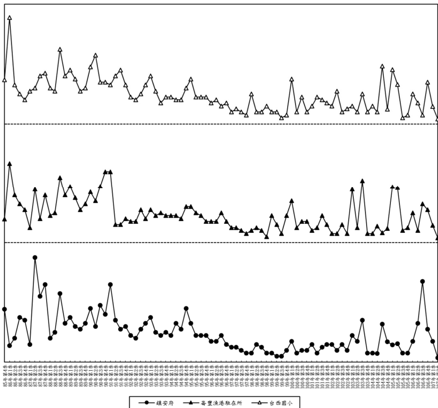
圖 3.1.1-2 本計畫歷次二氧化硫(SO 2 )最高小時值監測結果分析圖
