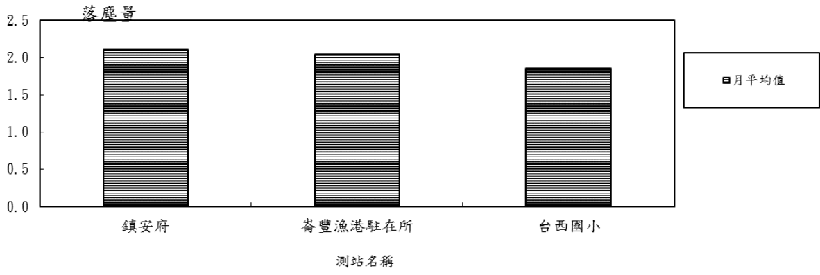
圖 2.1-10 107 年度第 2 季各測站落塵量平均值比較分析圖
