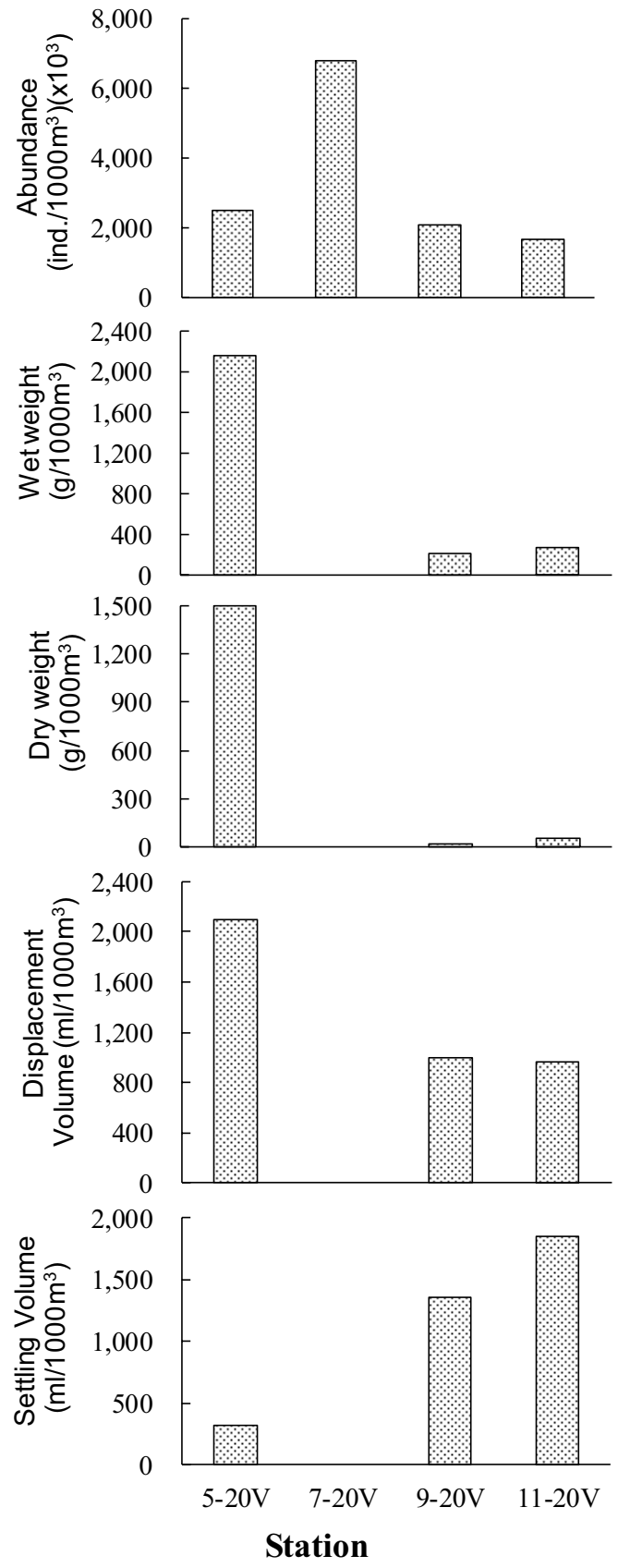
圖 2.10.1-3 民國 107 年 6 月 6 日雲林縣台西鄉 20 米水深垂直各測站中浮游動物之豐度及生物量的變化圖
