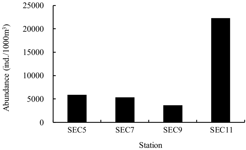
圖 2.11.3-6 雲林縣離島式基礎工業區沿海魚卵豐度 (107年5月28日)
