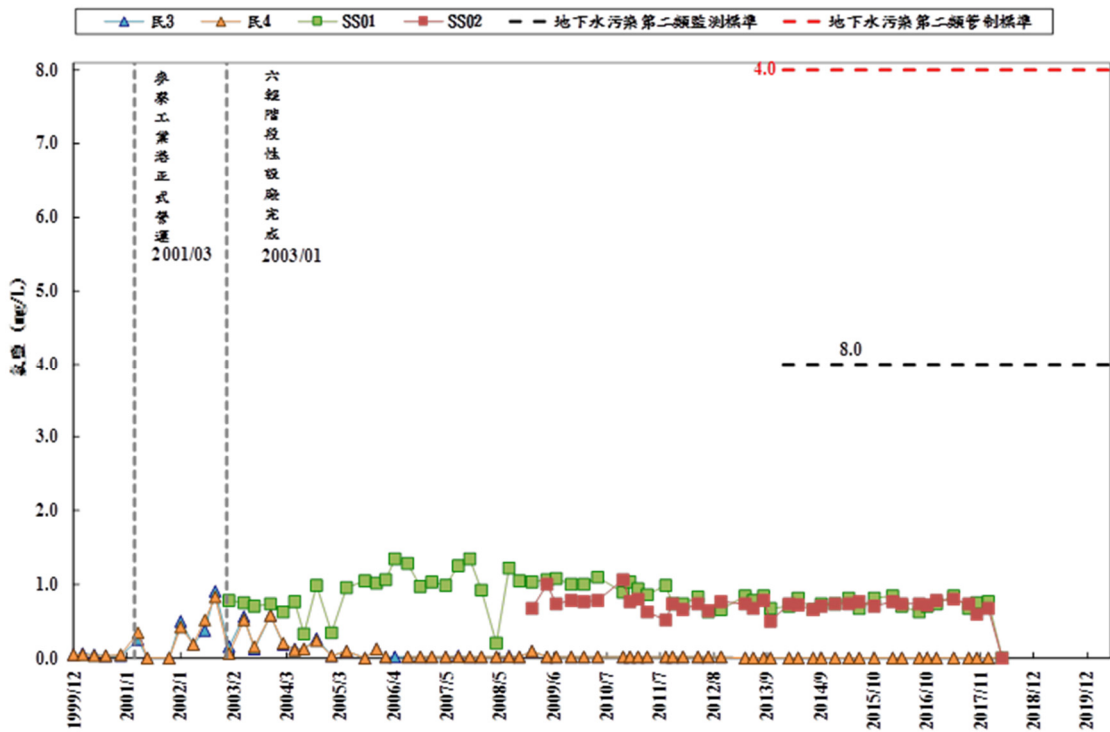
圖 3.1.6-4 氯鹽歷年濃度測值變化(環保署於 102 年 12 月 18 日修正發布氯鹽之監測標準及管制標準)
