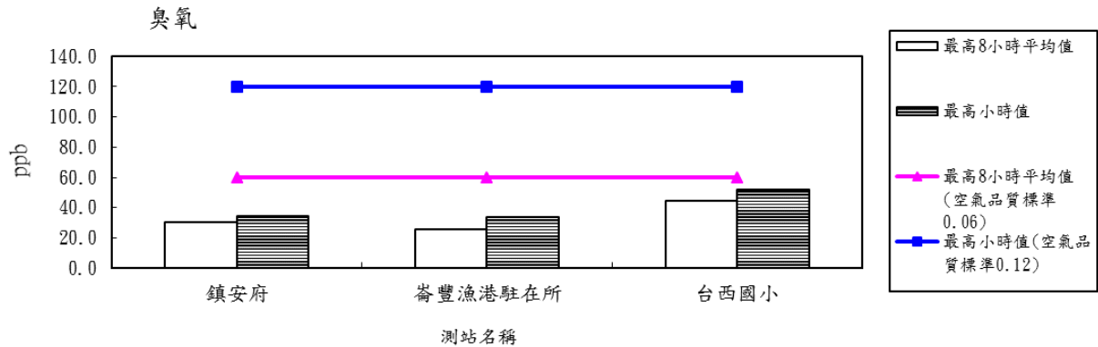
圖 2.1-5 107 年度第 2 季各測站臭氧(O 3 )最高 8 小時平均值及最高小時值比較分析圖
