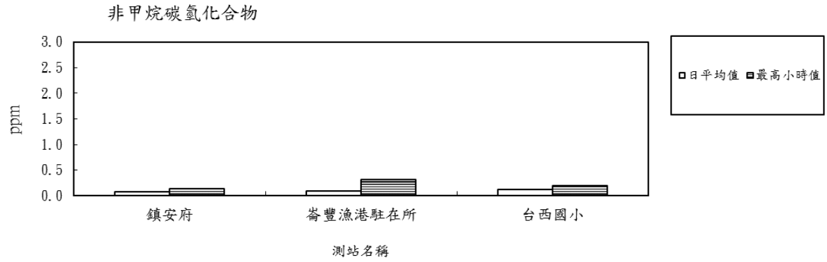
圖 2.1-7 107 年度第 2 季各測站非甲烷碳氫化合物(NMHC)日平均值及最高小時值比較分析圖
