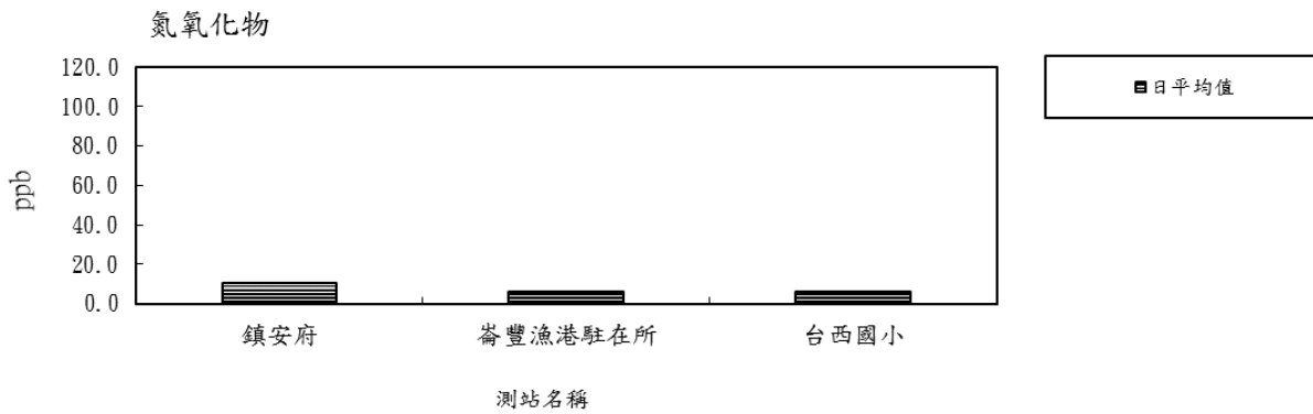
圖 2.1-3 107 年度第 2 季各測站氮氧化物(NO x )日平均值比較分析圖
