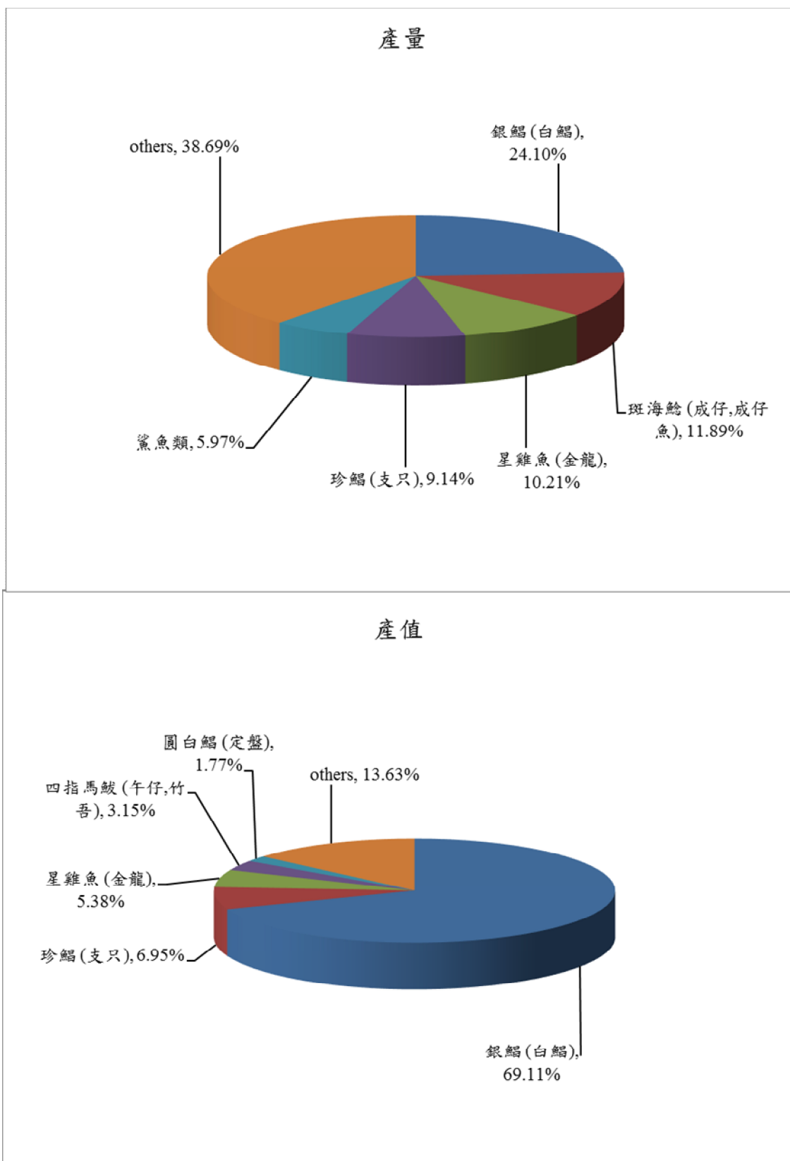
圖 2.11.1-2 雲林沿海地區流刺網漁業主要漁獲產值和產量百分比圖 (107 年 4-6 月)
