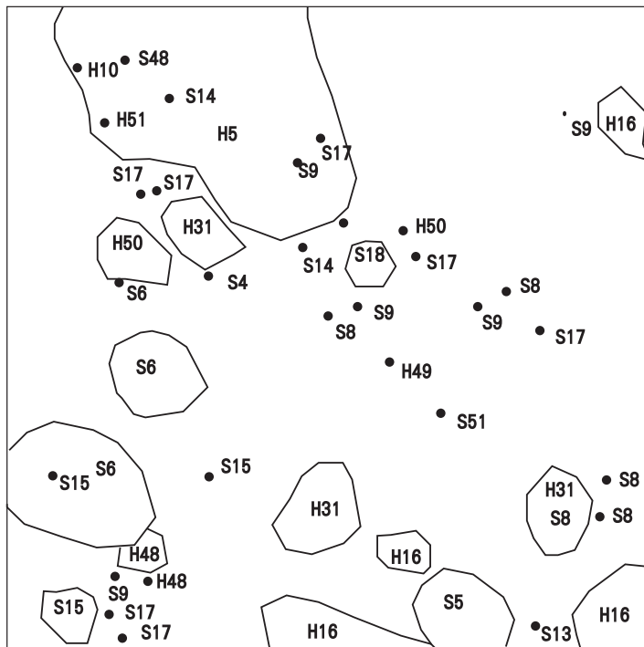
圖2.5-12 陸域植物生態夏季監測 台塑木麻黃造林地樣區下層植物分布圖
