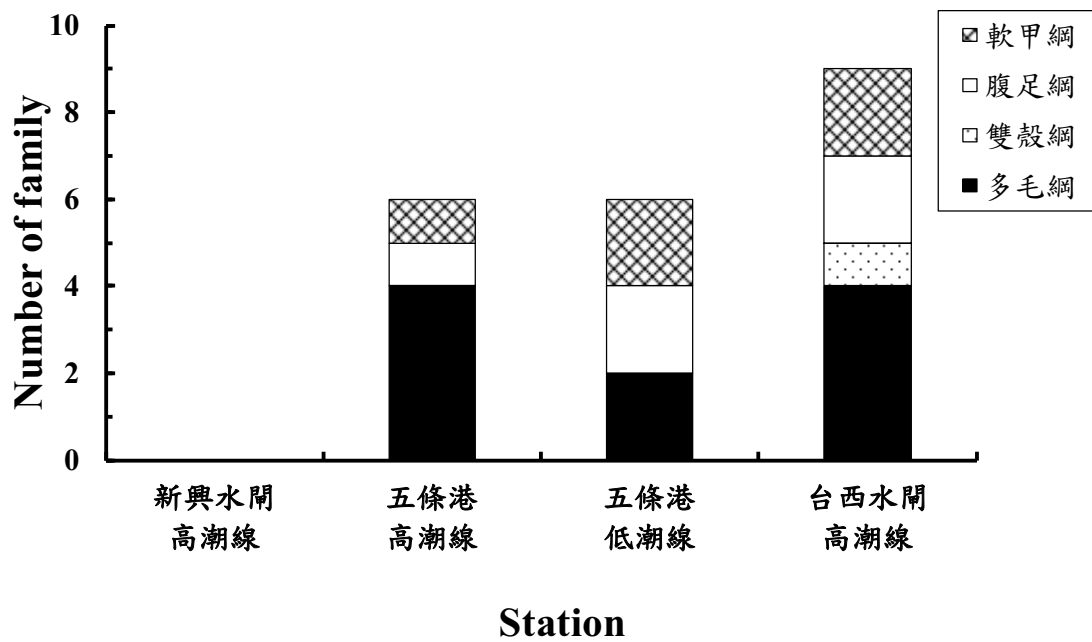
圖 2.10.3-1 民國 107 年第二季(5 月 15 日)離島工業區潮間帶各測站小型底棲生物之種類數變化
