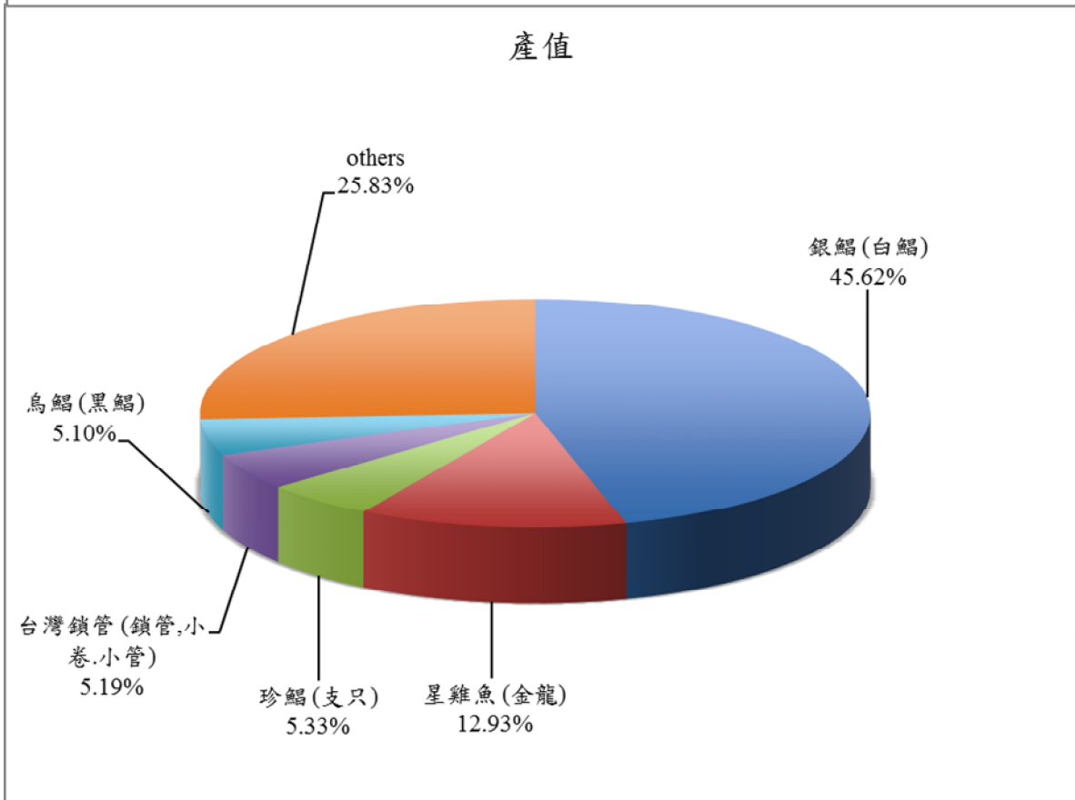
圖 2.11.1-3 雲林沿海地區雙拖網漁業主要漁獲產值和產量百分比圖 (107 年 4-6 月)
