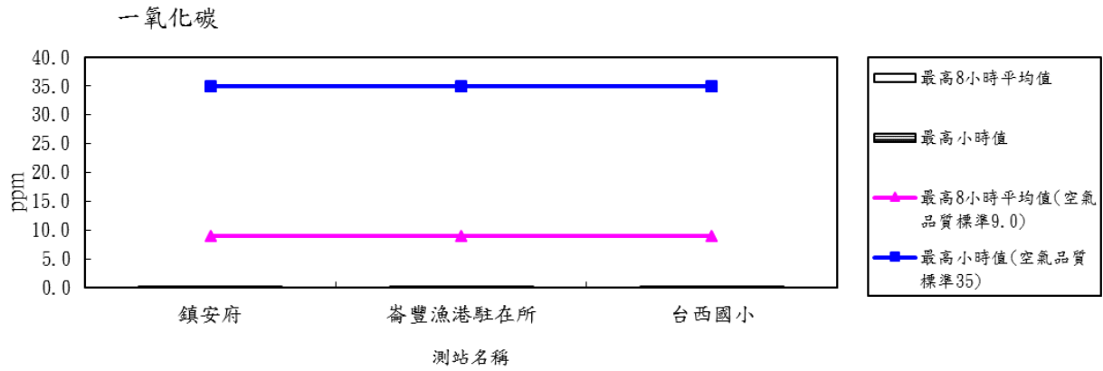
圖 2.1-1 107 年度第 2 季各測站一氧化碳(CO)最高 8 小時平均值及最高小時值比較分析圖
