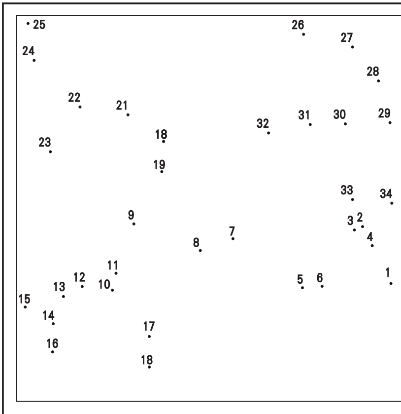
圖 2.5-1 陸域植物生態夏季監測 新吉濁水溪口樣區上層植物分布圖
