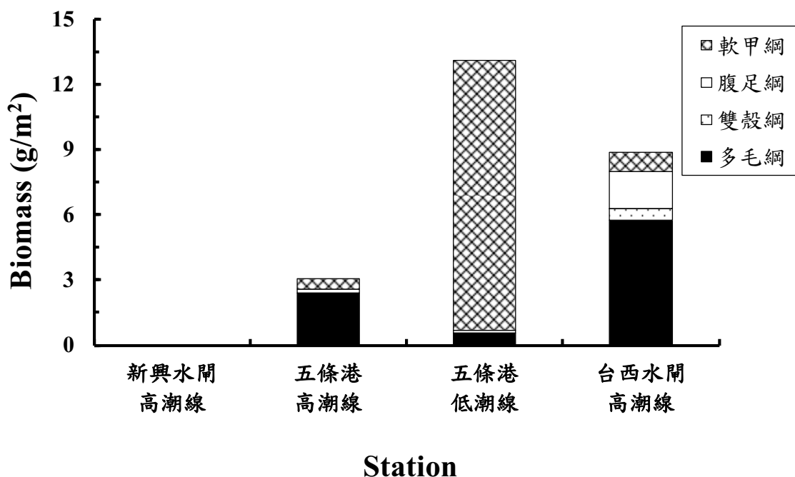
圖 2.10.3-3 民國 107 年第二季(5 月 15 日)離島工業區潮間帶各測站小型底棲生物之生物量(g/m 2 )變化
