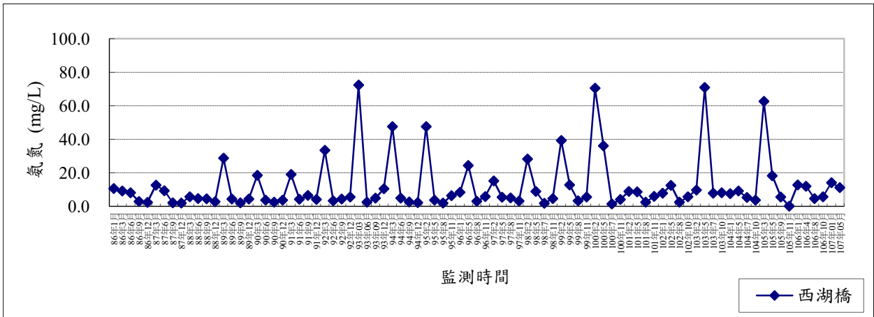
圖3.1.7-4 陸域水質歷次氨氮比較分析圖
