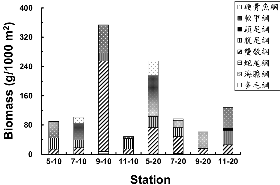
圖 2.10.2-3 民國 107 年第二季(6月 6 日)離島工業區亞潮帶各測站小型底棲動物之生物量之變化
