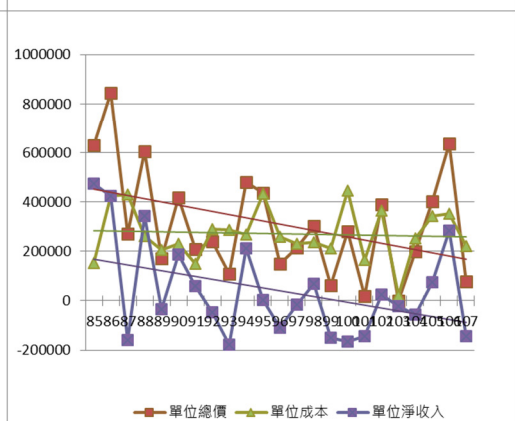
圖3.2.1-3 (續) 文蛤混養間卷戶85-107年單位產值變化圖(N.T.)
