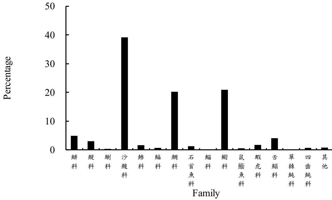
圖 2.11.3-1 雲林縣離島式基礎工業區沿海仔稚魚各大類組成 (107年5月28日)
