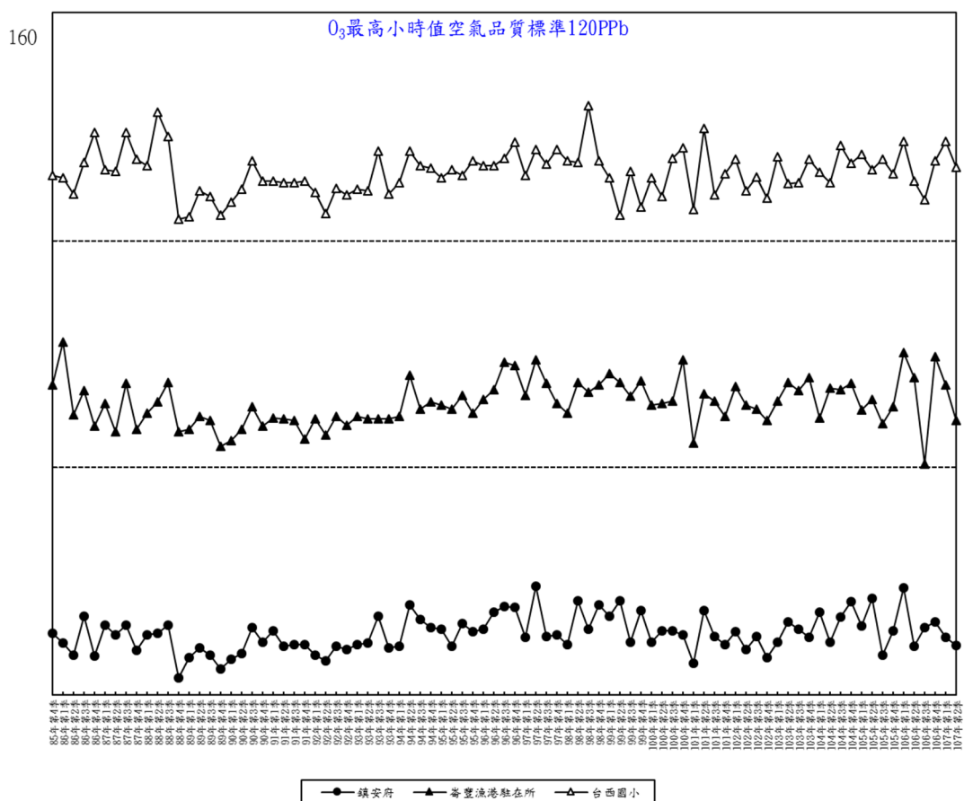
圖 3.1.1-4 本計畫歷次臭氧(O 3 )最高小時值監測結果分析圖
