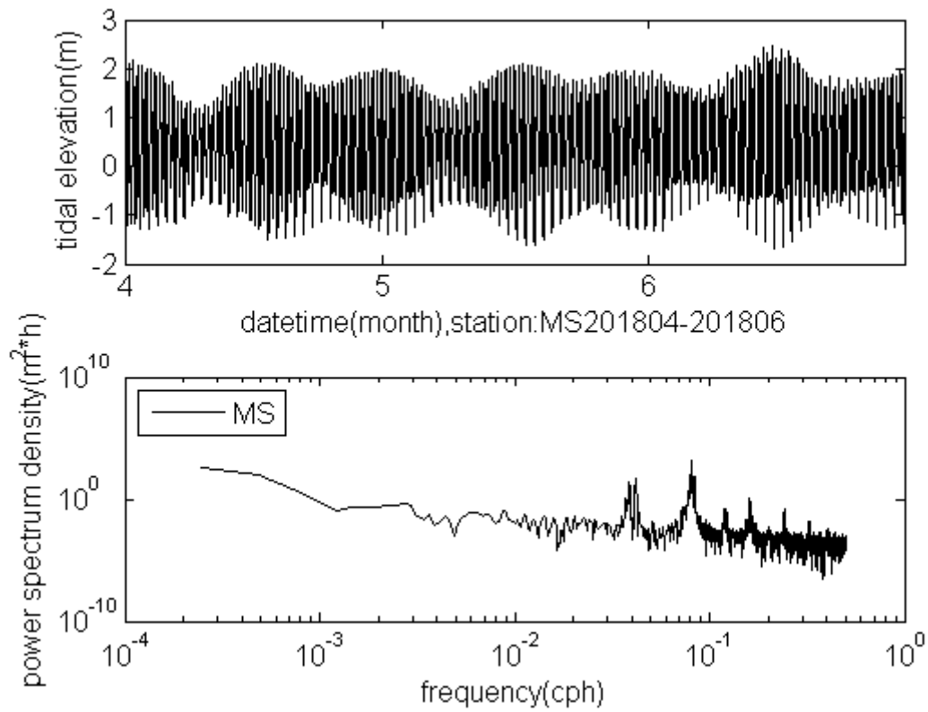
圖 2.13-3 MS 測站 2018 年 4~6 月實測潮位頻譜與逐時變化圖
