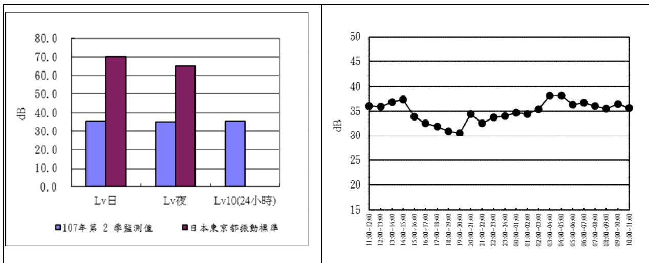
圖 2.3-2 海豐橋 107 年度第 2 季振動監測成果分析圖及逐時變化圖
