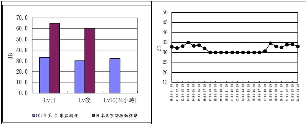
圖 2.3-1 安西府 107 年度第 2 季振動監測成果分析圖及逐時變化圖
