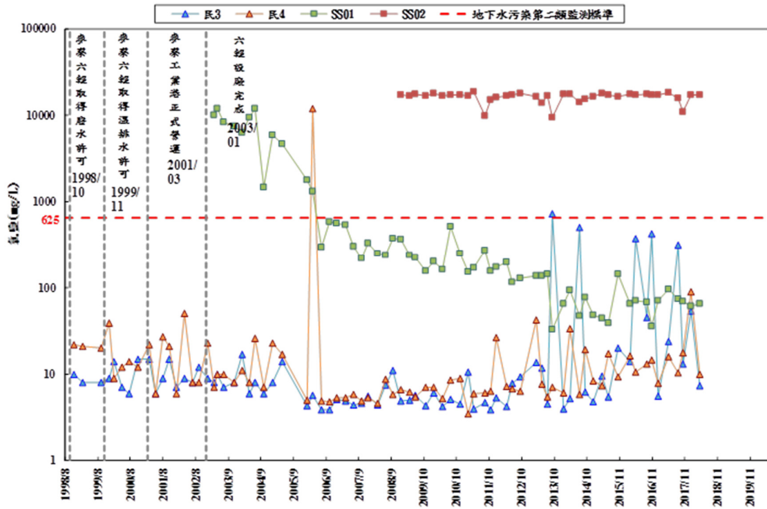
圖 3.1.6-3 氯鹽歷年濃度測值變化
