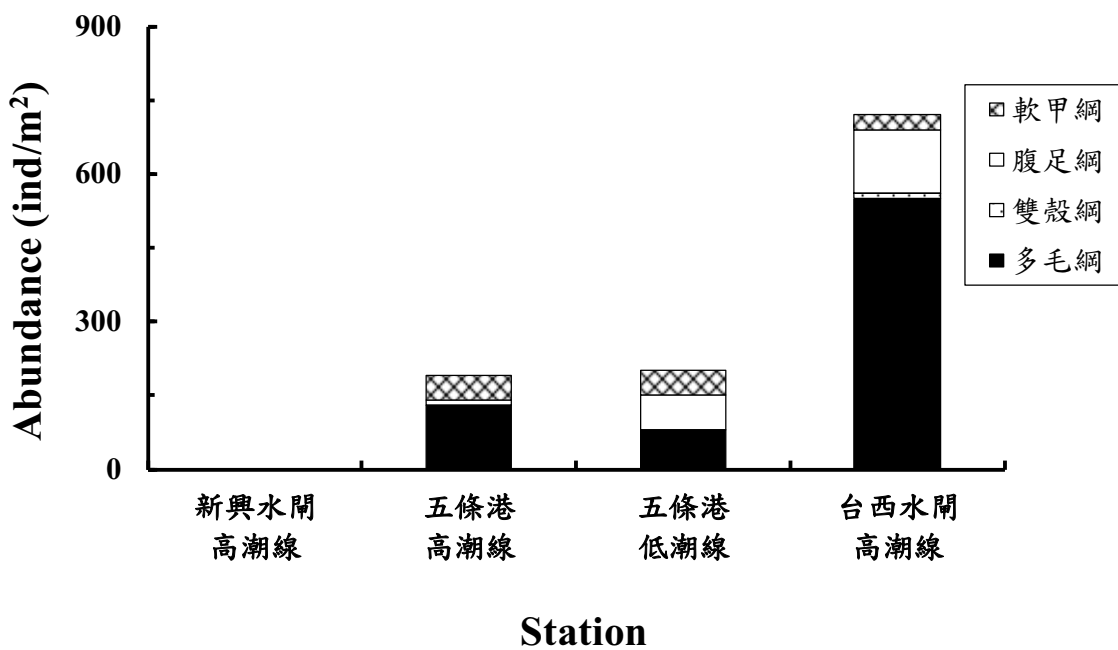
圖 2.10.3-2 民國 107 年第二季(5 月 15 日)離島工業區潮間帶各測站小型底棲生物之豐度(ind./m 2 )變化
