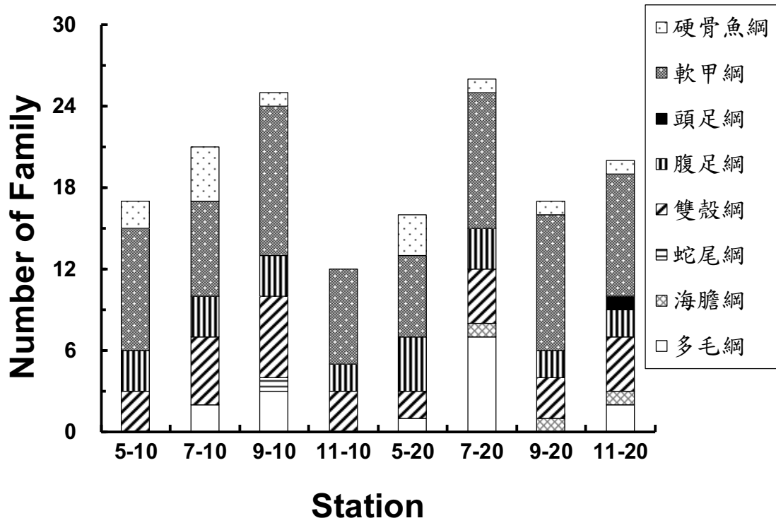
圖 2.10.2-1 民國 107 年第二季(6 月 6 日)離島工業區亞潮帶各測站小型底棲動物之科數變化
