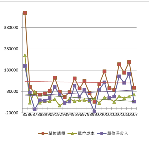
圖3.2.1-1 (續) 牡蠣間卷戶85-107年單位產值變化圖(N.T.)
