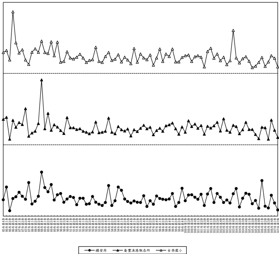
圖 3.1.1-8 本計畫歷次 PM 10 日平均值監測結果分析圖
