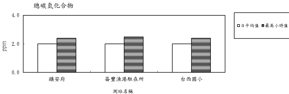
圖 2.1-6 107 年度第 2 季各測站總碳氫化合物(THC)日平均值及最高小時值比較分析圖
