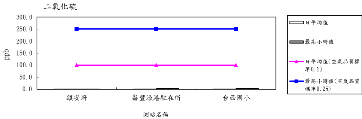
圖 2.1-2 107 年度第 2 季各測站二氧化硫(SO 2 )日平均值及最高小時值比較分析圖
