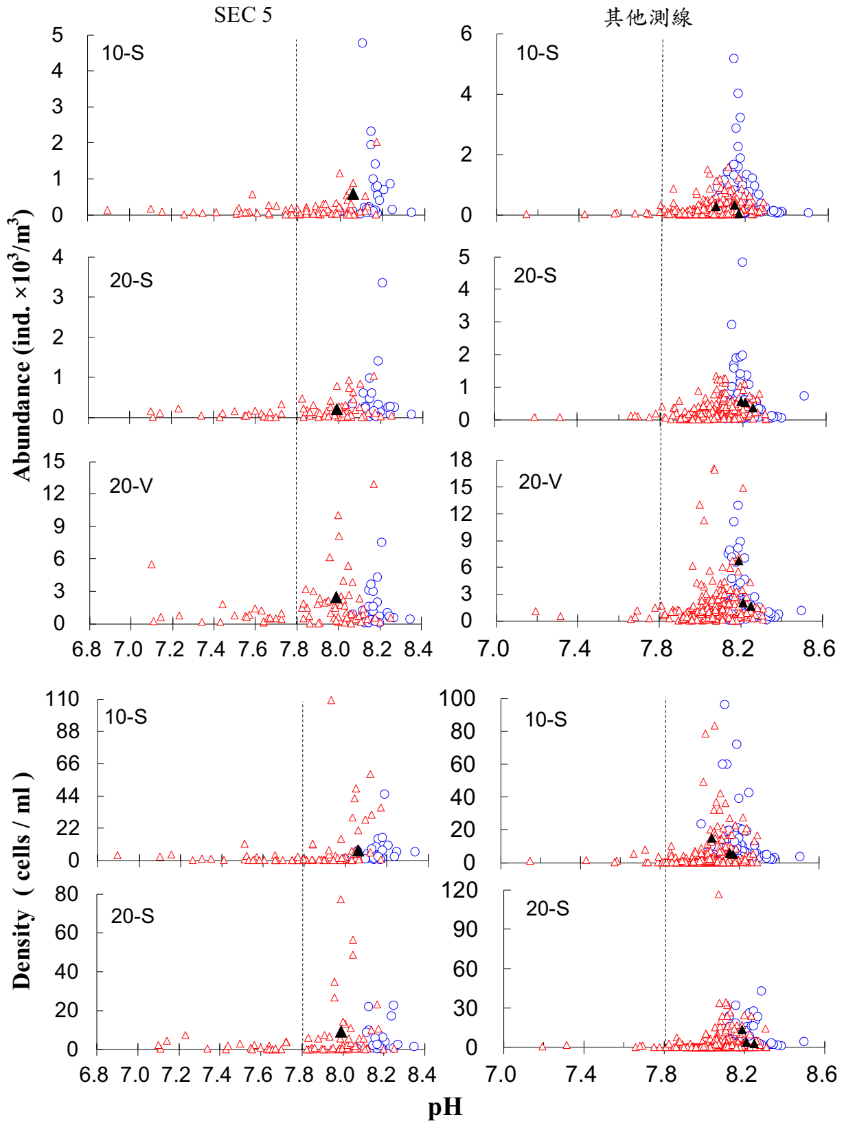
圖 2.10.1-9 歷年海域中之浮游動物豐度和浮游植物密度與 pH 之點圖 ( \circ : 民國 89 年以前 ; \Delta : 民國 89 年以後 ; \blacktriangle : 本季 )
