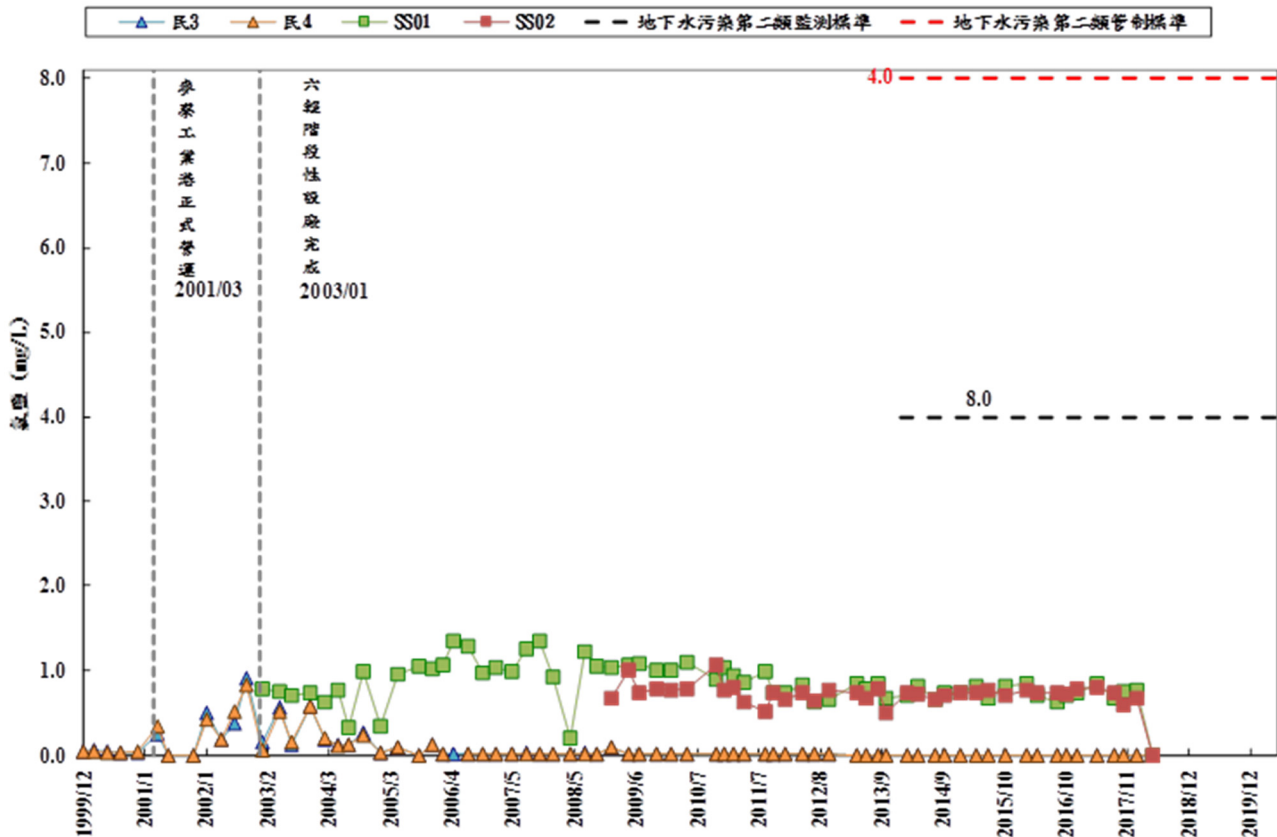
圖 3.1.6-7 鐵歷年濃度測值變化
