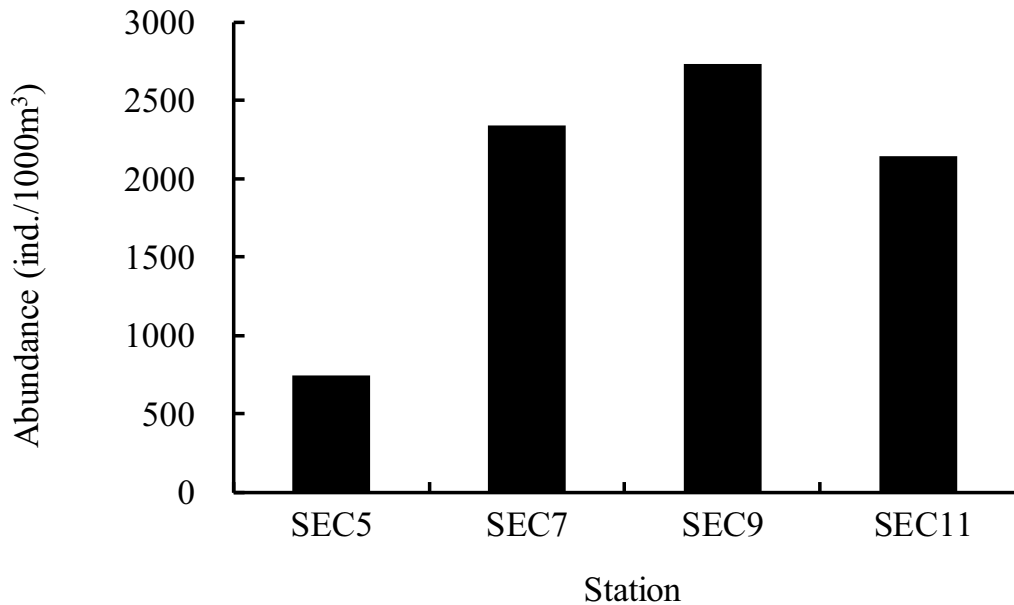
圖 2.11.3-8 雲林縣離島式基礎工業區沿海蟹幼生豐度 (107 年 5 月 28 日)
