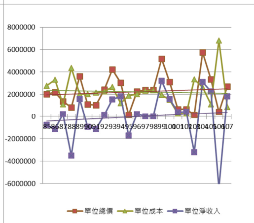
圖3.2.1-2 (續) 鯪魚間卷戶85-107年單位產值變化圖(N.T.)
