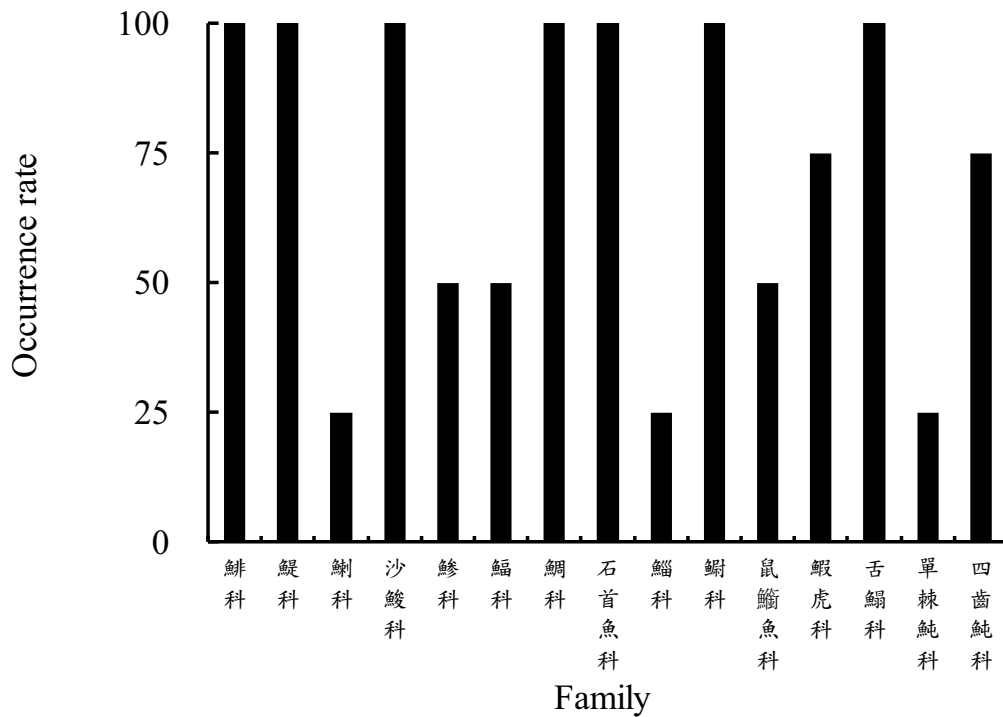
圖 2.11.3-2 雲林縣離島式基礎工業區沿海仔稚魚各大類出現率 (107年5月28日)
