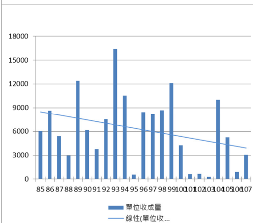
圖3.2.1-2 鯪魚間卷戶85-107年單位收成量比較圖(Kg)
