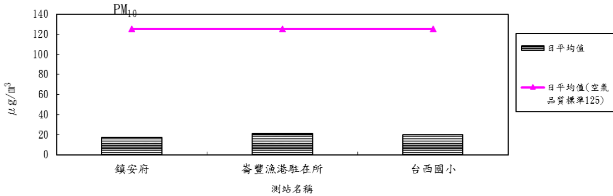
圖 2.1-9 107 年度第 2 季各測站 PM 10 日平均值比較分析圖
