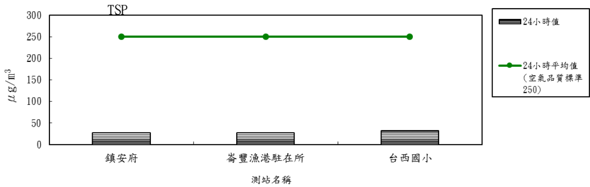
圖 2.1-8 107 年度第 2 季各測站 TSP 24 小時值比較分析圖
