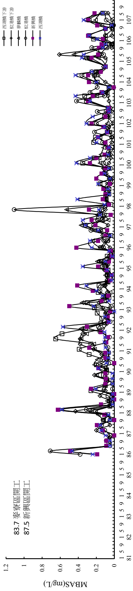
圖 3.1.8-1 (續26)離島工業區陸域河口歷年水質變化圖 時間(月, 81-106年)
