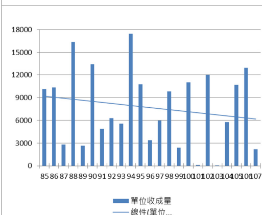
圖3.2.1-3 文蛤混養間卷戶85-107年單位收成量比較圖(Kg)
