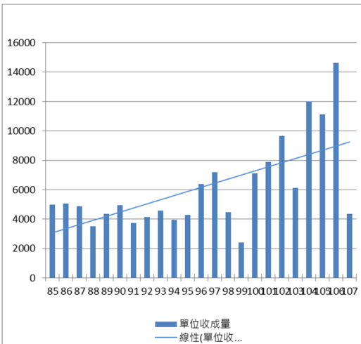
圖3.2.1-1 牡蠣間卷戶85-107年單位收成量比較圖(Kg)
