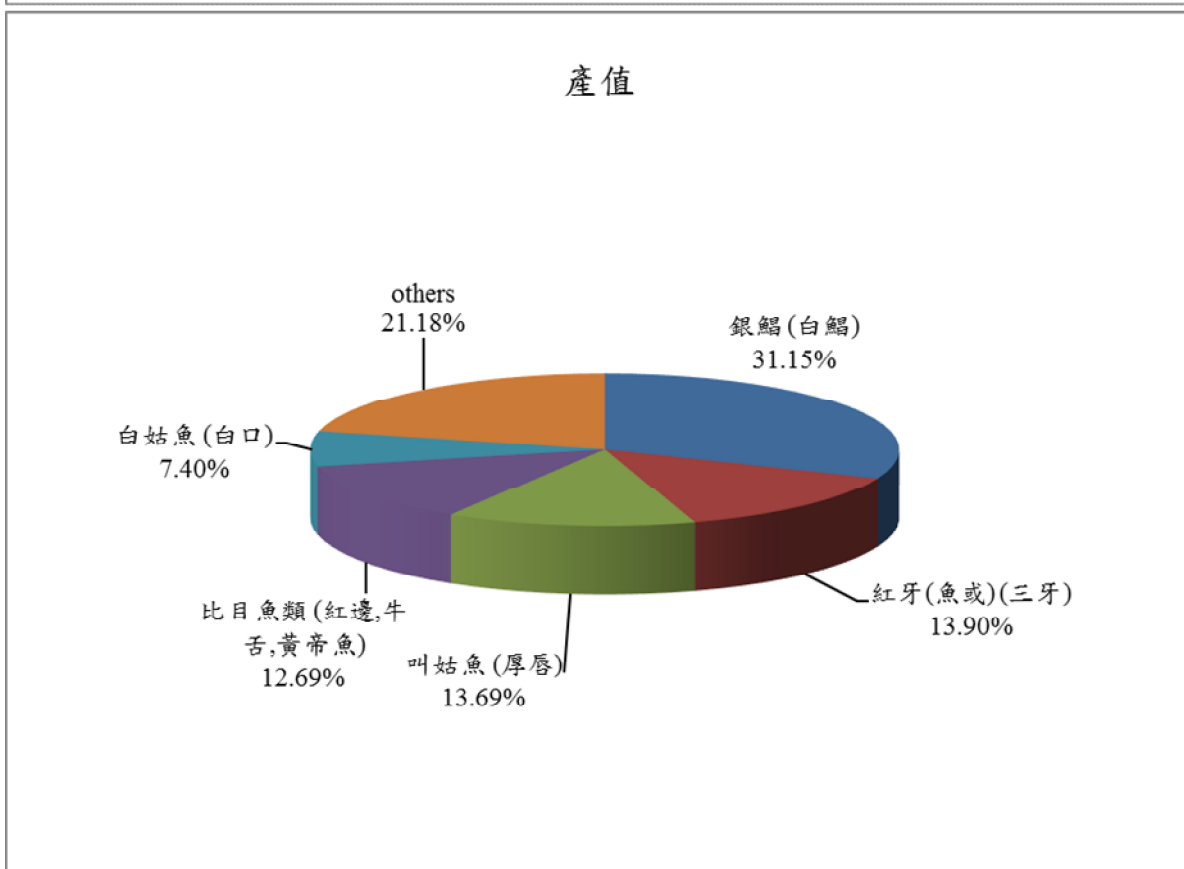
圖 2.11.1-1 雲林沿海地區蝦拖網漁業主要漁獲產值和產量百分比圖 (107 年 4-6 月)
