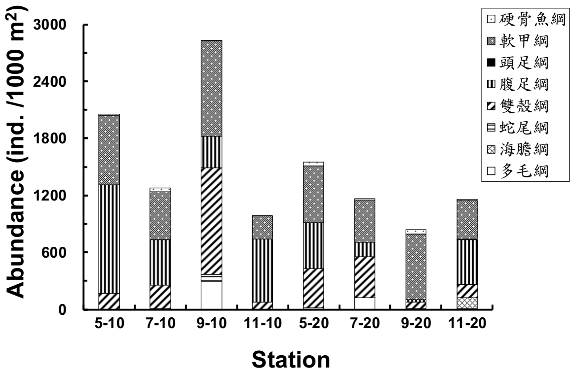
圖 2.10.2-2 民國 107 年第二季(6 月 6 日)離島工業區亞潮帶各測站小型底棲動物之豐度變化
