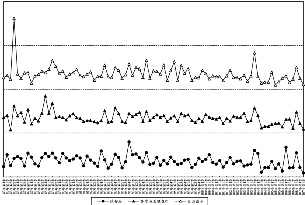
圖 3.1.1-7 本計畫歷次 TSP 24 小時值監測結果分析圖
