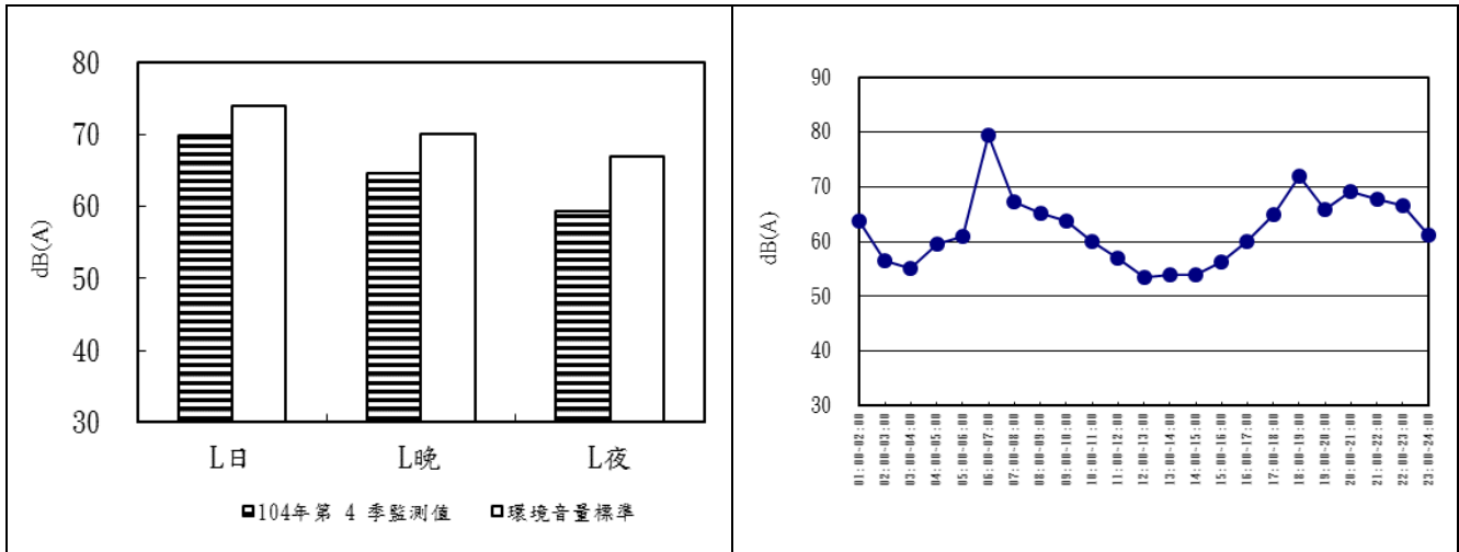
圖 2.2-1 安西府 107 年第 2 季噪音監測成果分析圖及逐時變化圖
