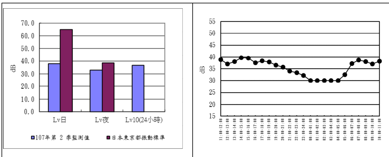
圖 2.3-3 崙豐國小 107 年度第 2 季振動監測成果分析圖及逐時變化圖
