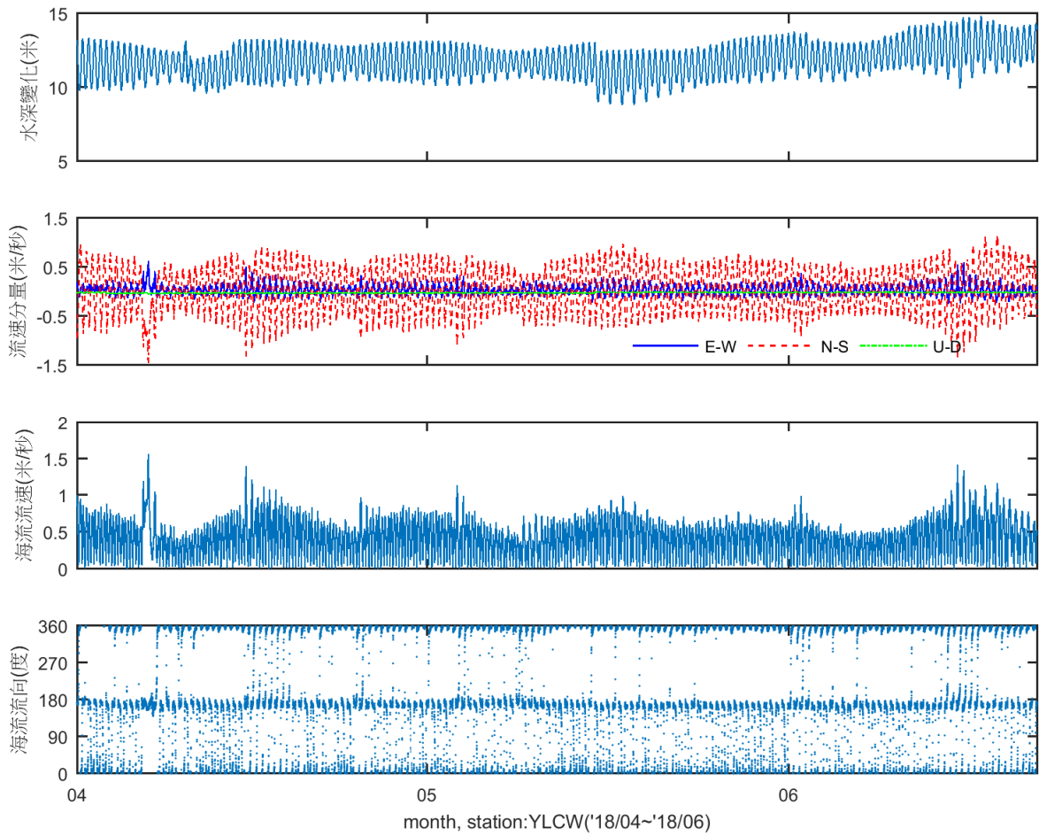
圖 2.13-9 YLCW 測站 2018 年 4~6 月海流分量與流速流向時序列
