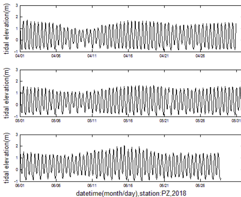
圖 2.13-2 PZ 測站 2018 年 4~6 月各月實測潮位逐時變化圖
