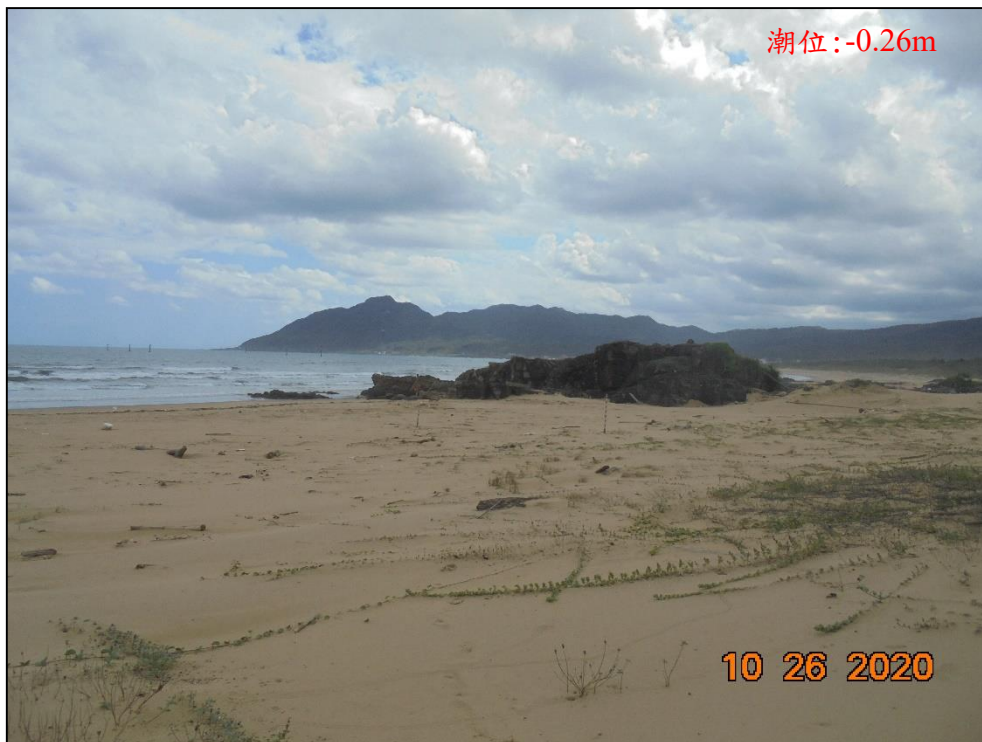
圖 4-9b 監測區南側大岩礁（黑石仔）旁防風籬地形（2020/10/26）
