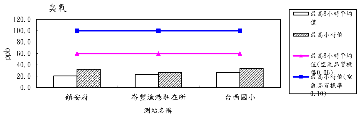
圖 2.1-5 115 年度第 2 季各測站臭氧( \text{O}_3 )最高 8 小時平均值及最高小時值比較分析圖
