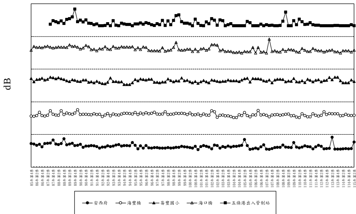
圖 3.1.3-1 本計畫歷次振動 L_{v10} 日監測結果分析圖
