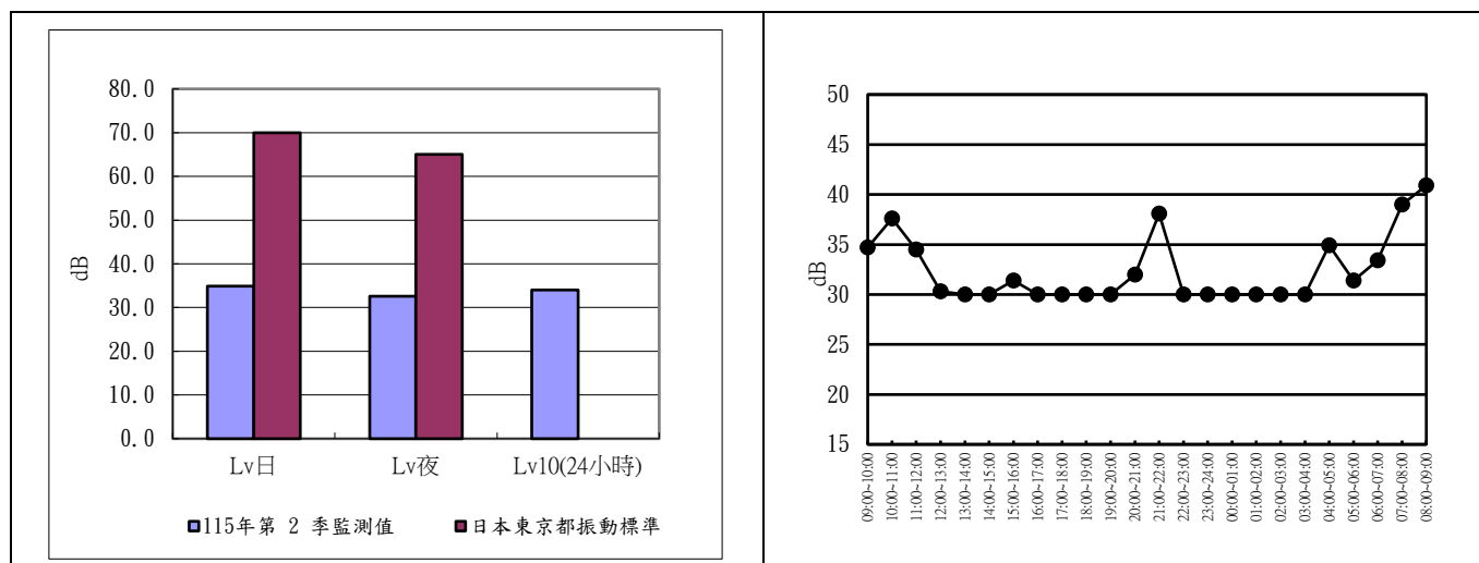
圖 2.3-4 海口橋 115 年度第 2 季振動監測成果分析圖及逐時變化圖
