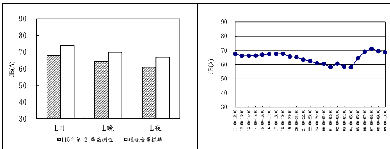
圖 2.2-2 海豐橋 115 年第 2 季噪音監測成果分析圖及逐時變化圖
