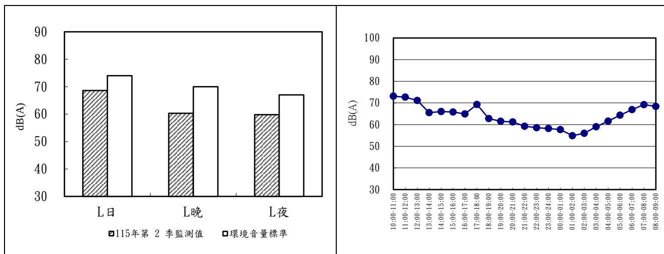
圖 2.2-1 安西府 115 年第 2 季噪音監測成果分析圖及逐時變化圖
