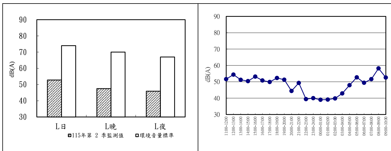
圖 2.2-5 五條港出入管制站 115 年第 2 季噪音監測成果分析圖及逐時變化圖
