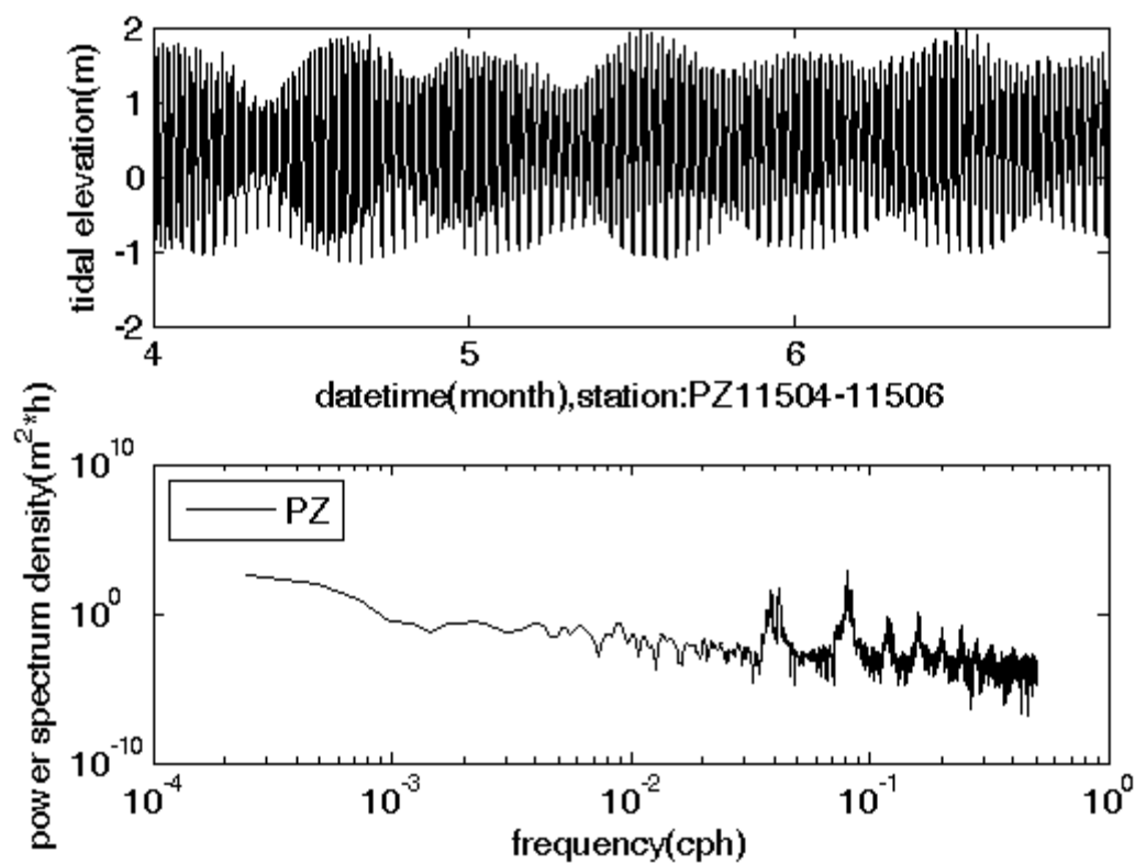
圖 2.13-4 PZ 測站 115 年 4~6 月實測潮位頻譜與逐時變化圖
