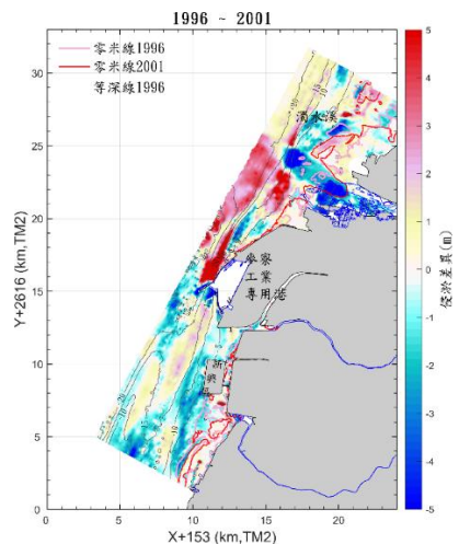
a. 85 年至 90 年地形侵淤變化
