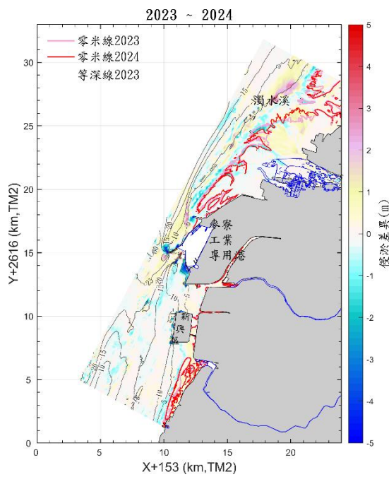
c. 112年至113年地形侵淤變化
