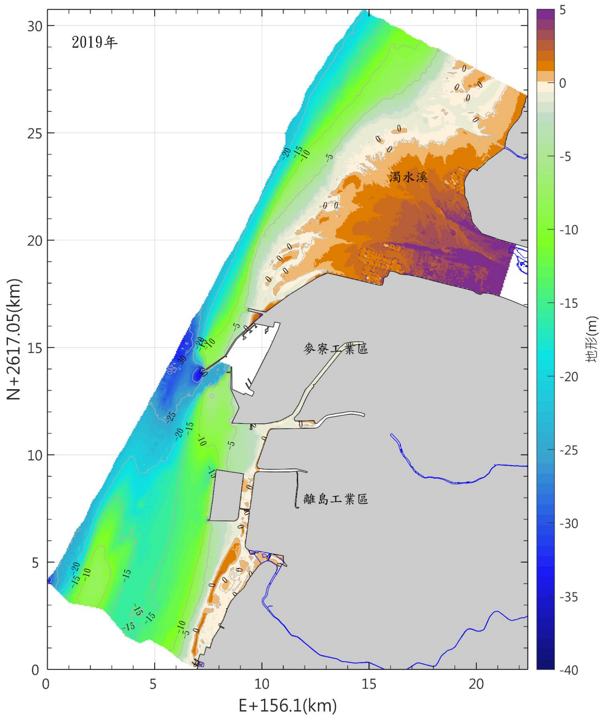
圖 3.1.12-36 本區海域 108 年海域地形圖(續)
