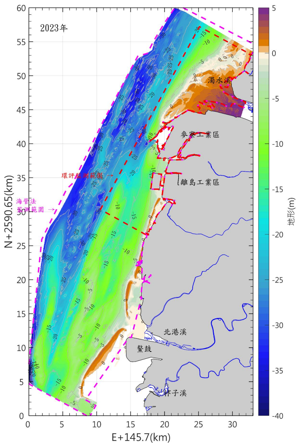
圖 3.1.12-40 本區海域 112 年海域地形圖(續)
