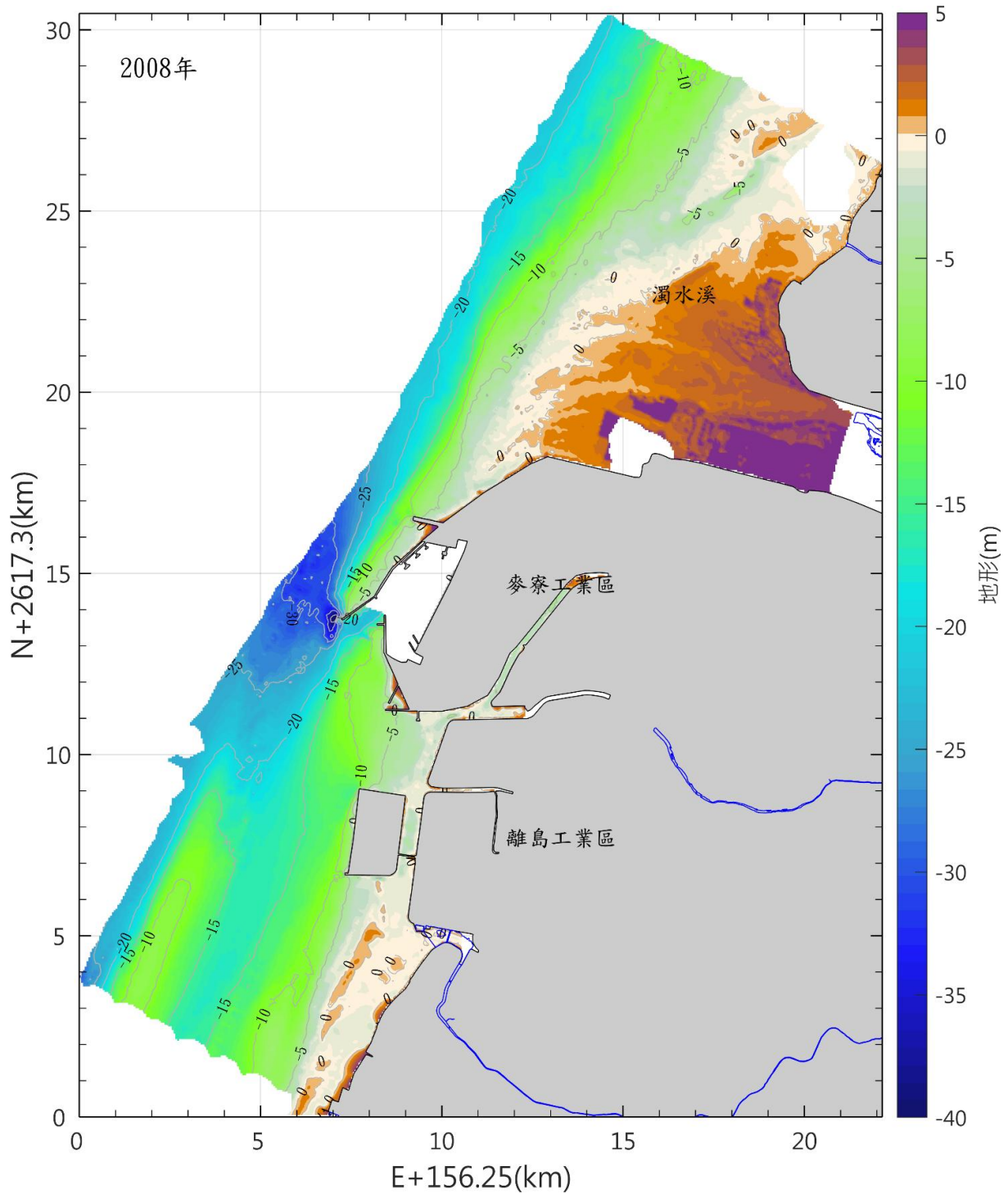
圖 3.1.12-25 本區海域 97 年海地形圖(續)
