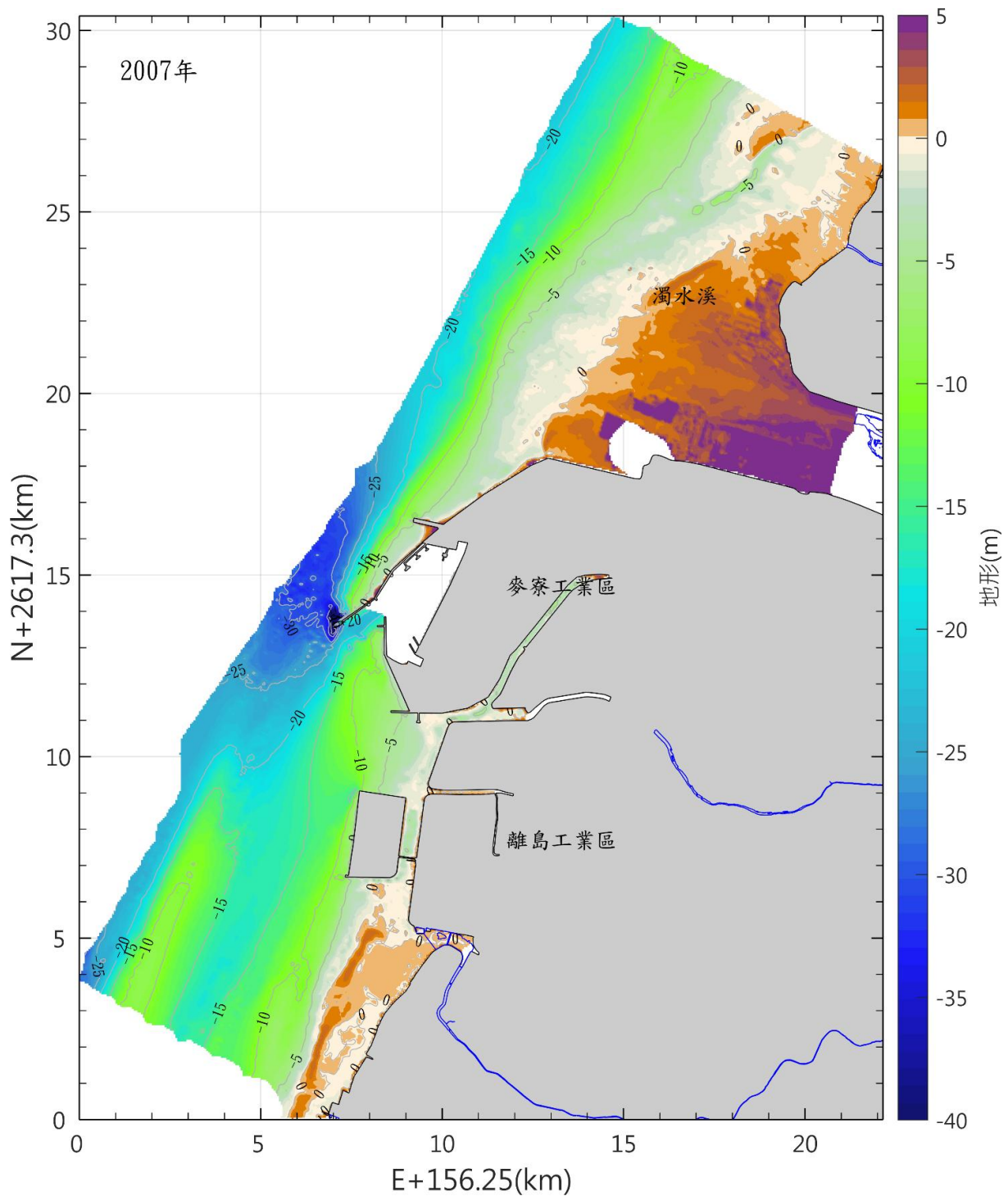
圖 3.1.12-24 本區海域 96 年海域地形圖(續)
