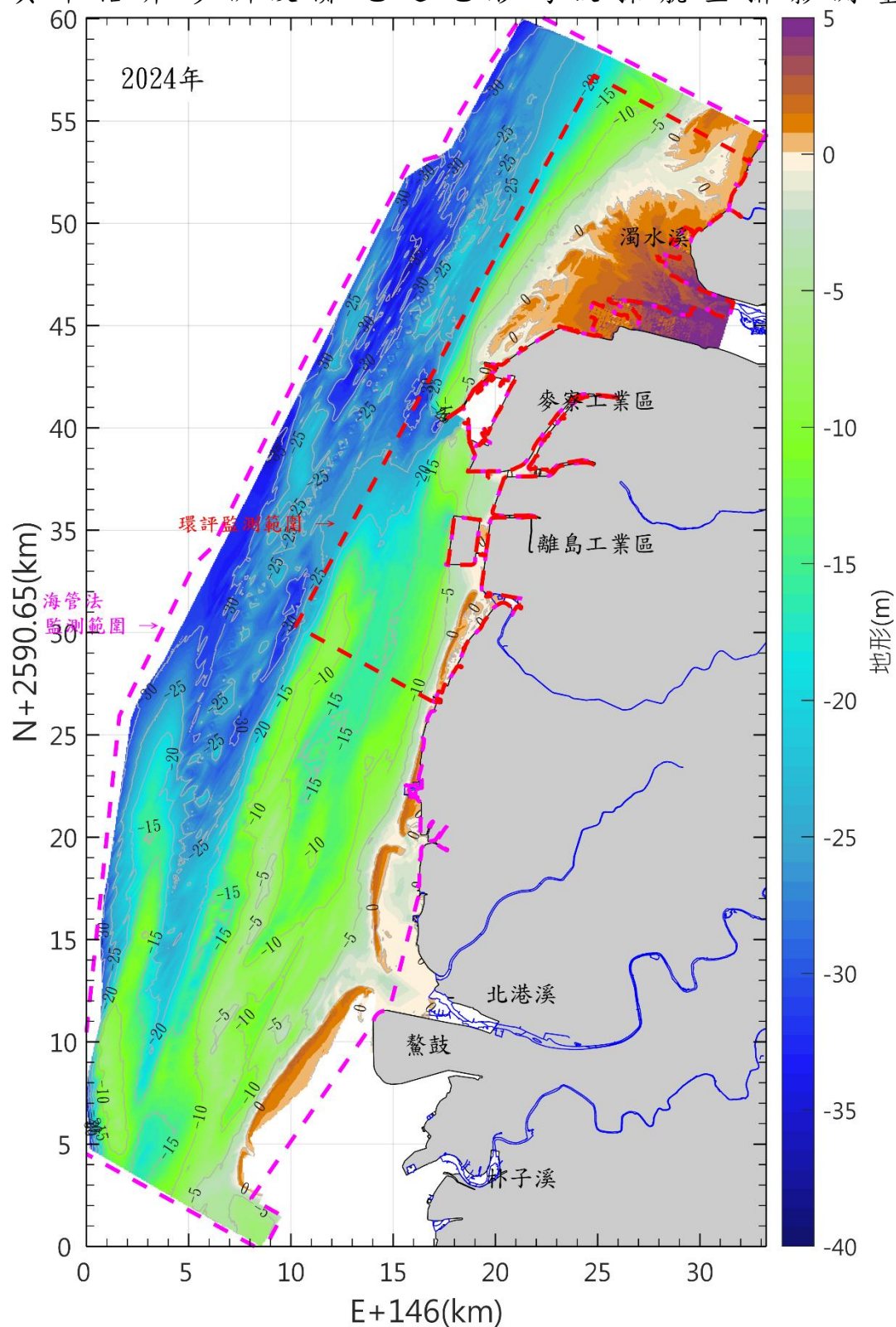
圖 3.1.12-41 本區海域 113 年海域地形圖(續)
