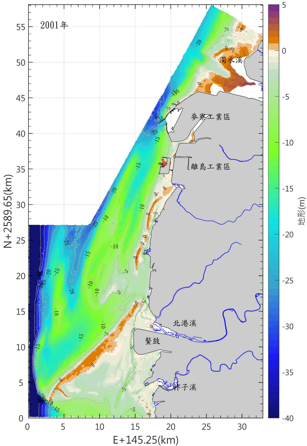
圖 3.1.12-18 本區海域 90 年海域地形圖(續)
