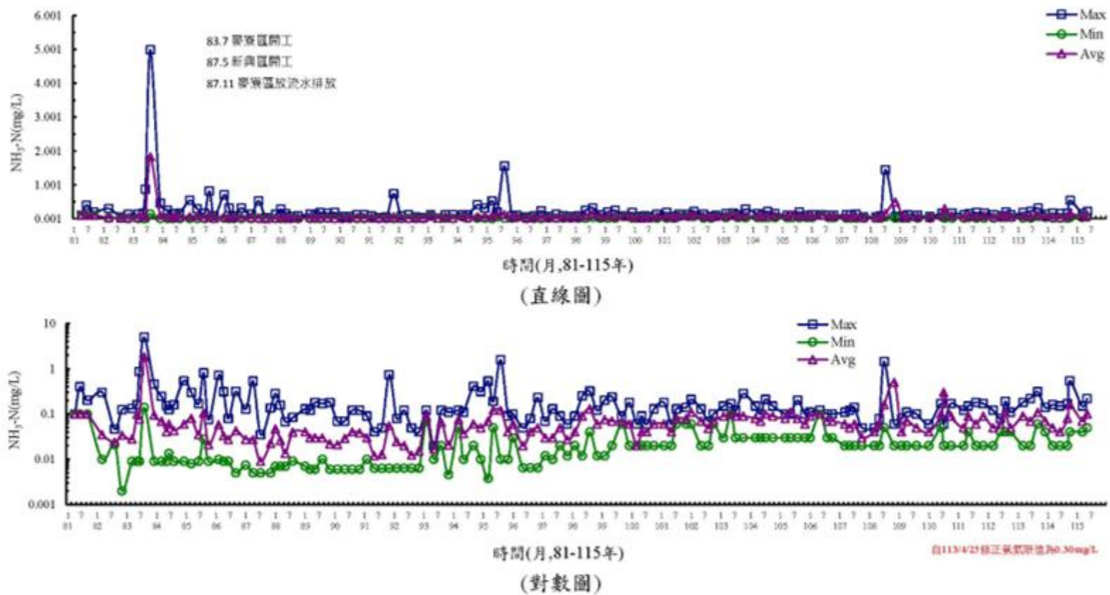
圖 3.1.9-8 離島產業園區海域歷年水質變化圖( \text{NH}_3\text{-N} )
