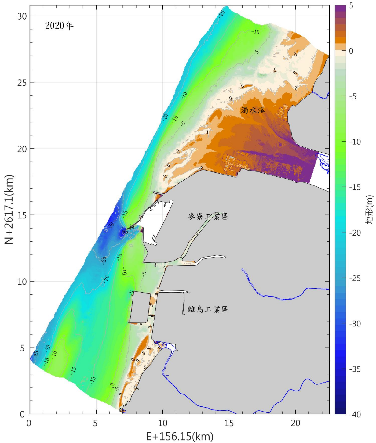
圖 3.1.12-37 本區海域 109 年海域地形圖(續)
