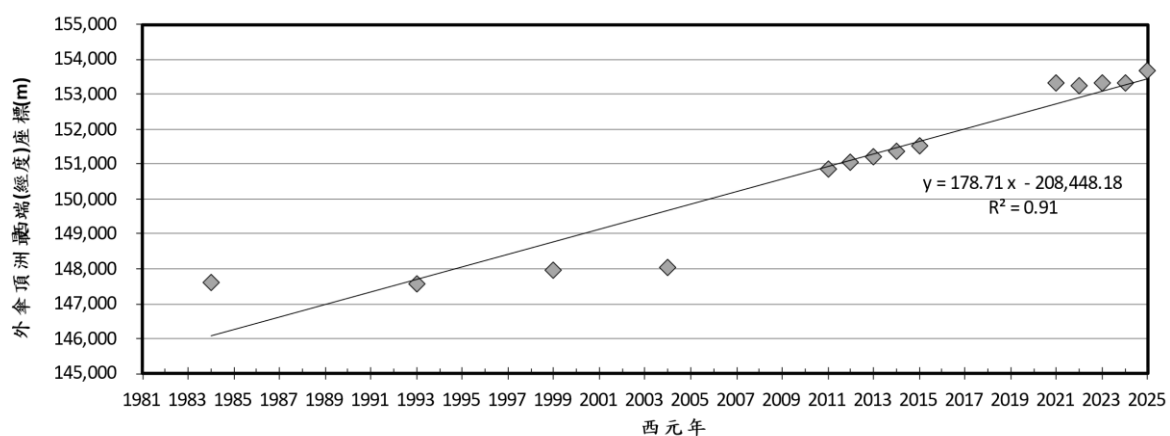
圖 3.1.12-10 外傘頂洲最北端南移變化(73~114)
