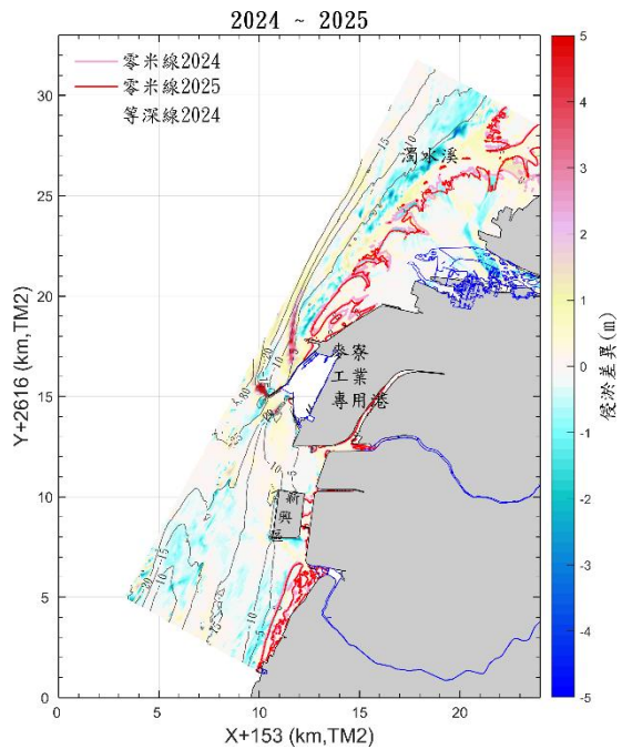
d. 113年至114年地形侵淤變化
