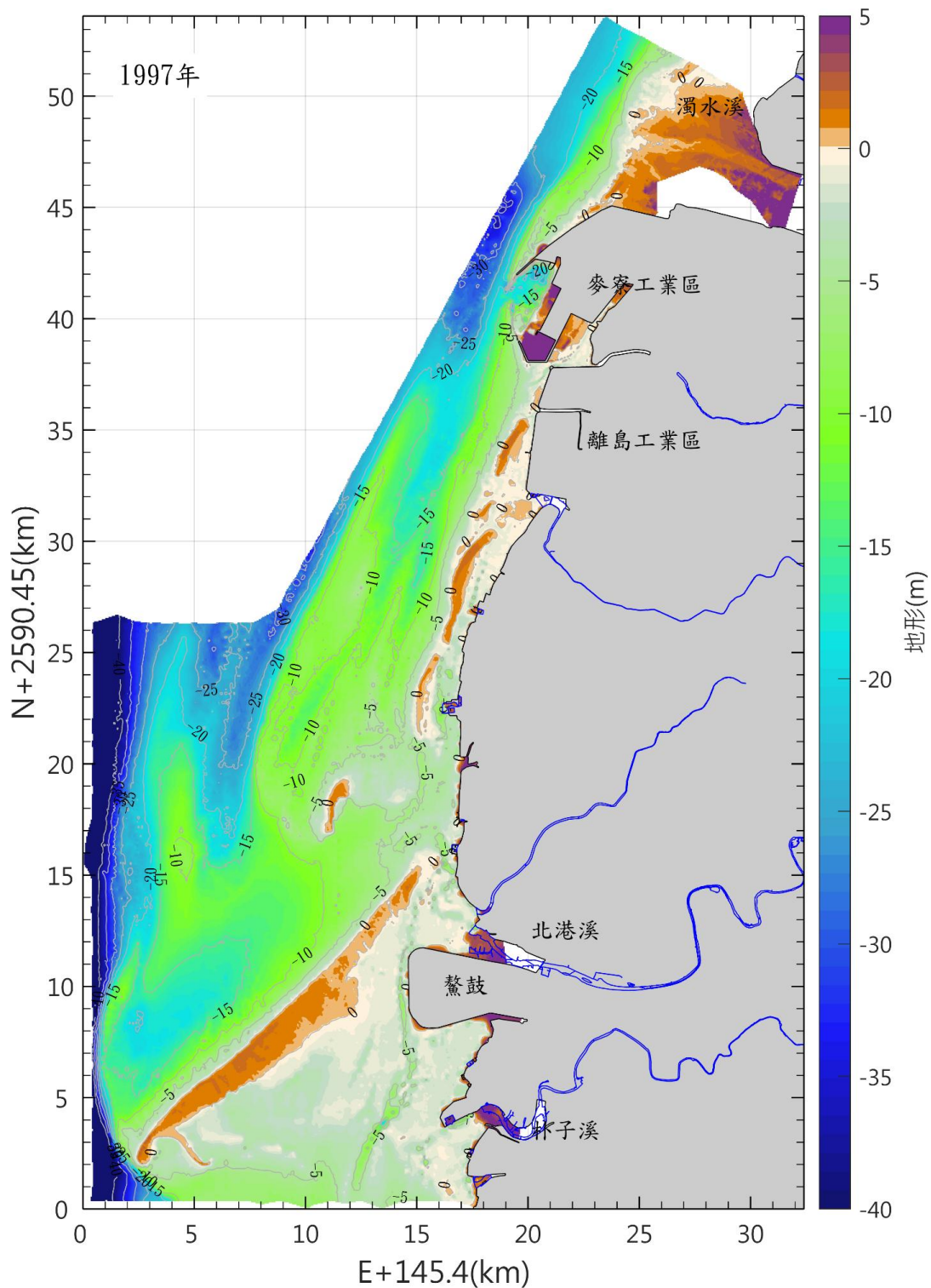
圖 3.1.12-14 本區海域 86 年海域地形圖(續)
