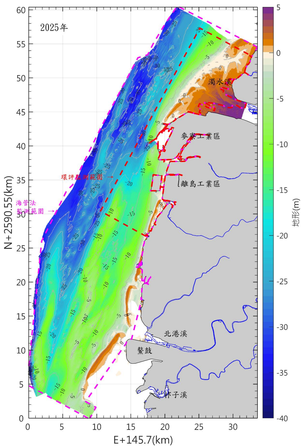
圖 3.1.12-42 本區海域 114 年海域地形圖(續)
