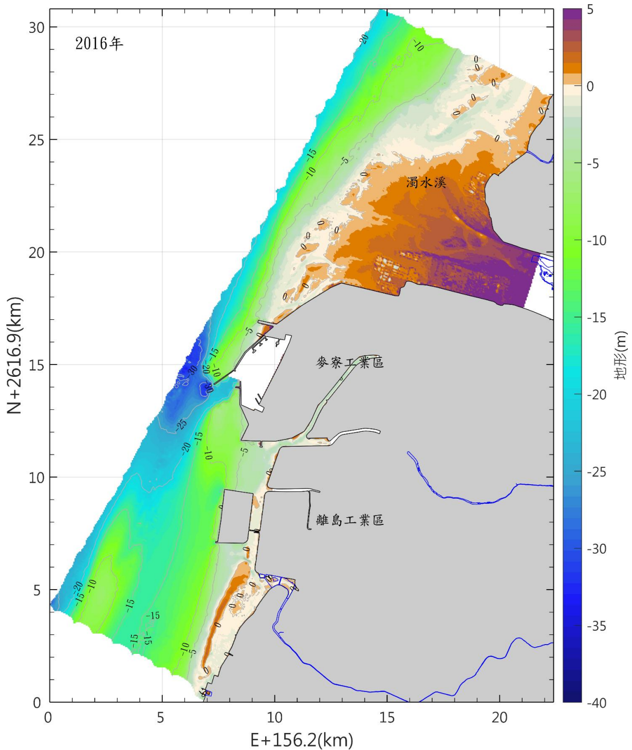
圖 3.1.12-33 本區海域 105 年海域地形圖(續)
