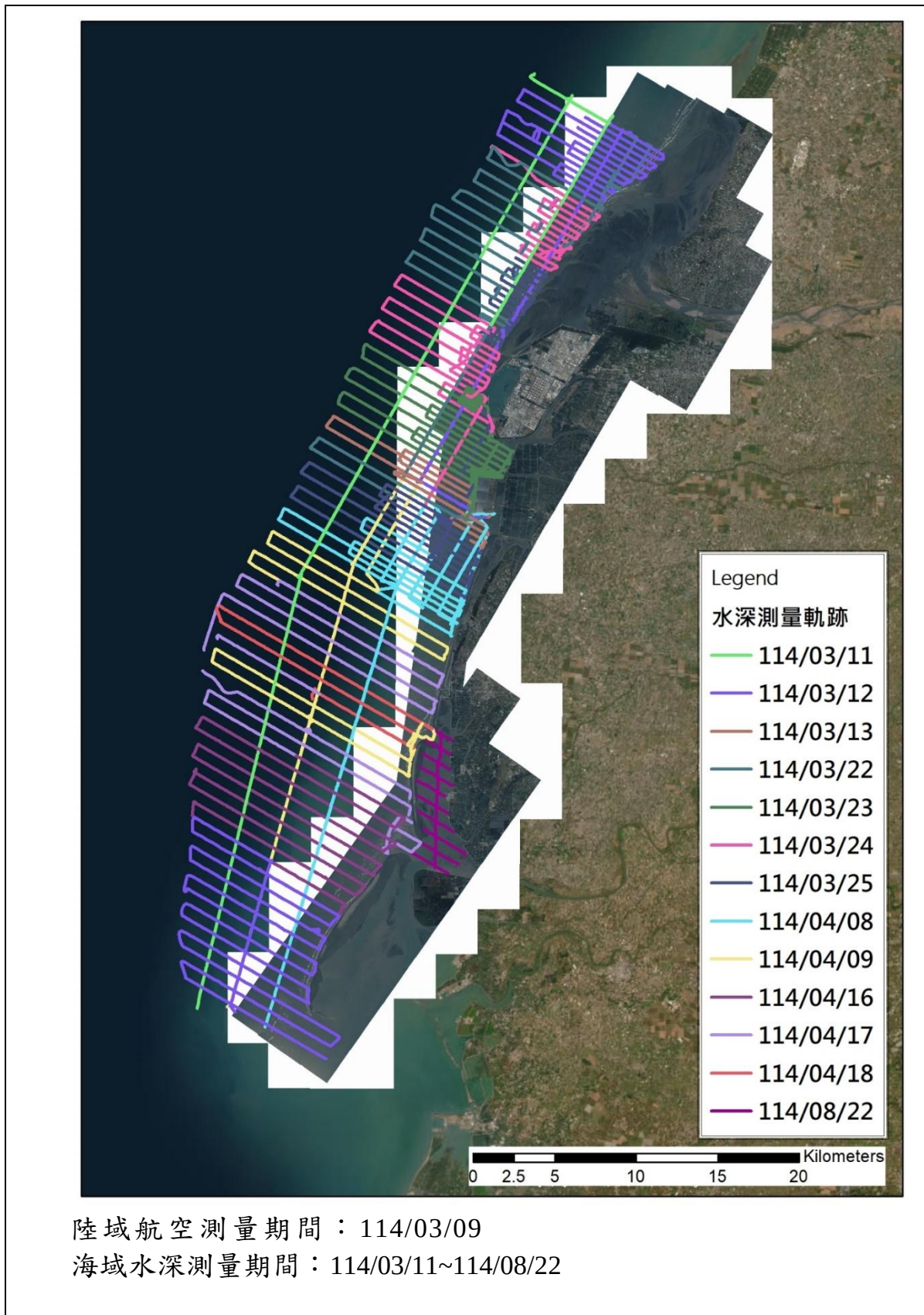
圖 2.12-1 本區海域 114 年海域地形圖
