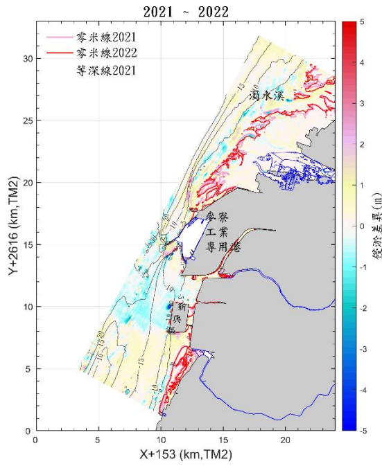
a. 110年至111年地形侵淤變化
