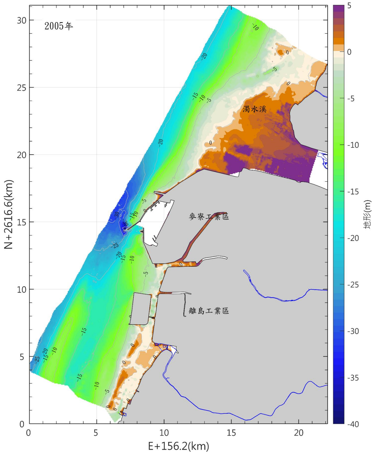
圖 3.1.12-22 本區海域 94 年海域地形圖(續)
