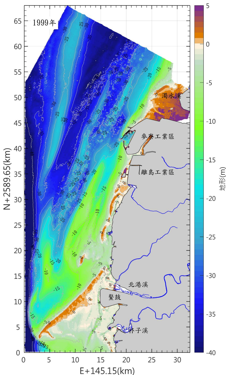
圖 3.1.12-16 本區海域 88 年海域地形圖(續)
