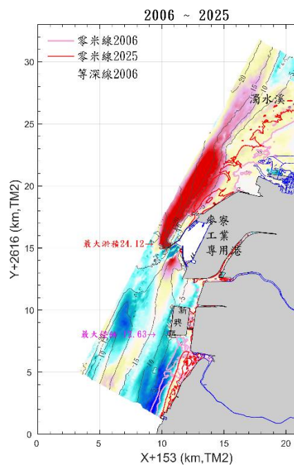
c.95年至114年地形侵淤變化
