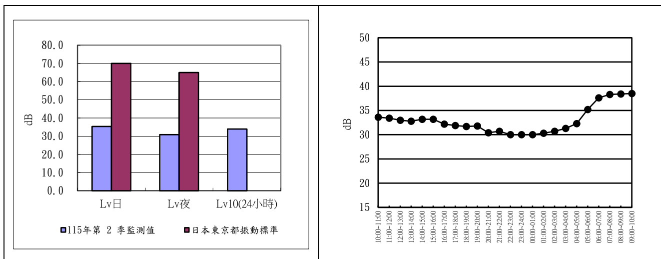
圖 2.3-2 海豐橋 115 年度第 2 季振動監測成果分析圖及逐時變化圖
