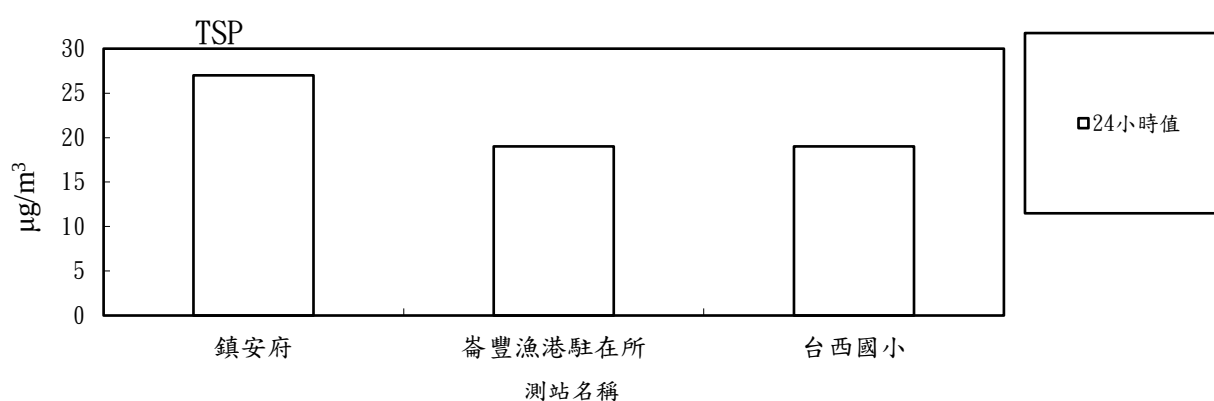
圖 2.1-8 115 年度第 2 季各測站 TSP 24 小時值比較分析圖
