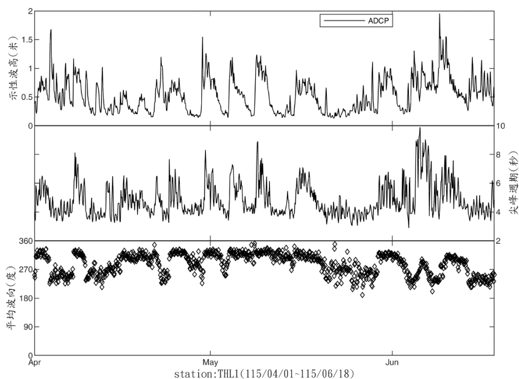
圖 2.13-6 THL1 測站 115 年 4 月~115 年 6 月波浪時序列
