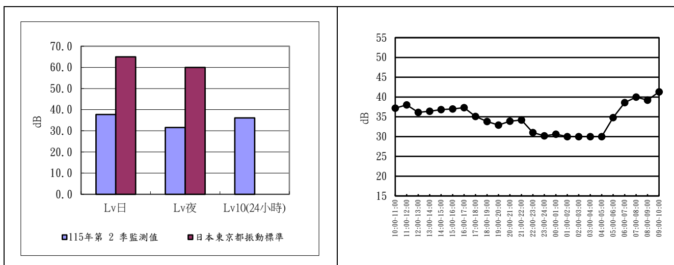
圖 2.3-3 崙豐國小 115 年度第 2 季振動監測成果分析圖及逐時變化圖
