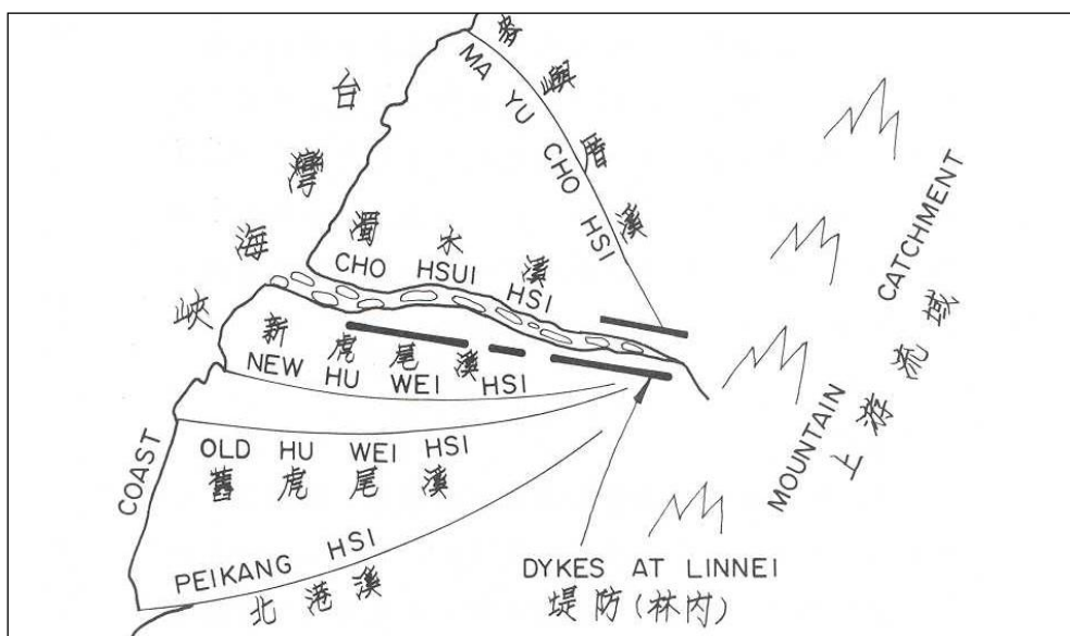
圖 3.1.12-2 濁水溪河系治導計畫示意圖
