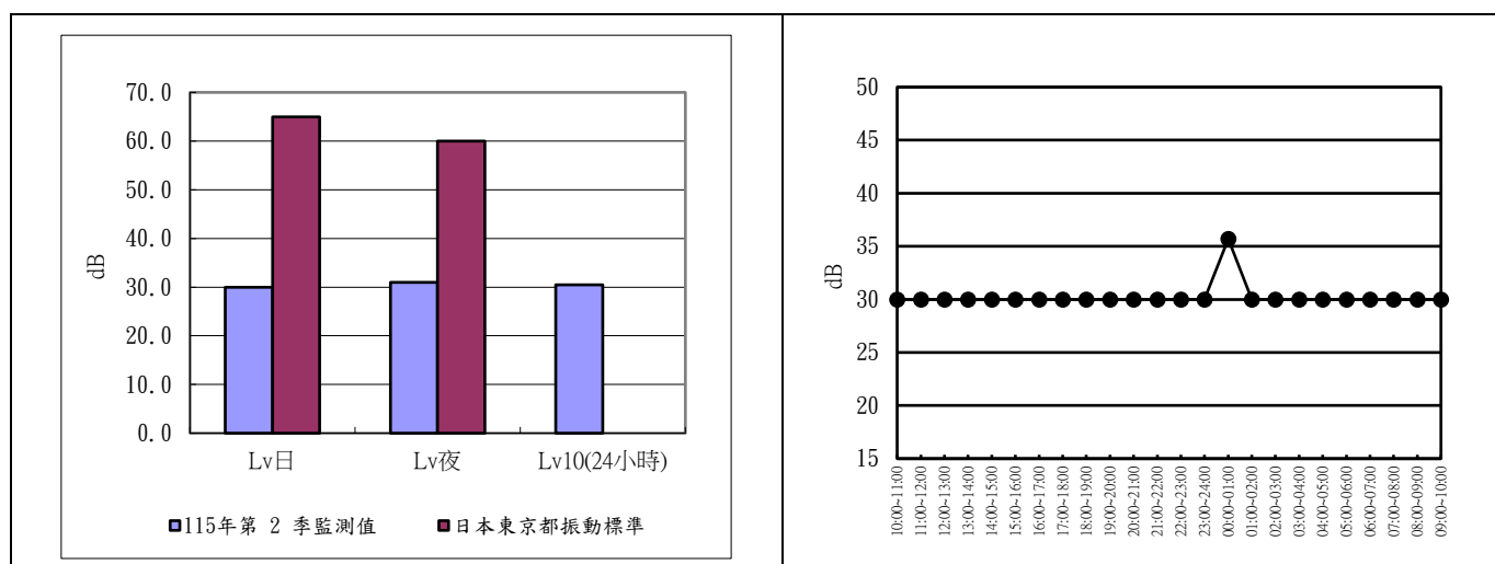
圖 2.3-5 五條港出入管制 115 年度第 2 季振動監測成果分析圖及逐時變化圖
