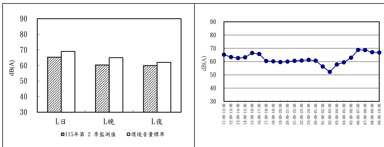
圖 2.2-3 崙豐國小 115 年第 2 季噪音監測成果分析圖及逐時變化圖
