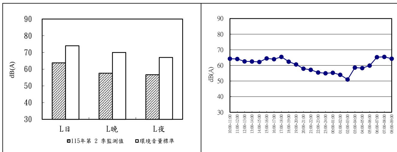
圖 2.2-4 海口橋 115 年第 2 季噪音監測成果分析圖及逐時變化圖
