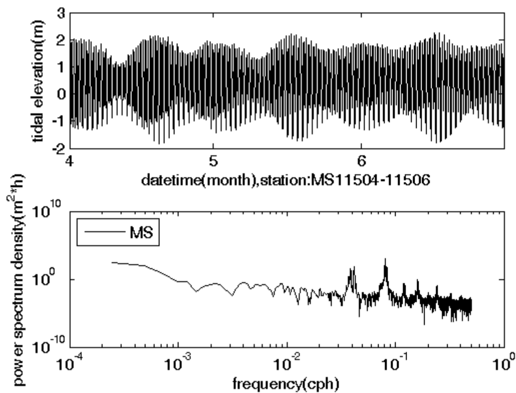
圖 2.13-3 MS 測站 115 年 4~6 月實測潮位頻譜與逐時變化圖
