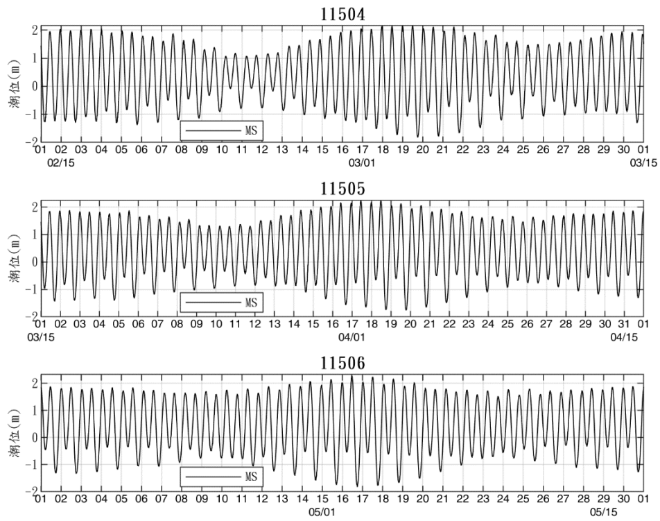
圖 2.13-1 MS 測站 115 年 4~6 月各月實測潮位逐時變化圖
