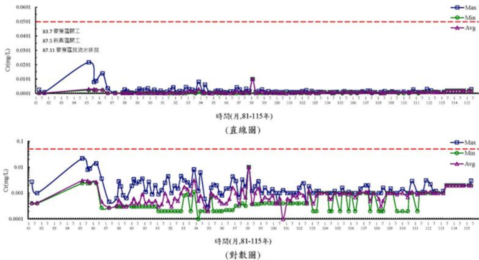
圖 3.1.9-18 離島產業園區海域歷年水質變化圖(Cr)
