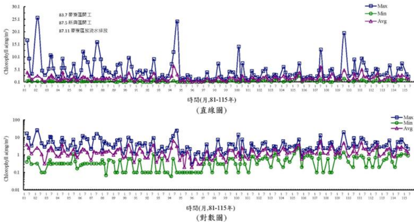
圖 3.1.9-13 離島產業園區海域歷年水質變化圖(Chlorophyll a)
