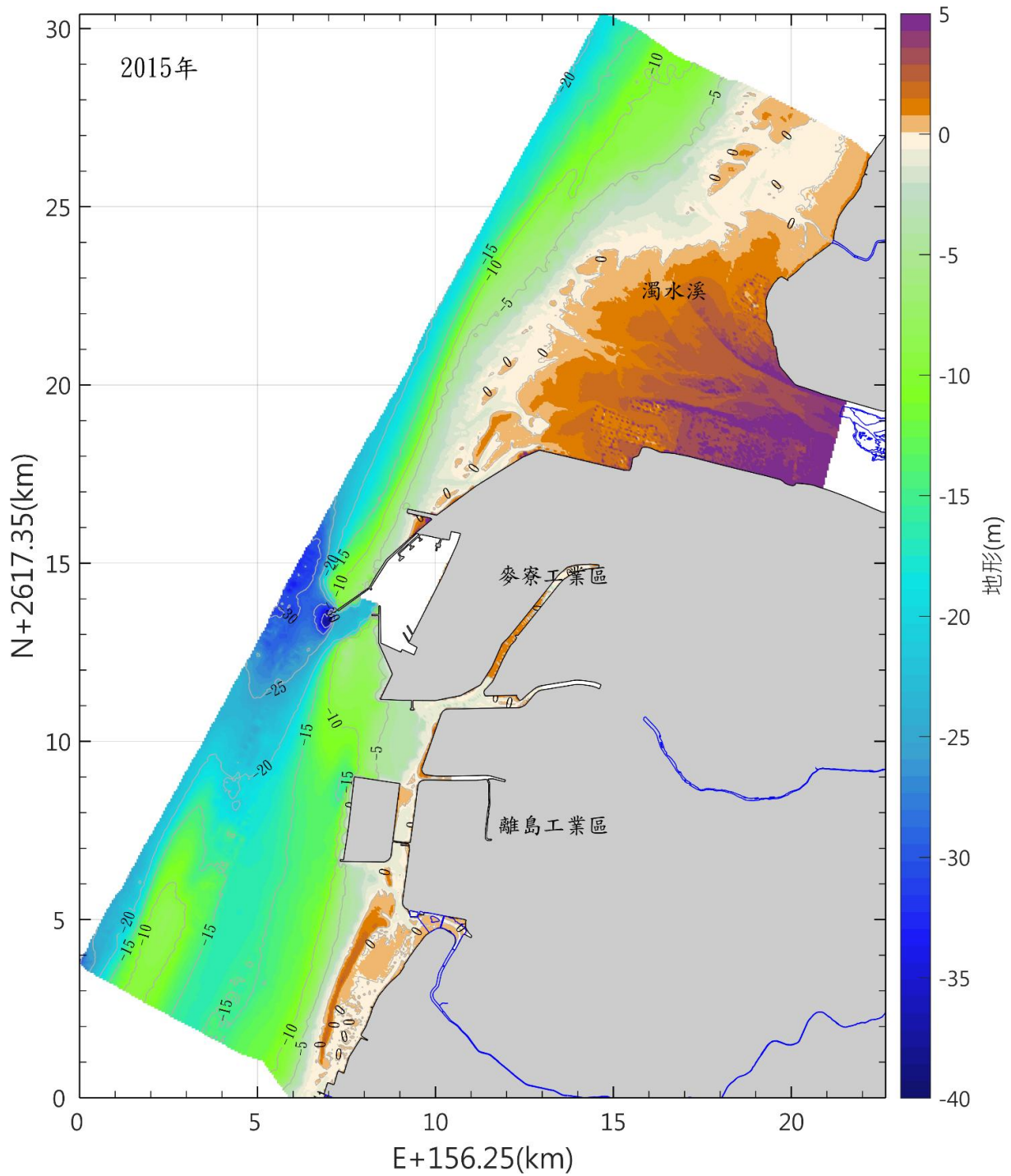
圖 3.1.12-32 本區海域 104 年海域地形圖(續)
