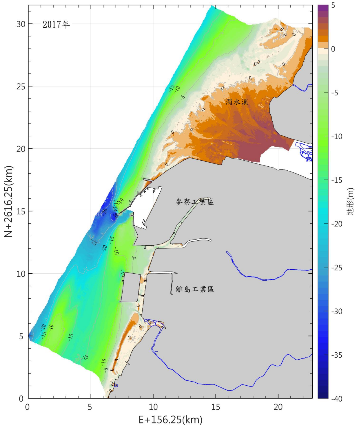
圖 3.1.12-34 本區海域 106 年海域地形圖(續)
