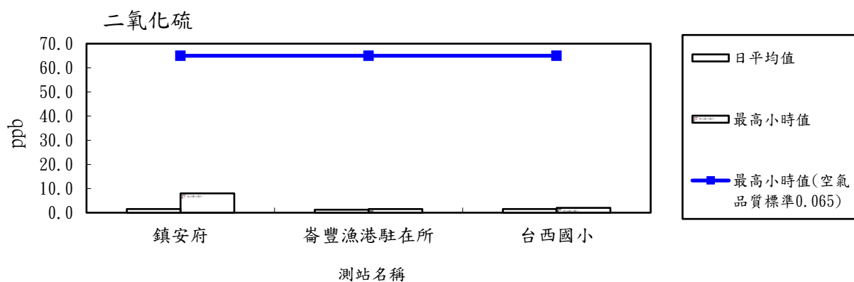
圖 2.1-2 115 年度第 2 季各測站二氧化硫(SO 2 )最高小時值比較分析圖
