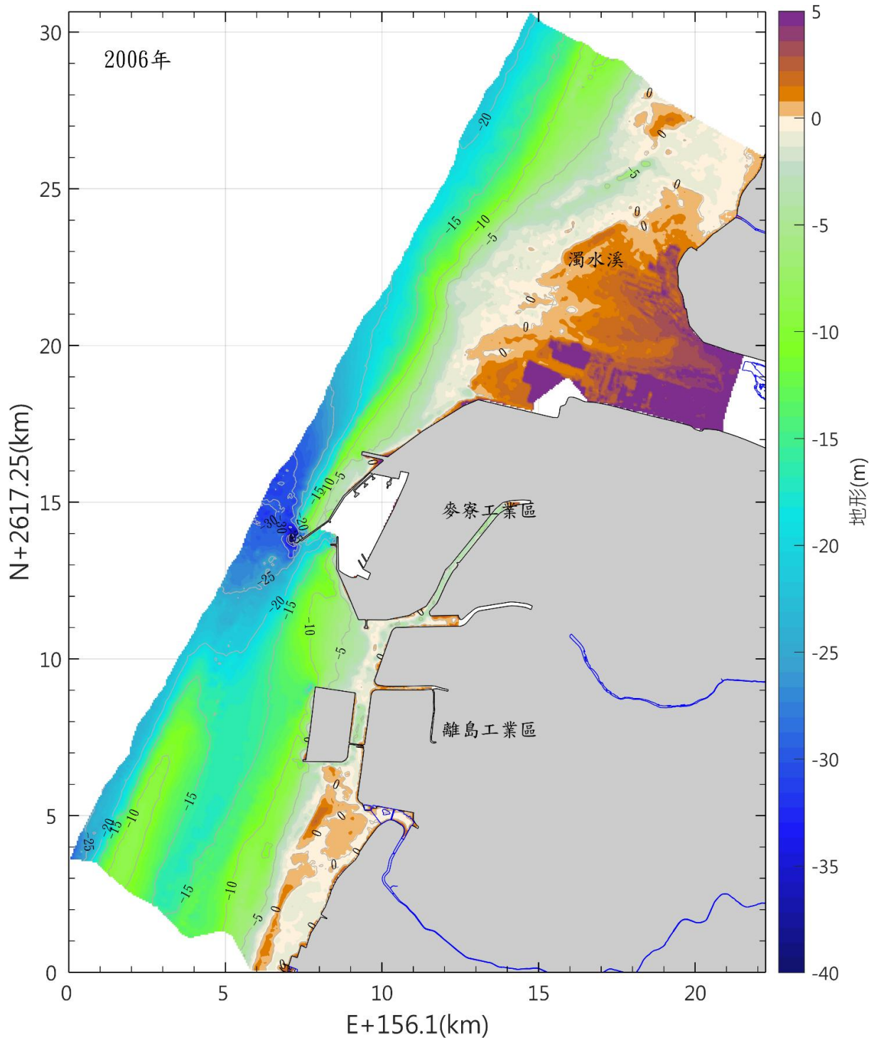
圖 3.1.12-23 本區海域 95 年海域地形圖(續)
