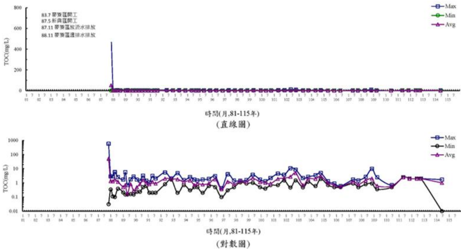
圖 3.1.9-24 離島產業園區海域歷年水質變化圖(TOC)
