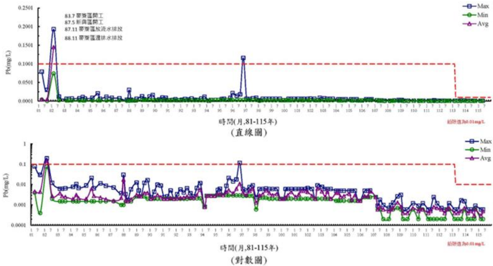
圖 3.1.9-16 離島產業園區海域歷年水質變化圖(Pb)
