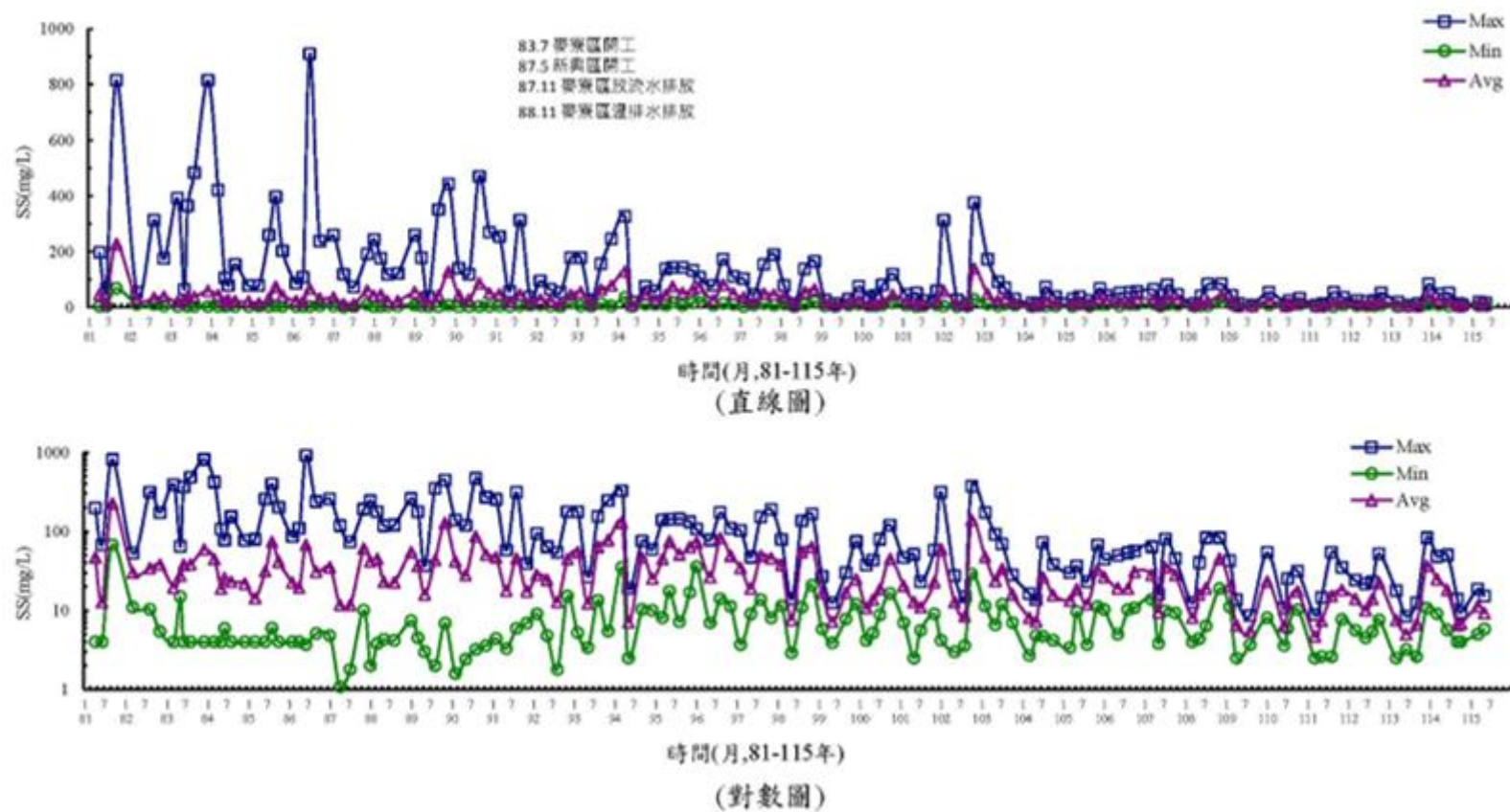
圖 3.1.9-5 離島產業園區海域歷年水質變化圖(SS)
