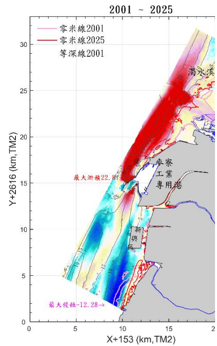
b.90年至114年地形侵淤變化
