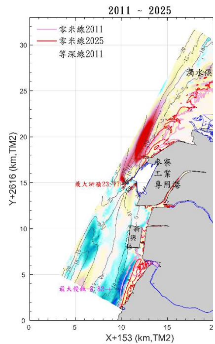
d.100年至114年地形侵淤變化
