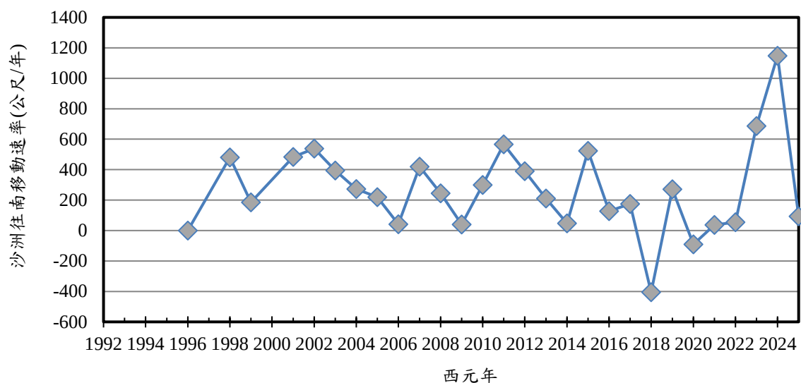
圖 3.1.12-7 三條崙沙洲最南端每年變遷速率
