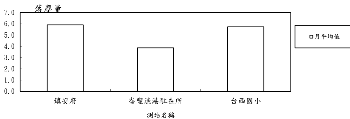
圖 2.1-10 115 年度第 2 季各測站落塵量平均值比較分析圖
