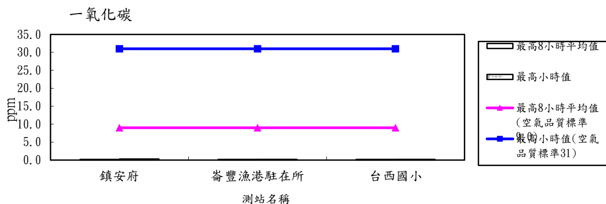
圖 2.1-1 115 年度第 2 季各測站一氧化碳(CO)最高 8 小時平均值及最高小時值比較分析圖
