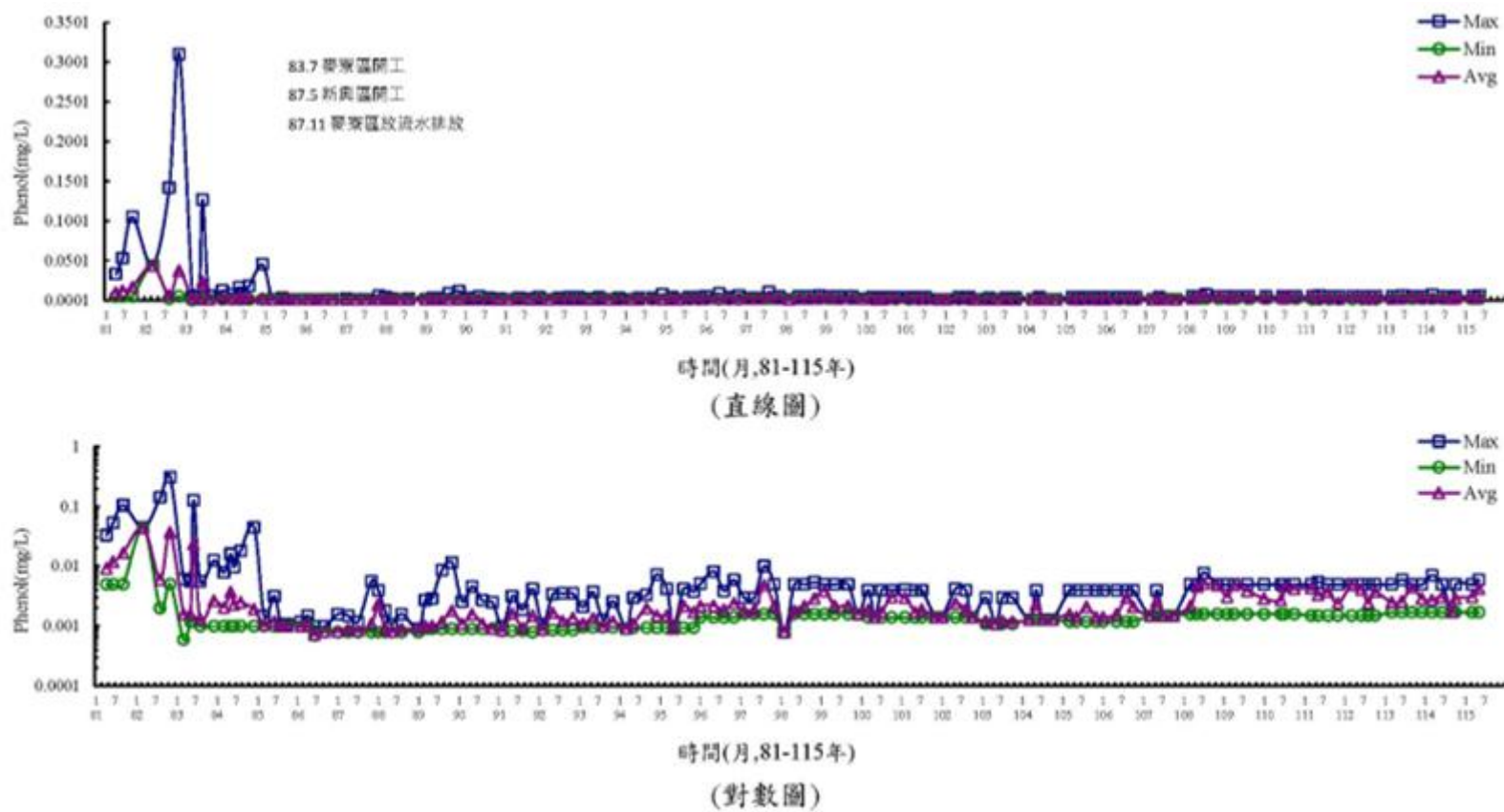
圖 3.1.9-11 離島產業園區海域歷年水質變化圖(Phenol)
