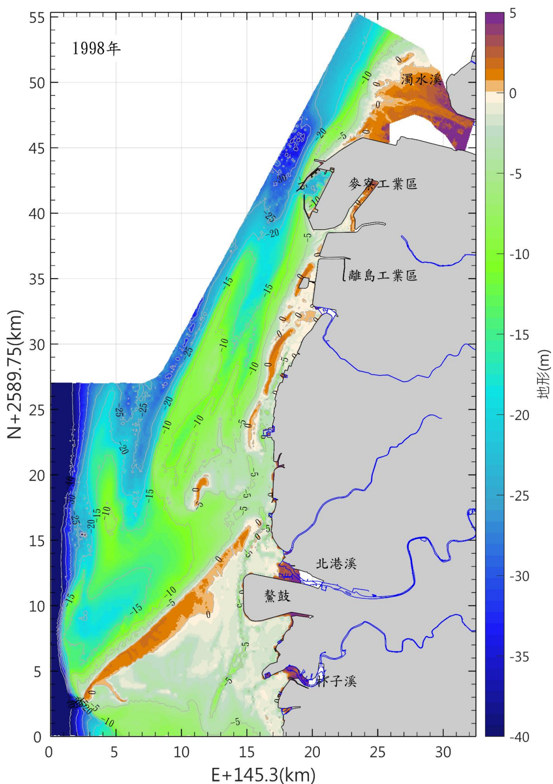
圖 3.1.12-15 本區海域 87 年海域地形圖(續)
