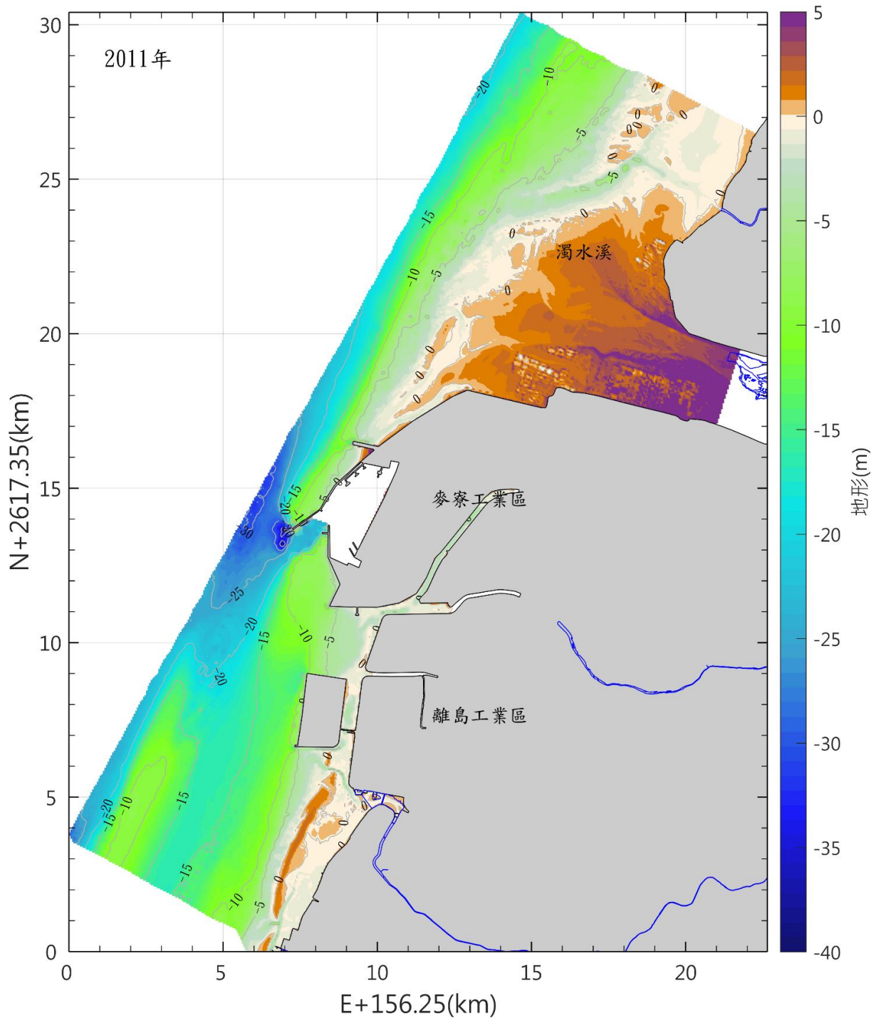
圖 3.1.12-28 本區海域 100 年海域地形圖(續)
