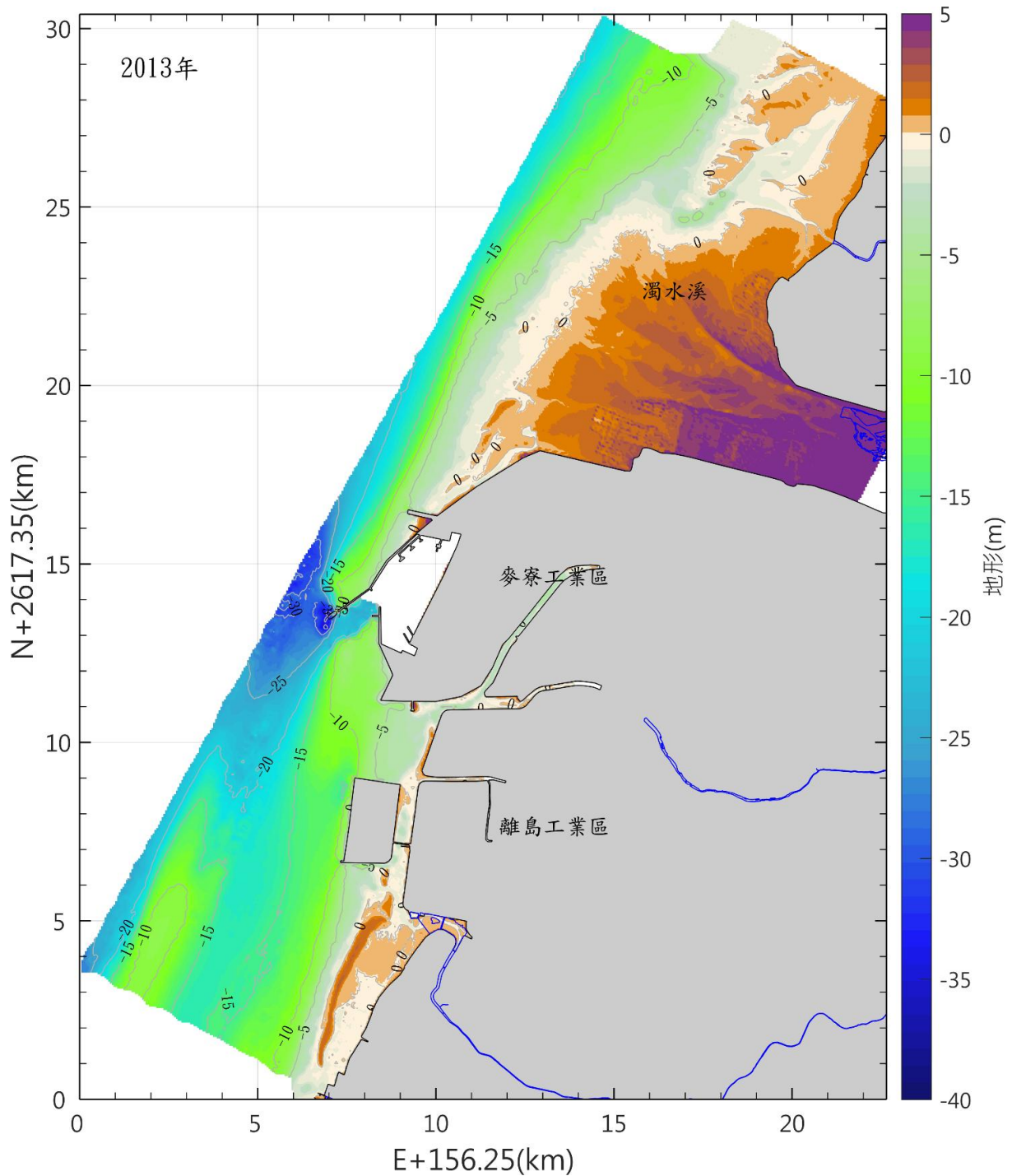
圖 3.1.12-30 本區海域 102 年海域地形圖(續)
