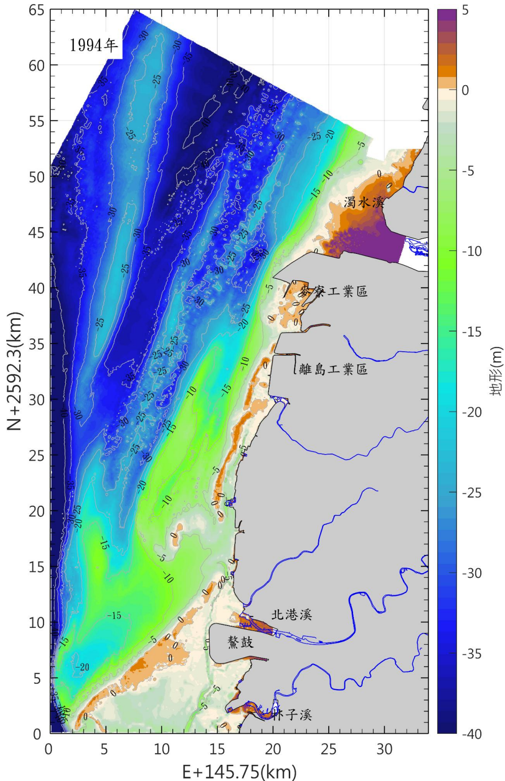
圖 3.1.12-12 本區海域 83 年海域地形圖(續)
