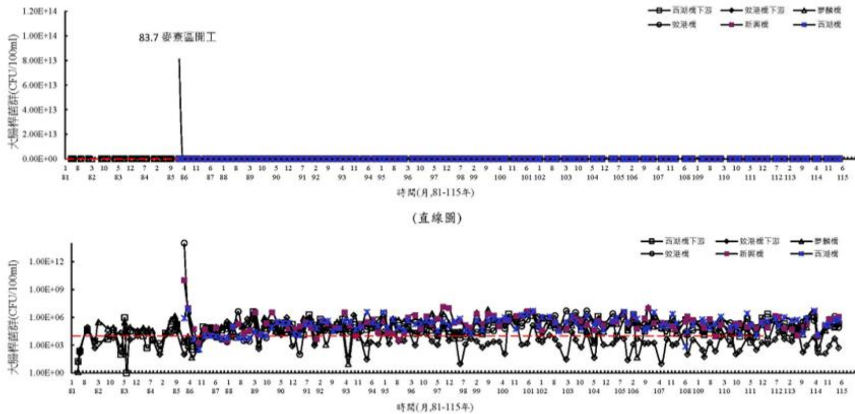
圖 3.1.8-1 離島產業園區陸域河口歷年水質變化圖(續 7)
