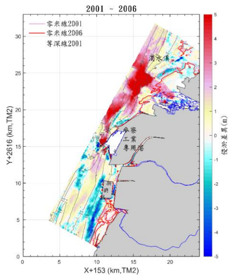
b. 90 年至 95 年地形侵淤變化
