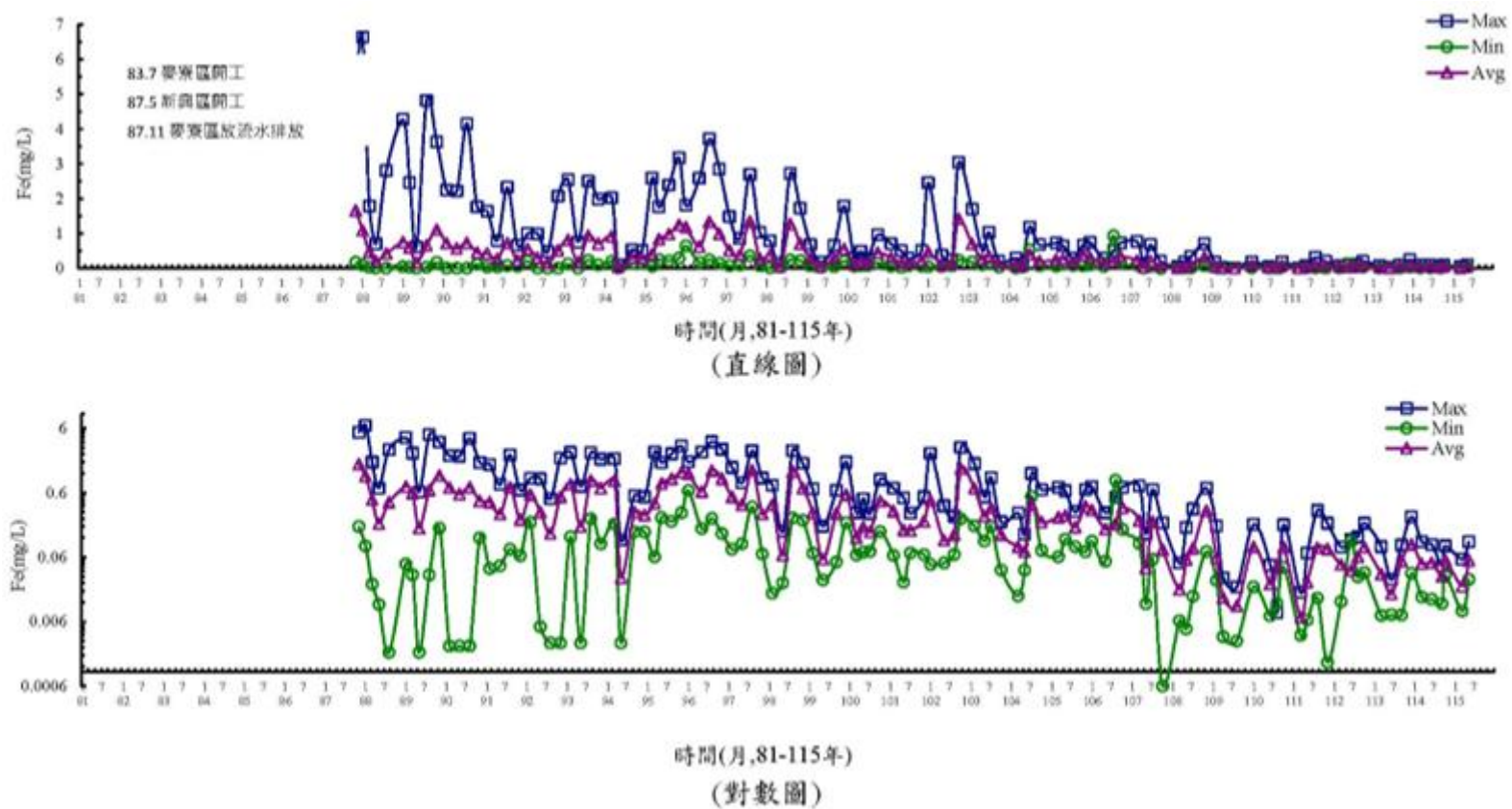
圖 3.1.9-27 離島產業園區海域歷年水質變化圖(Fe)
