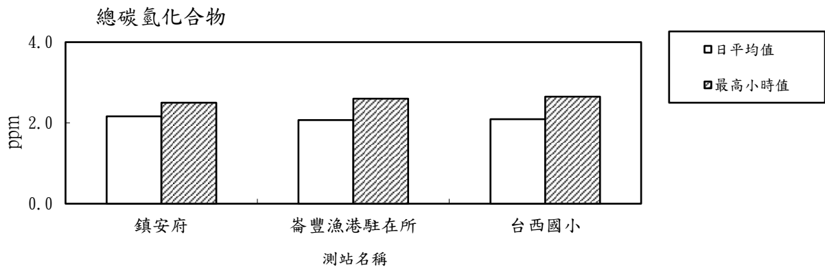
圖 2.1-6 115 年度第 2 季各測站總碳氫化合物(THC)日平均值及最高小時值比較分析圖
