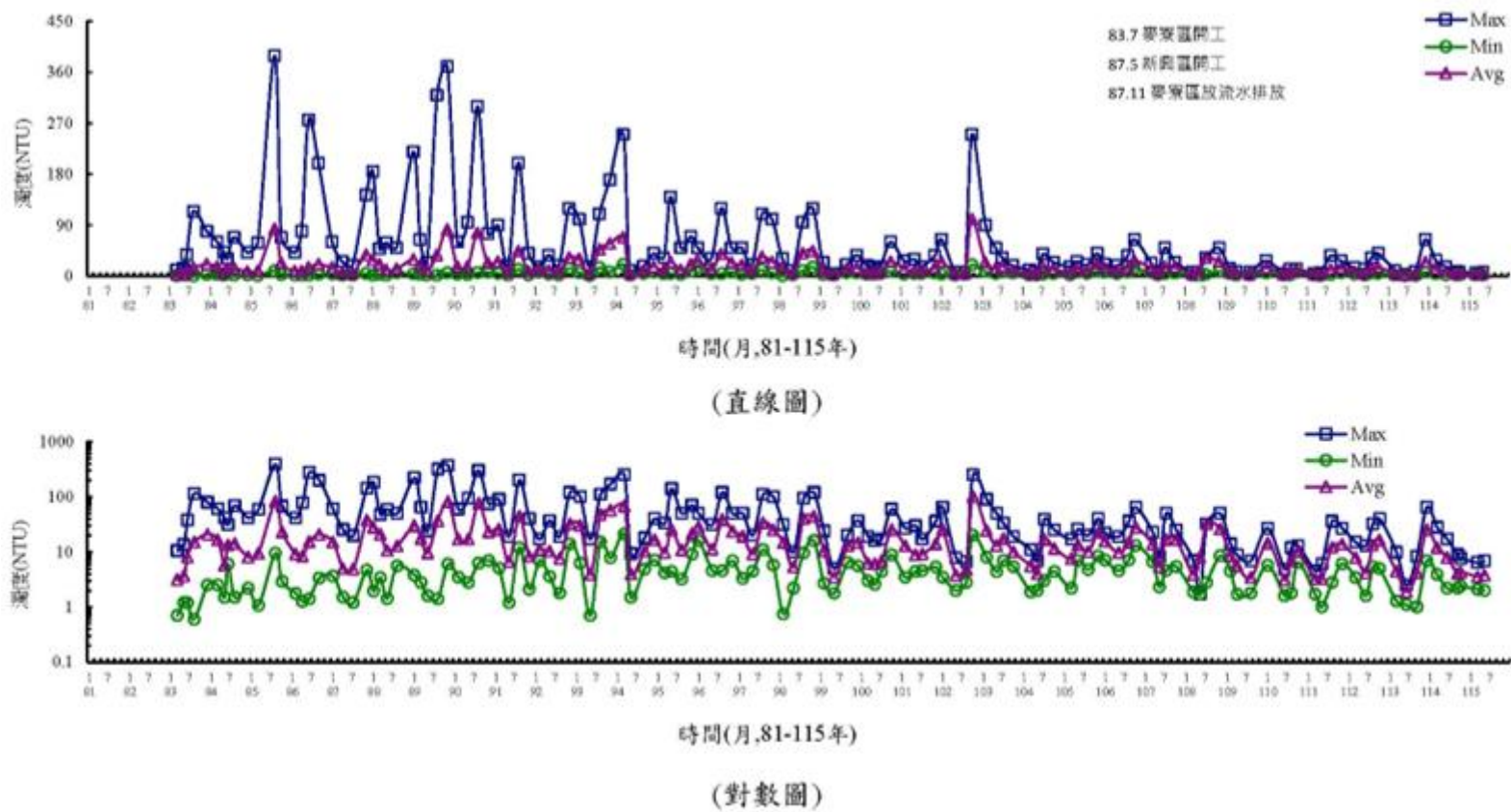
圖 3.1.9-6 離島產業園區海域歷年水質變化圖(濁度)
