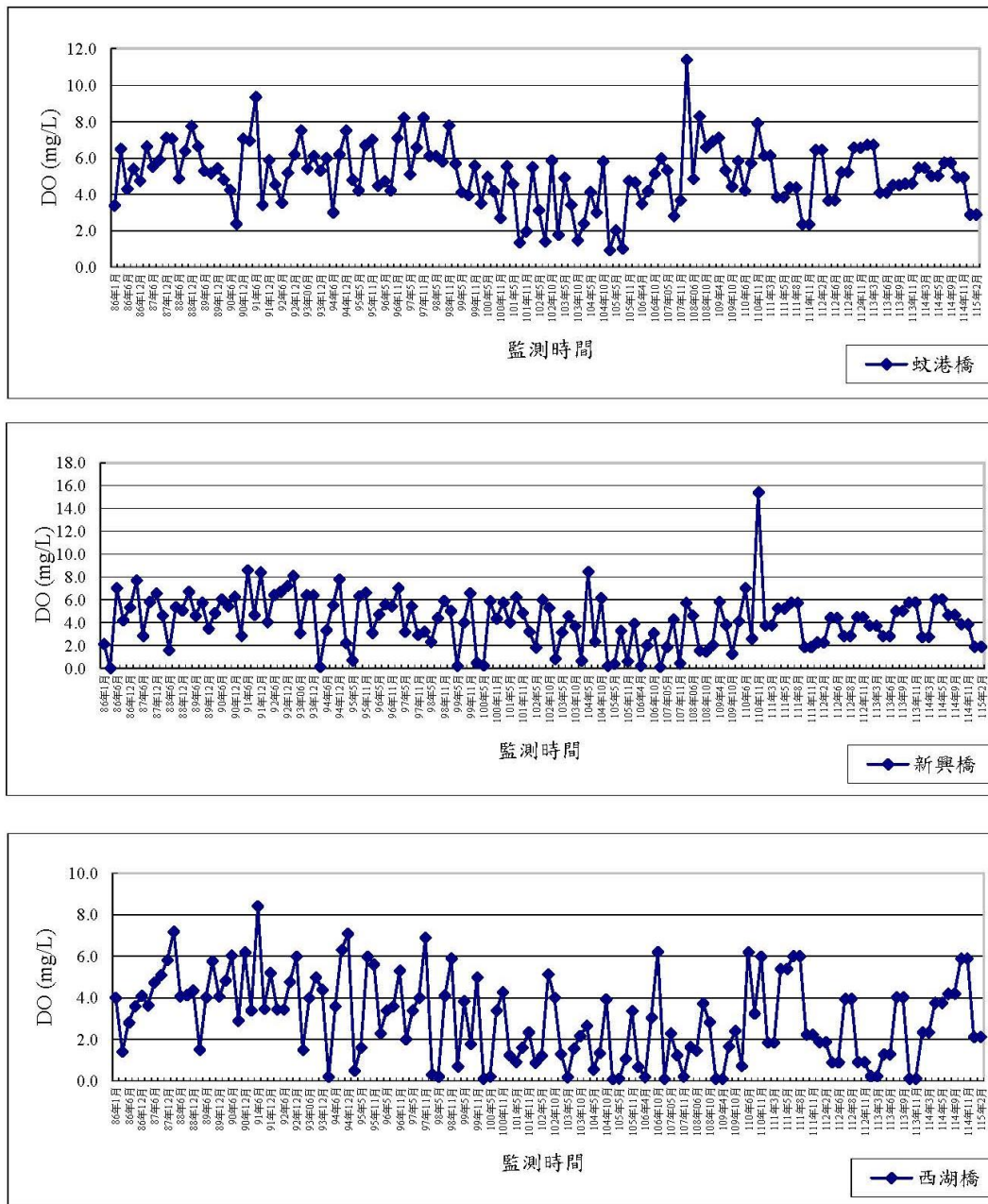
圖 3.1.7-2 陸域水質歷次溶氧比較分析圖
