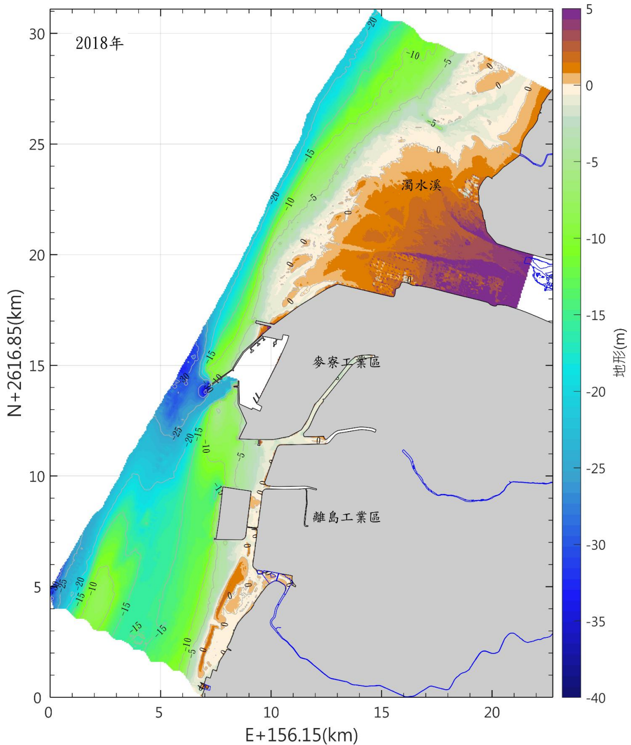
圖 3.1.12-35 本區海域 107 年海域地形圖(續)
