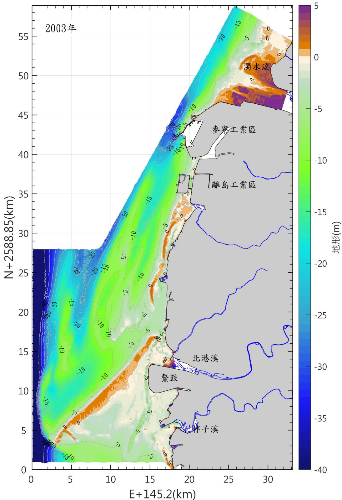
圖 3.1.12-20 本區海域 92 年海域地形圖(續)
