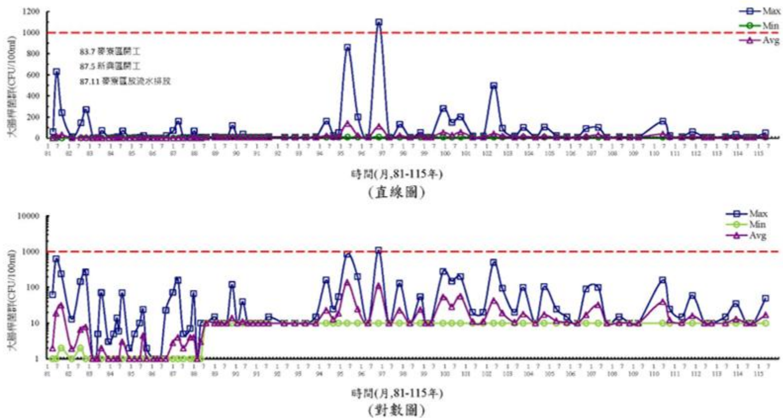
圖 3.1.9-7 離島產業園區海域歷年水質變化圖(大腸桿菌群)
