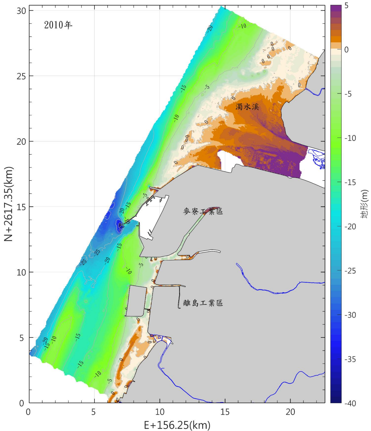
圖 3.1.12-27 本區海域 99 年海地形圖(續)
