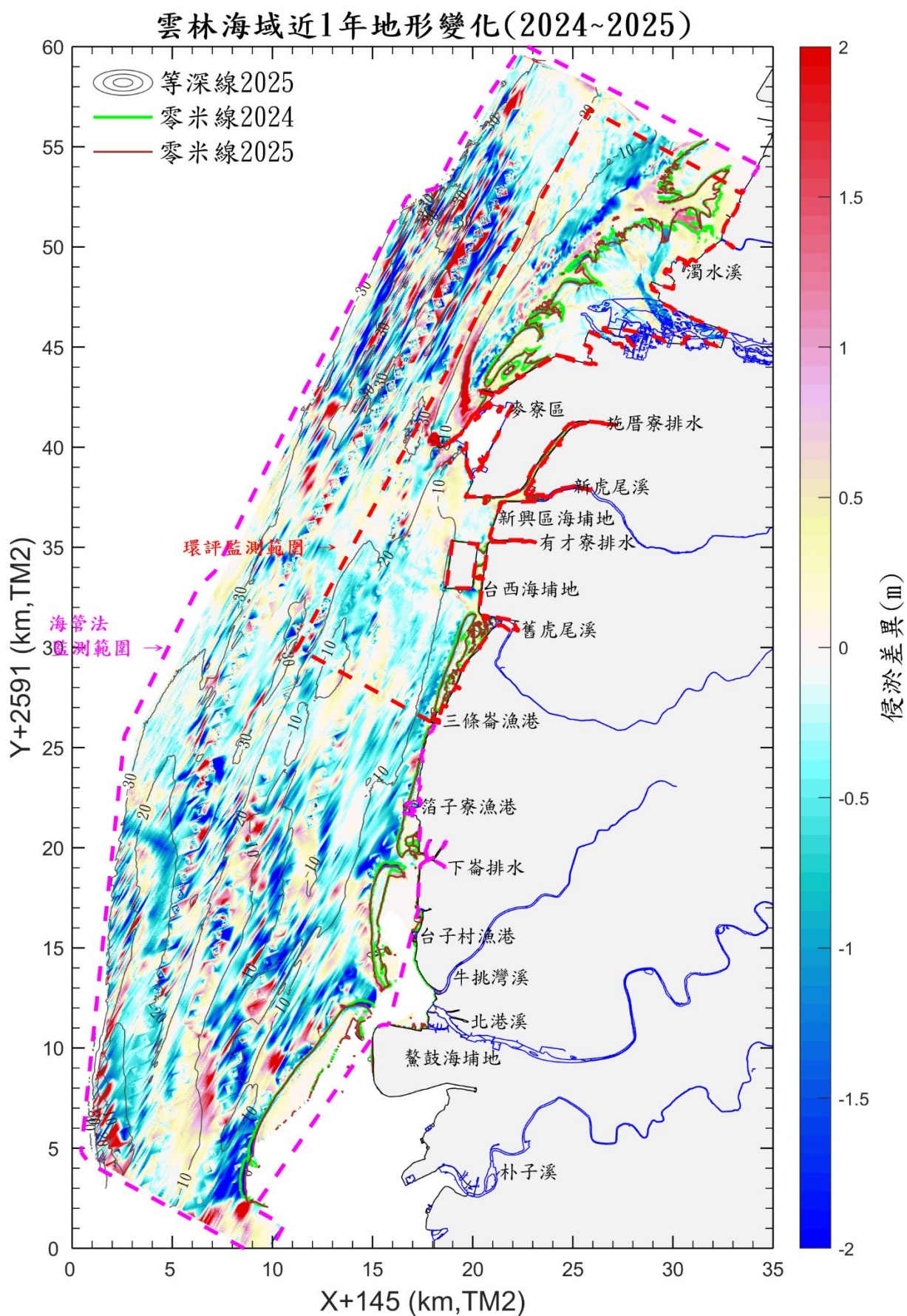
圖 2.12-3 本區地形測量變動量計算圖(113~114)
