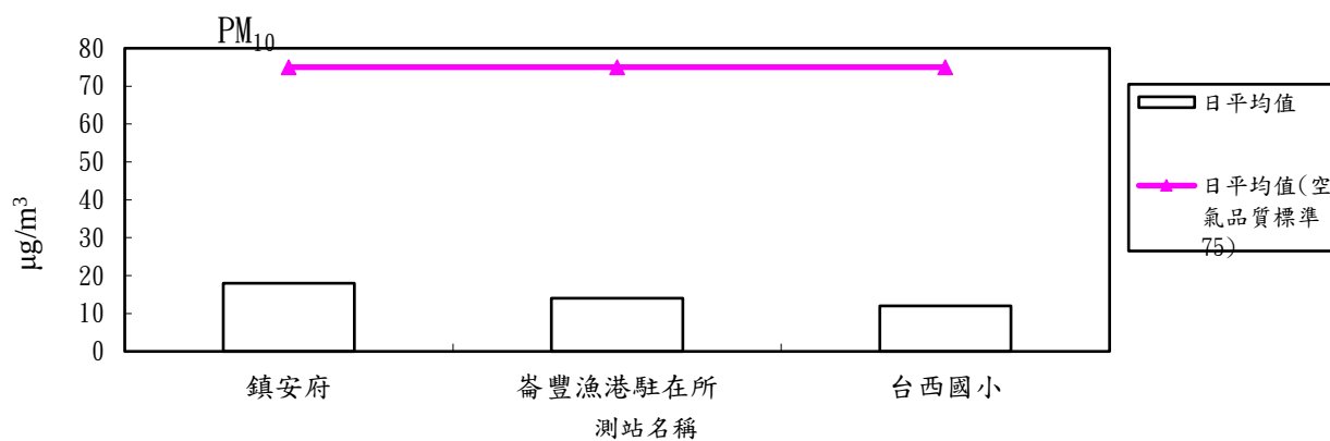
圖 2.1-9 115 年度第 2 季各測站 PM 10 日平均值比較分析圖
