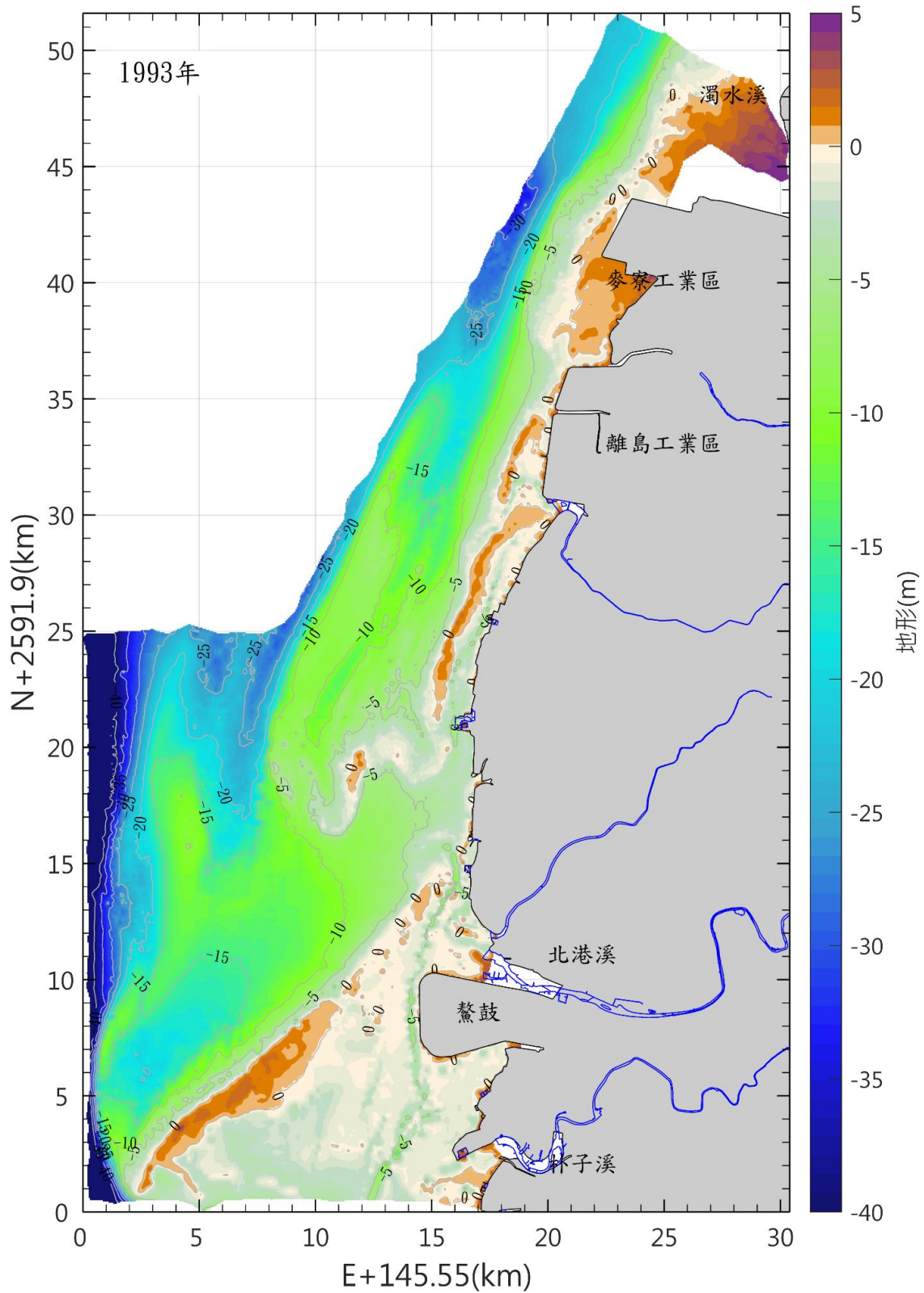
圖 3.1.12-11 本區海域 82 年海域地形圖
