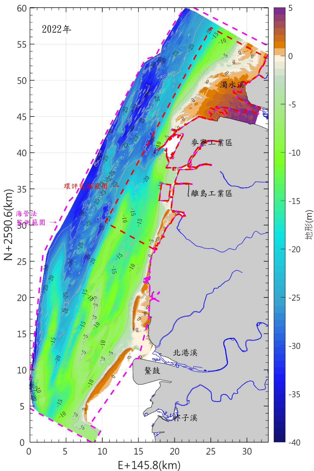
圖 3.1.12-39 本區海域 111 年海域地形圖(續)
