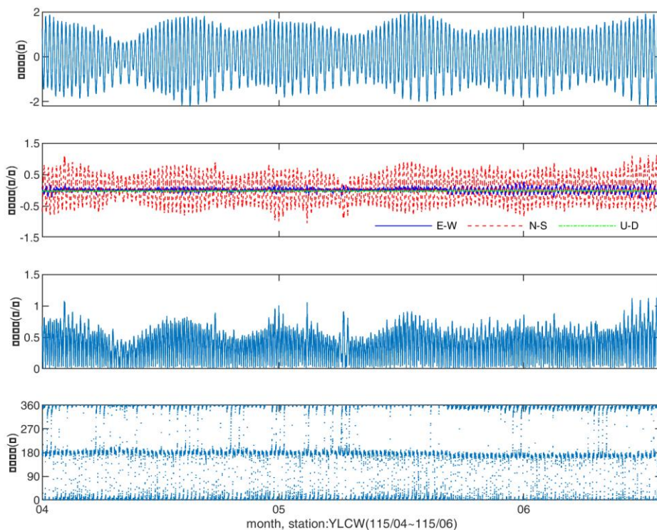
圖 2.13-10 YLCW 測站 115 年 4 月~115 年 6 月海流分量與流速流向時序列
