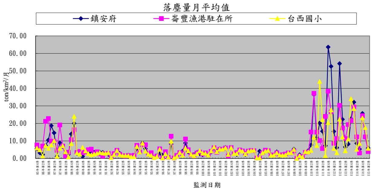
圖 3.1.1-9 本計畫歷次落塵量監測結果分析圖
