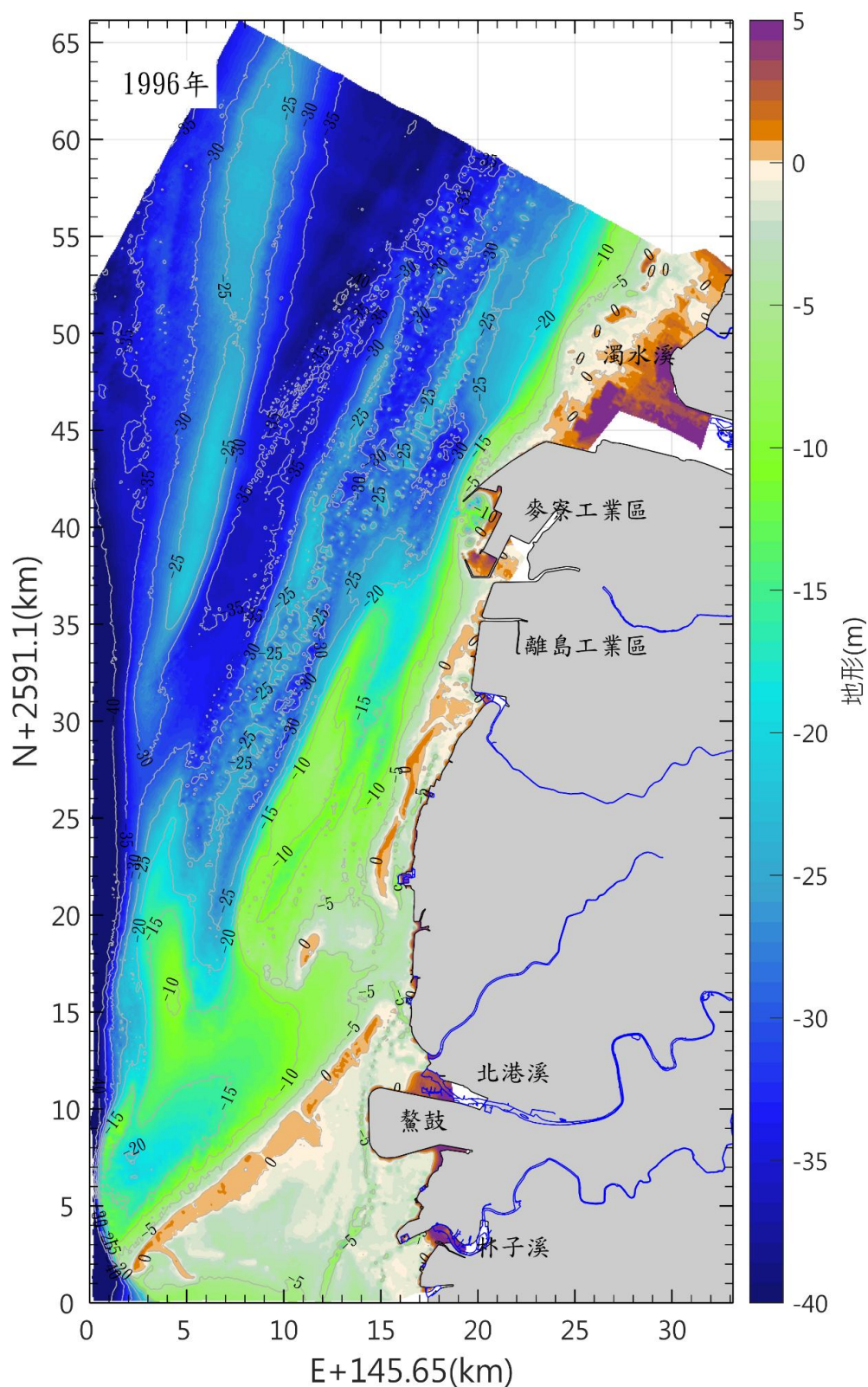
圖 3.1.12-13 本區海域 85 年海域地形圖(續)
