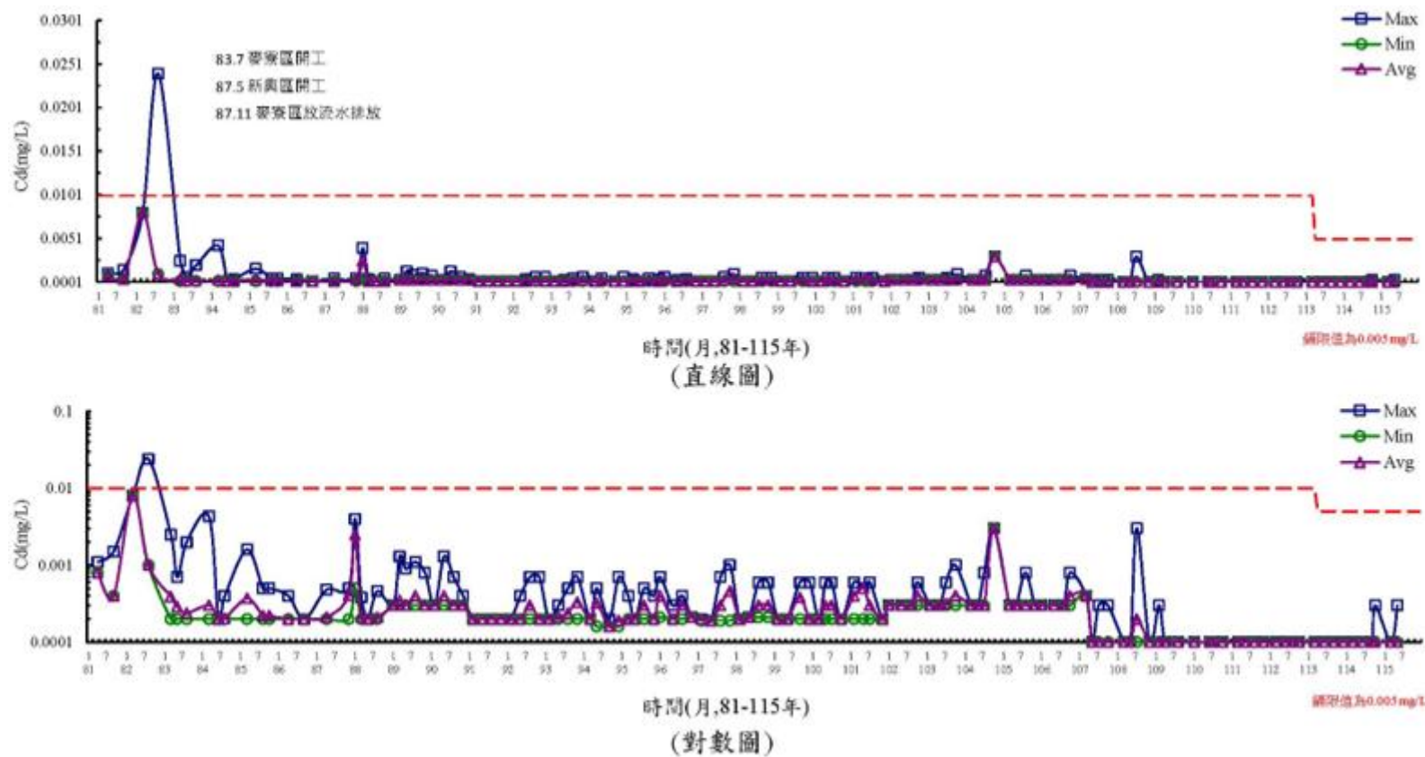
圖 3.1.9-15 離島產業園區海域歷年水質變化圖(Cd)
