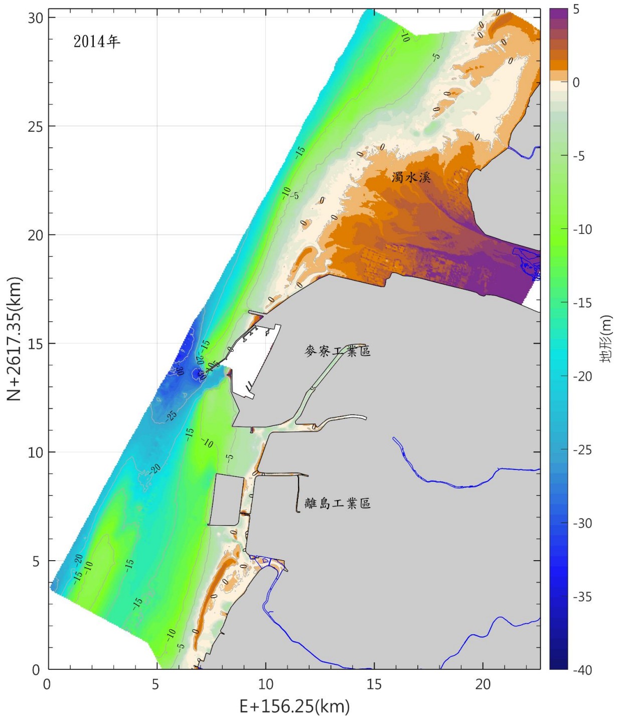
圖 3.1.12-31 本區海域 103 年海域地形圖(續)
