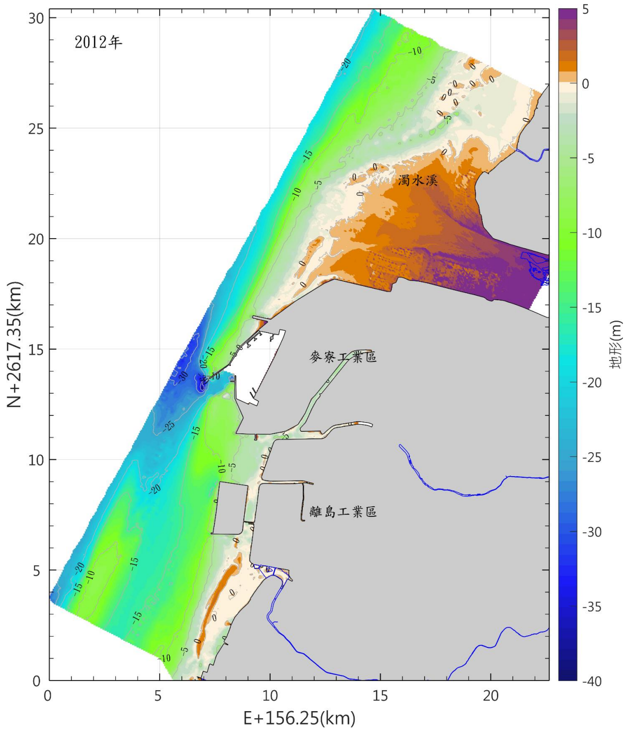
圖 3.1.12-29 本區海域 101 年海域地形圖(續)
