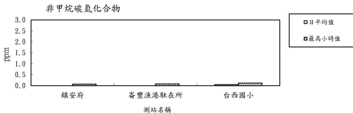
圖 2.1-7 115 年度第 2 季各測站非甲烷碳氫化合物(NMHC)日平均值及最高小時值比較分析圖
