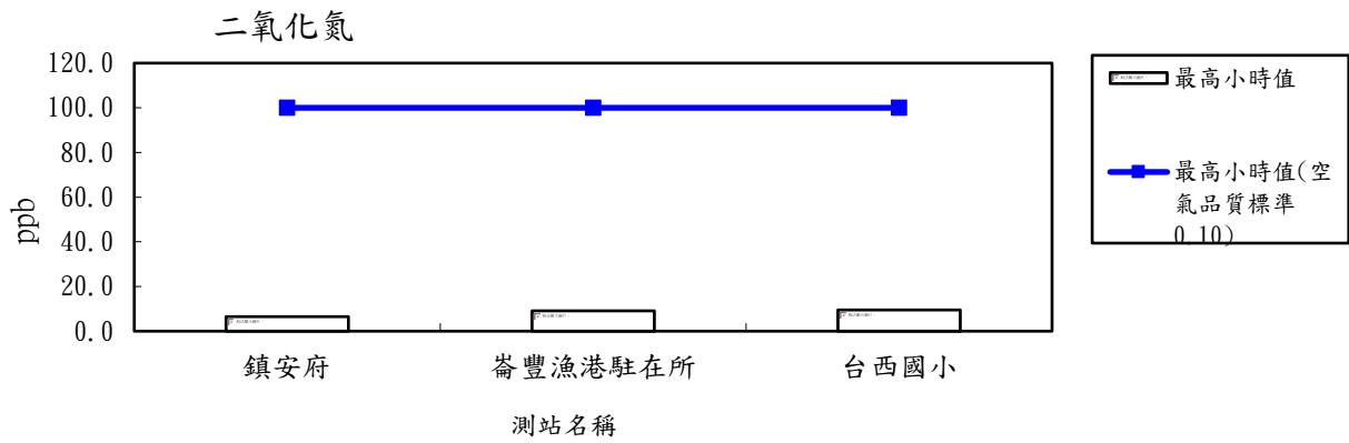
圖 2.1-4 115 年度第 2 季各測站二氧化氮( \text{NO}_2 )最高小時值比較分析圖
