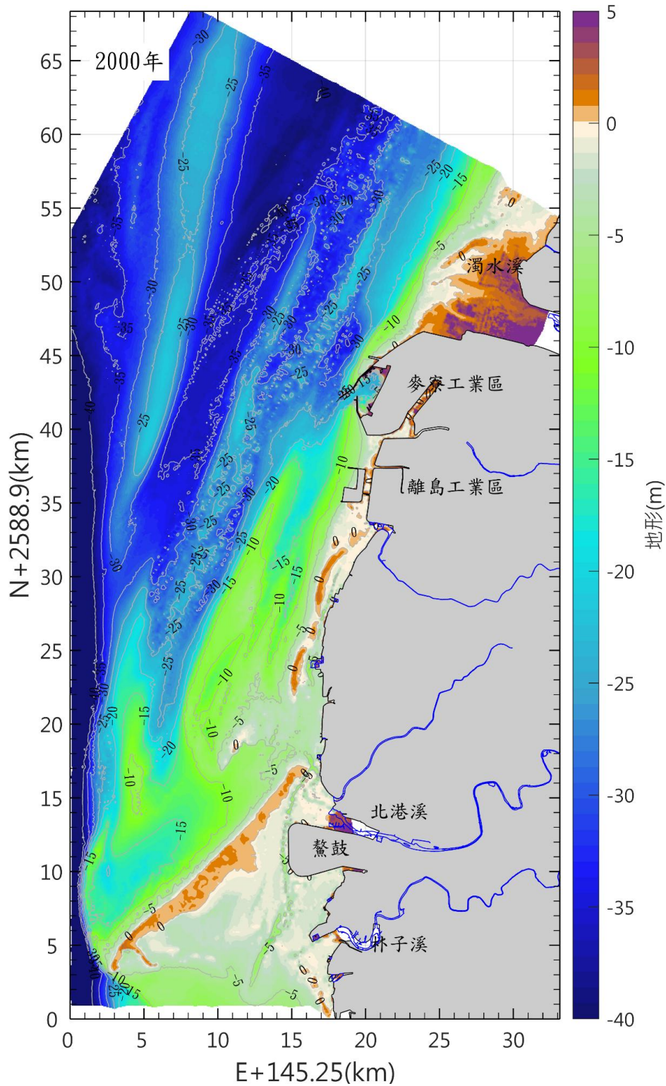
圖 3.1.12-17 本區海域 89 年海域地形圖(續)
