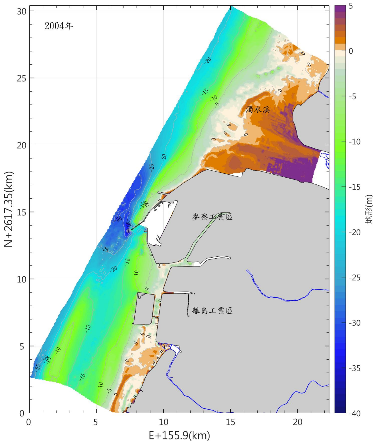
圖 3.1.12-21 本區海域 93 年海域地形圖(續)
