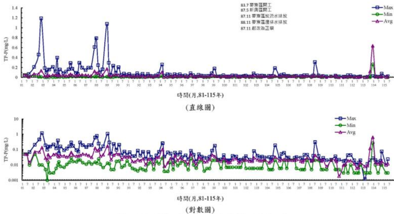
圖 3.1.9-10 離島產業園區海域歷年水質變化圖(TP-P)
