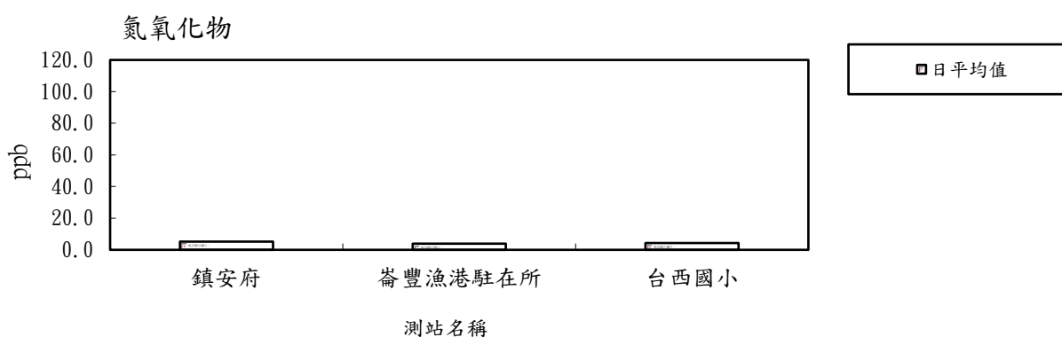
圖 2.1-3 115 年度第 2 季各測站氮氧化物(NO x )日平均值比較分析圖
