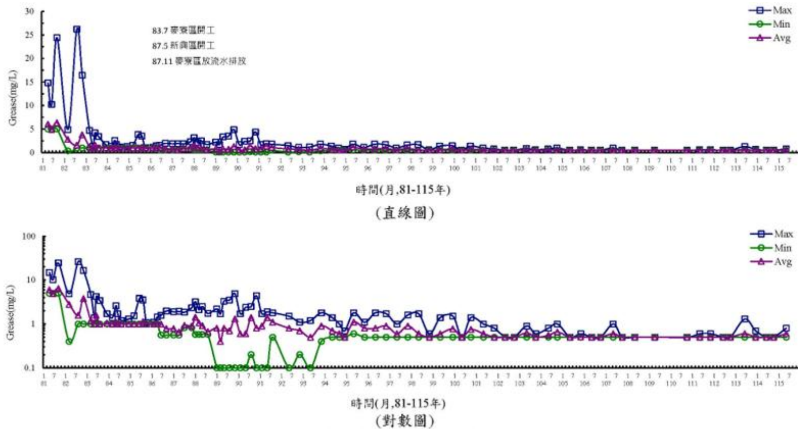
圖 3.1.9-12 離島產業園區海域歷年水質變化圖(Grease)
