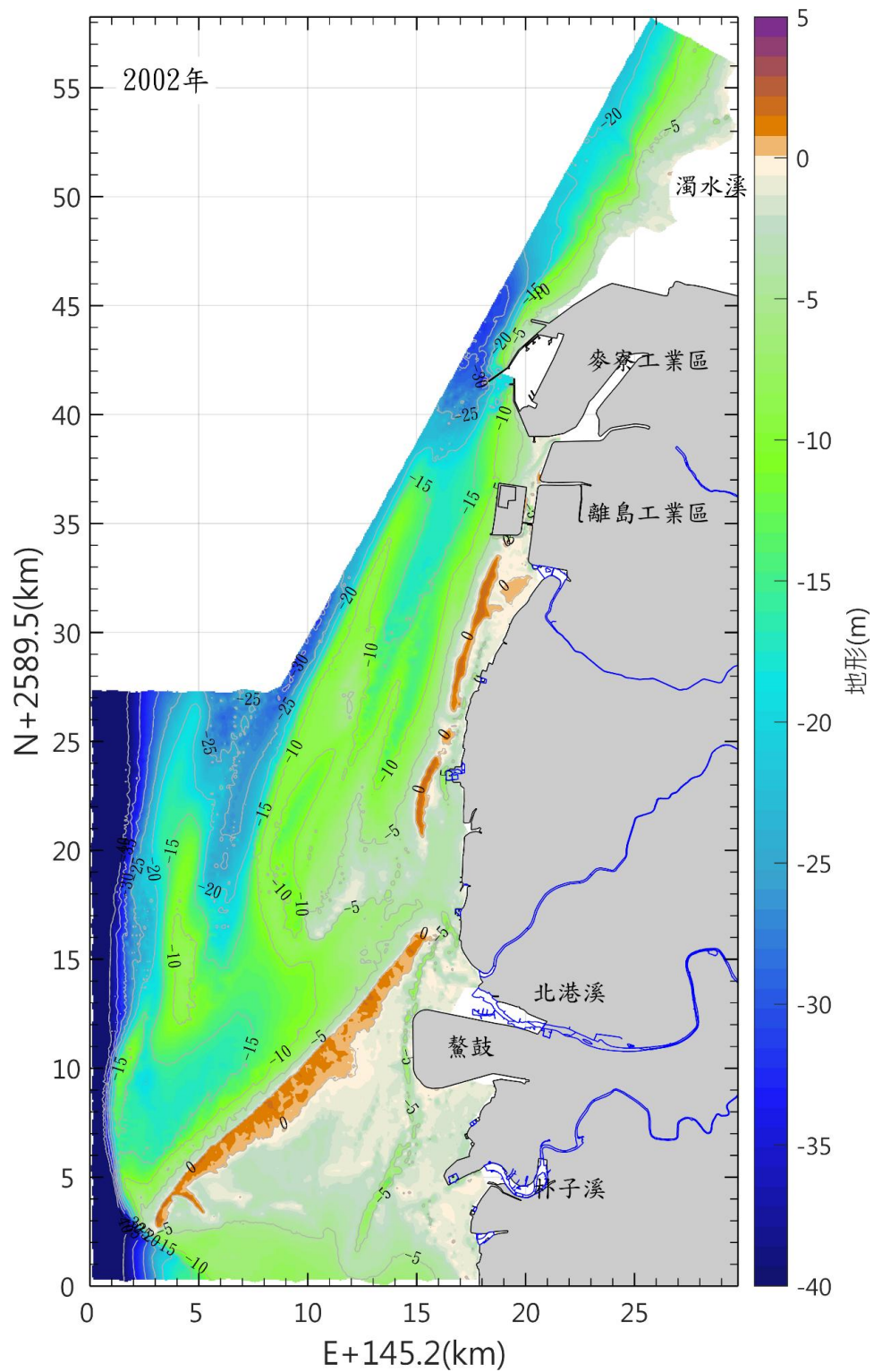
圖 3.1.12-19 本區海域 91 年海域地形圖(續)
