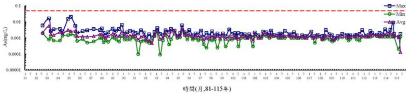
圖 3.1.9-21 離島產業園區海域歷年水質變化圖(As)
