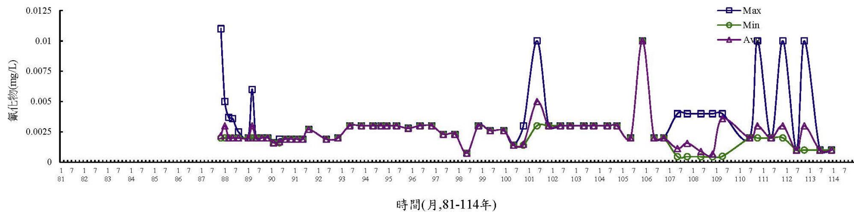
圖 3.1.9-23 離島產業園區海域歷年水質變化圖(氰化物)
