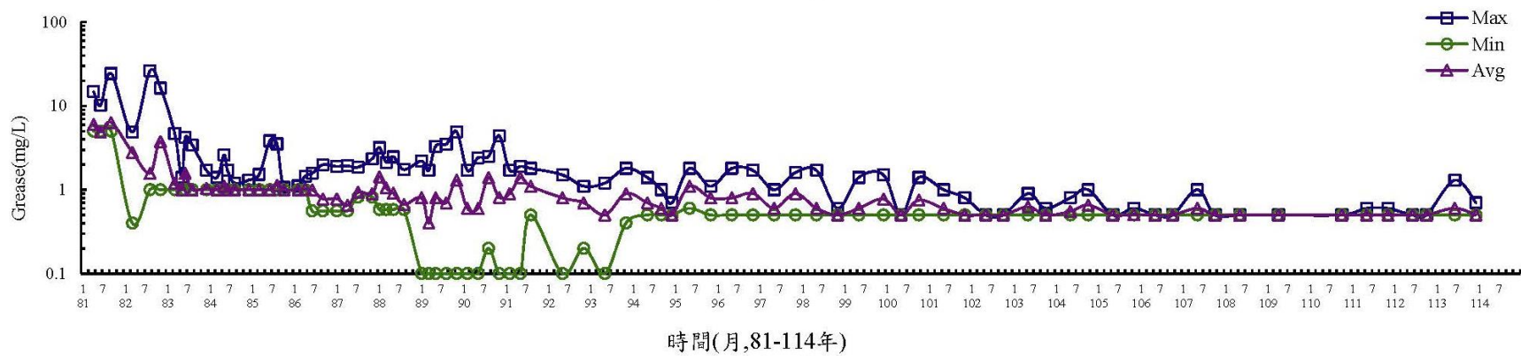
圖 3.1.9-12 離島產業園區海域歷年水質變化圖(Grease)
