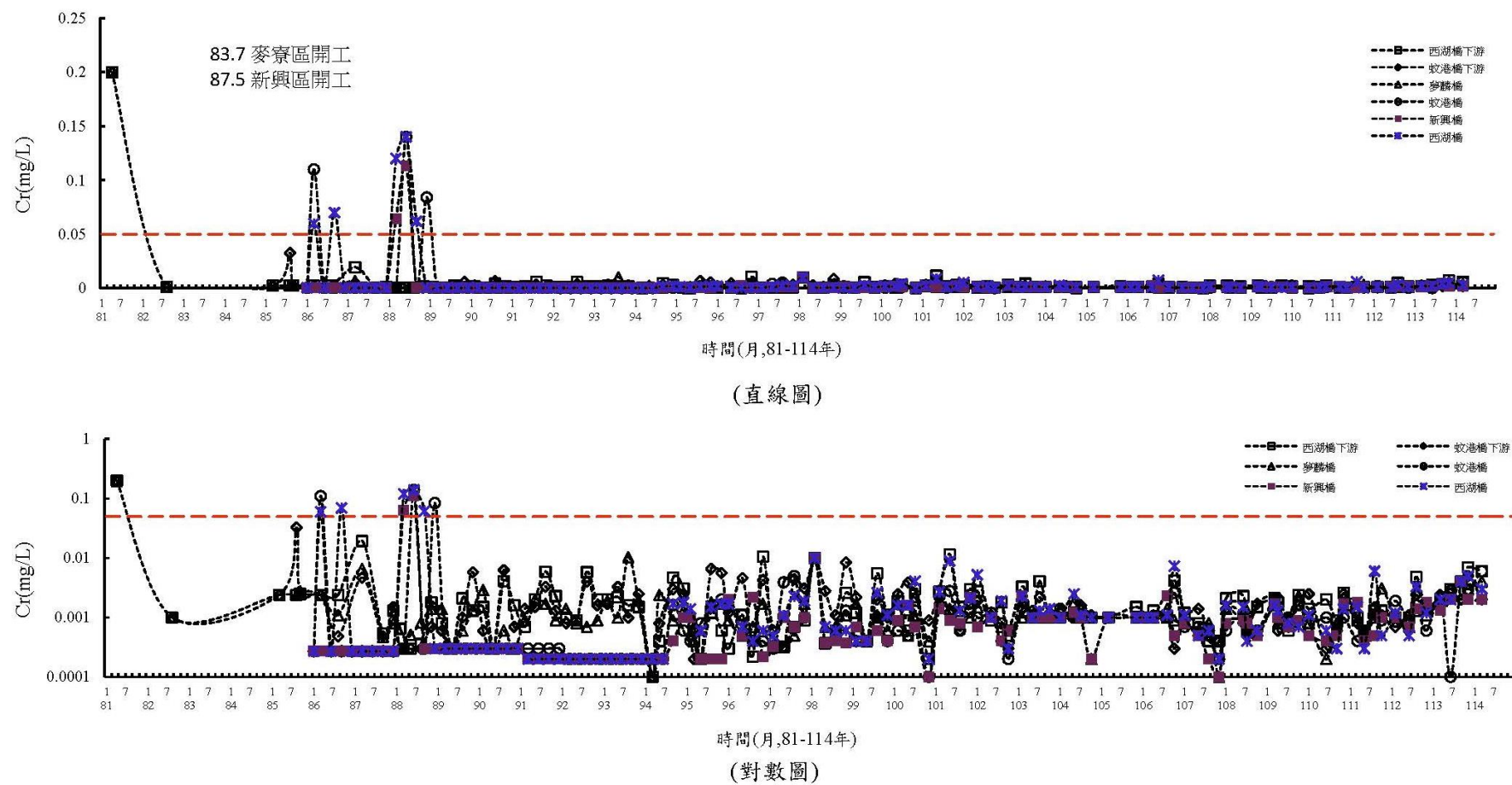
圖 3.1.8-1 離島產業園區陸域河口歷年水質變化圖(續 19)
