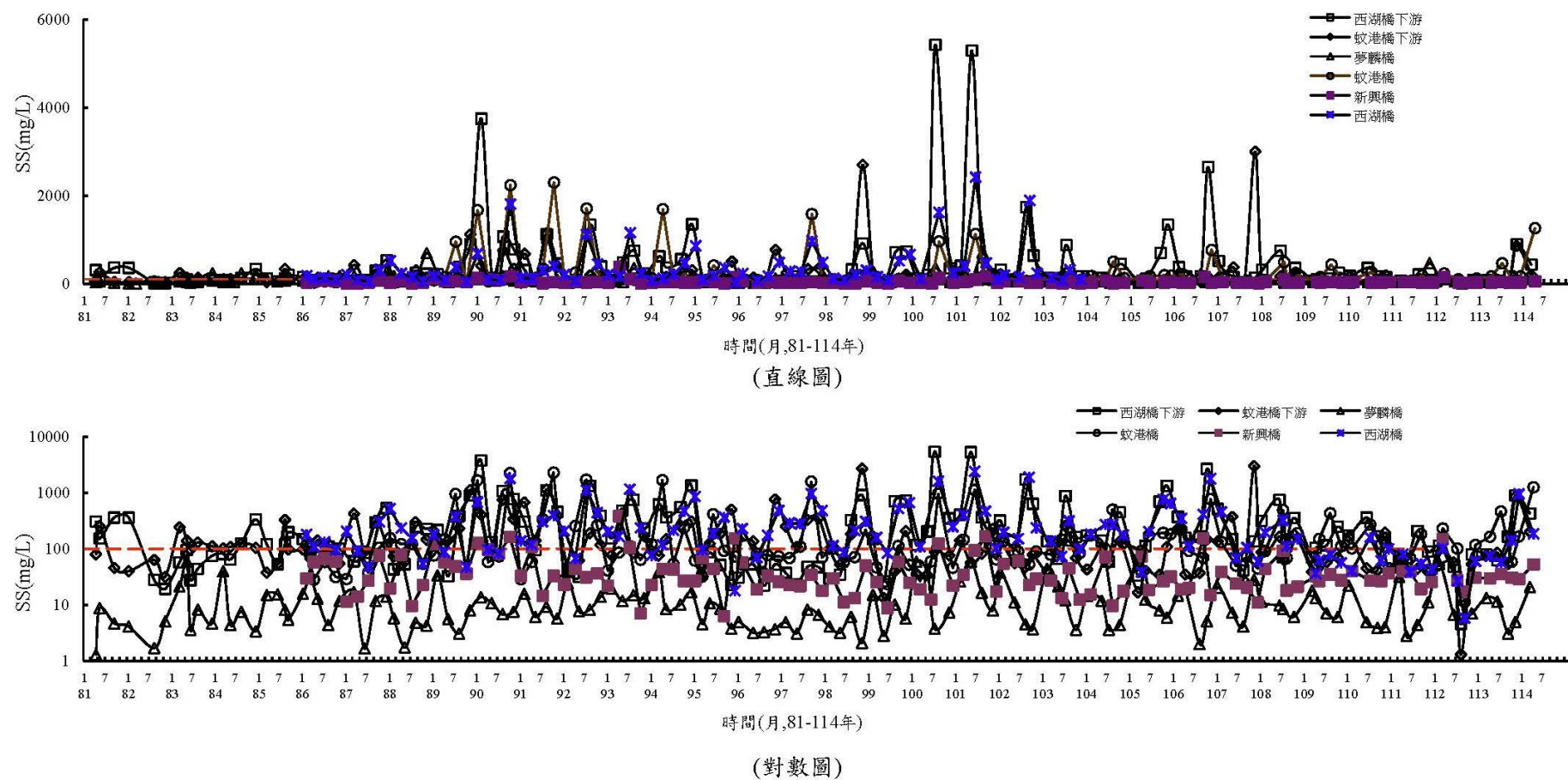
圖 3.1.8-1 離島產業園區陸域河口歷年水質變化圖(續 4)
