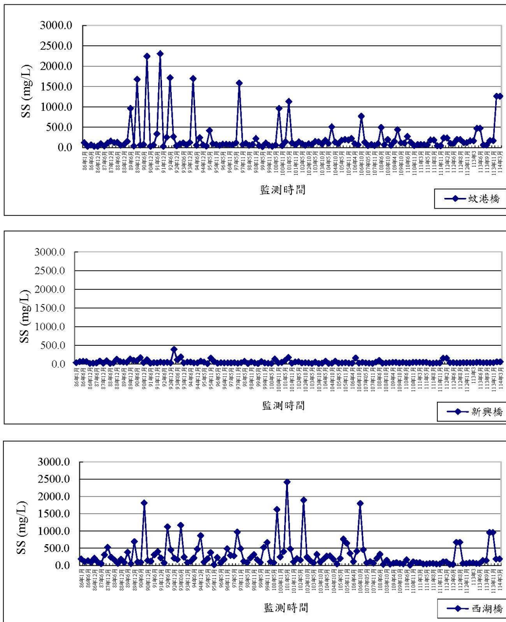
圖 3.1.7-1 陸域水質歷次懸浮固體比較分析圖
