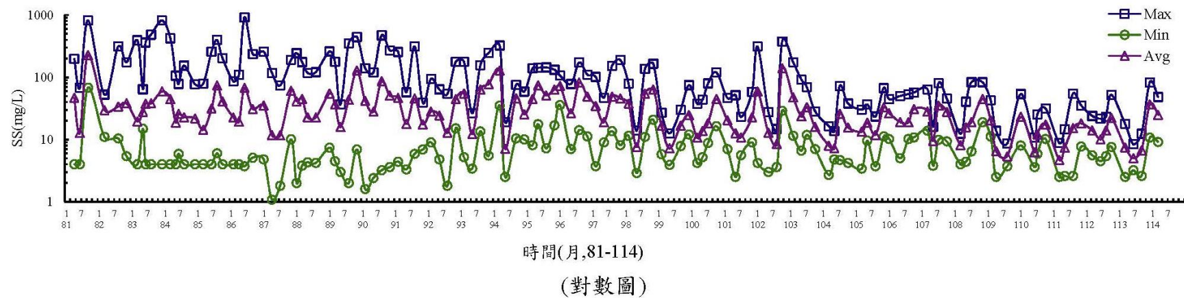
圖 3.1.9-5 離島產業園區海域歷年水質變化圖(SS)
