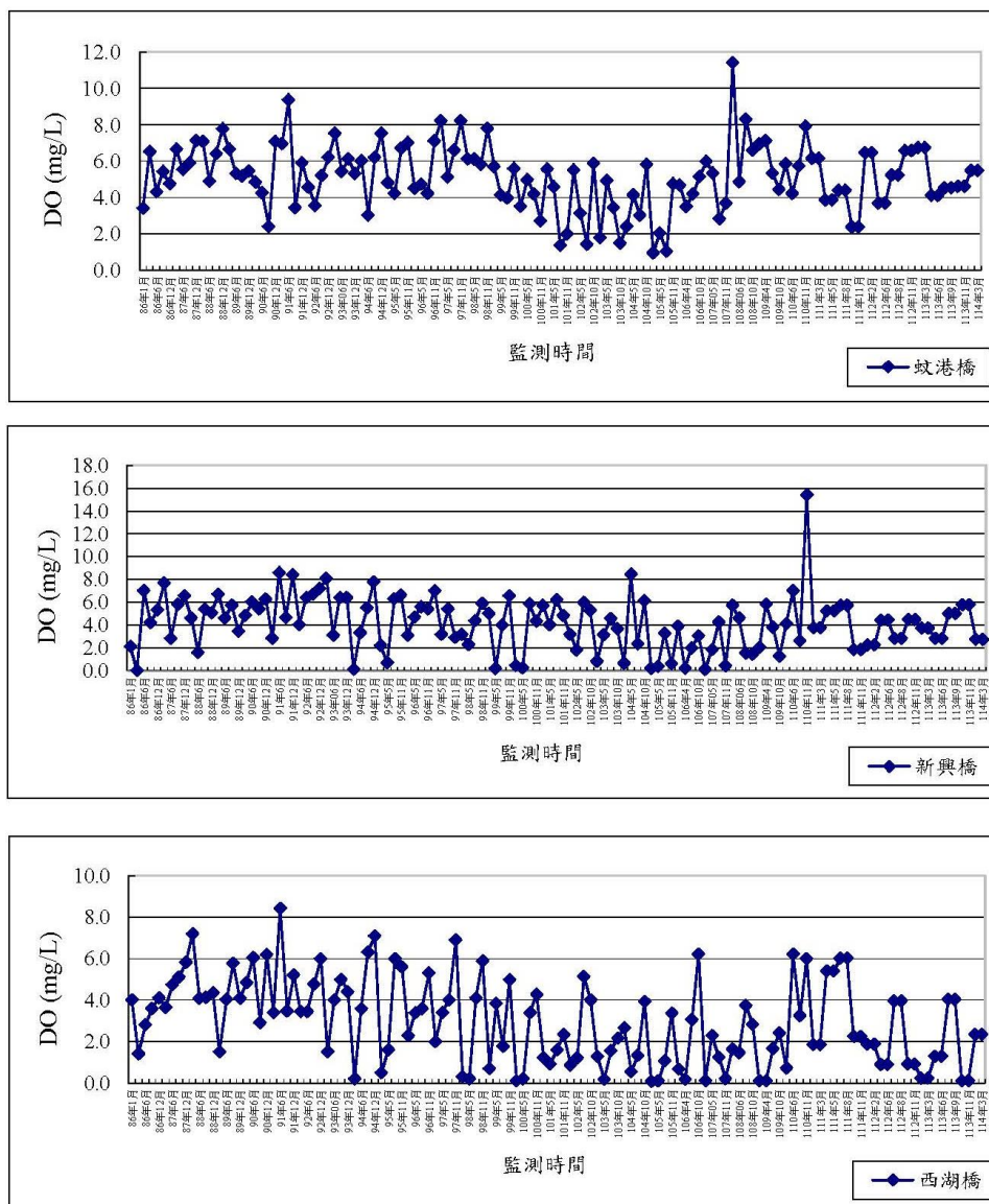
圖 3.1.7-2 陸域水質歷次溶氧比較分析圖
