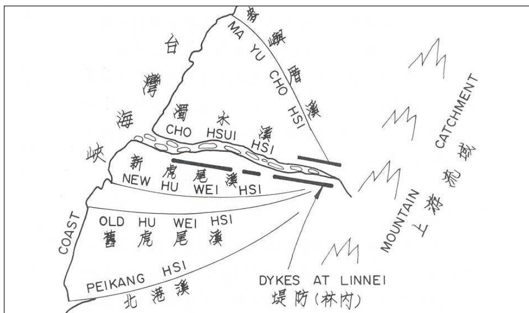
圖 3.1.12-1 濁水溪河系古河道位置變遷示意圖
