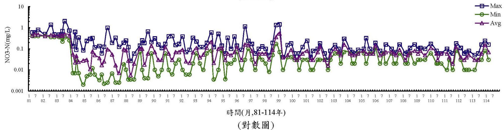
圖 3.1.9-9 離島產業園區海域歷年水質變化圖(NO 3 -N)
