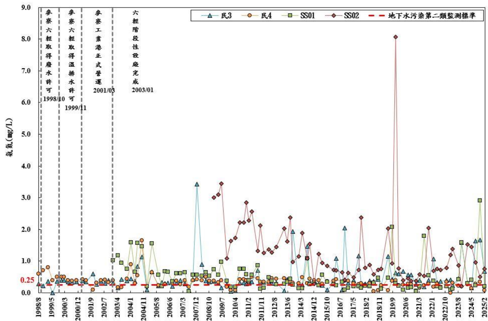
圖 3.1.6-5 氨氮歷年濃度測值變化
