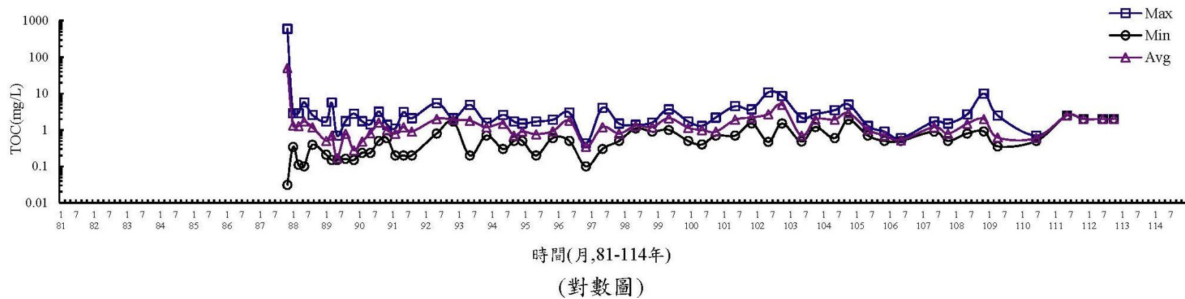
圖 3.1.9-24 離島產業園區海域歷年水質變化圖(TOC)
