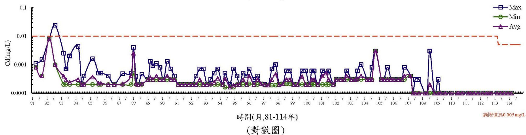
圖 3.1.9-15 離島產業園區海域歷年水質變化圖(Cd)
