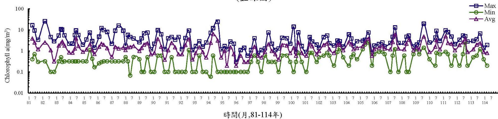
圖 3.1.9-13 離島產業園區海域歷年水質變化圖(Chlorophyll a)
