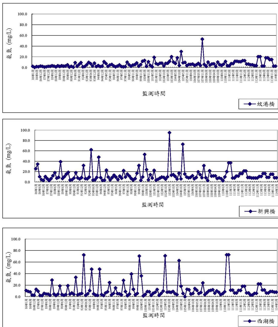
圖 3.1.7-4 陸域水質歷次氨氮比較分析圖
