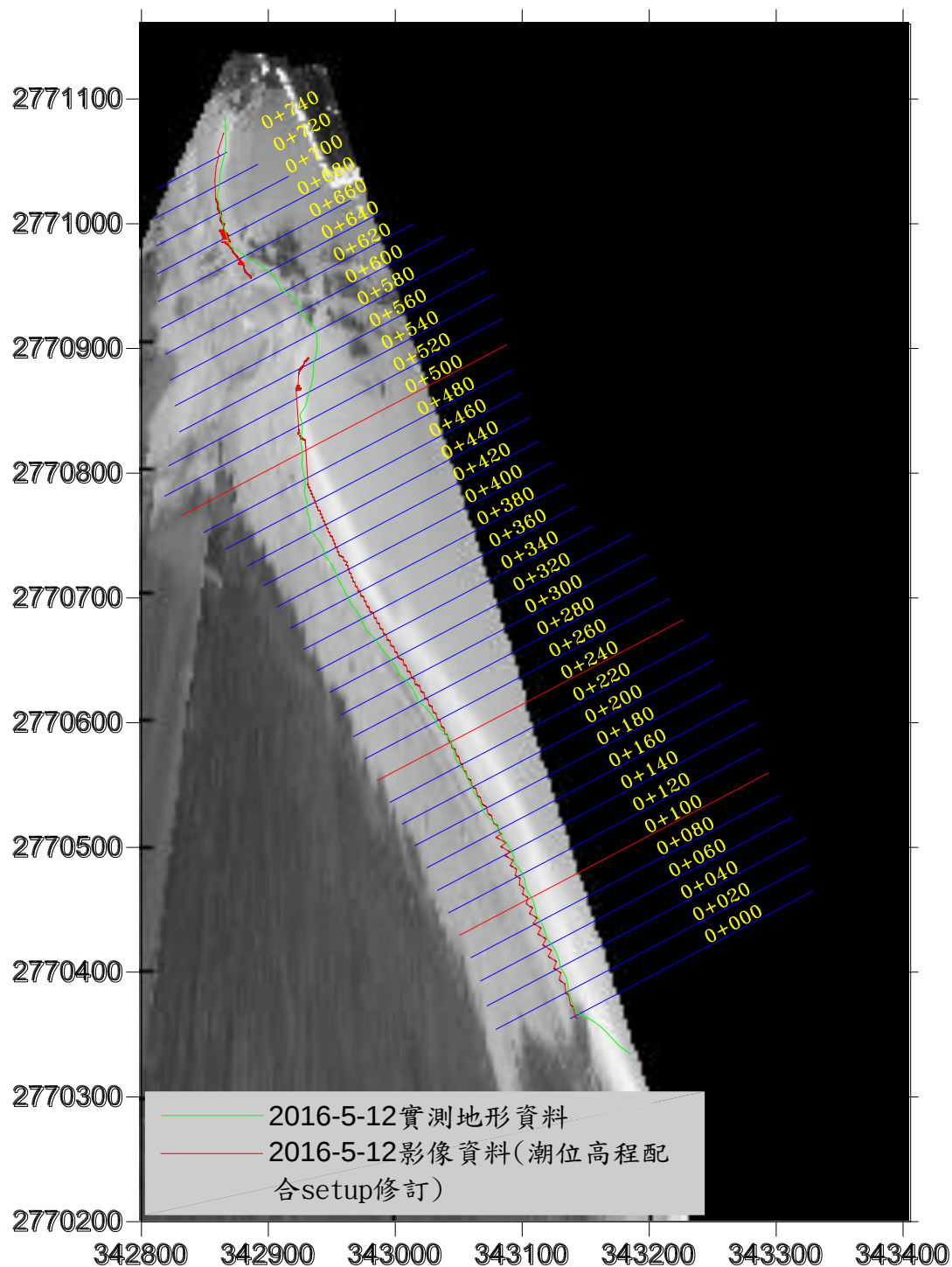
圖 3-22 水位線分析結果圖(2016/5/12)
