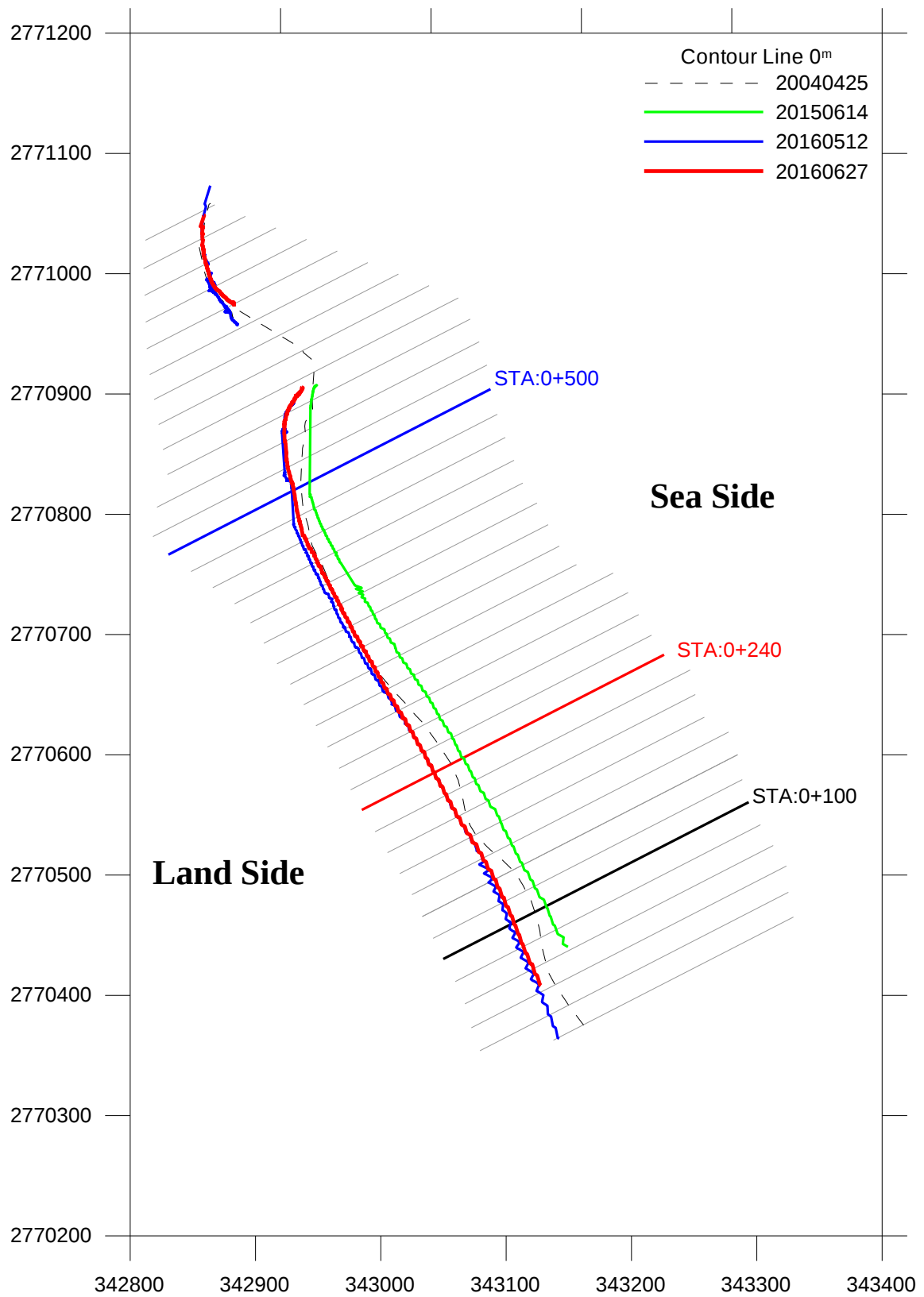
圖 4-15 鹽寮海岸線變遷分析比較圖
