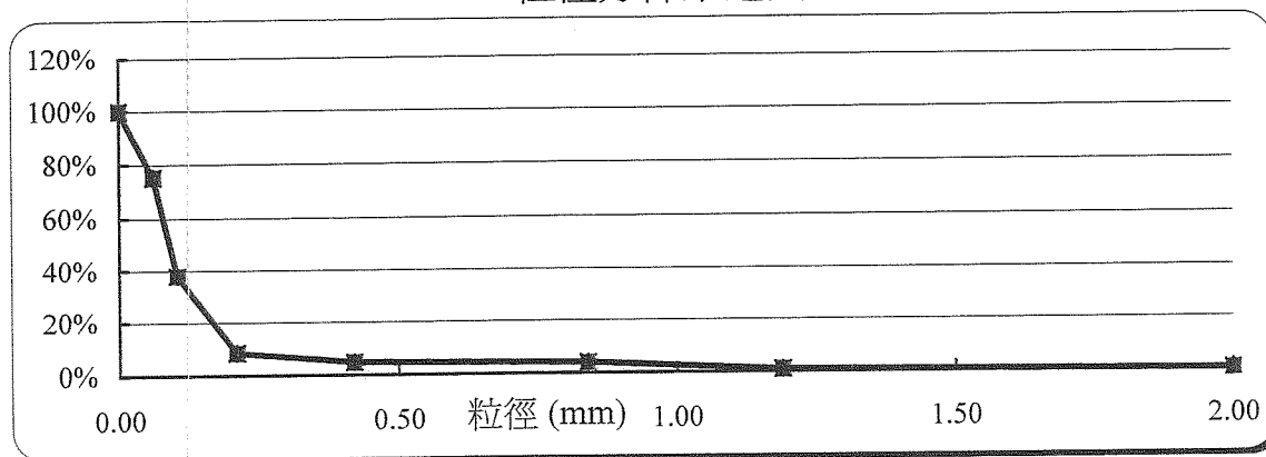
ML-1H 粒徑分佈累進圖
