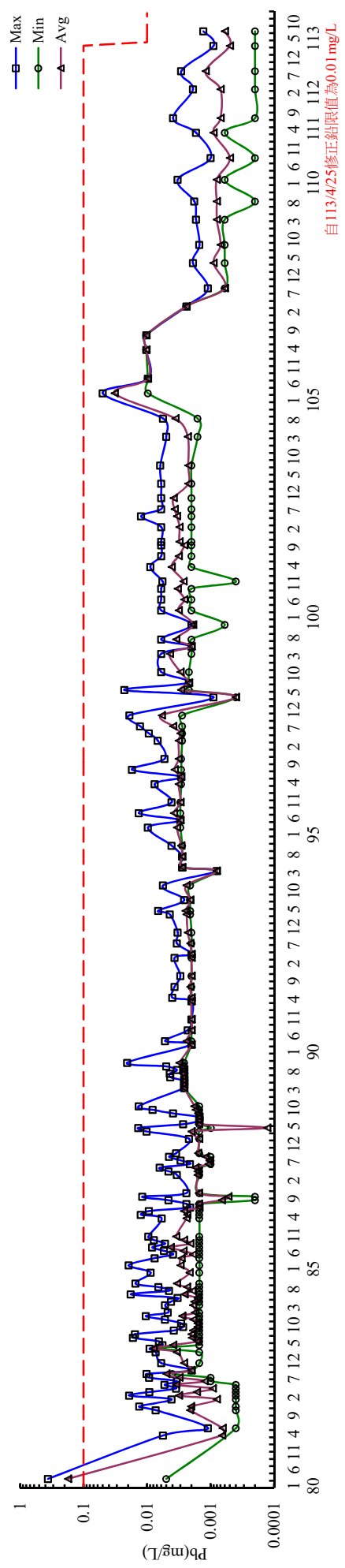
時間(民國年),對數圖 附圖III.9-14(b) 彰濱海域歷次鉛調查結果
