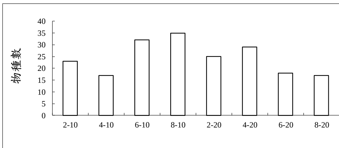
附錄 III.10-1 圖 1 113 年 8 月彰濱產業園區附近海域亞潮帶各測站底棲生物物種數之比較
