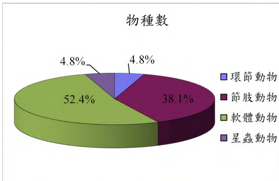
附錄 III.10-1 圖 5 民國 113 年 8 月潮間帶各大類生物之物種數百分比
