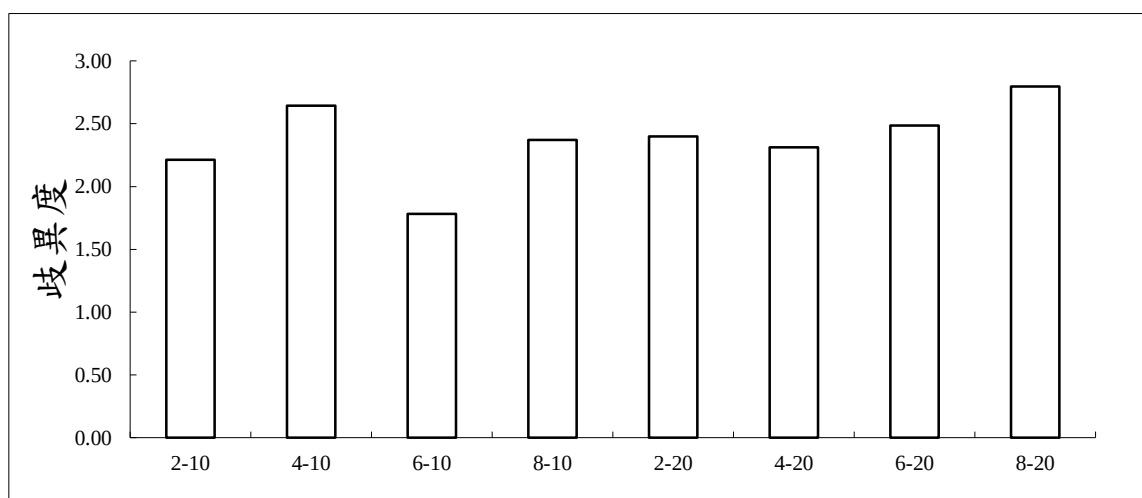
附錄 III.10-1 圖 3 113 年 8 月彰濱產業園區附近海域亞潮帶各測站底棲生物歧異度之比較
