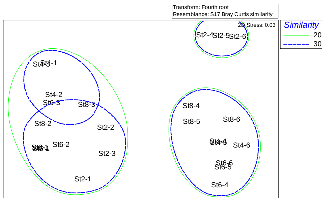
附錄 III.10-2 圖 4 民國 113 年 8 月於彰濱產業園區附近海域潮間帶各測站之群聚 MDS 圖
