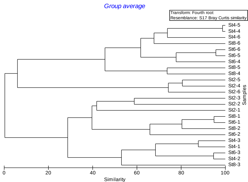
附錄 III.10-2 圖 3 民國 113 年 8 月於彰濱產業園區附近海域潮間帶各測站之群聚分析樹狀圖
