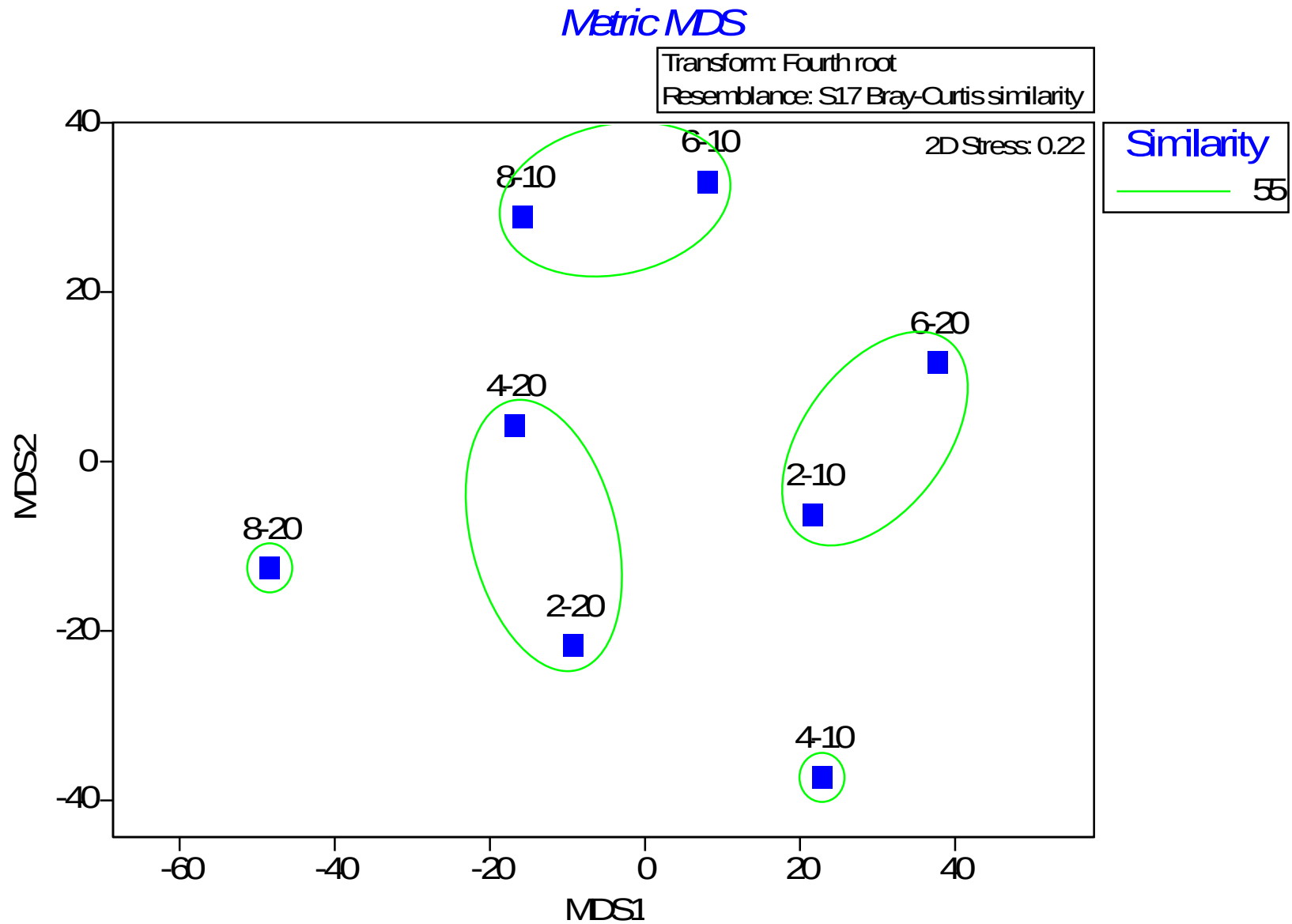
附錄 III.10-1 圖 5 113 年 8 月彰濱產業園區附近海域亞潮帶各測站間底棲生物 MDS 分析圖
