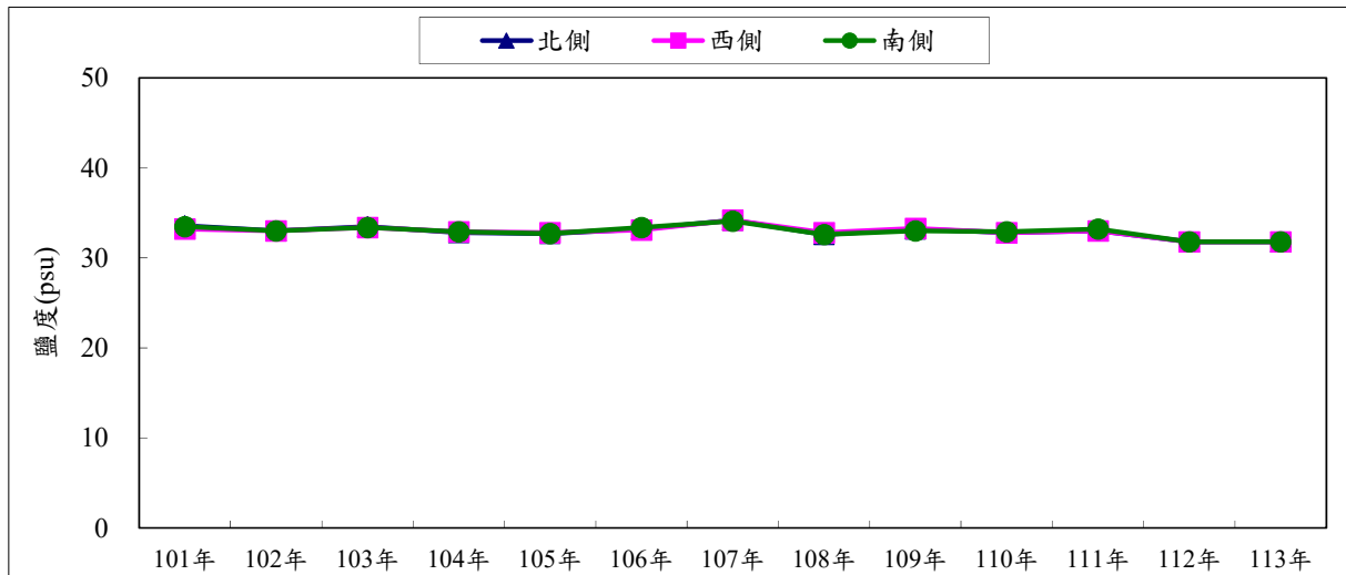
圖 3.1-12 歷年同期各測站鹽度監測成果彙整
