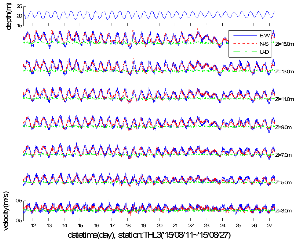
附錄III.11圖-2 THL3流速、流向、南北向、東西向速度分量逐時變化圖
