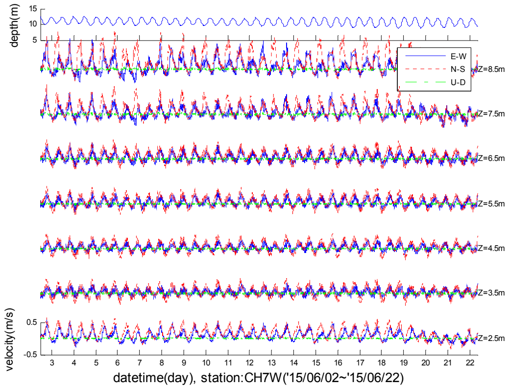
附錄III.11圖-1 CH7W流速、流向、南北向、東西向速度分量逐時變化圖
