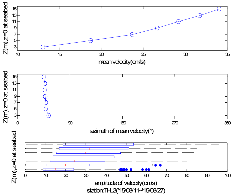
附錄III.11圖-8 THL3分層平均流速、平均流向剖面及流速振幅鬚盒圖
