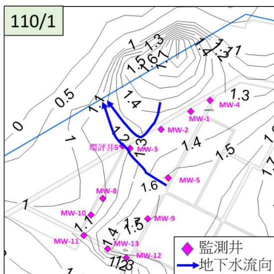
附圖五 環評井5局部流場(110年1月)
