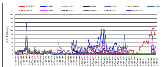
附圖一 環評井 5 與掩埋場周圍監測井之氨氮測值歷線圖
