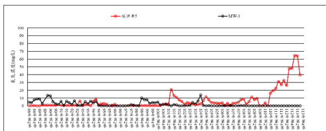
附圖二 環評井5與MW-3氨氮歷線圖
