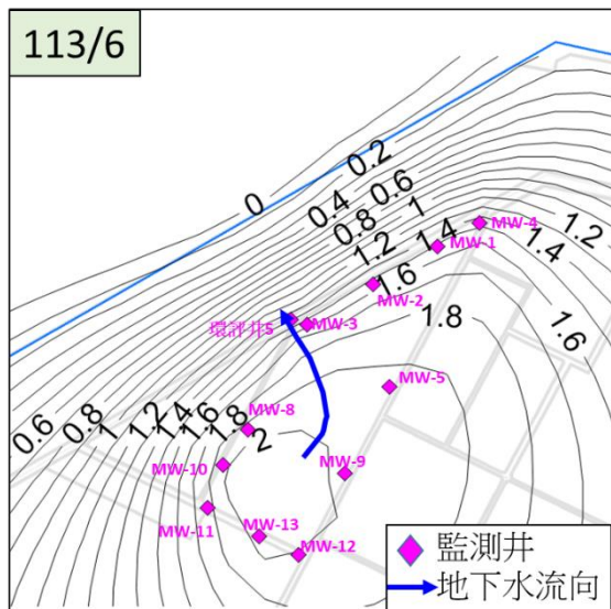
附圖六 環評井5局部流場(113年6月)
