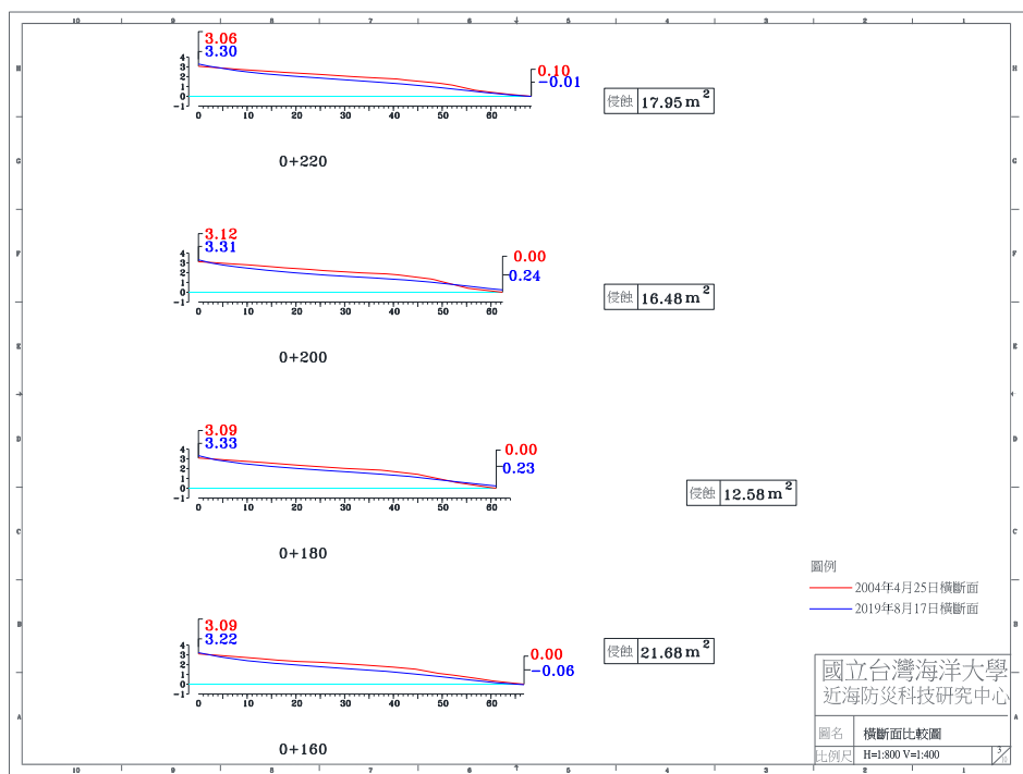
圖 4-4(h) 2019 年 8 月 17 日 A 監測區橫斷面比較圖
