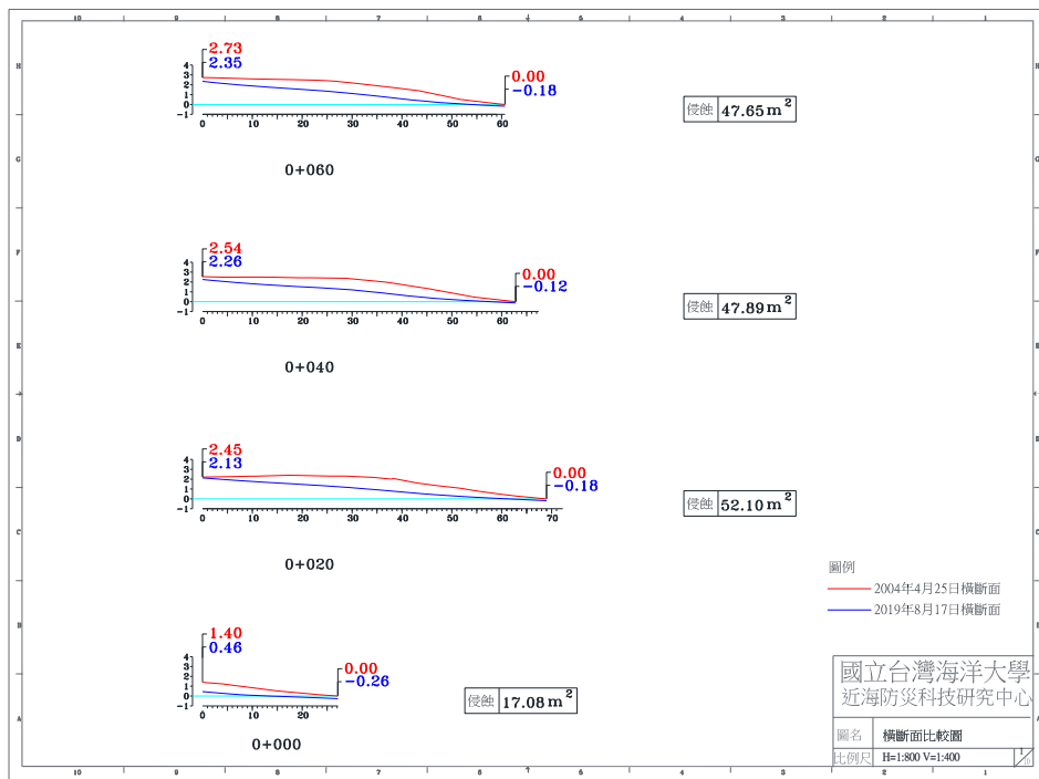
圖 4-4(j) 2019 年 8 月 17 日 A 監測區橫斷面比較圖
