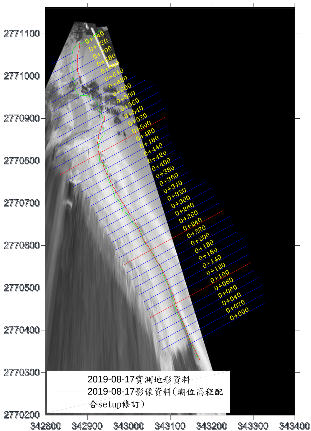
圖 3-22 水位線分析結果圖(2019/8/17)
