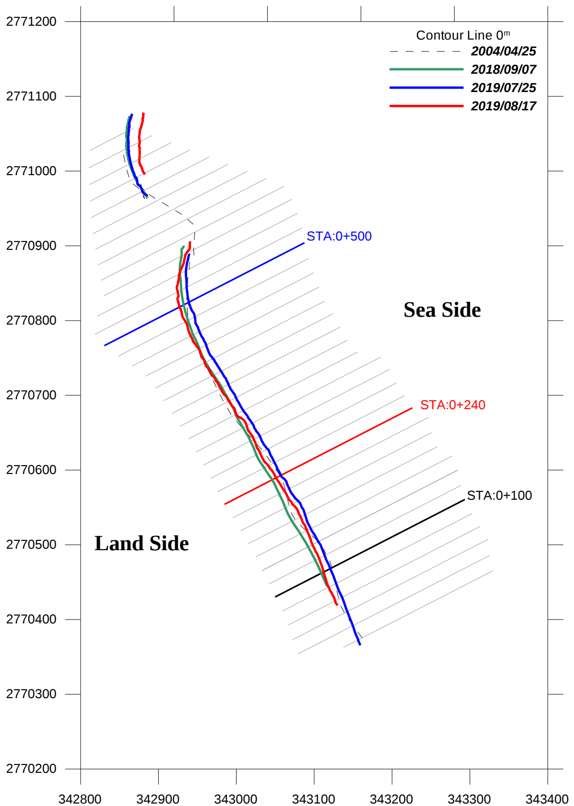
圖 4-20 鹽寮海岸線變遷分析比較圖
