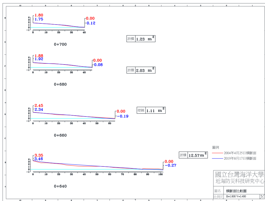
圖 4-4(b) 2019 年 8 月 17 日 A 監測區橫斷面比較圖
