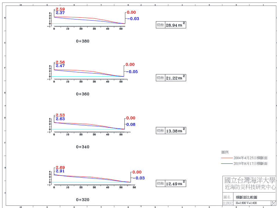
圖 4-4(f) 2019 年 8 月 17 日 A 監測區橫斷面比較圖
