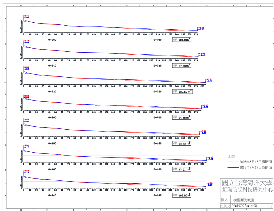
圖 4-5(e) 2019 年 8 月 17 日 B 監測區橫斷面比較圖
