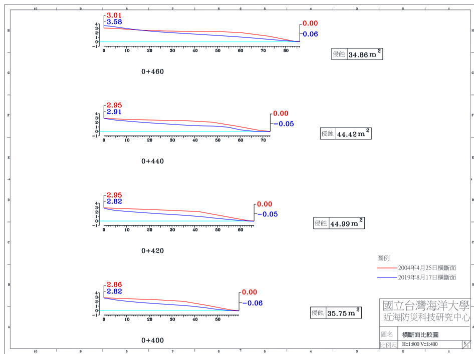
圖 4-4(e) 2019 年 8 月 17 日 A 監測區橫斷面比較圖
