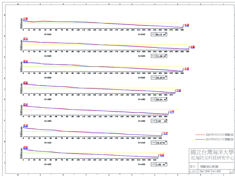
圖 4-5(c) 2019 年 8 月 17 日 B 監測區橫斷面比較圖
