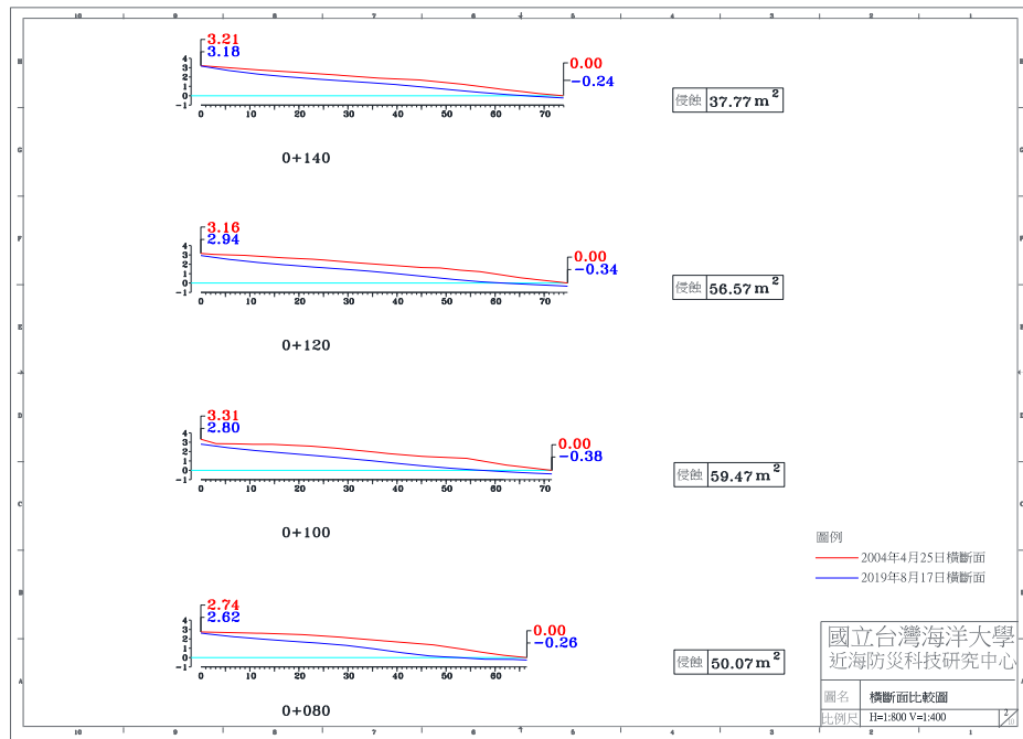
圖 4-4(i) 2019 年 8 月 17 日 A 監測區橫斷面比較圖
