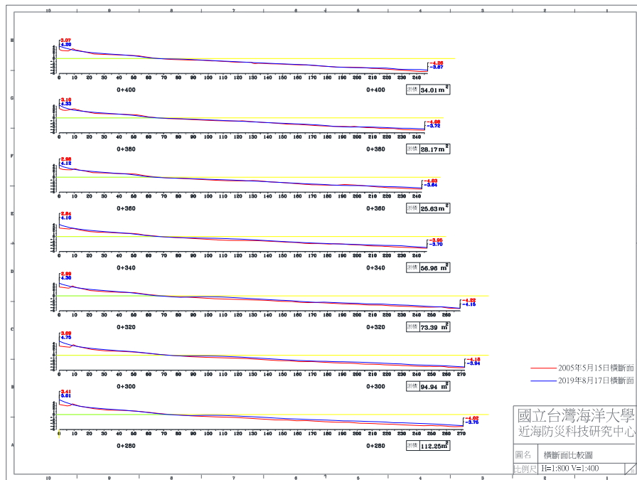
圖 4-5(d) 2019 年 8 月 17 日 B 監測區橫斷面比較圖
