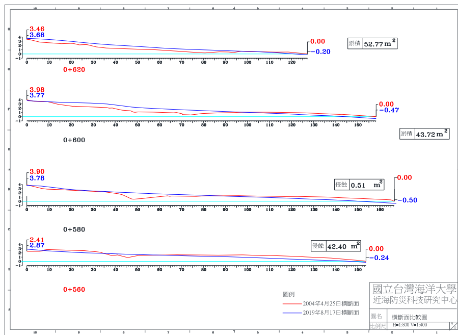
圖 4-4(c) 2019 年 8 月 17 日 A 監測區橫斷面比較圖
