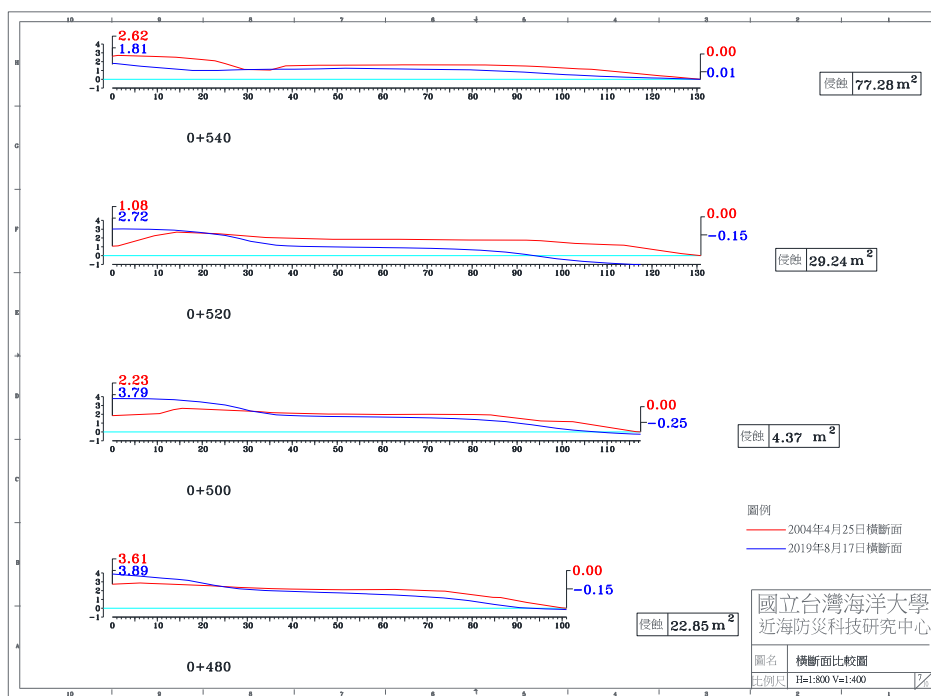
圖 4-4(d) 2019 年 8 月 17 日 A 監測區橫斷面比較圖
