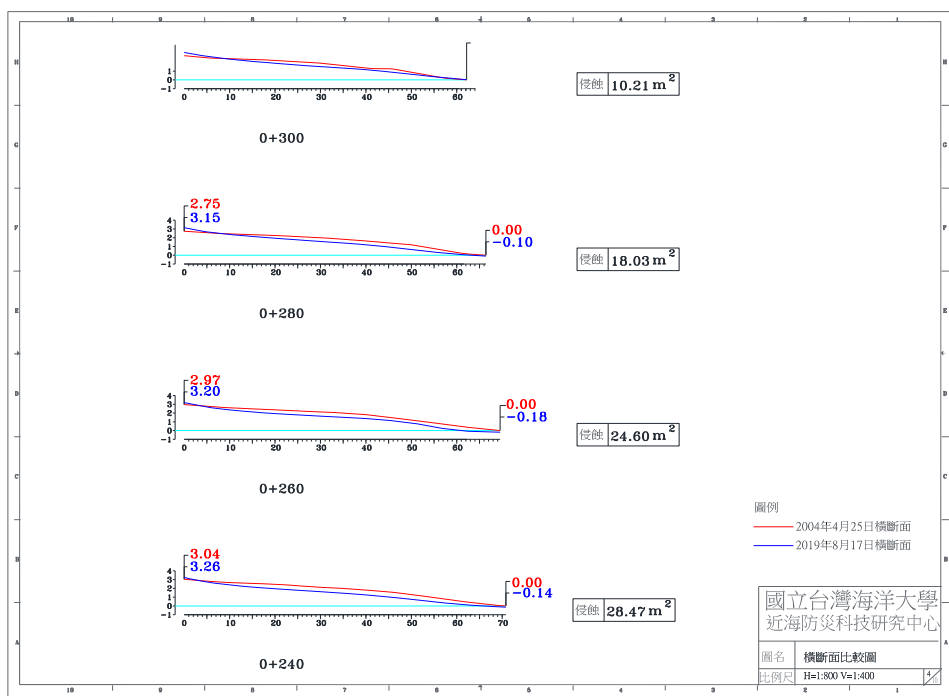
圖 4-4(g) 2019 年 8 月 17 日 A 監測區橫斷面比較圖
