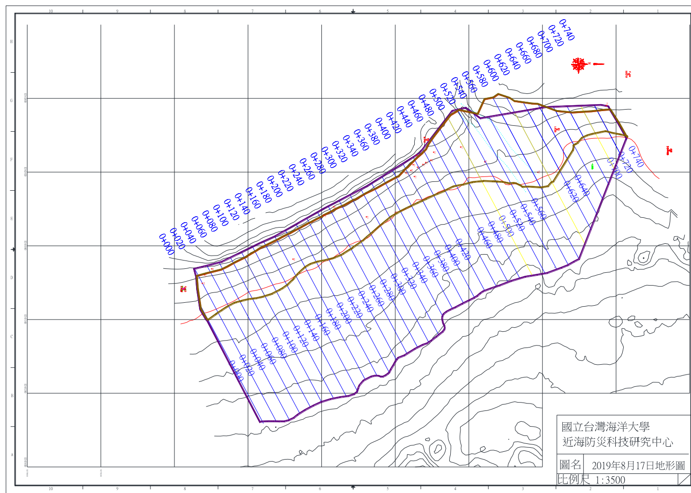
圖 4-1 2019 年 8 月 17 日監測地形圖
