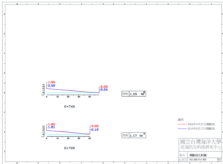
圖 4-4(a) 2019 年 8 月 17 日 A 監測區橫斷面比較圖
