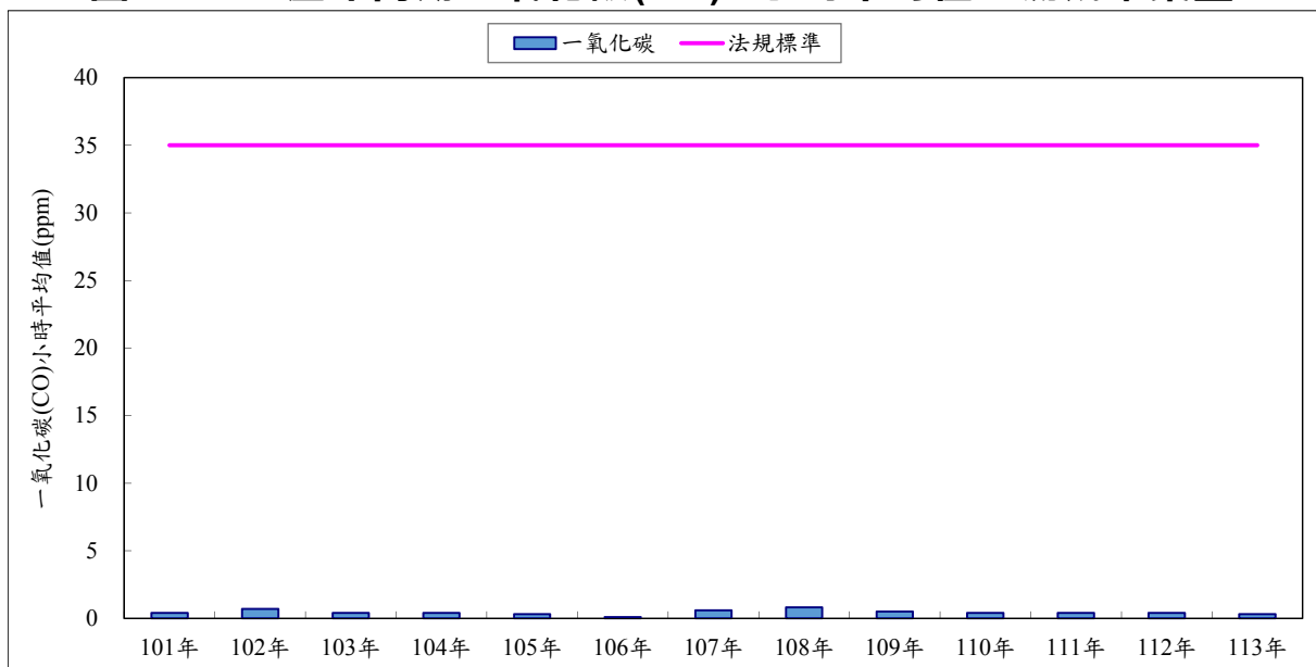
圖 3.1-8 歷年同期一氧化碳(CO)小時平均值監測成果彙整
