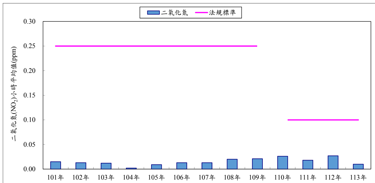
圖 3.1-4 歷年同期二氧化氮(NO 2 )小時平均值監測成果彙整
