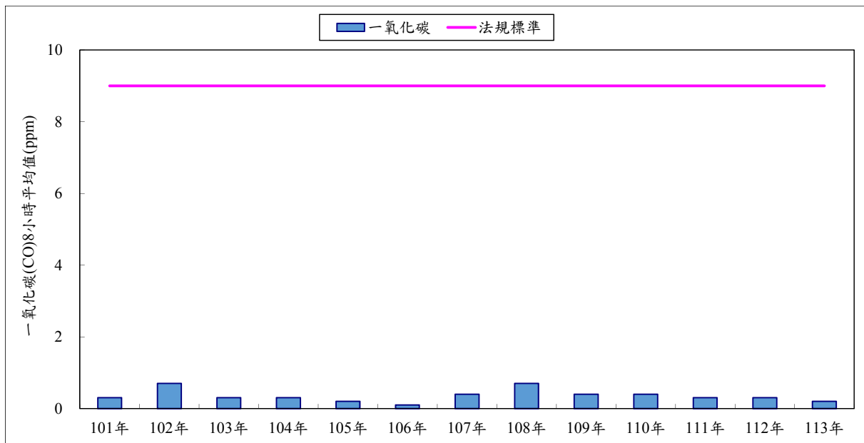
圖 3.1-7 歷年同期一氧化碳(CO)8 小時平均值監測成果彙整
