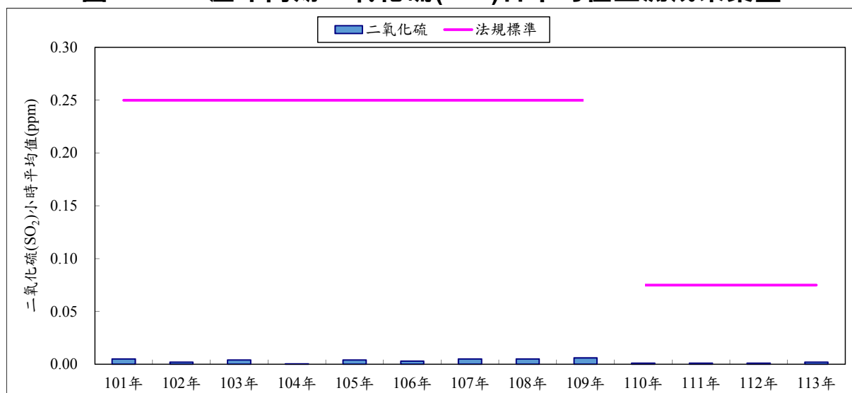
圖 3.1-6 歷年同期二氧化硫(SO 2 )小時平均值監測成果彙整
