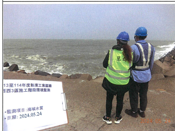
海域水質：113.05.24
