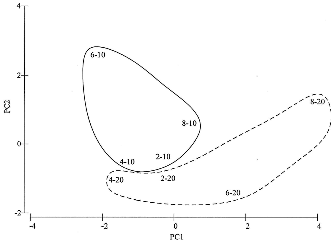
圖 2.10.2-3 民國 109 年 3 月彰濱工業區附近海域各測站浮游動物群聚分析圖(圖中第一個數字代表測站，第二個數字代表深度)
