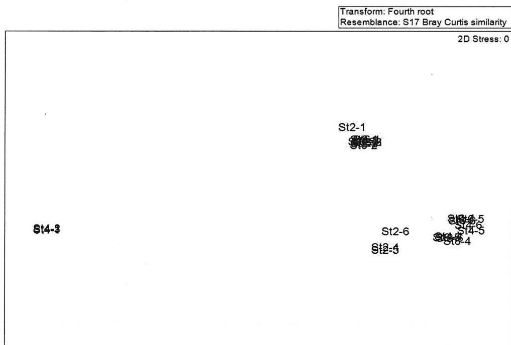
附錄III.10-2圖4 民國109年3月於彰濱工業區附近海域潮間帶各測站之群聚MDS圖。
