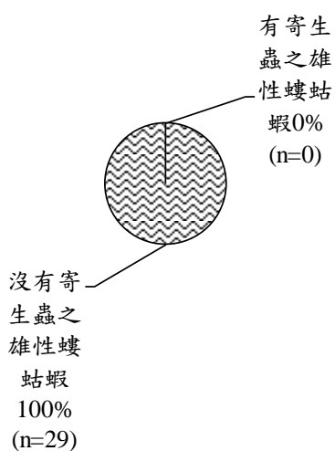
圖III.6-26 本季雄性螻蛄蝦被等足目寄生的百分率 (n=29)。
