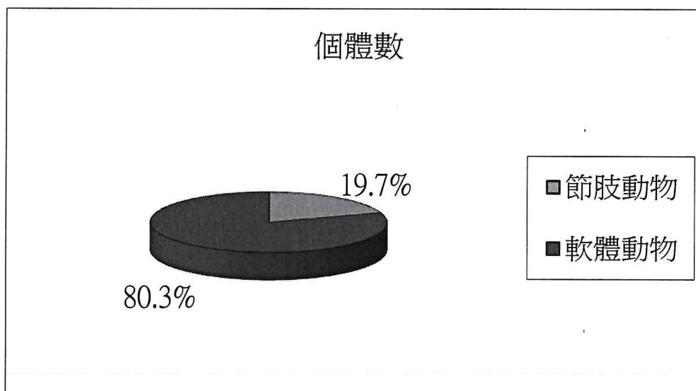
附錄III.10-1圖6 民國109年3月潮間帶各大類生物之個體數百分比
