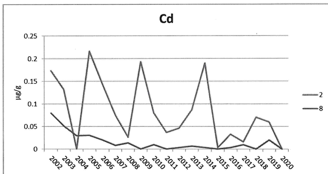
附錄 III.10-2 圖 15. 2002~2020 年 3 月測站 2 及 8 短指和尚蟹體內鎘含量之測站比較圖
