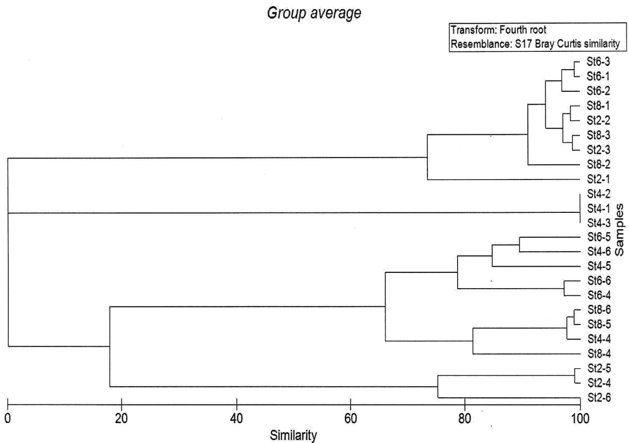
附錄III.10-2圖3 民國109年3月於彰濱工業區附近海域潮間帶各測站之群聚分析樹狀圖。
