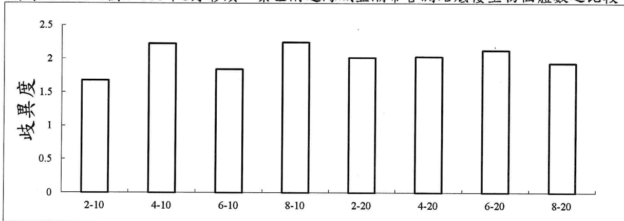
附錄III.10-1圖3 109年3月彰濱工業區附近海域亞潮帶各測站底棲生物歧異度之比較
