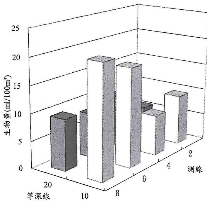
圖 2.10.2-1 民國 109 年 3 月彰化濱海工業區附近海域浮游動物之豐度及生物量分布圖
