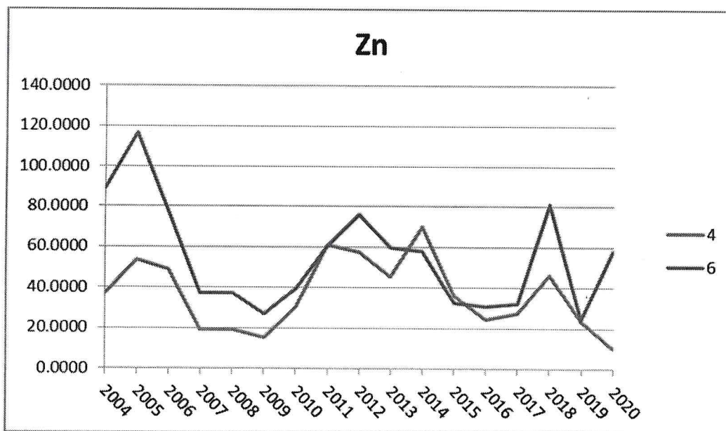
附錄 III.10-2 圖 20. 2004~2020 年 3 月測站 4 及 6 漁舟蜆螺體內鋅含量之測站比較圖
