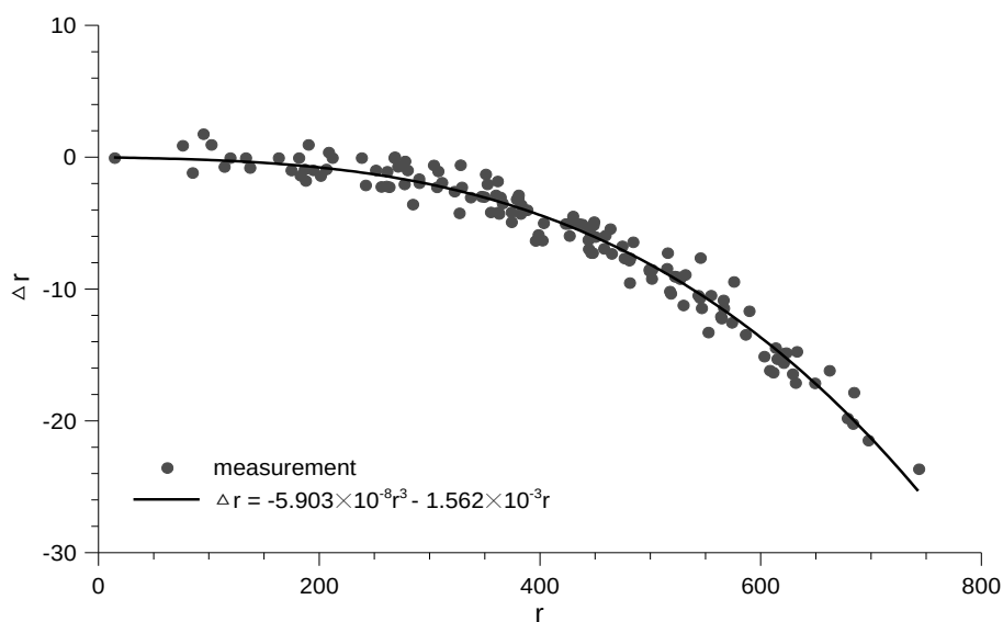
圖 3-18 攝影鏡頭編號 CAM1 之徑向扭曲迴歸結果圖
