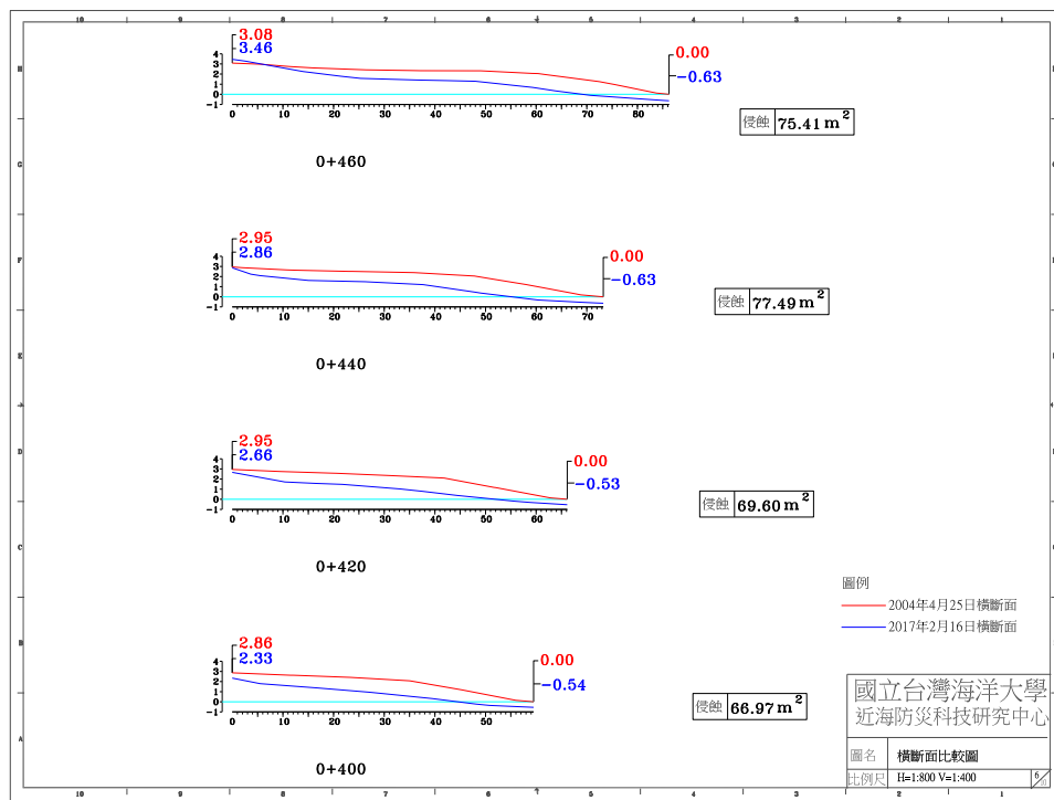
圖 4-4(e) 2017 年 2 月 16 日 A 監測區橫斷面比較圖
