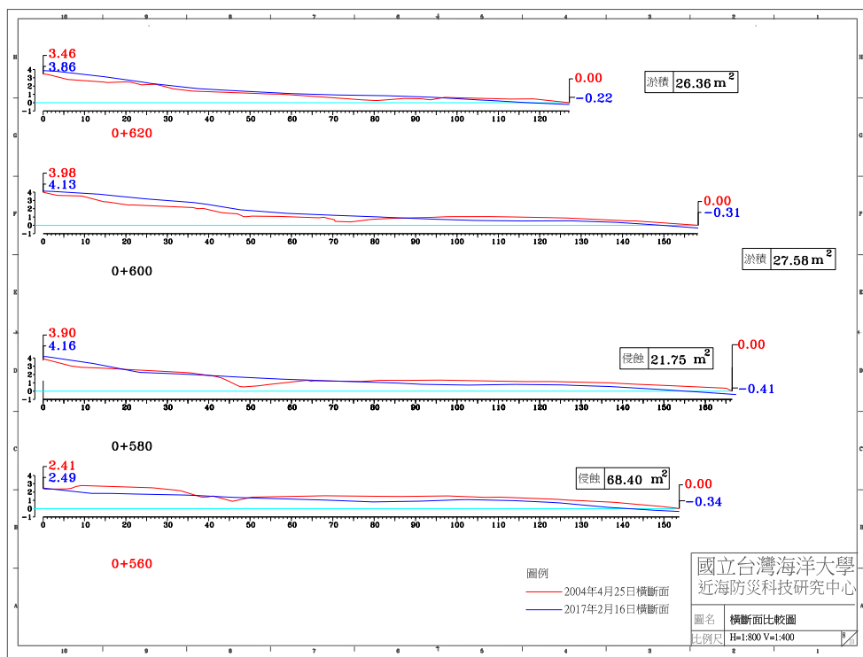
圖 4-4(c) 2017 年 2 月 16 日 A 監測區橫斷面比較圖
