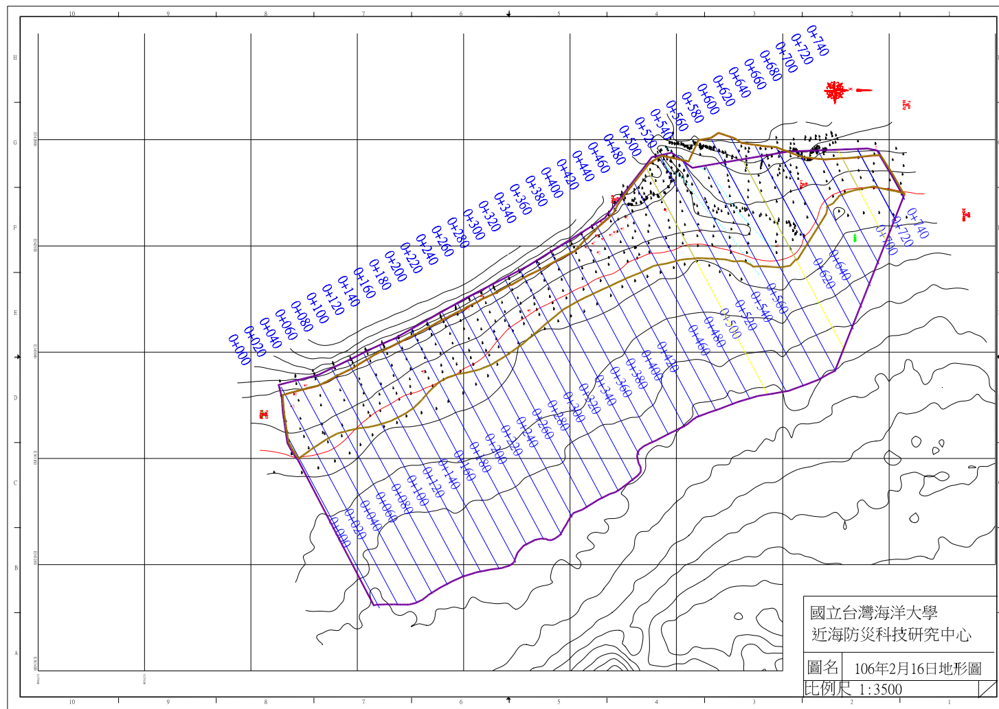
圖 4-1 2017 年 2 月 16 日監測地形圖
