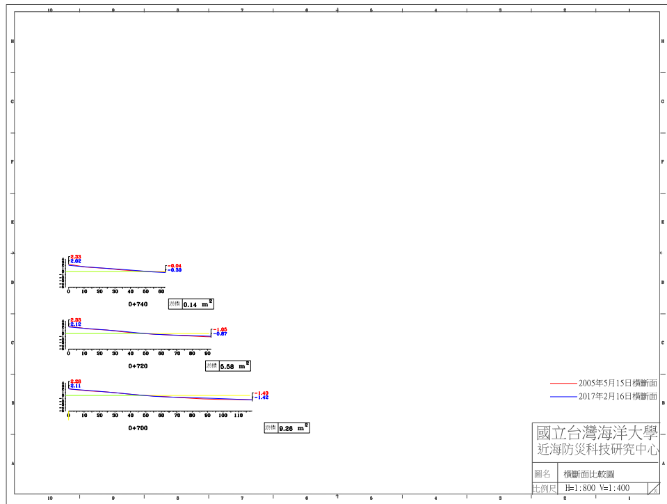
圖 4-5(a) 2017 年 2 月 16 日 B 監測區橫斷面比較圖
