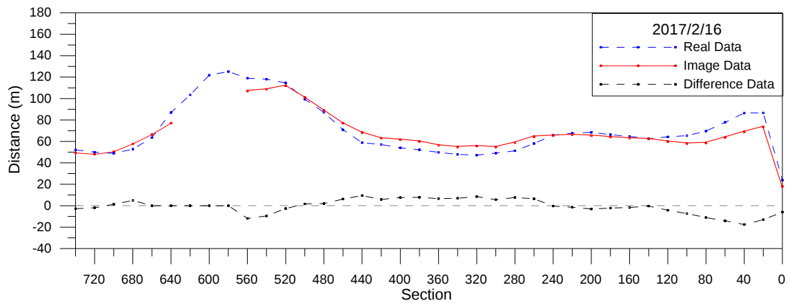
圖 3-23 海岸線分析比較圖(2017/2/16)
