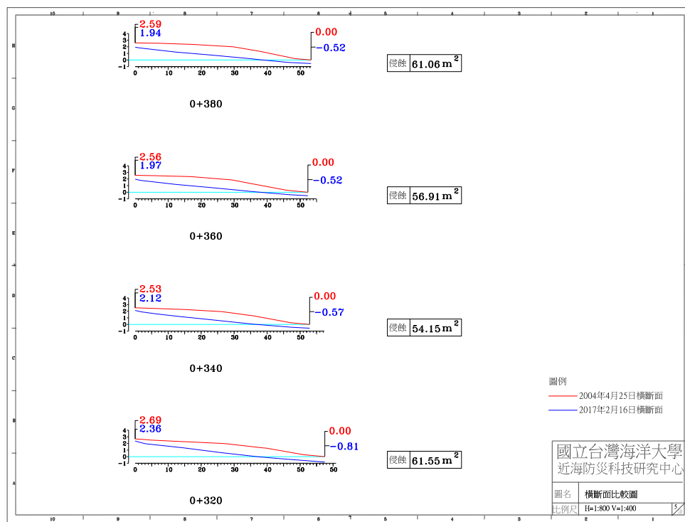
圖 4-4(f) 2017 年 2 月 16 日 A 監測區橫斷面比較圖
