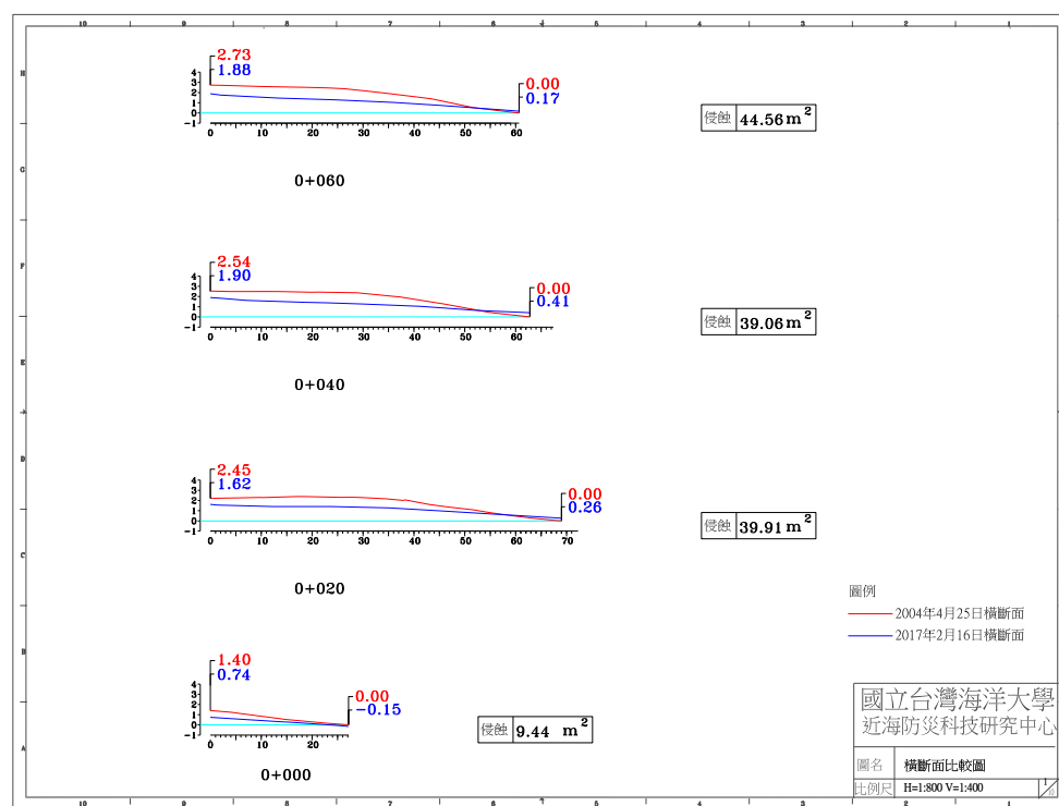
圖 4-4(j) 2017 年 2 月 16 日 A 監測區橫斷面比較圖
