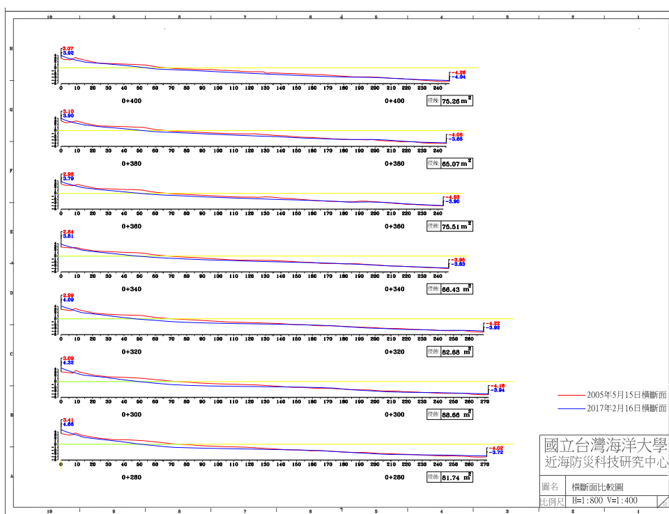
圖 4-5(d) 2017 年 2 月 16 日 B 監測區橫斷面比較圖
