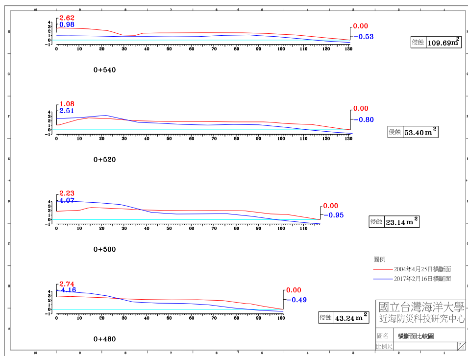
圖 4-4(d) 2017 年 2 月 16 日 A 監測區橫斷面比較圖
