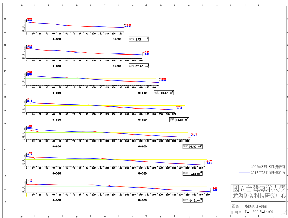
圖 4-5(b) 2017 年 2 月 16 日 B 監測區橫斷面比較圖
