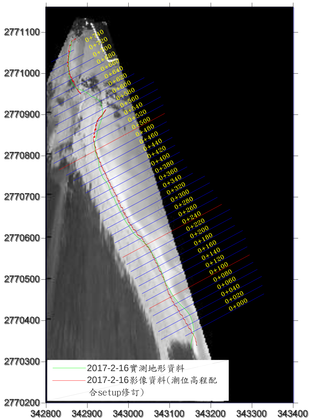
圖 3-22 水位線分析結果圖(2017/2/16)
