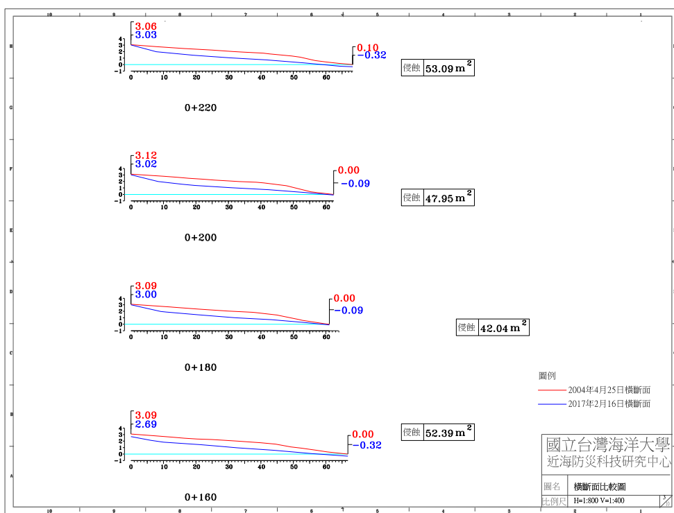
圖 4-4(h) 2017 年 2 月 16 日 A 監測區橫斷面比較圖
