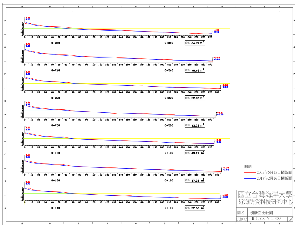
圖 4-5(e) 2017 年 2 月 16 日 B 監測區橫斷面比較圖
