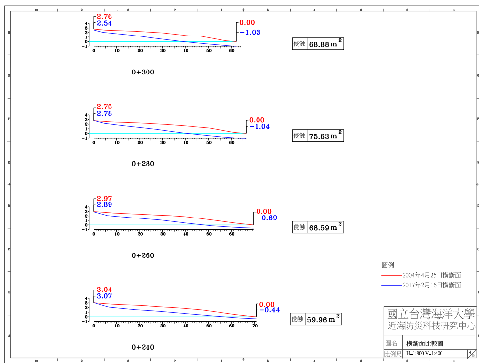
圖 4-4(g) 2017 年 2 月 16 日 A 監測區橫斷面比較圖
