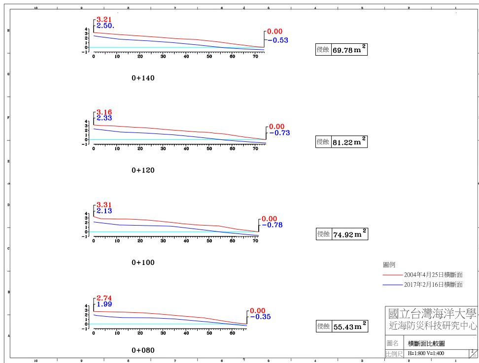
圖 4-4(i) 2017 年 2 月 16 日 A 監測區橫斷面比較圖
