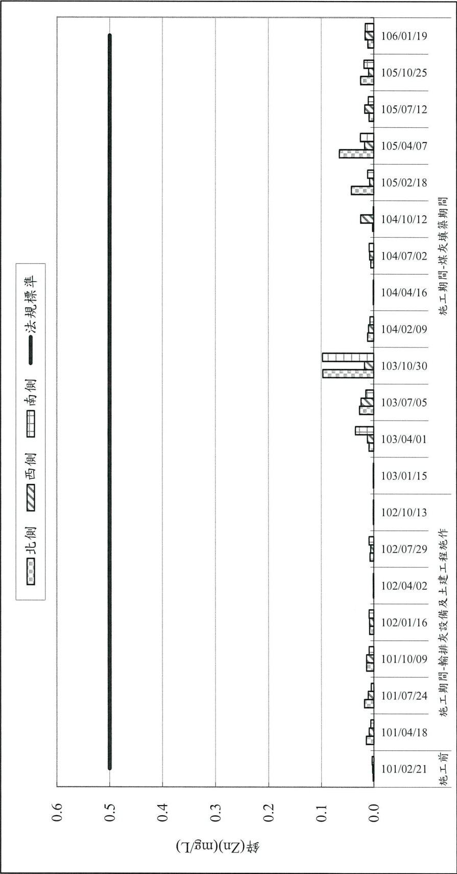
圖 2.2-9 歷季各測站鋅(Zn)監測成果彙整
