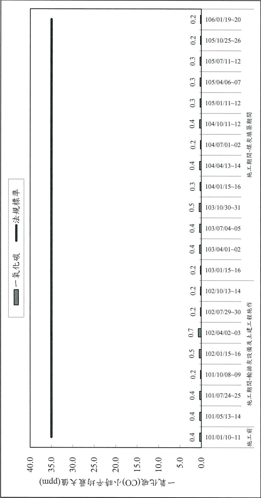
圖 2.1-6 歷季一氧化碳(CO)小時平均最大值監測成果彙整
