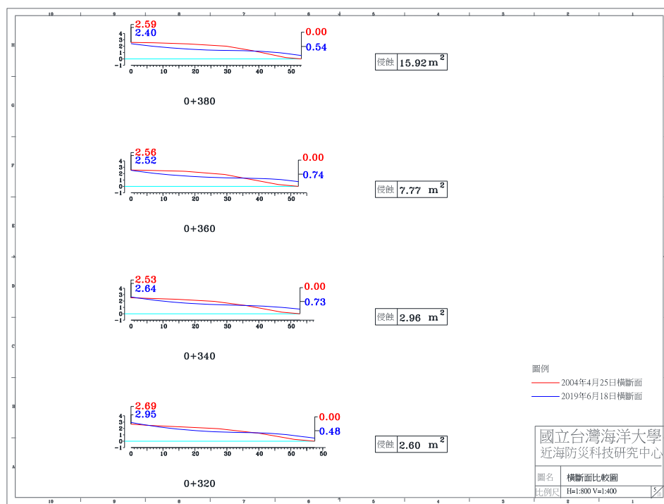
圖 4-4(f) 2019 年 6 月 18 日 A 監測區橫斷面比較圖
