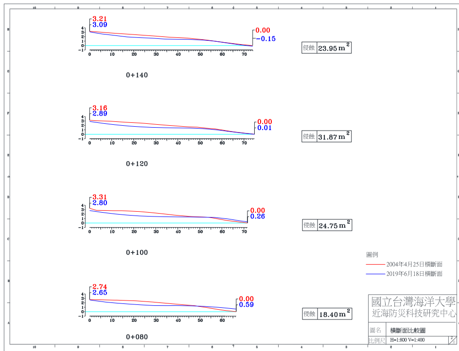
圖 4-4(i) 2019 年 6 月 18 日 A 監測區橫斷面比較圖
