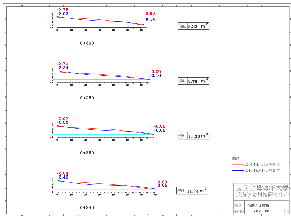
圖 4-4(g) 2019 年 6 月 18 日 A 監測區橫斷面比較圖
