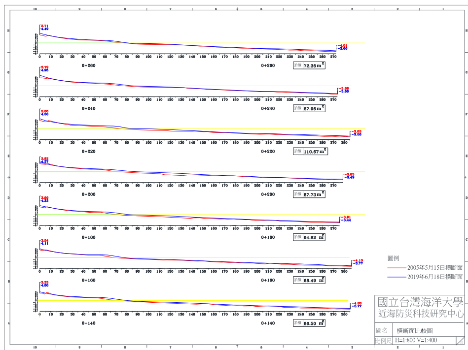
圖 4-5(e) 2019 年 6 月 18 日 B 監測區橫斷面比較圖
