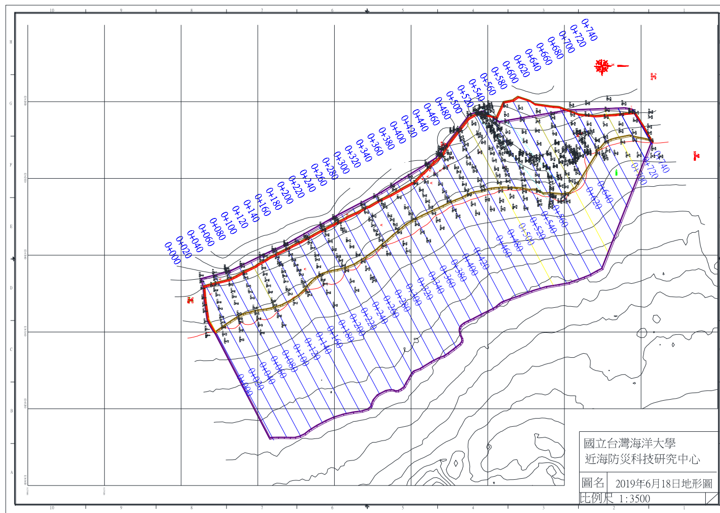
圖 4-1 2019 年 6 月 18 日監測地形圖
