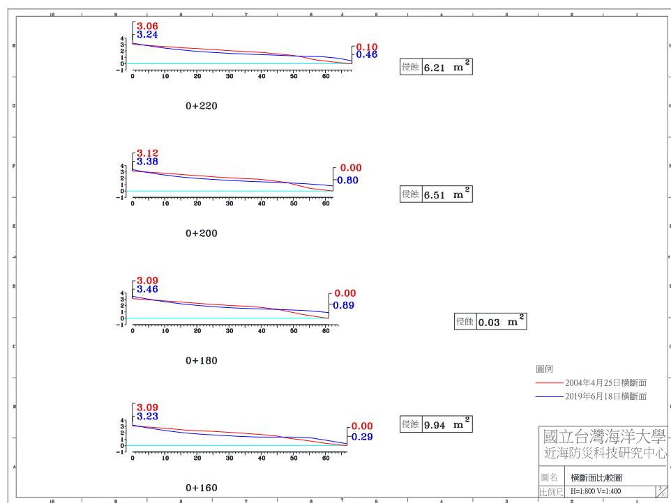
圖 4-4(h) 2019 年 6 月 18 日 A 監測區橫斷面比較圖
