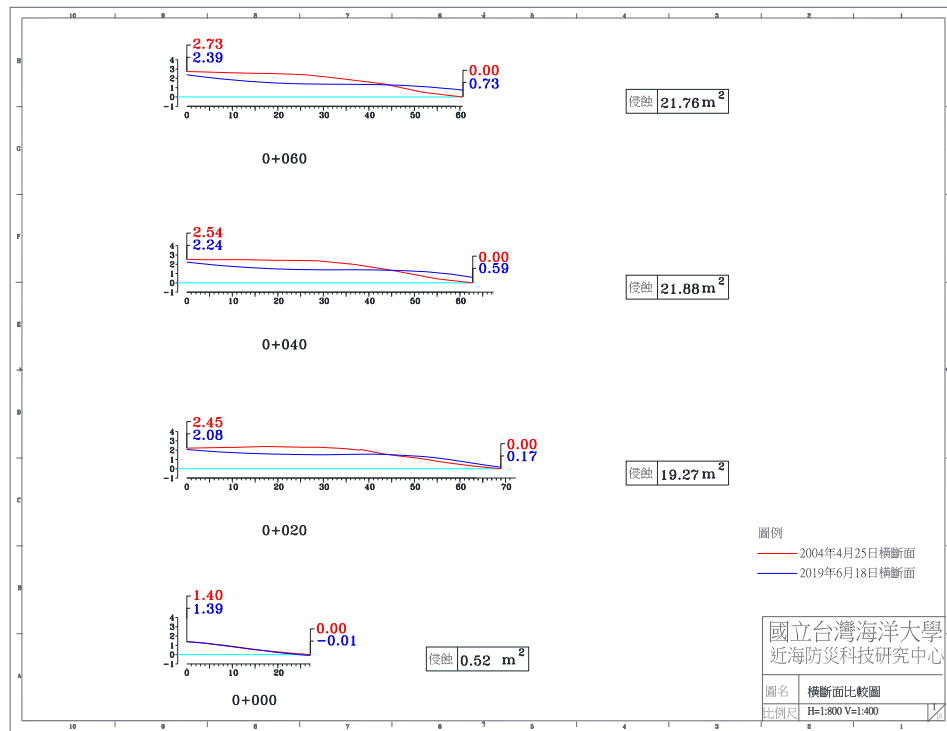
圖 4-4(j) 2019 年 6 月 18 日 A 監測區橫斷面比較圖
