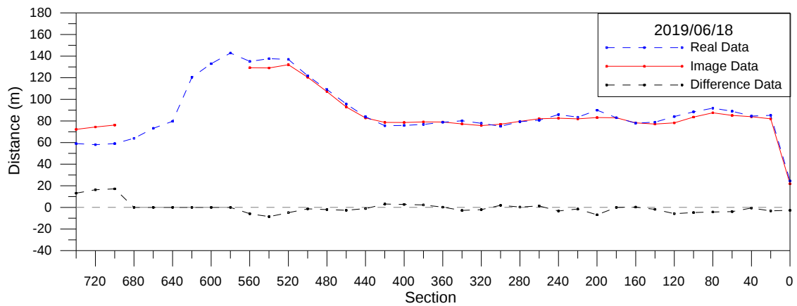
圖 3-23 海岸線分析比較圖(2019/6/18)
