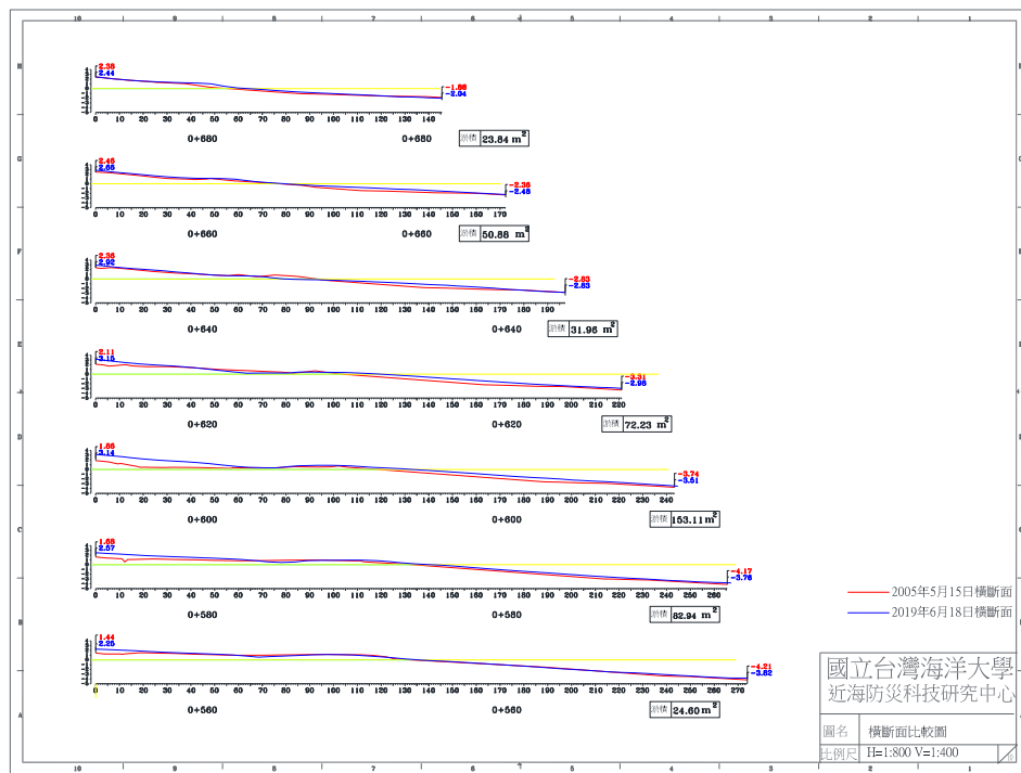
圖 4-5(b) 2019 年 6 月 18 日 B 監測區橫斷面比較圖
