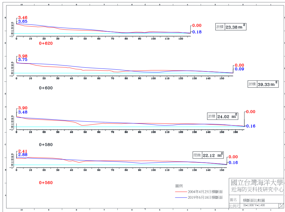
圖 4-4(c) 2019 年 6 月 18 日 A 監測區橫斷面比較圖
