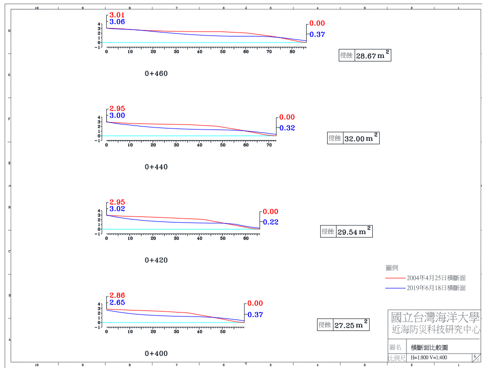
圖 4-4(e) 2019 年 6 月 18 日 A 監測區橫斷面比較圖
