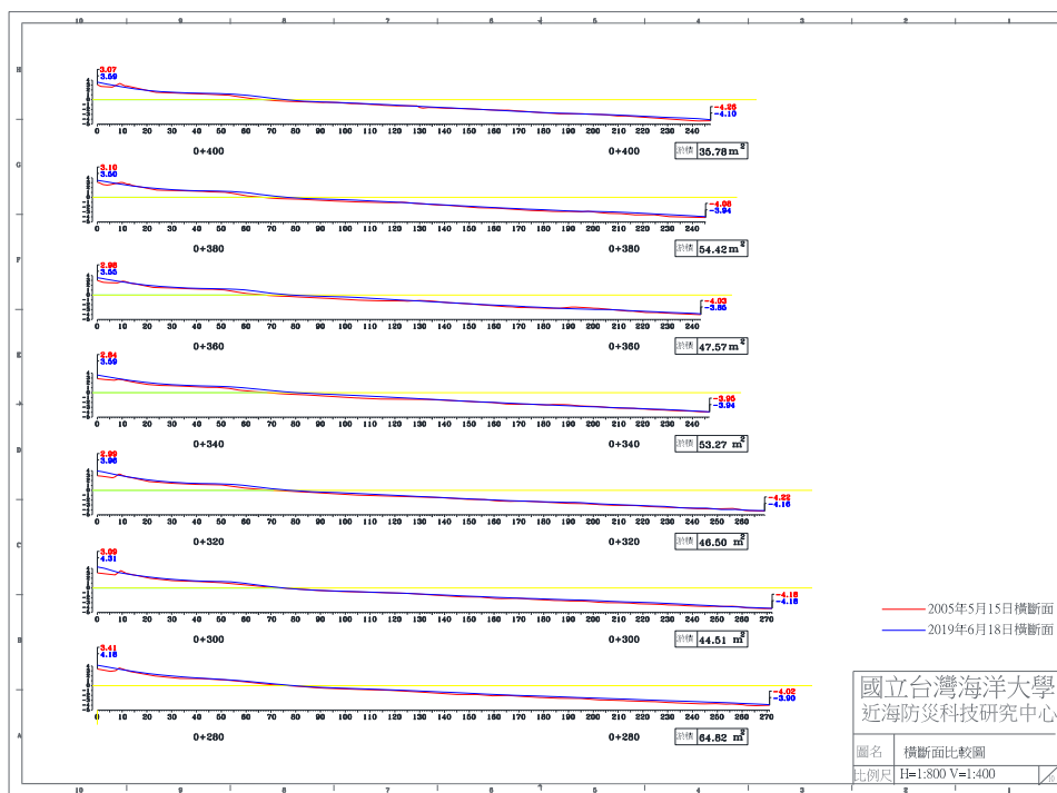
圖 4-5(d) 2019 年 6 月 18 日 B 監測區橫斷面比較圖
