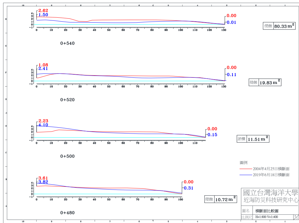
圖 4-4(d) 2019 年 6 月 18 日 A 監測區橫斷面比較圖
