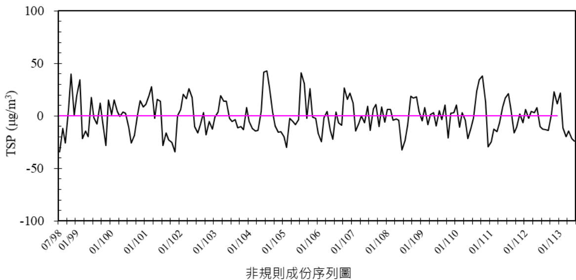
圖 2.6- 24 土庫站 98 年 7 月至 113 年 6 月總懸浮微粒濃度趨勢圖
