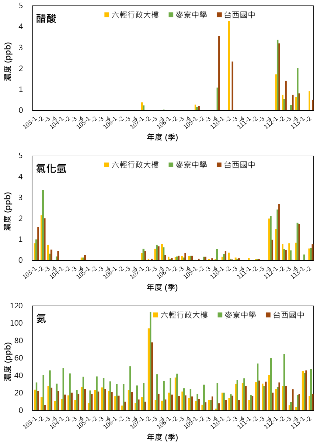
圖 2.5- 3 103 年至 113 年第二季逸散性氣體監測物種濃度比較圖（續）
