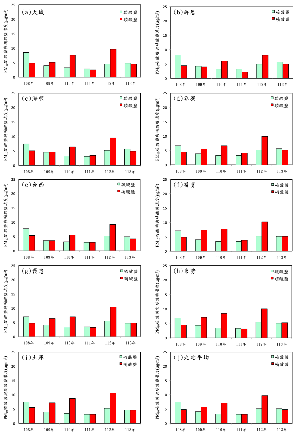
圖 2.2- 2 108 年至 113 年第二季 PM_{10} 硫酸鹽與硝酸鹽平均濃度
