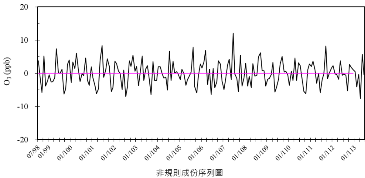
圖 2.6- 16 麥寮站 98 年 7 月至 113 年 6 月臭氧濃度趨勢圖
