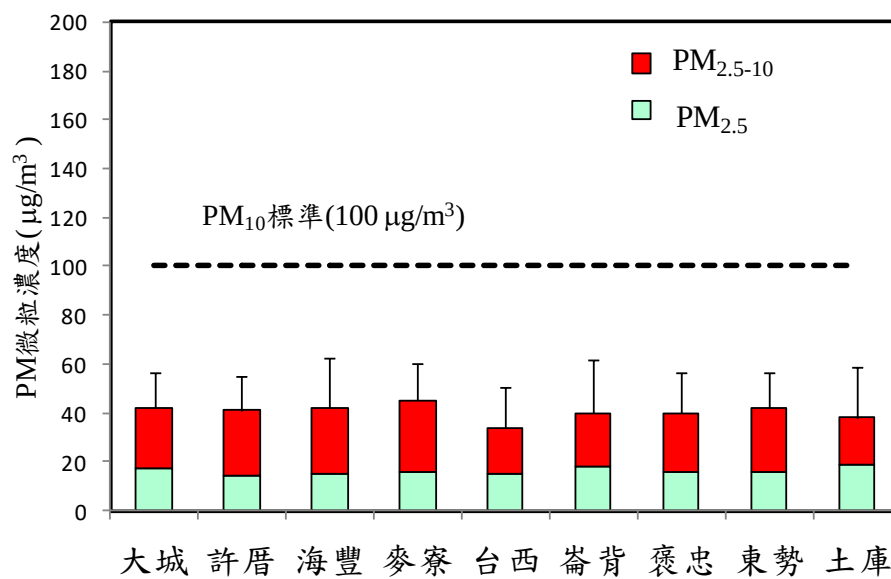
圖 2.1- 2 113 年第二季 PM 2.5 及 PM 2.5-10 粒子質量平均濃度
