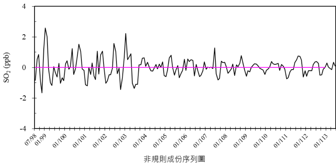
圖 2.6- 8 台西站 98 年 7 月至 113 年 6 月二氧化硫濃度趨勢圖
