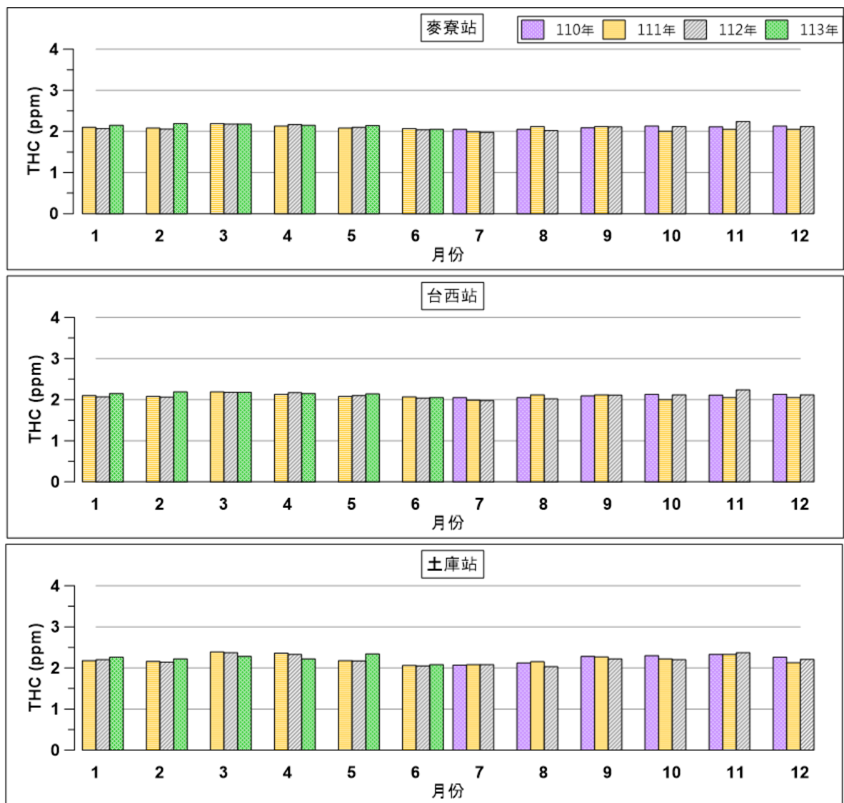
圖 2.6- 32 環評 3 站 110 年 7 月至 113 年 6 月總碳氫化合物月均值比較圖
