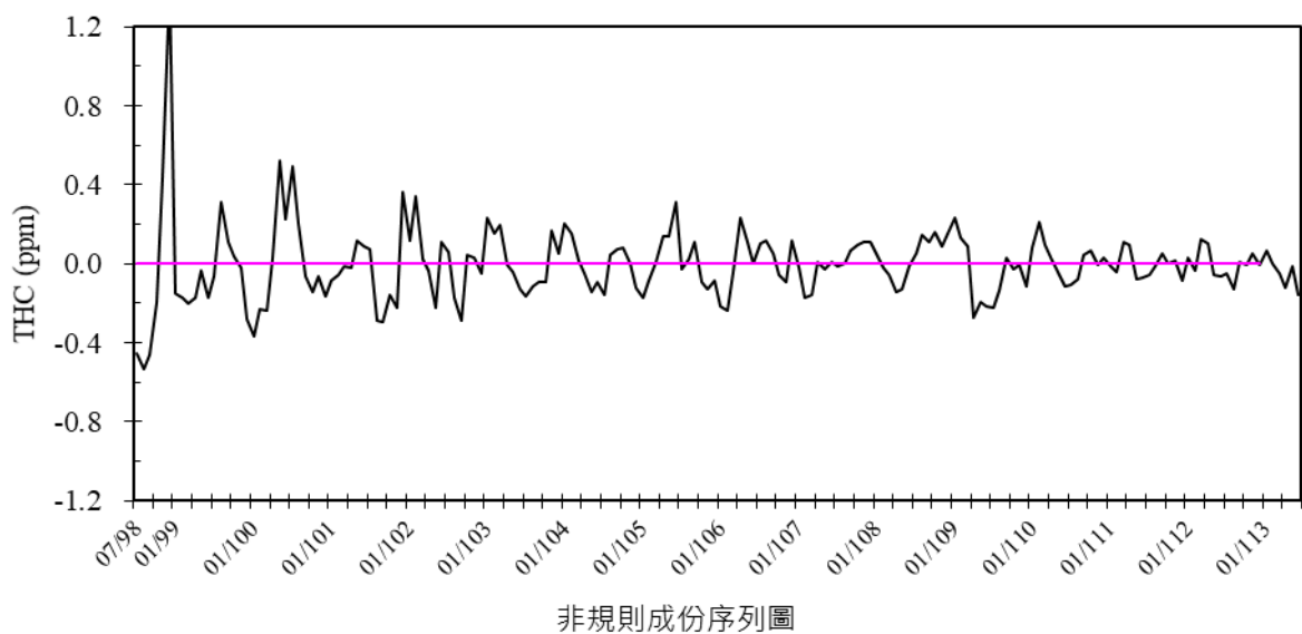
圖 2.6- 6 土庫站 98 年 7 月至 113 年 6 月總碳氫化合物濃度趨勢圖
