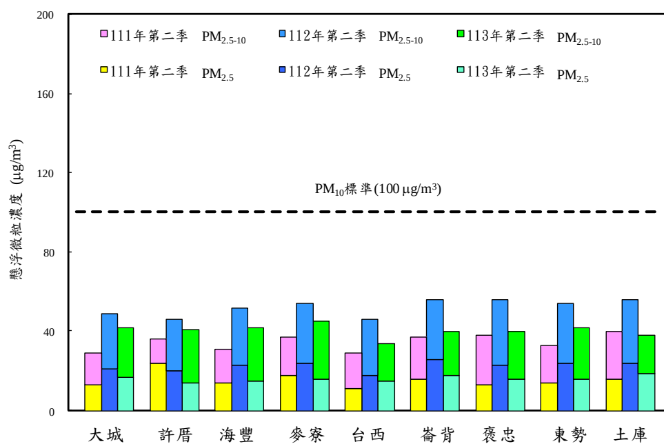
圖 2.1- 4 113 年第二季與歷年同季 PM_{2.5} 及 PM_{2.5-10} 粒子質量平均濃度比較
