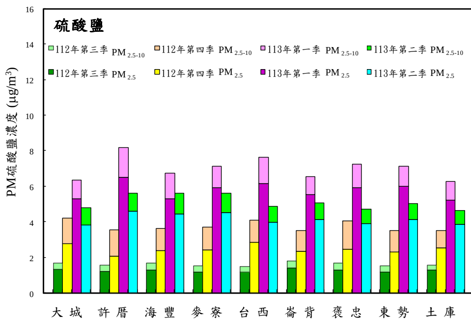
圖 2.1- 7 113 年第二季與前三季 PM 2.5 及 PM 2.5-10 硫酸鹽濃度比較
