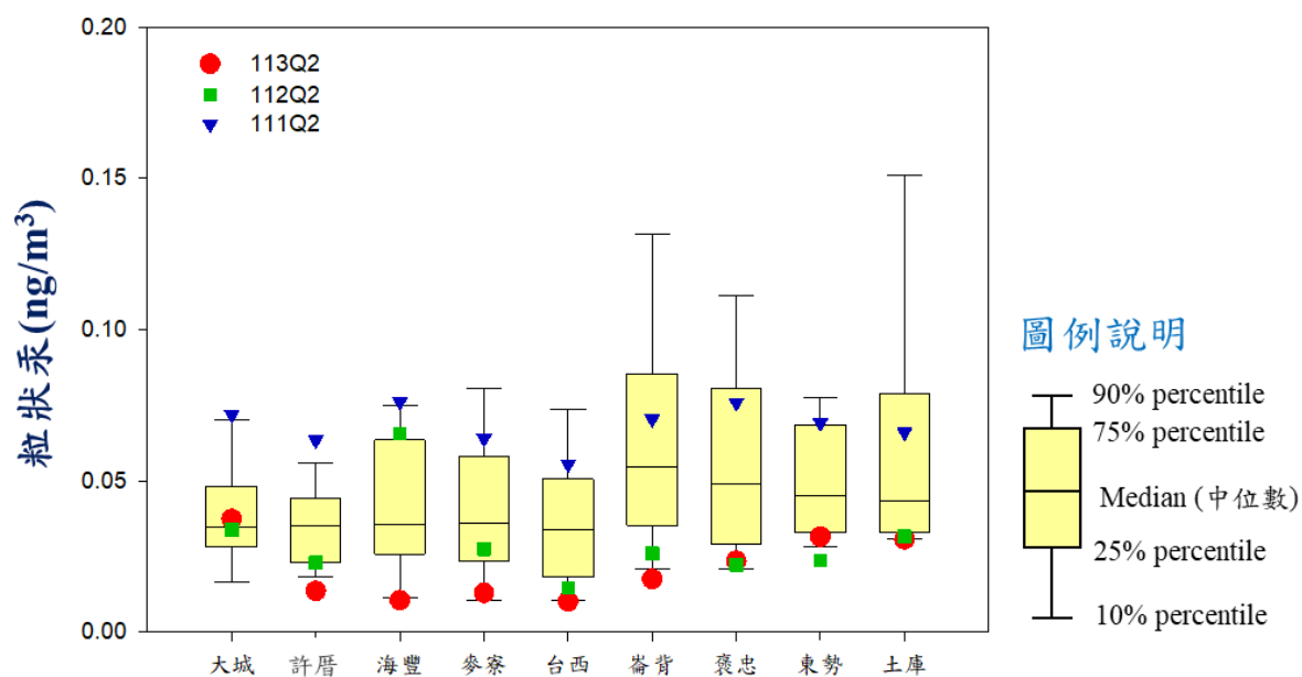
圖 2.3- 3 108 年第二季至 113 年第二季各測站粒狀汞 (ng/m 3 )
