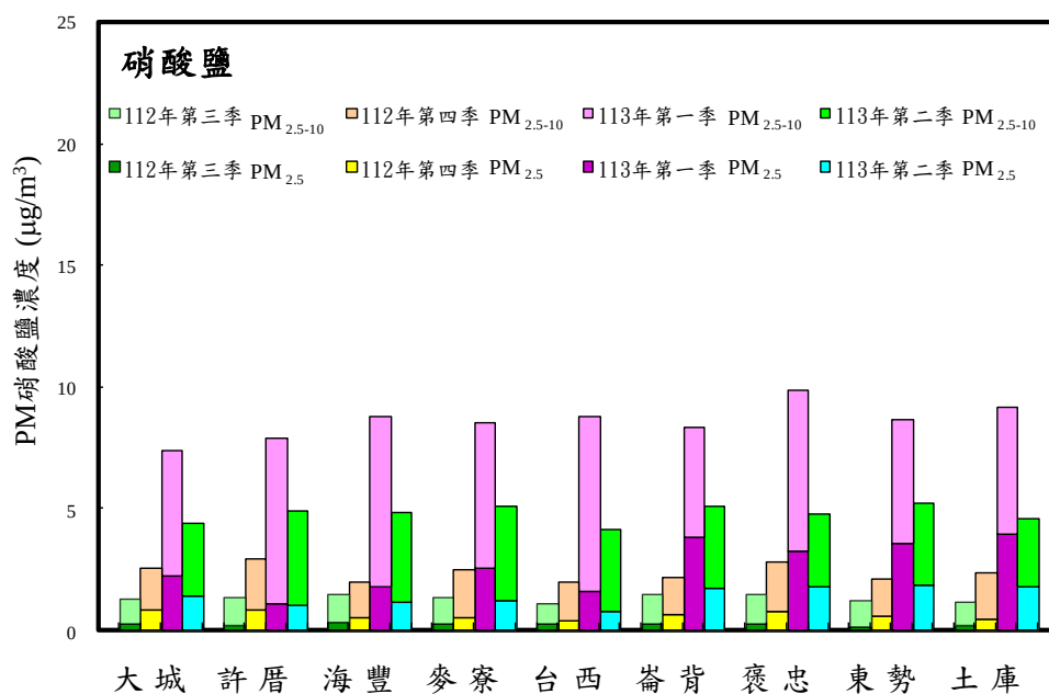
圖 2.1-8 113 年第二季與前三季 PM 2.5 及 PM 2.5-10 硝酸鹽濃度比較
