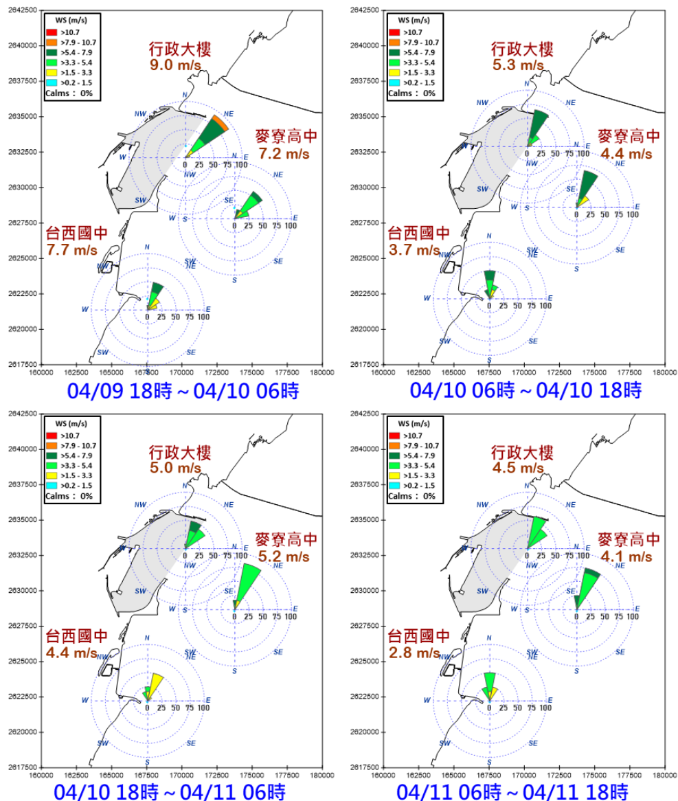
圖 2.4- 1 113 年第二季逸散性氣體採樣期間風玫瑰圖
