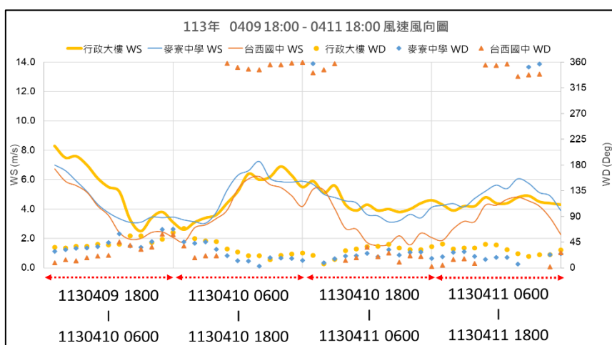
圖 2.5- 2 113 年第二季採樣期間風速風向圖
