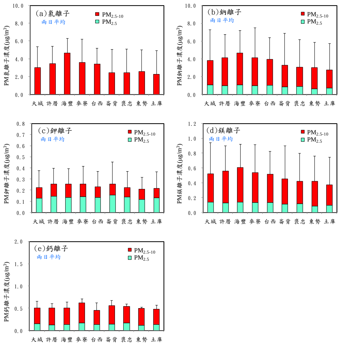
圖 2.1- 14 113 年第二季 PM 2.5 及 PM 2.5-10 水溶性無機離子平均濃度圖
