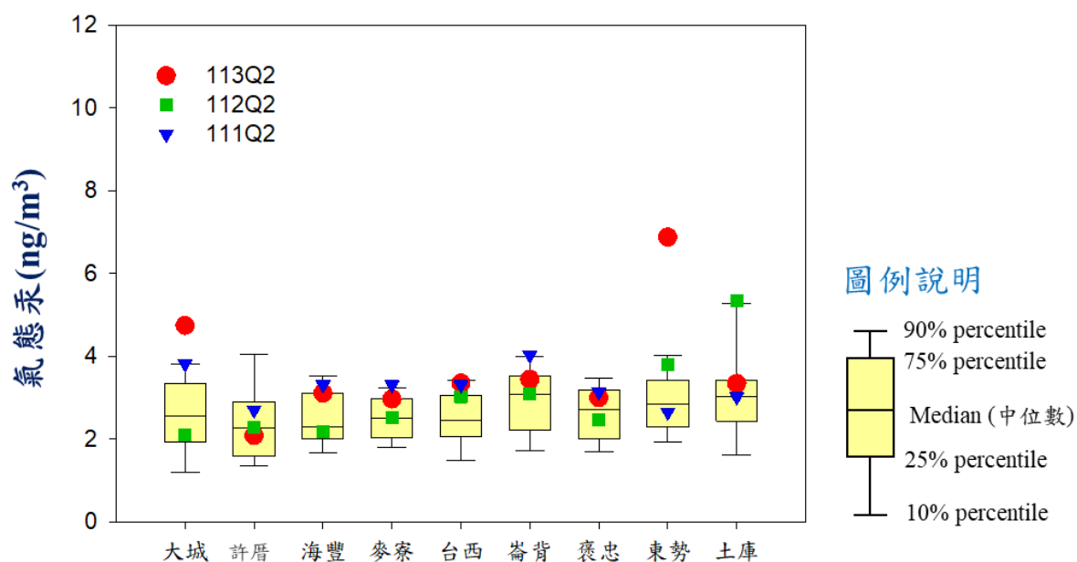
圖 2.3- 4 108 年第二季至 113 年第二季各測站氣態汞 (ng/m 3 )
