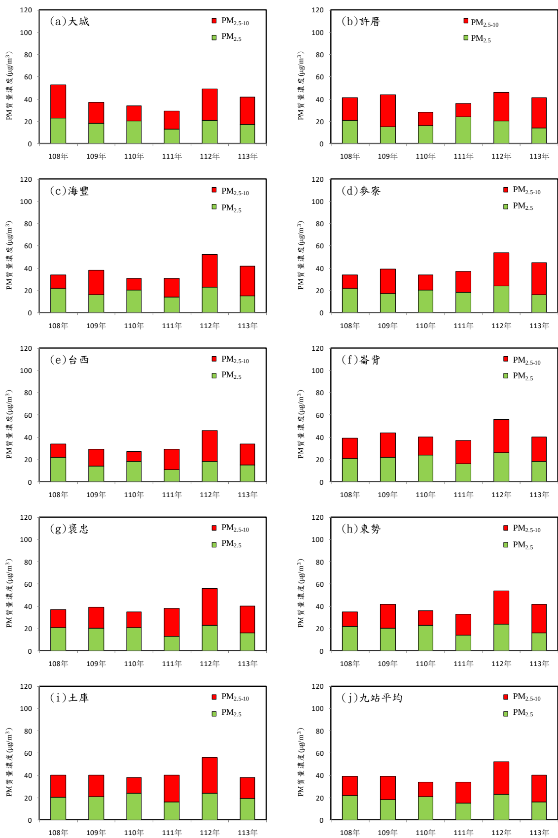
圖 2.2- 1 108 年至 113 年第二季 PM 2.5 、PM 10 粒子質量濃度比較圖
