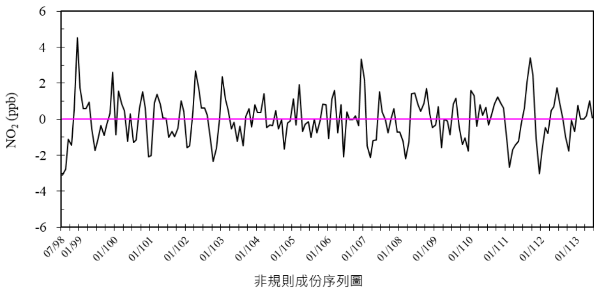
圖 2.6- 11 台西站 98 年 7 月至 113 年 6 月二氧化氮濃度趨勢圖
