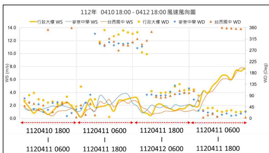
圖 2.5- 1 112 年第二季採樣期間風速風向圖
