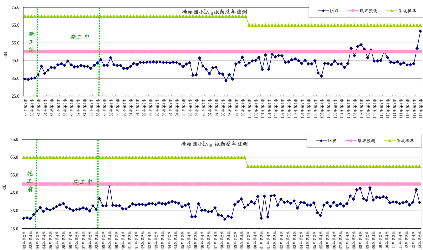
圖3-36 橋頭國小測點振動歷年監測變化趨勢圖
