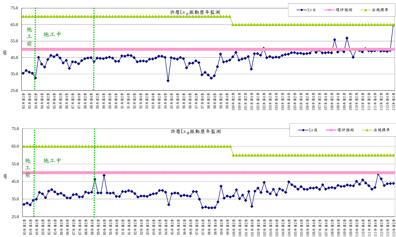
圖3-37 許厝厝測點振動歷年監測變化趨勢圖
