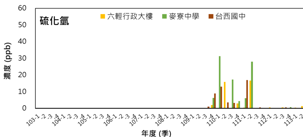
圖 2.5- 3 103 年至 113 年第二季逸散性氣體監測物種濃度比較圖（續）
