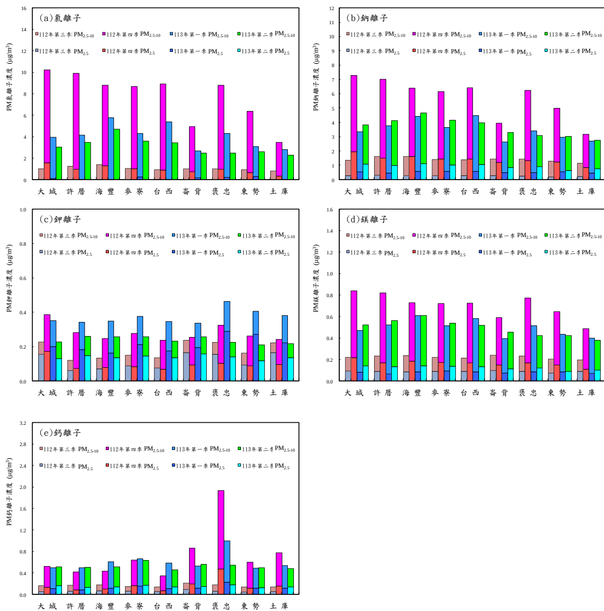
圖 2.1- 15 113 年第二季及前三季 PM 2.5 及 PM 2.5-10 水溶性無機離子平均濃度圖
