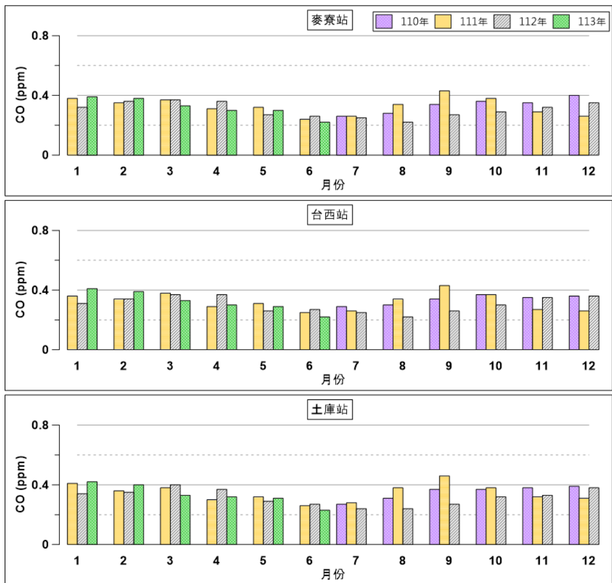
圖 2.6- 35 環評 3 站 110 年 7 月至 113 年 6 月一氧化碳月均值比較圖
