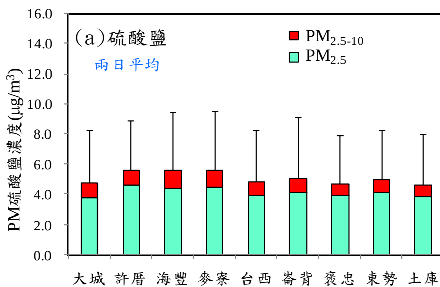
圖 2.1- 5 113 年第二季 PM_{2.5} 及 PM_{2.5-10} 硫酸鹽平均濃度
