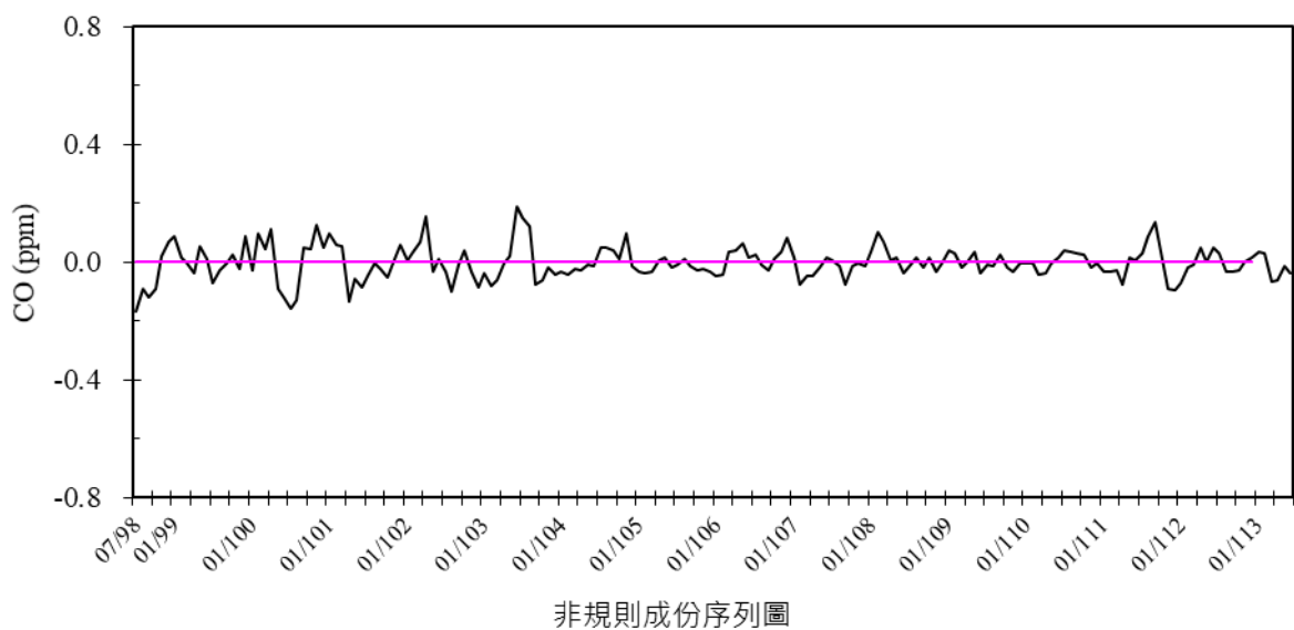
圖 2.6- 14 台西站 98 年 7 月至 113 年 6 月一氧化碳濃度趨勢圖
