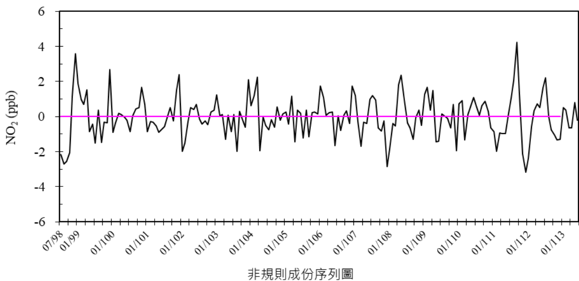
圖 2.6- 10 麥寮站 98 年 7 月至 113 年 6 月二氧化氮濃度趨勢圖
