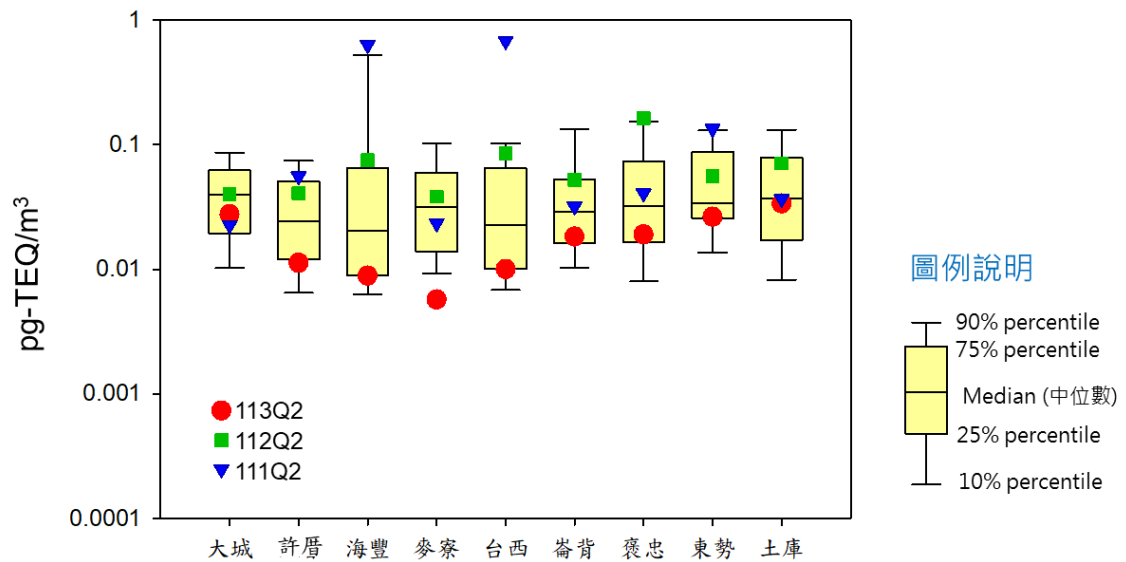
圖 2.3- 2 108 年第二季至 113 年第二季各測站戴奧辛及呋喃監測結果比較
