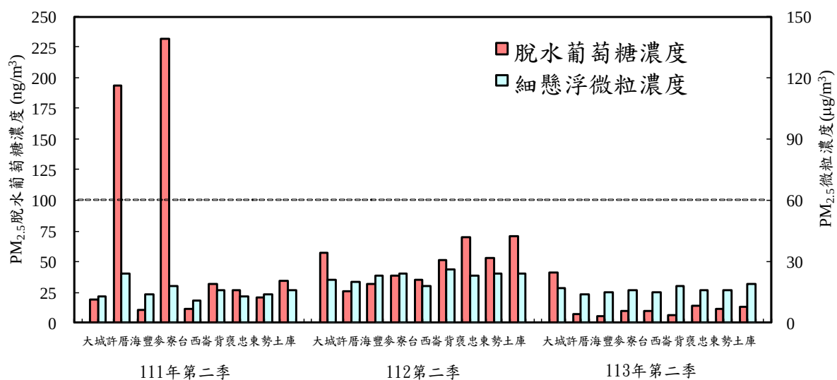
圖 2.1- 12 111 年至 113 年第二季 PM 2.5 脫水葡萄糖與粒子濃度比較
