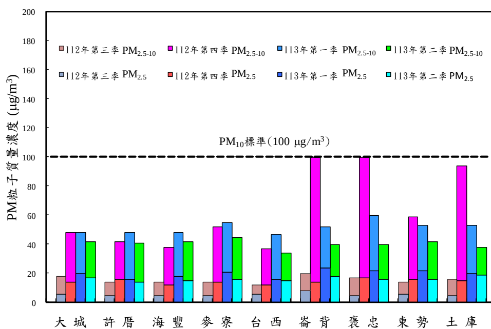
圖 2.1- 3 113 年第二季與前三季 PM 2.5 及 PM 2.5-10 粒子質量平均濃度比較
