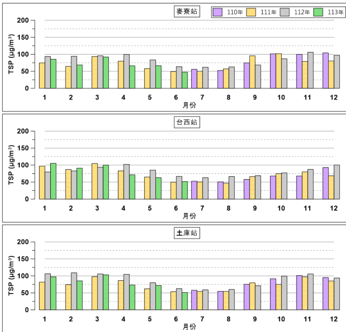
圖 2.6- 38 環評 3 站 110 年 7 月至 113 年 6 月總懸浮微粒月均值比較圖
