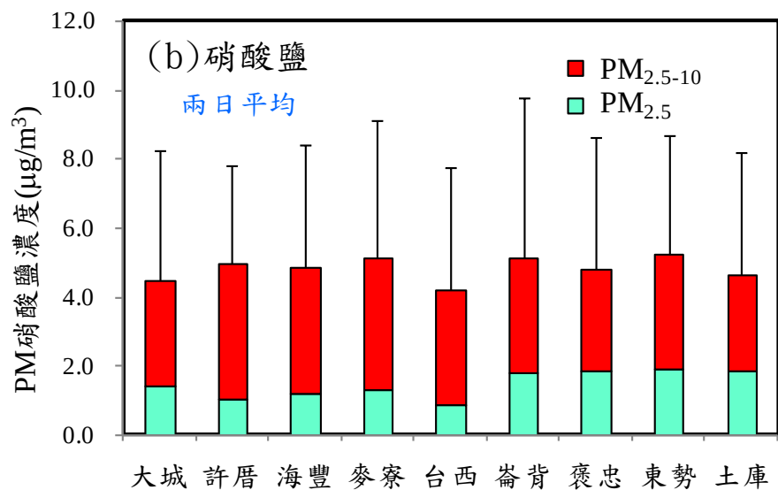
圖 2.1- 6 113 年第二季 PM 2.5 及 PM 2.5-10 硝酸鹽平均濃度
