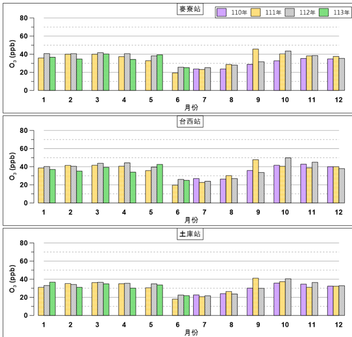
圖 2.6- 36 環評 3 站 110 年 7 月至 113 年 6 月臭氧月均值比較圖
