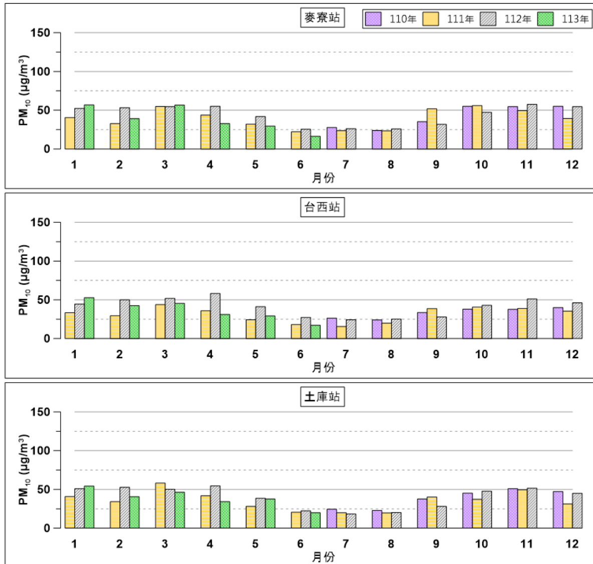
圖 2.6- 31 環評 3 站 110 年 7 月至 113 年 6 月懸浮微粒月均值比較圖
