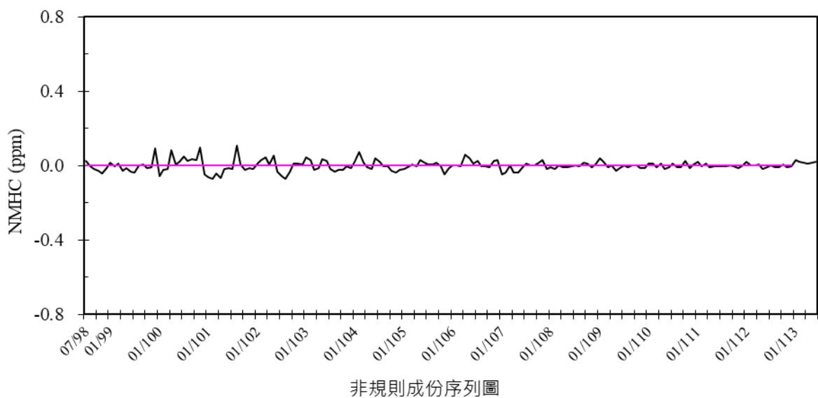
圖 2.6- 19 麥寮站 98 年 7 月至 113 年 6 月非甲烷碳氫化合物濃度趨勢圖
