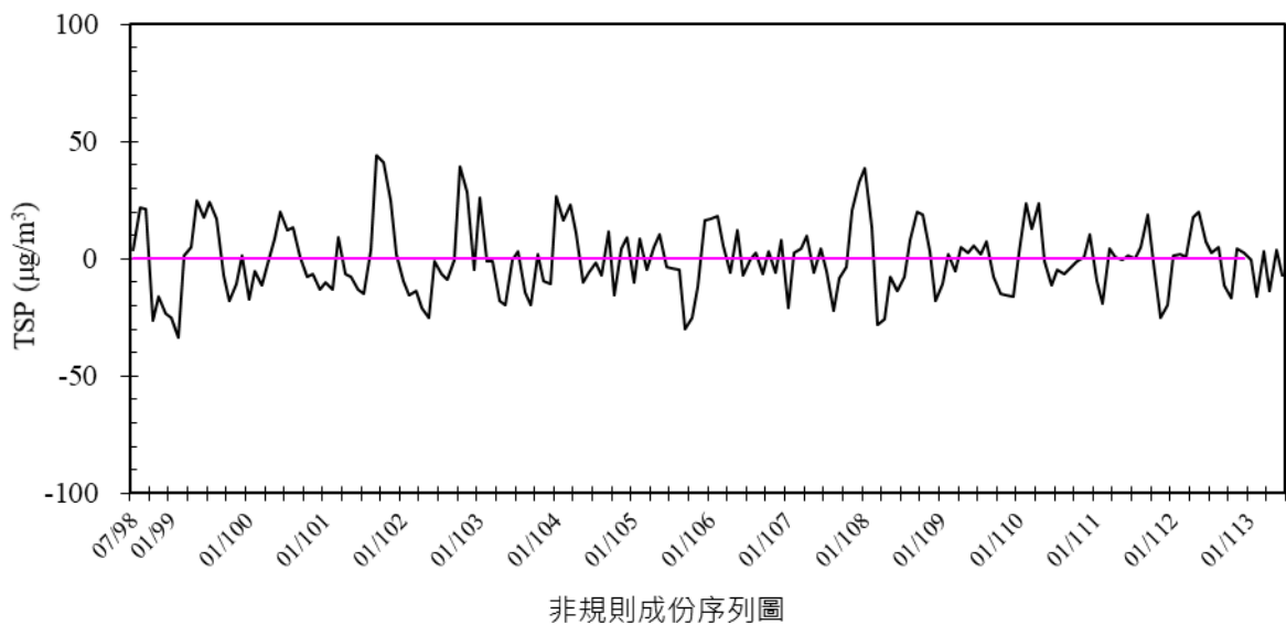
圖 2.6- 22 麥寮站 98 年 7 月至 113 年 6 月總懸浮微粒濃度趨勢圖
