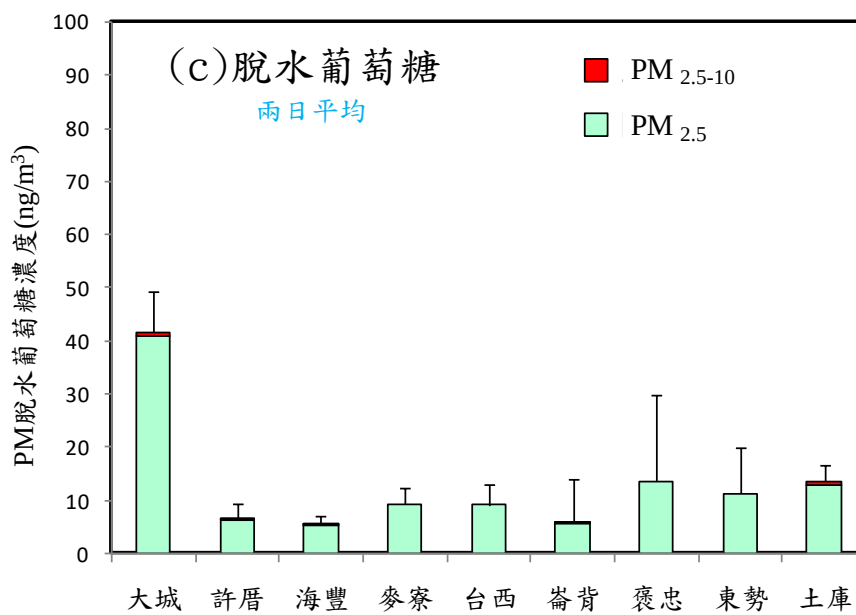
圖 2.1- 11 113 年第二季脫水葡萄糖質量濃度
