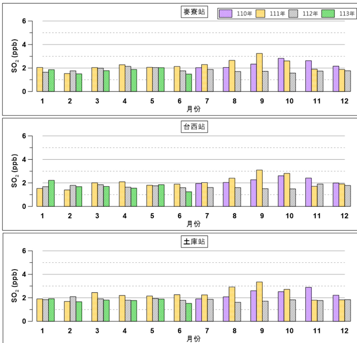
圖 2.6- 33 環評 3 站 110 年 7 月至 113 年 6 月二氧化硫月均值比較圖
