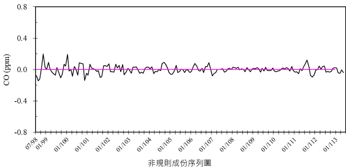
圖 2.6- 13 麥寮站 98 年 7 月至 113 年 6 月一氧化碳濃度趨勢圖
