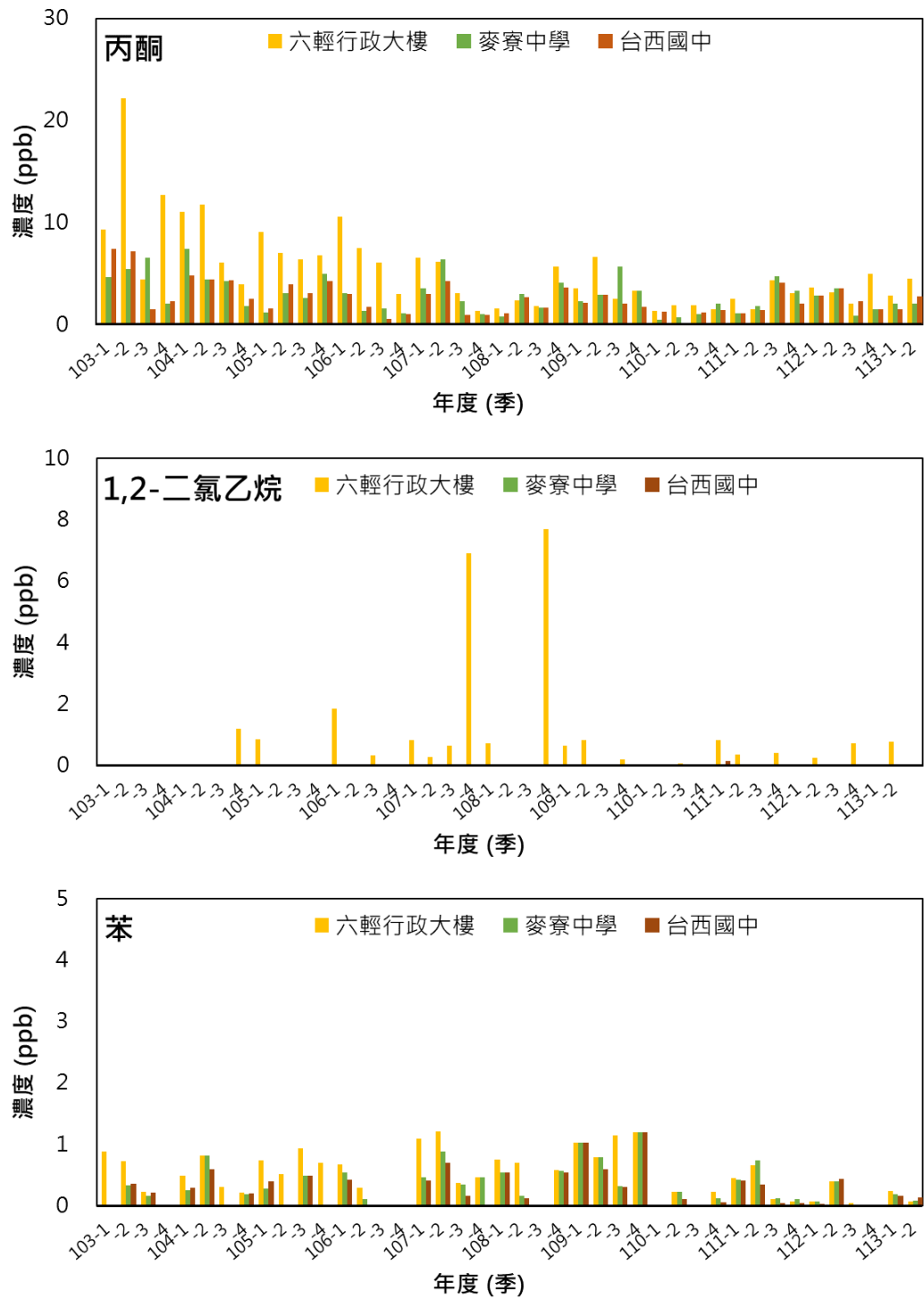
圖 2.5- 3 103 年至 113 年第二季逸散性氣體監測物種濃度比較圖
