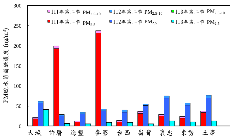
圖 2.1- 13 113 年第二季與歷年同季 PM 2.5 及 PM 2.5-10 脫水葡萄糖濃度比較
