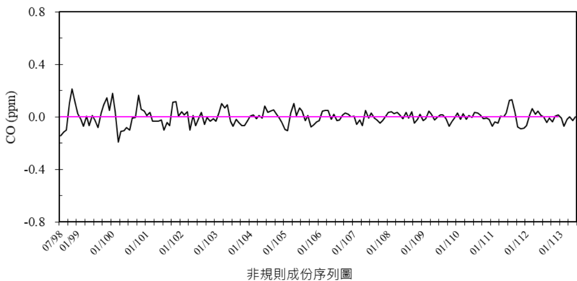
圖 2.6- 15 土庫站 98 年 7 月至 113 年 6 月一氧化碳濃度趨勢圖
