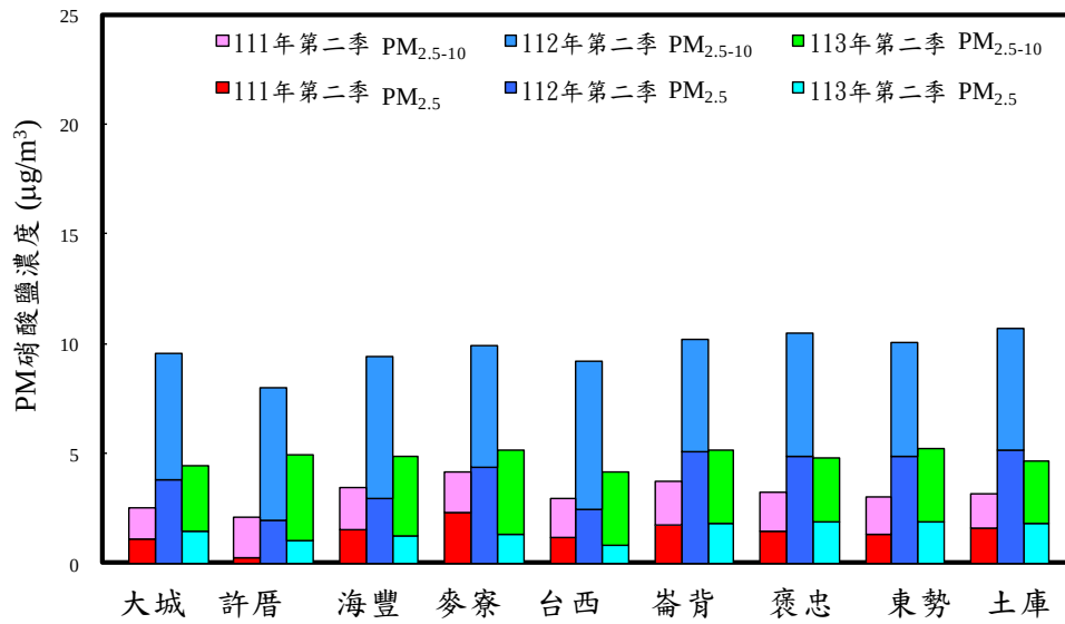
圖 2.1- 10 113 年第二季與歷年同季 PM 2.5 及 PM 2.5-10 硝酸鹽濃度比較
