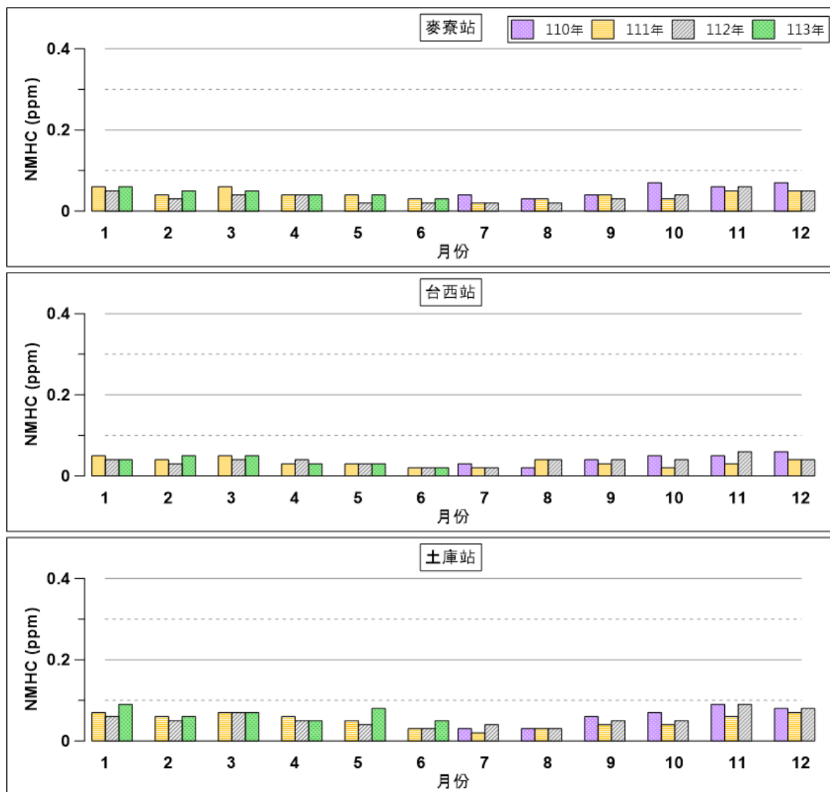
圖 2.6- 37 環評 3 站 110 年 7 月至 113 年 6 月非甲烷碳氫化合物月均值比較圖
