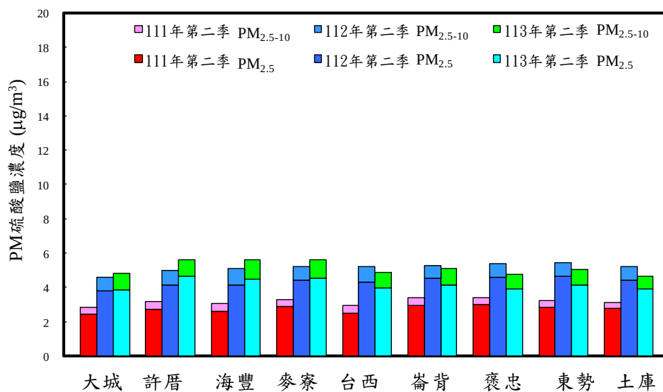
圖 2.1-9 113 年第二季與歷年同季 PM 2.5 及 PM 2.5-10 硫酸鹽濃度比較
