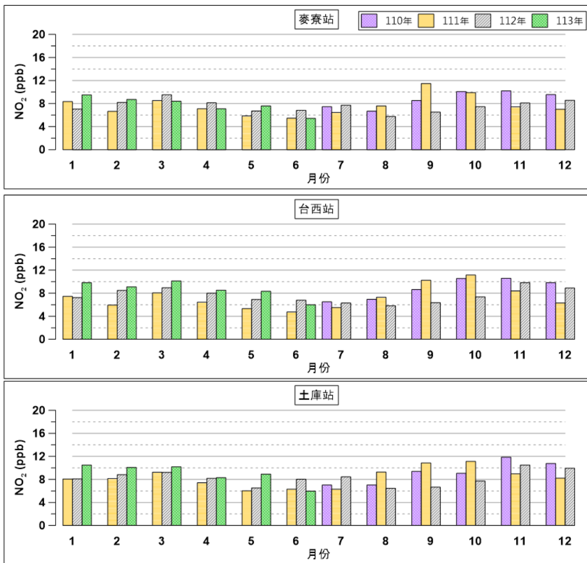
圖 2.6- 34 環評 3 站 110 年 7 月至 113 年 6 月二氧化氮月均值比較圖
