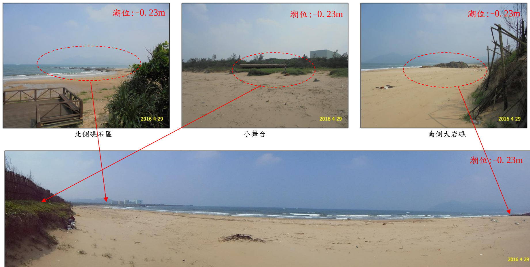
圖 3-6 鹽寮海岸短期性養灘區地形地貌圖(2016/4/29)
