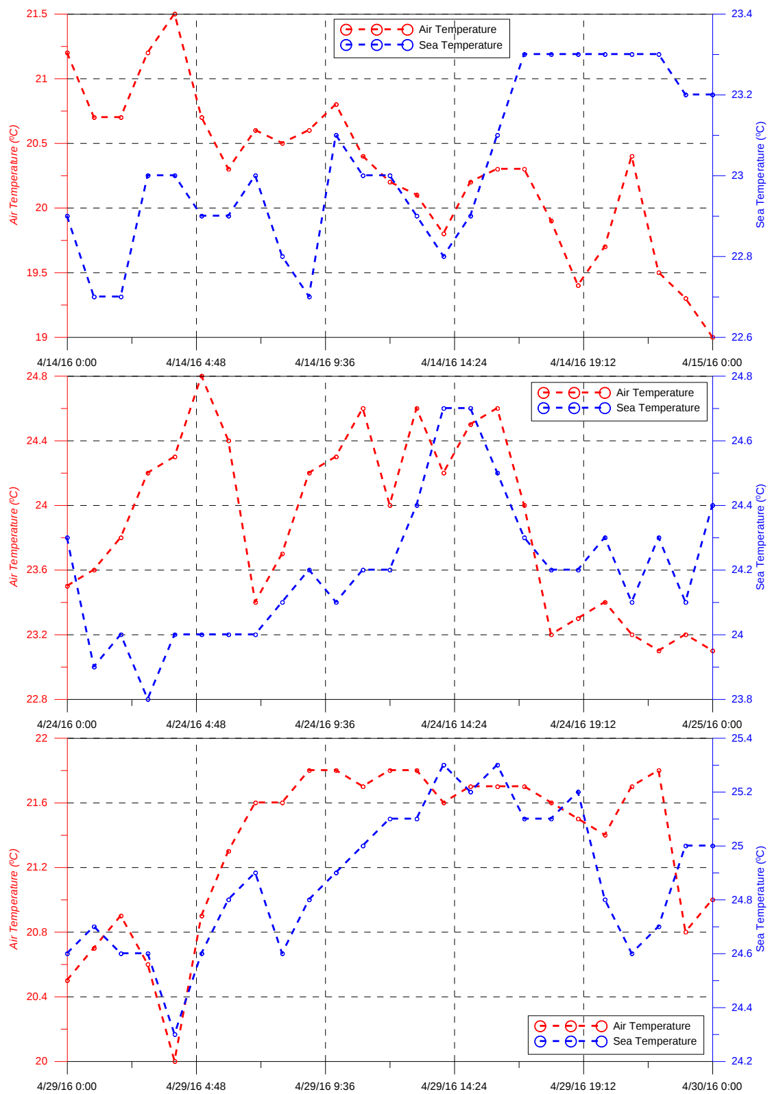
圖 2-4 溫度時序列變化圖
