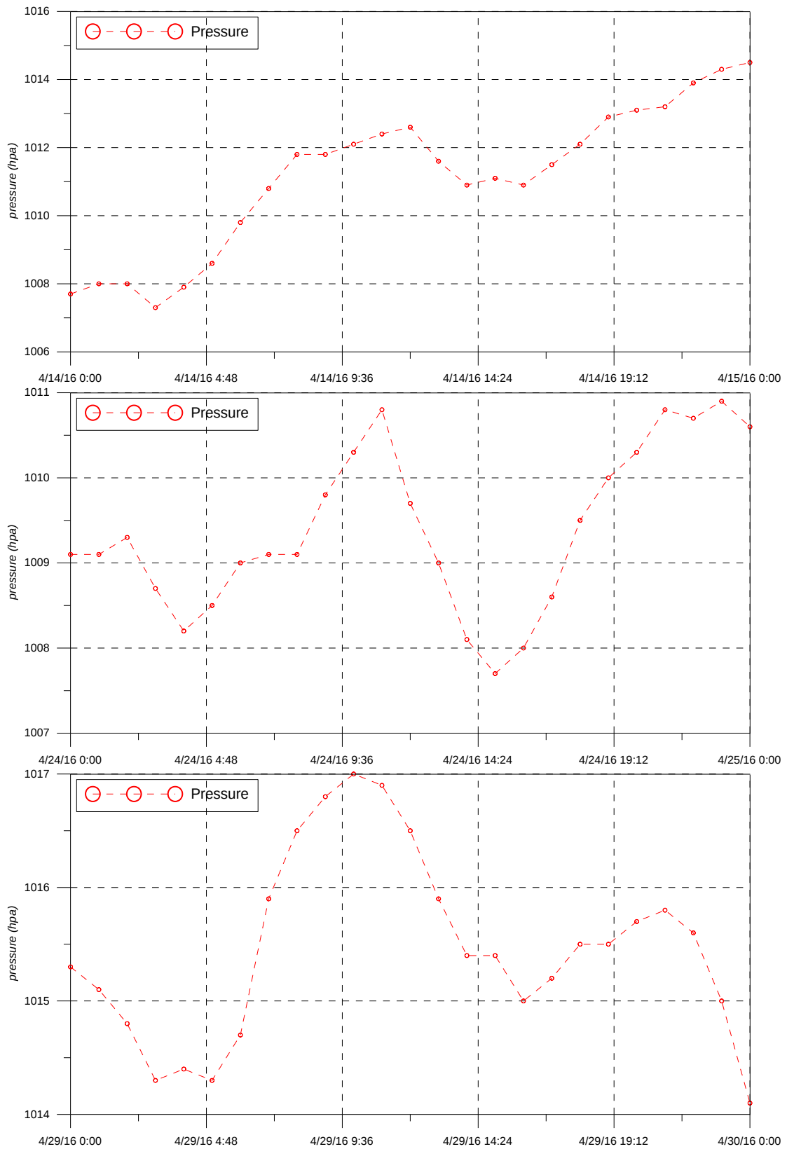
圖 2-5 壓力時序列變化圖
