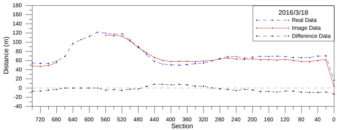
圖 3-23 海岸線分析比較圖(2016/3/18)
