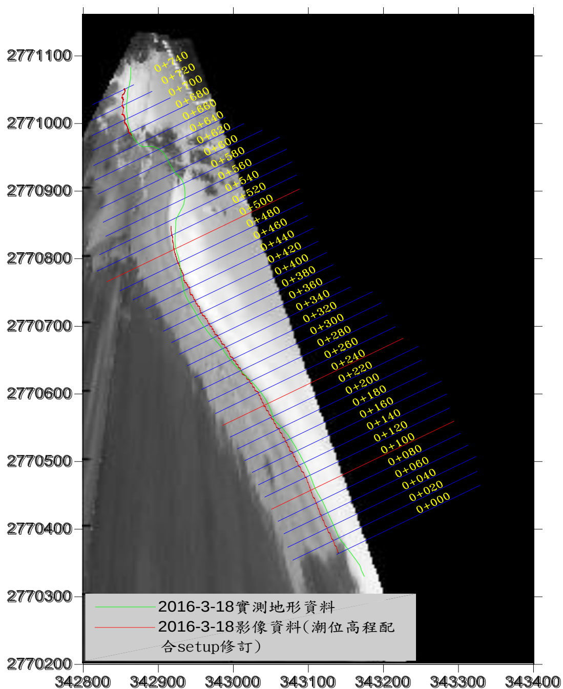
圖 3-22 水位線分析結果圖(2016/3/18)
