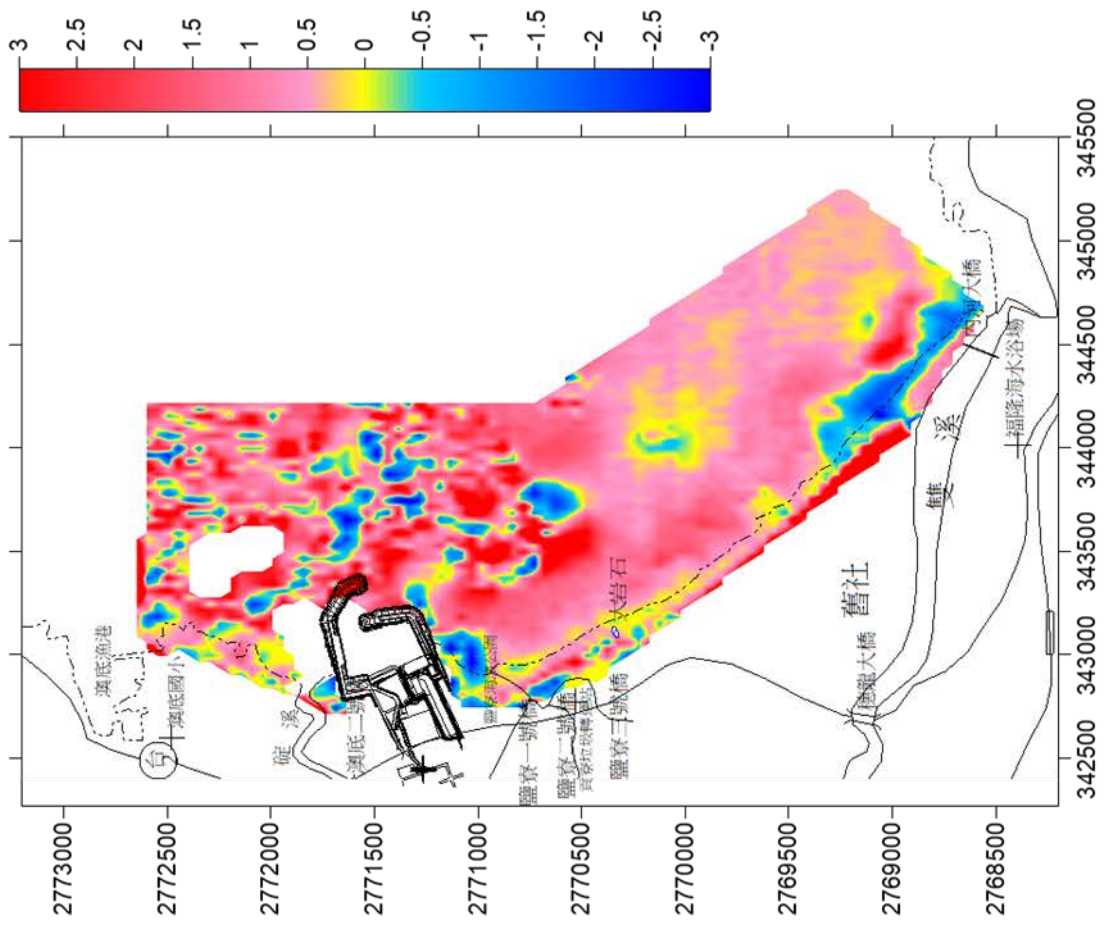
圖 3.1-17 核四環境監測海岸地形 108 年第 2 季與 87 年第 2 季侵淤比較圖
