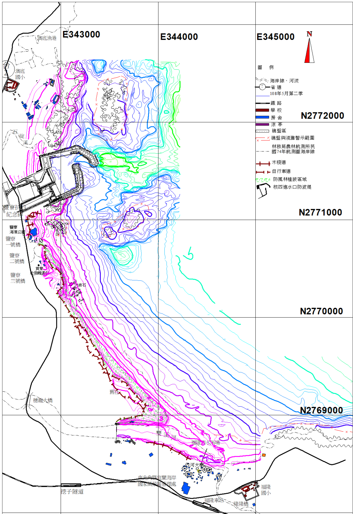
圖 2.5-2 核四封存期間境監測海岸地形 108 年第 2 季 海岸地形監測結果
