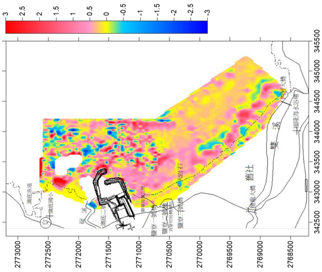
圖3.1-16 核四環境監測海岸地形108年第2季與107年第2季侵淤比較圖
