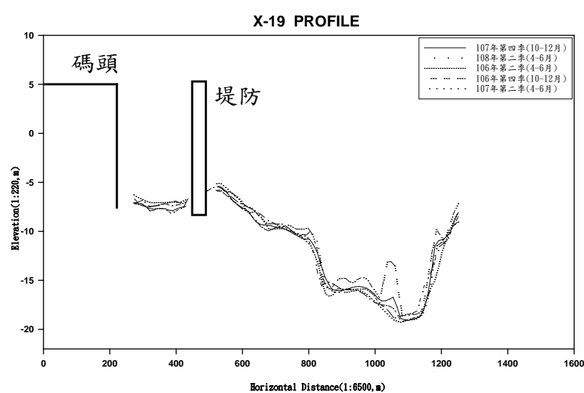
附錄IV.5-3 106年第二季、106年第四季、107年第二季、107年第四季、108年第二季海域監測剖面比較圖(續2)
