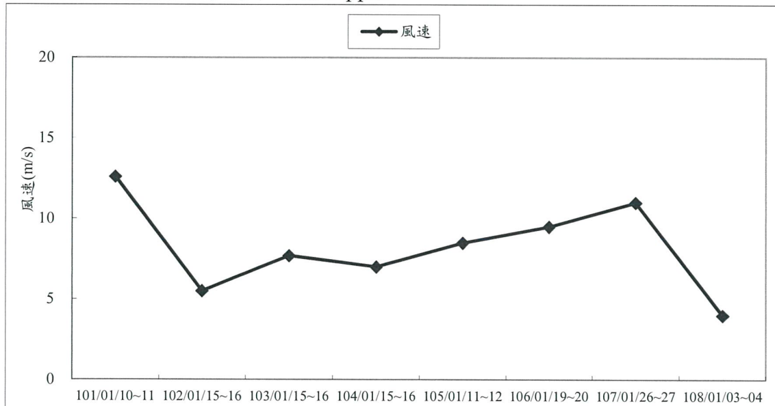
圖 3.1-1 歷年同期風速監測成果彙整
