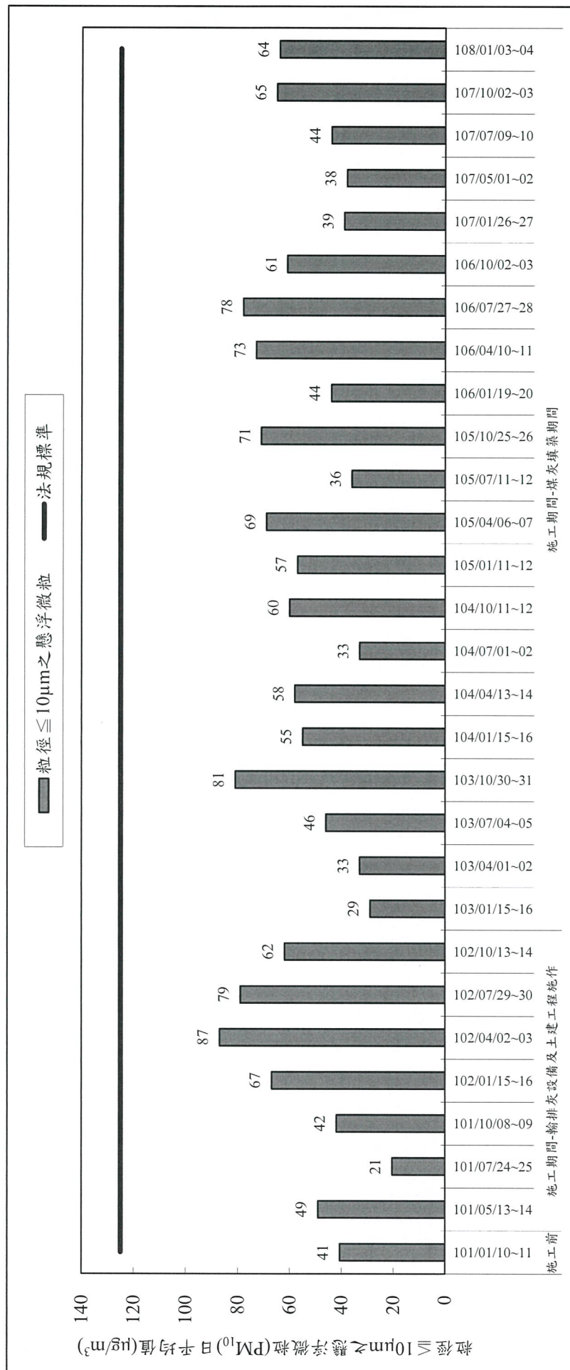
圖 2.1-2 歷季粒徑 \leq 10\mu\text{m} 之懸浮微粒( \text{PM}_{10} )日平均值監測成果彙整
