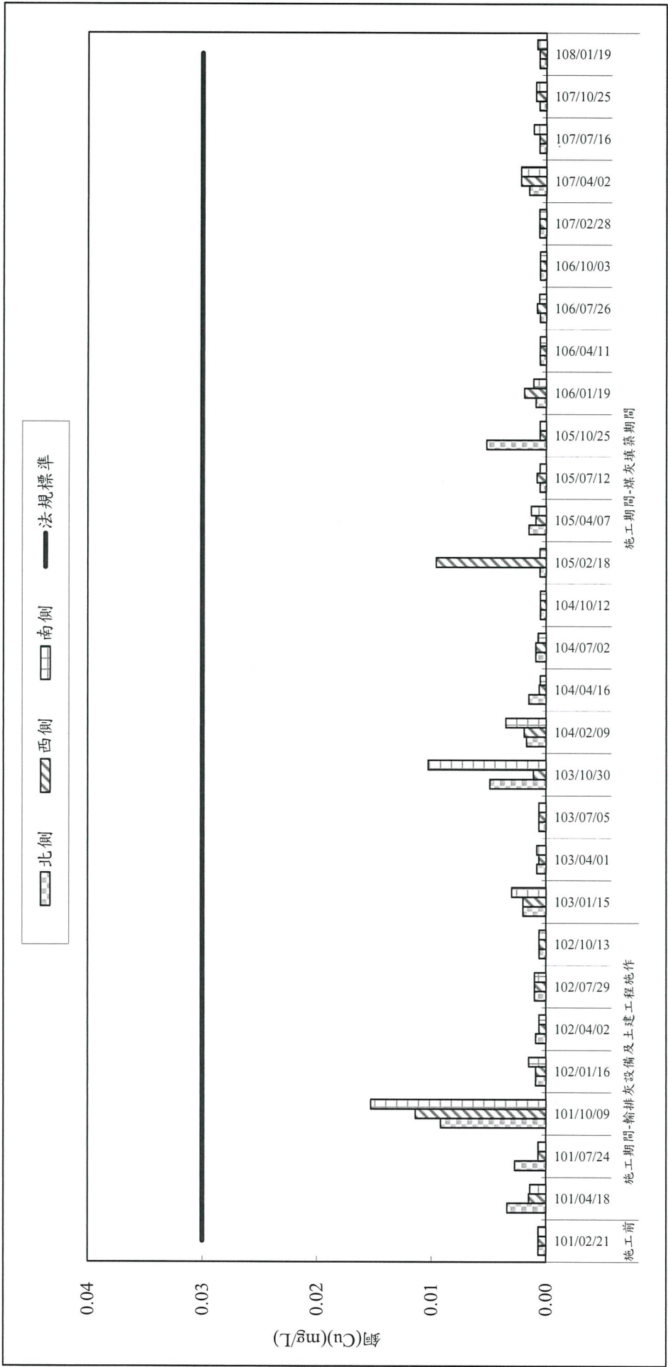
圖 2.2-7 歷季各測站銅(Cu)監測成果彙整
