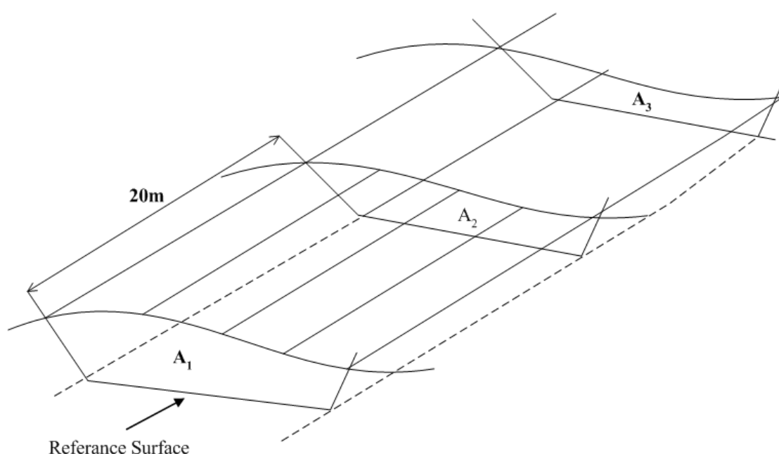
圖 3-3 土方計算原理示意圖
