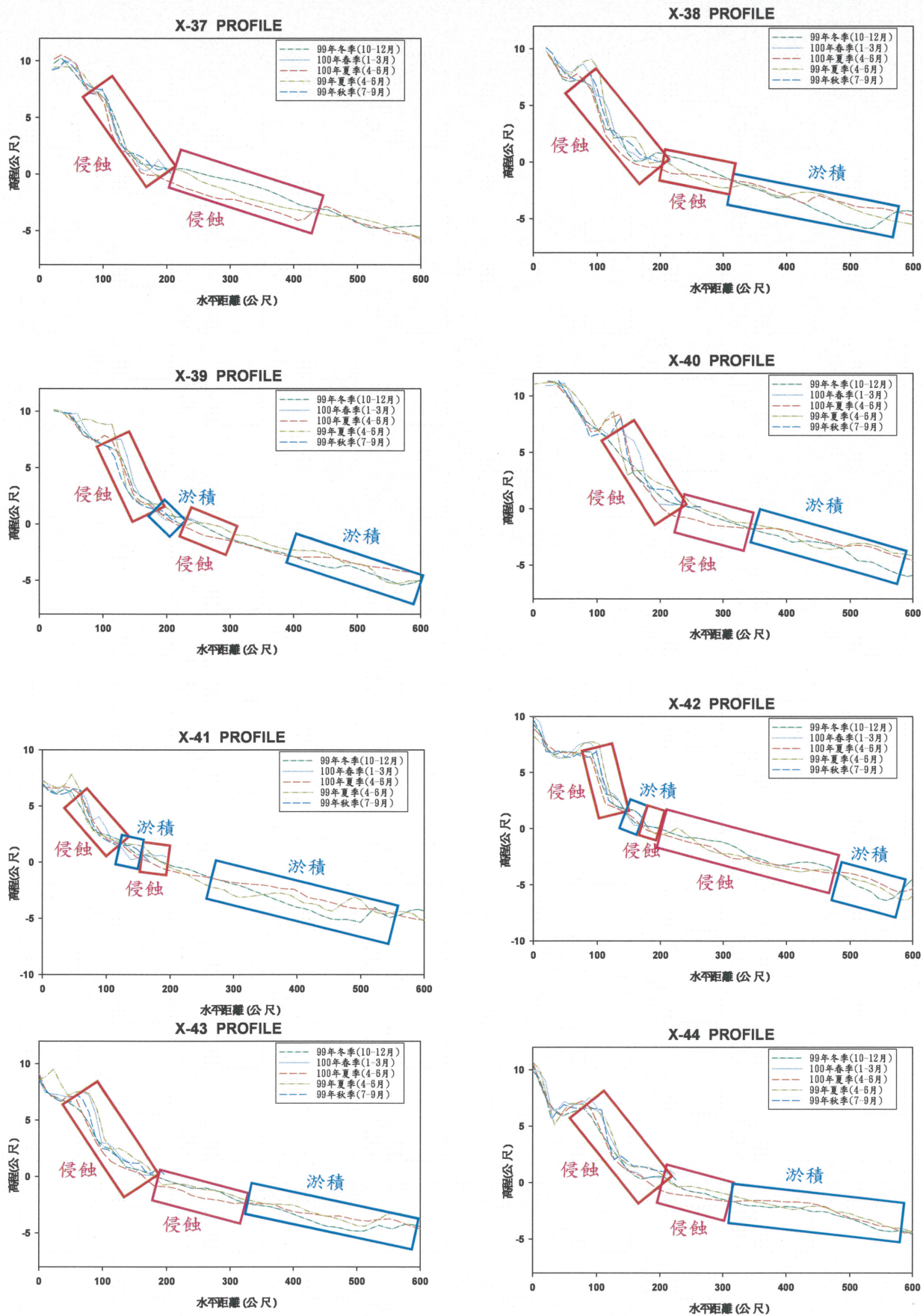
圖 3.1-56 核四附近海岸地形監測各剖面水深變化比較 (續2)
