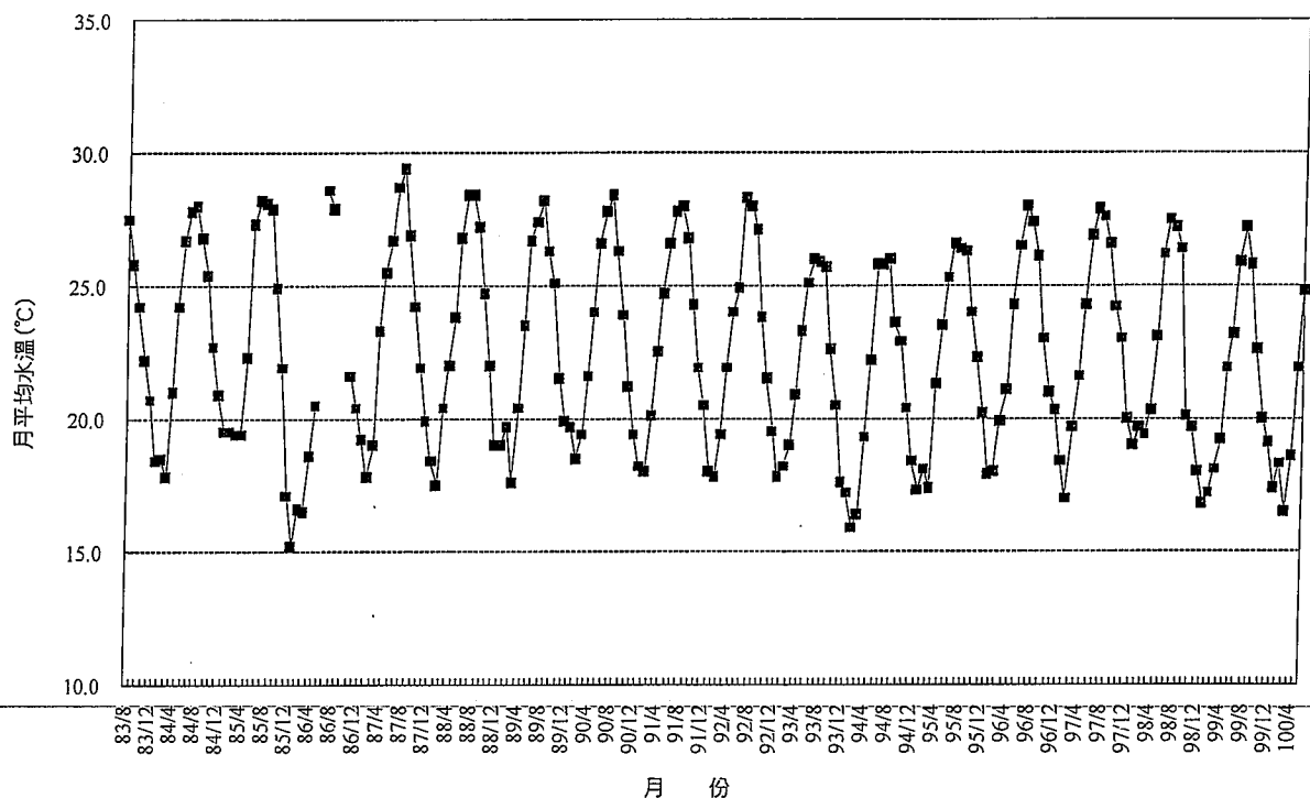
圖 2.13-4 核四施工環境監測海象調查沿岸水溫月平均變化圖 調查日期：83 年 8 月至 100 年 6 月
