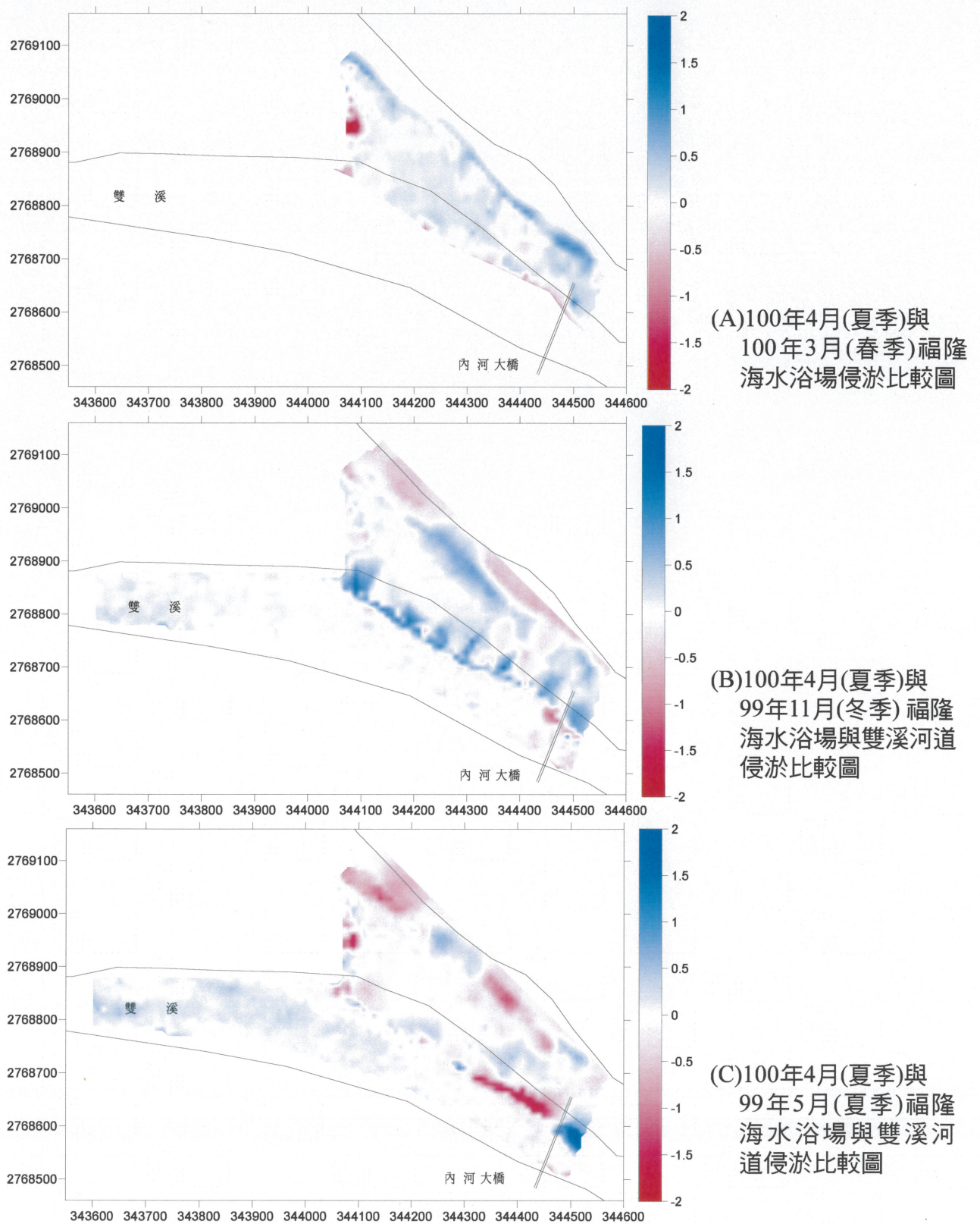
圖 3.1-53 福隆海水浴場與雙溪河道侵淤比較圖
