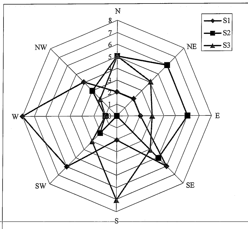
圖 3.1-42 各測站最大淨輸砂方向歷年累計次數雷達圖
