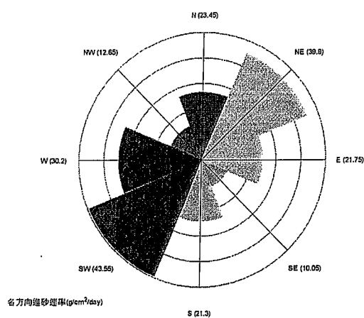
S4測站各方向進砂速率雷達圖 S4測站各方向淨進砂速率雷達圖
