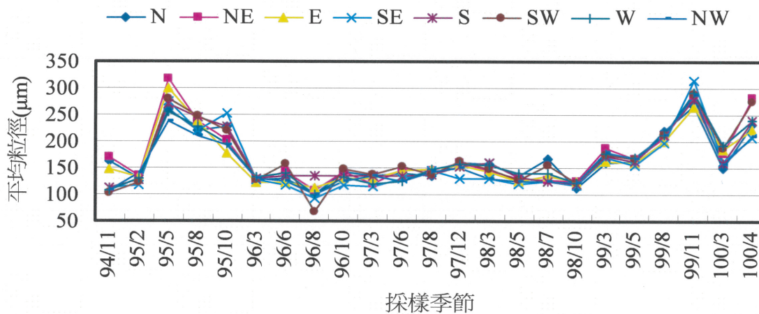
圖3.1-37 漂砂測站各方向歷次採樣平均粒徑比較圖
