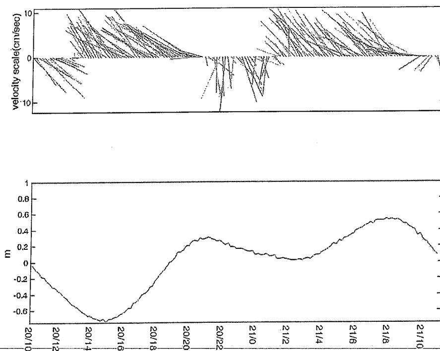
圖2.15-3 本季（100年第2季）流速流向棍棒圖及潮汐水位變化圖
