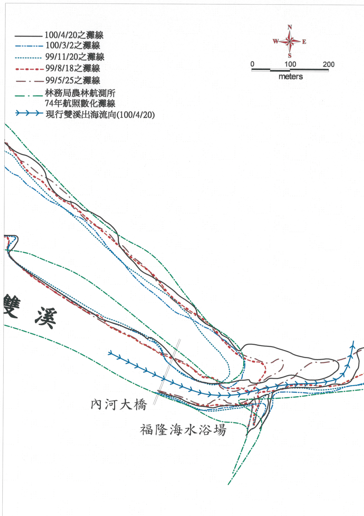
圖 3.1-55 福隆海水浴場附近灘線變化及出海流向比較示意圖
