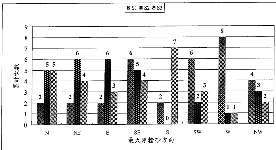
圖 3.1-41 各測站最大淨輸砂方向歷年累計次數比較圖
