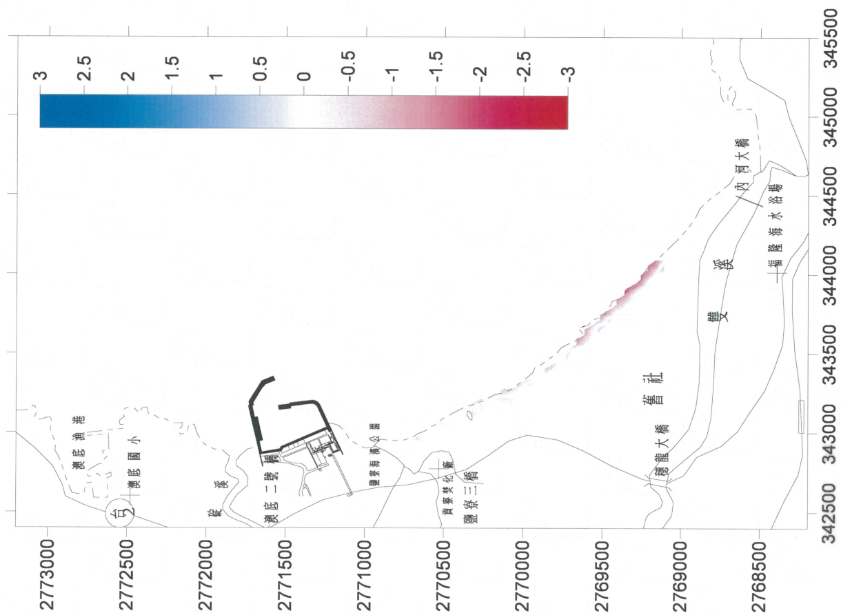
圖 3.1-49 100年4月(夏季)與100年3月(春季)鹽 寮侵淤比較圖
