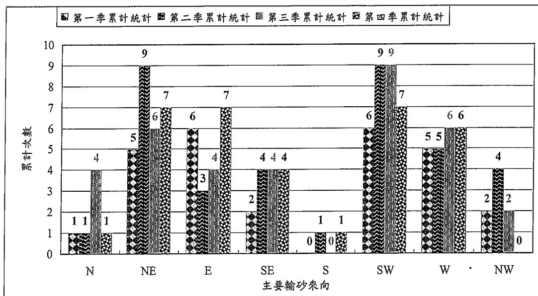
圖 3.1-43 歷年主要輸砂來向分季累計次數比較圖
