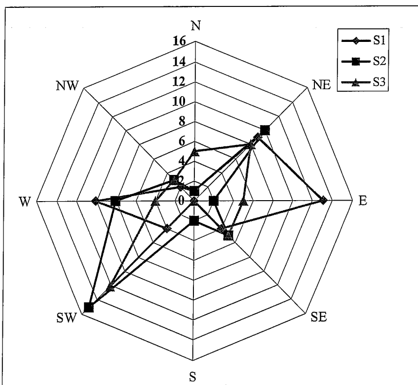
圖 3.1-40 各測站主要輸砂來向歷年累計次數雷達圖
