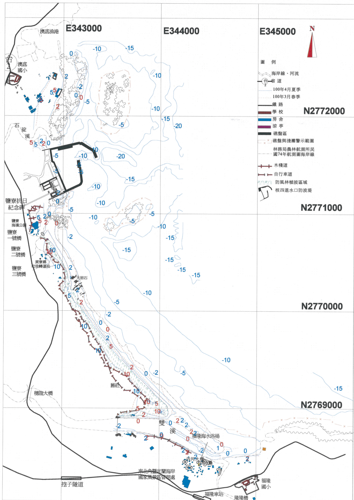
圖 2.16-5 核四施工環境監測海岸地形 100 年 4 月（夏季）與 100 年 3 月（春季）監測結果比較
