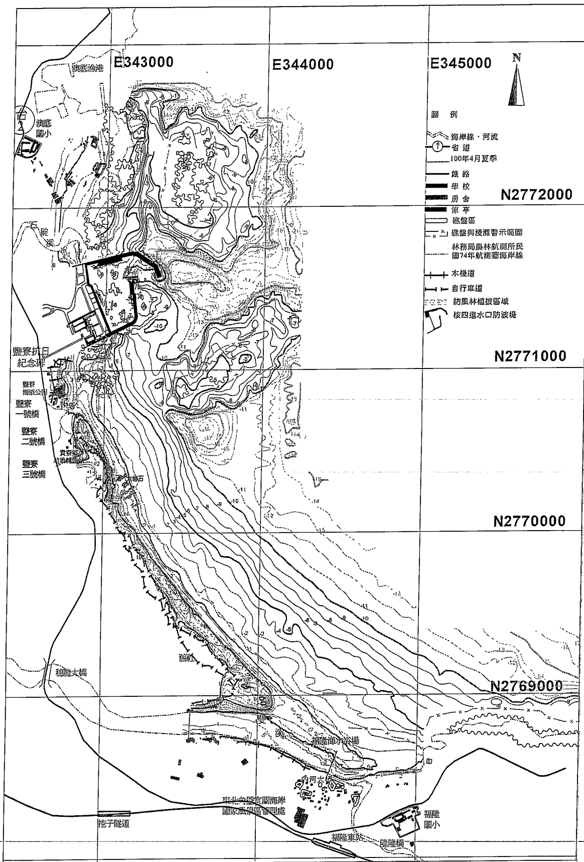
圖 2.16-2 核四施工環境監測海岸地形 100 年 4 月(夏季) 海岸地形監測結果
