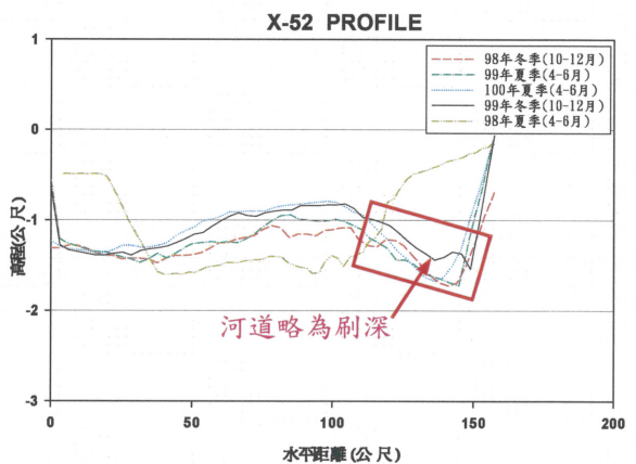
圖 3.1-56 核四附近海岸地形監測各剖面水深變化比較 (續3)
