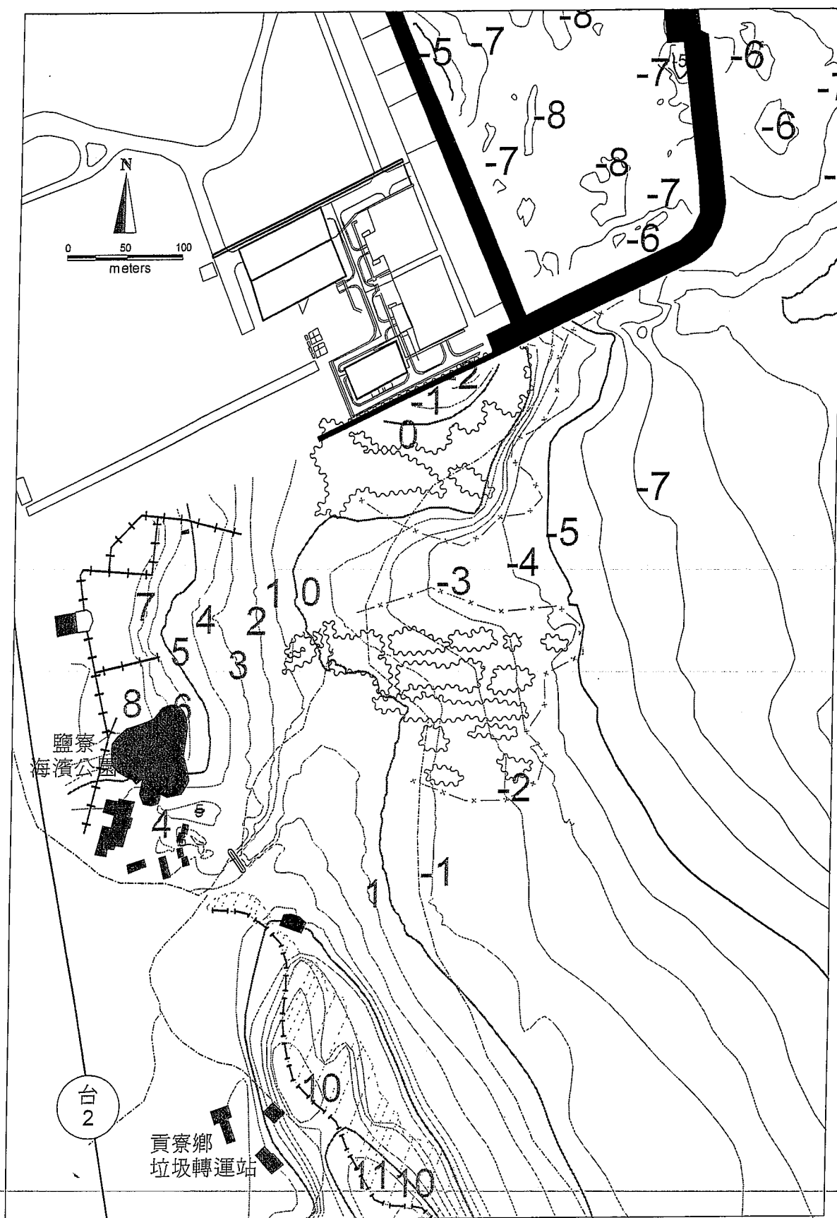
圖 2.16-3 鹽寮公園附近 100 年 4 月（夏季）海岸地形 監測結果
