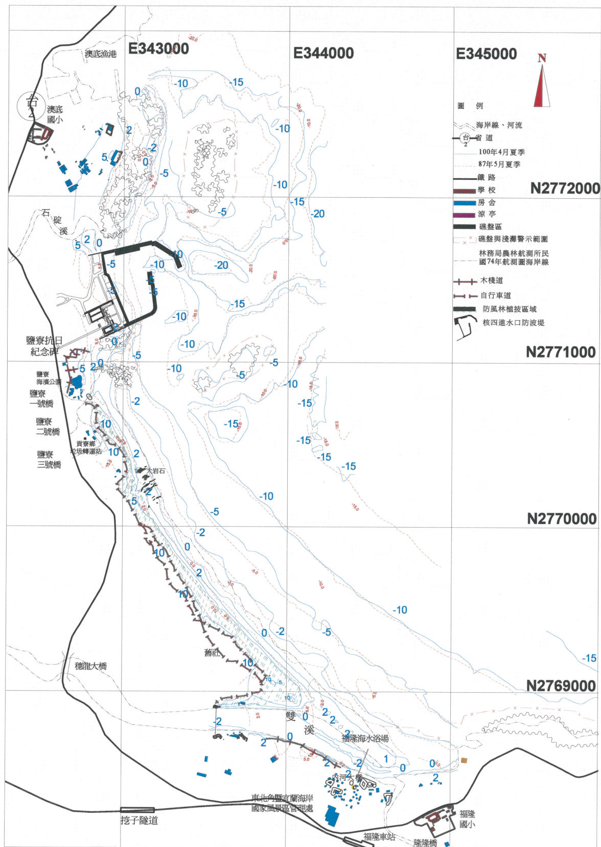
圖 3.1-48 核四施工環境監測海岸地形 100 年 4 月（夏季）與 87 年 5 月（夏季）監測結果比較（海事工程施工前）
