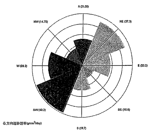
S5測站各方向進砂速率雷達圖 S5 測站各方向淨進砂速率雷達圖
