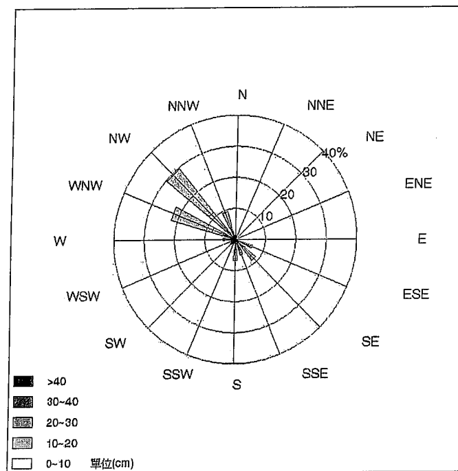
圖2.15-2 本季（100年第2季）海流儀實測流速流向玫瑰圖
