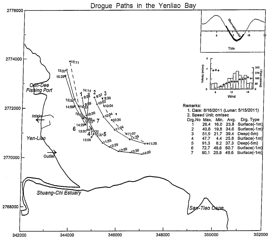
圖 2.13-3 核四施工環境監測海象調查 100 年 6 月 16 日漂流浮標追蹤軌跡圖
