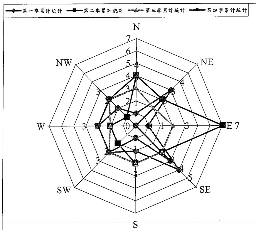
圖 3.1-46 歷年最大淨輸砂方向分季累計次數雷達圖
