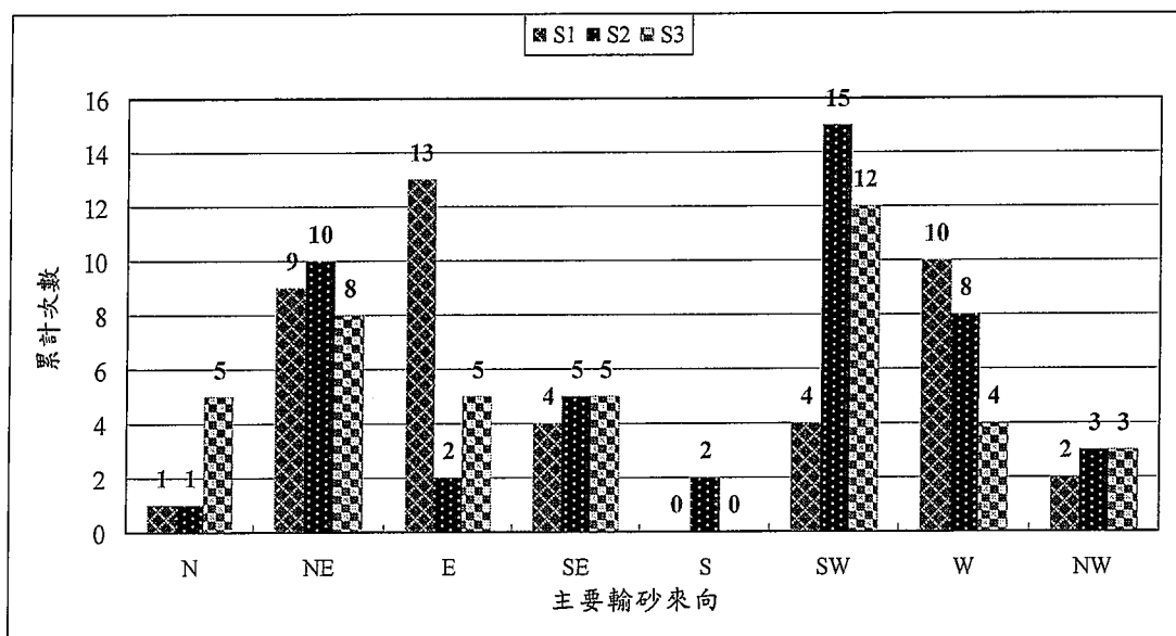
圖 3.1-39 各測站主要輸砂來向歷年累計次數比較圖
