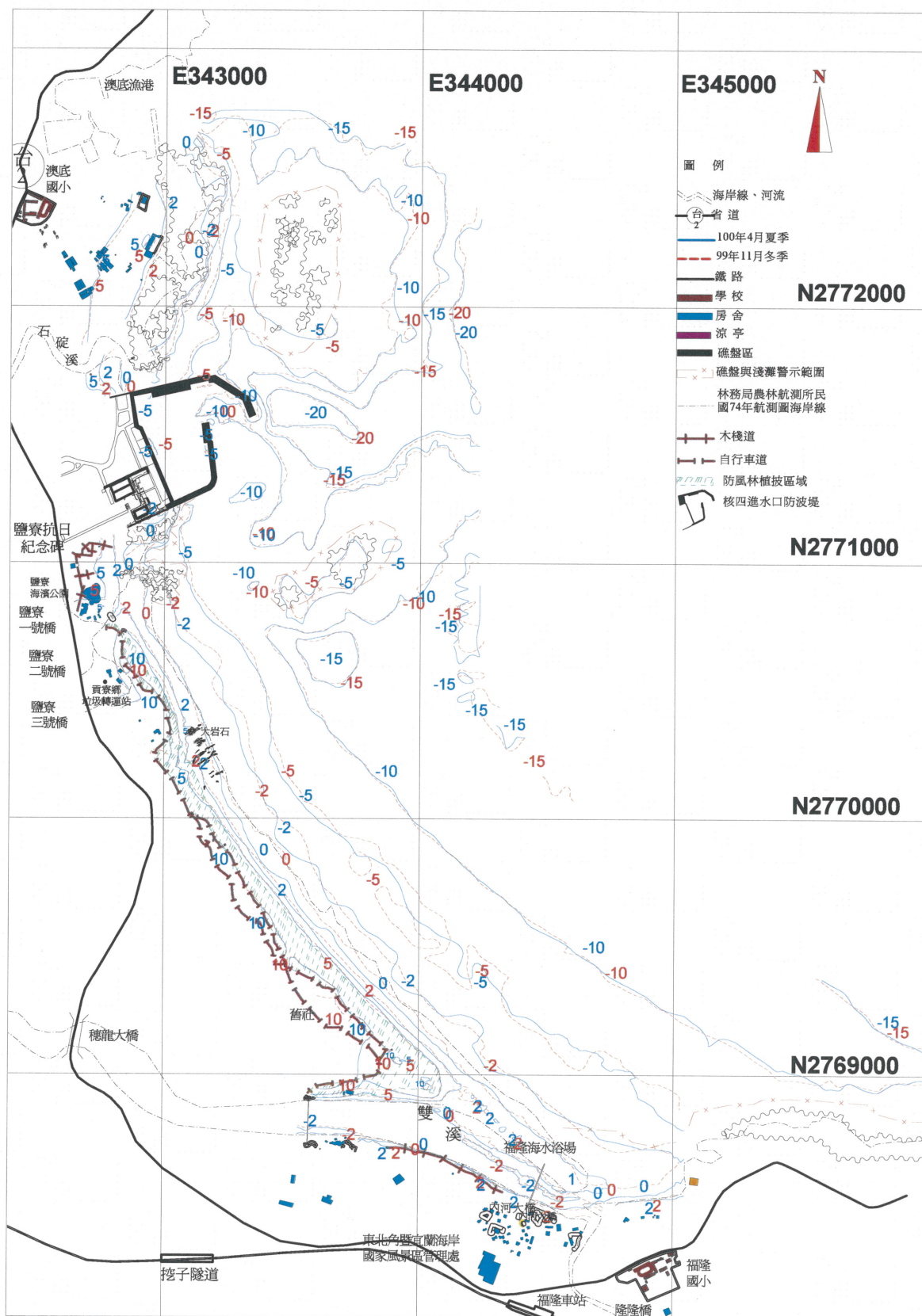
圖 2.16-7 核四施工環境監測海岸地形 100 年 4 月（夏季）與 99 年 11 月（冬季）監測結果比較
