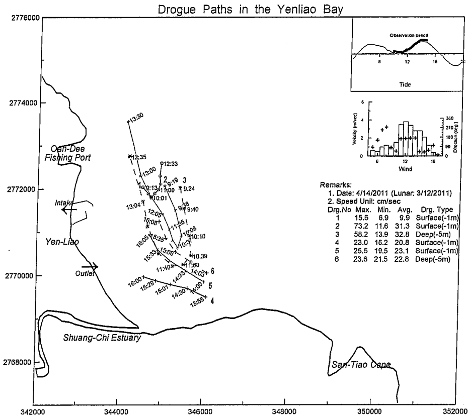
圖 2.13-1 核四施工環境監測海象調查 100 年 4 月 14 日漂流浮標追蹤軌跡圖
