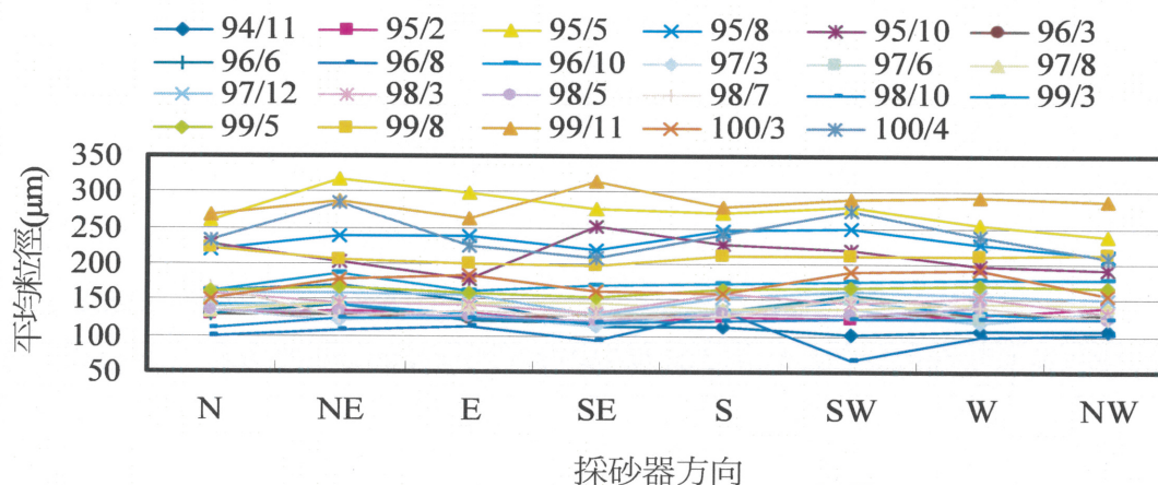
圖3.1-38 漂砂測站各方向各採樣期平均粒徑比較圖
