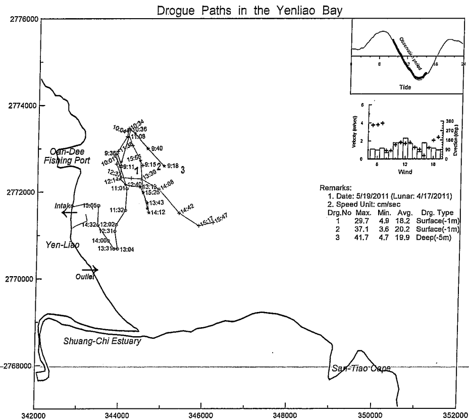
圖 2.13-2 核四施工環境監測海象調查 100 年 5 月 19 日漂流浮標追蹤軌跡圖
