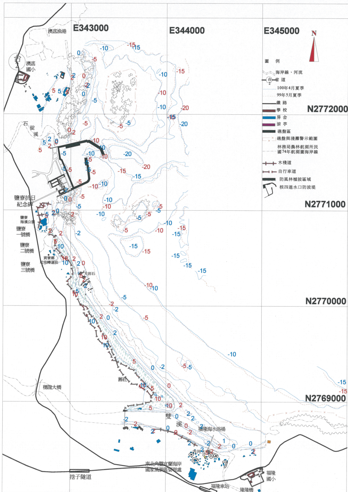
圖 3.1-47 核四施工環境監測海岸地形 100 年 4 月（夏季）與 99 年 5 月（夏季）監測結果比較
