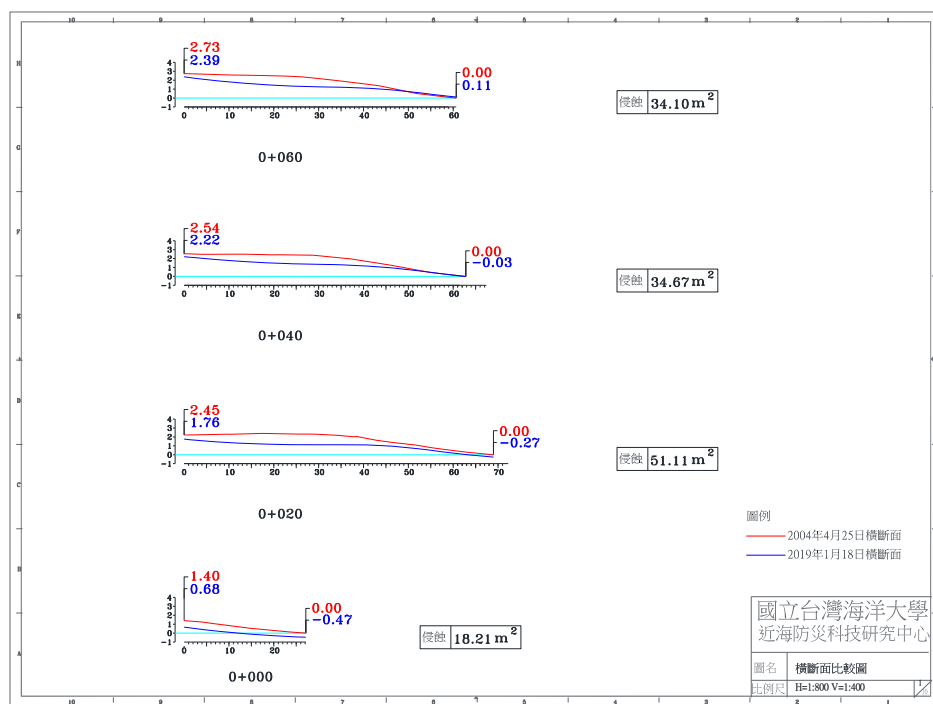
圖 4-4(j) 2018 年 12 月 7 日 A 監測區橫斷面比較圖
