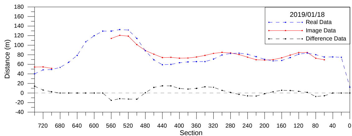
圖 3-23 海岸線分析比較圖(2018/12/4)
