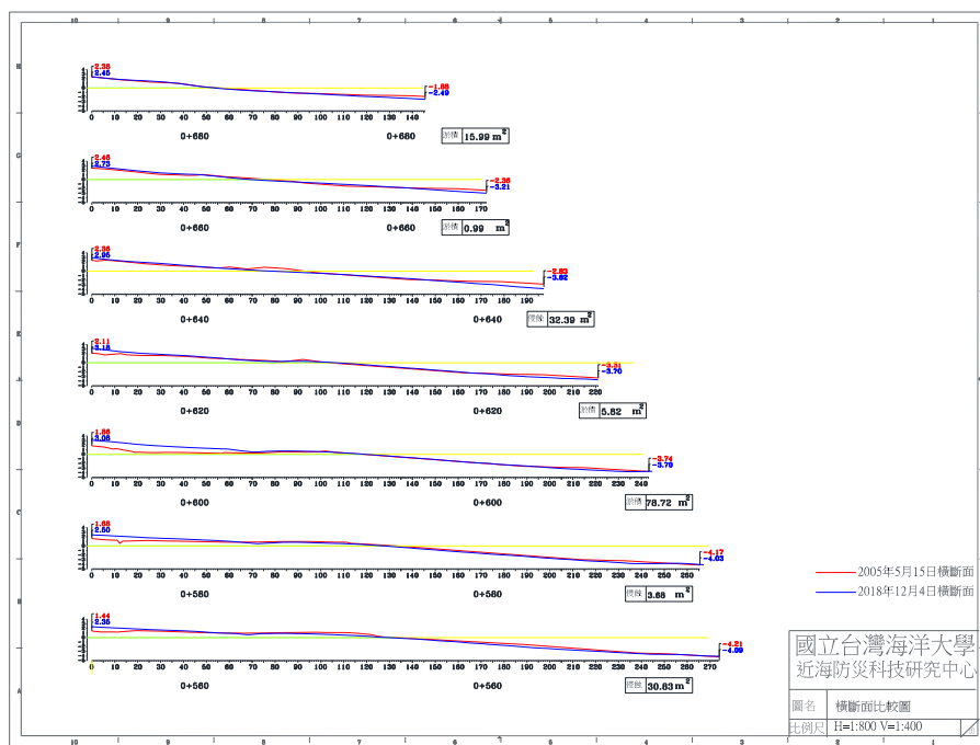
圖 4-5(b) 2018 年 12 月 7 日 B 監測區橫斷面比較圖
