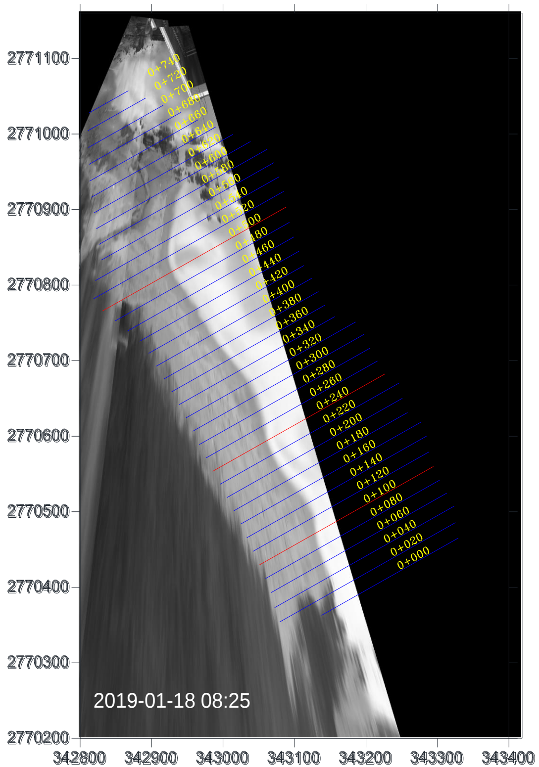
圖 4-19 鹽寮海岸地形影像全景圖(2019/1/18 08:25)
