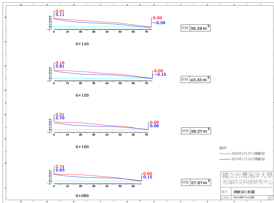
圖 4-4(i) 2018 年 12 月 7 日 A 監測區橫斷面比較圖
