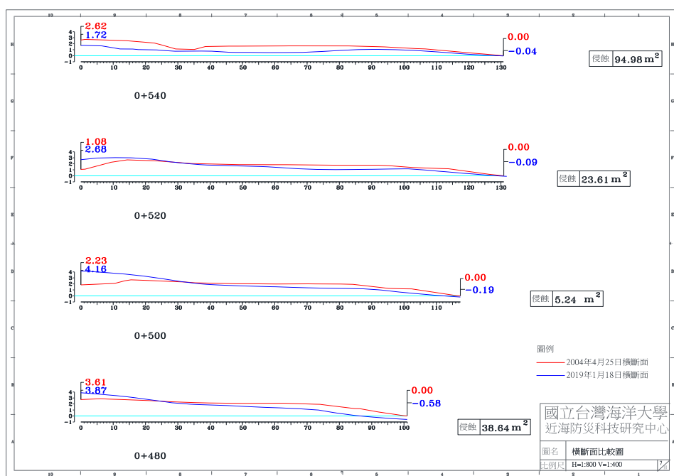
圖 4-4(d) 2018 年 12 月 7 日 A 監測區橫斷面比較圖
