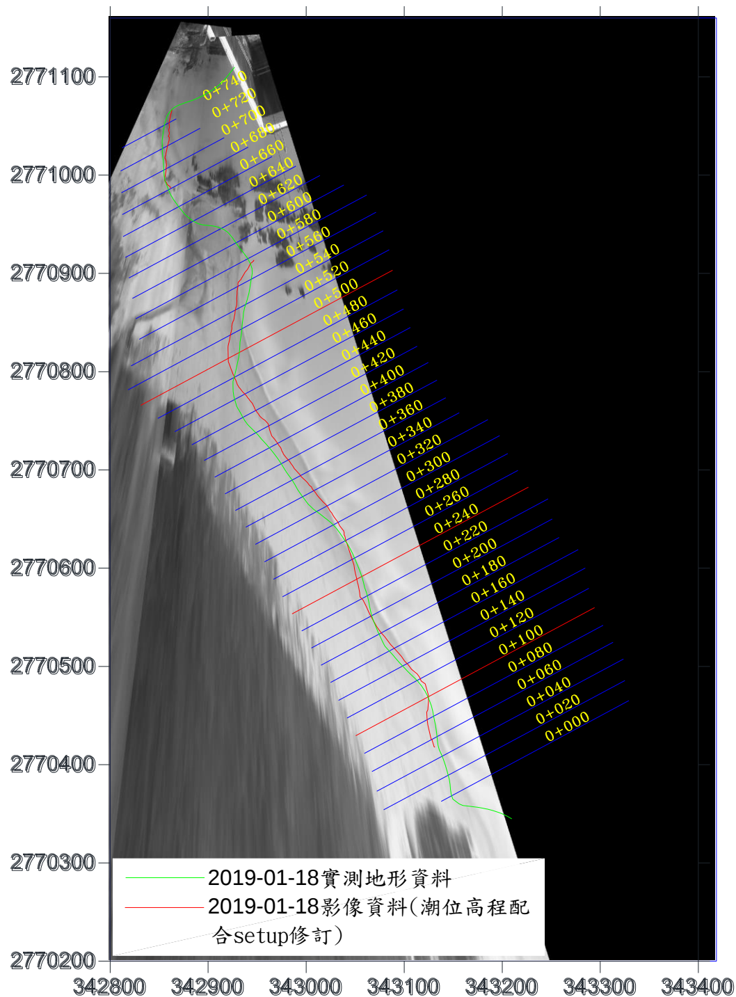
圖 3-22 水位線分析結果圖(2019/01/18)
