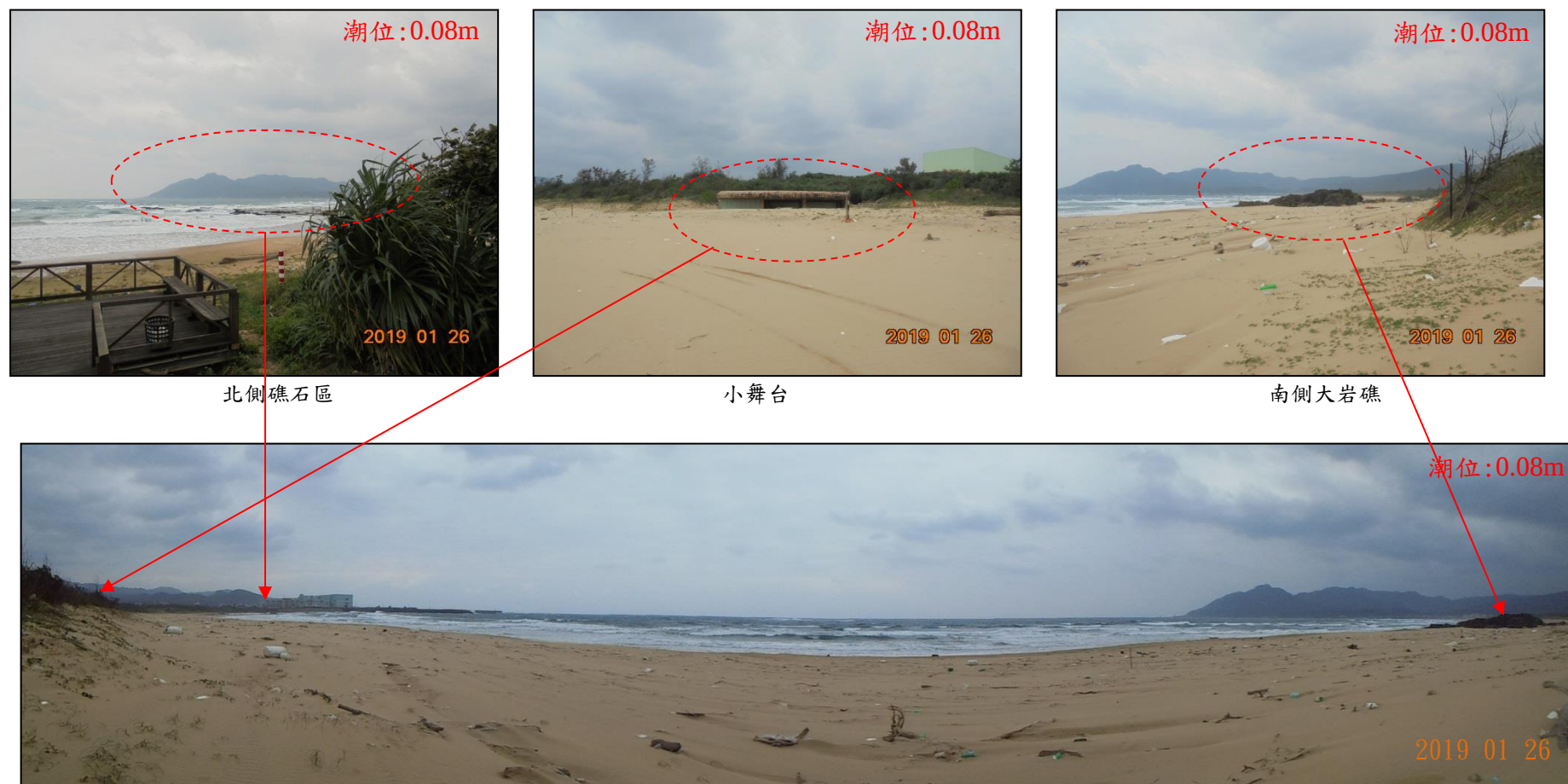
圖 3-6 鹽寮海岸短期性養灘區地形地貌圖 (2019/01/26)
