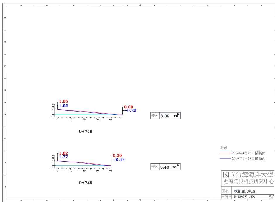
圖 4-4(a) 2018 年 12 月 7 日 A 監測區橫斷面比較圖
