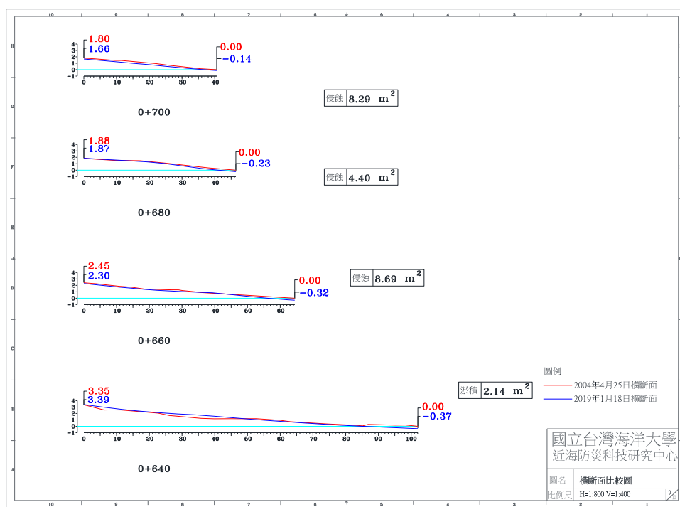
圖 4-4(b) 2018 年 12 月 7 日 A 監測區橫斷面比較圖
