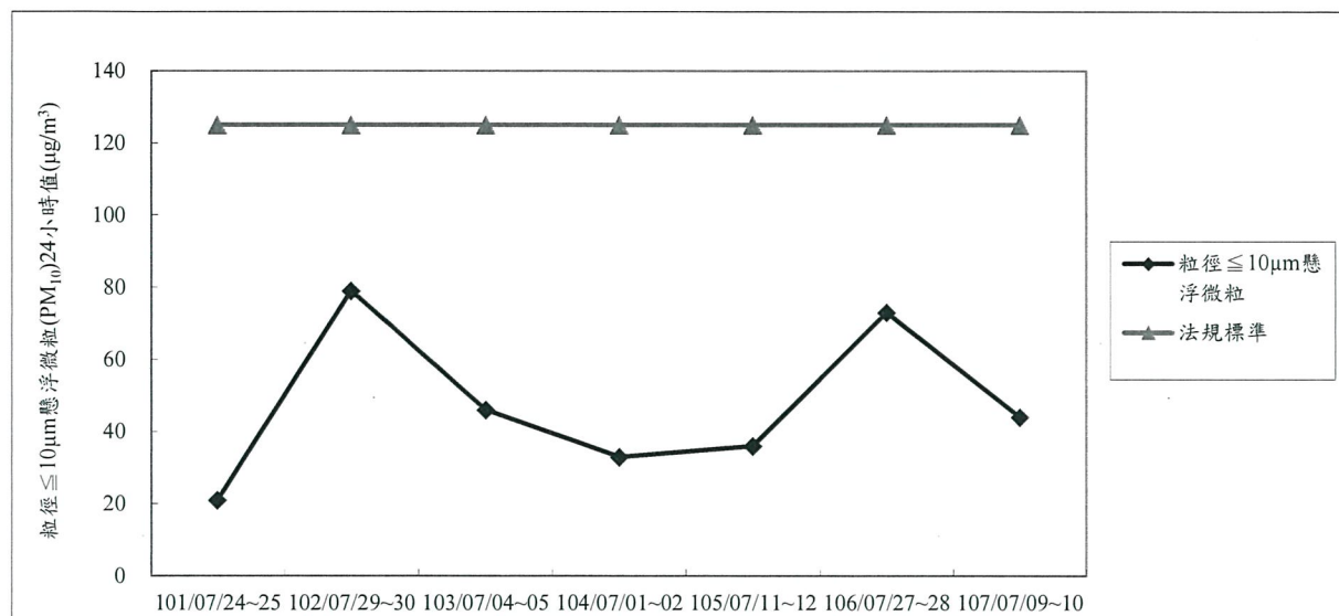
圖 3.1-3 歷年同期粒徑≤10μm 之懸浮微粒(PM 10 )日平均值監測成果彙整
