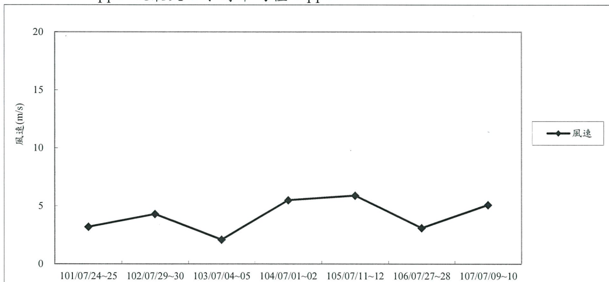
圖 3.1-1 歷年同期風速監測成果彙整
