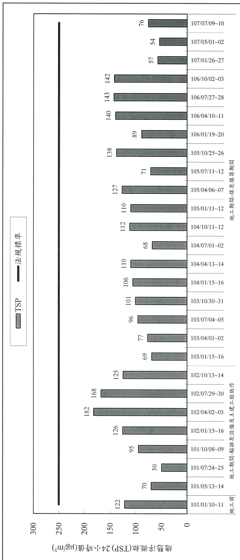
圖 2.1-1 歷季總懸浮微粒(TSP)24 小時值監測成果彙整
