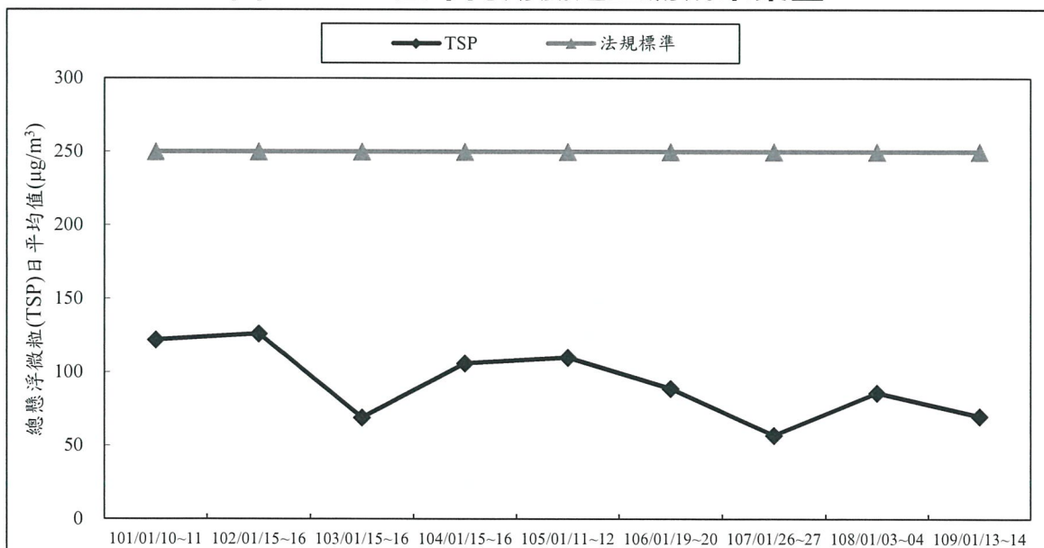
圖 3.1-2 歷年同期總懸浮微粒(TSP)24 小時值監測成果彙整
