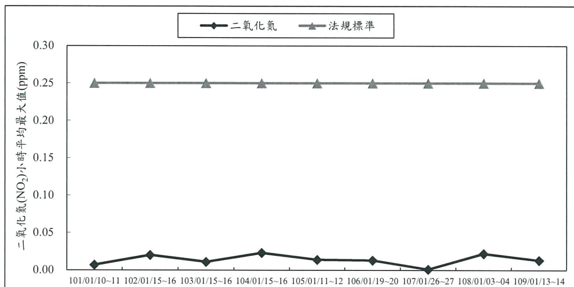
圖 3.1-4 歷年同期二氧化氮( \text{NO}_2 )小時平均最大值監測成果彙整
