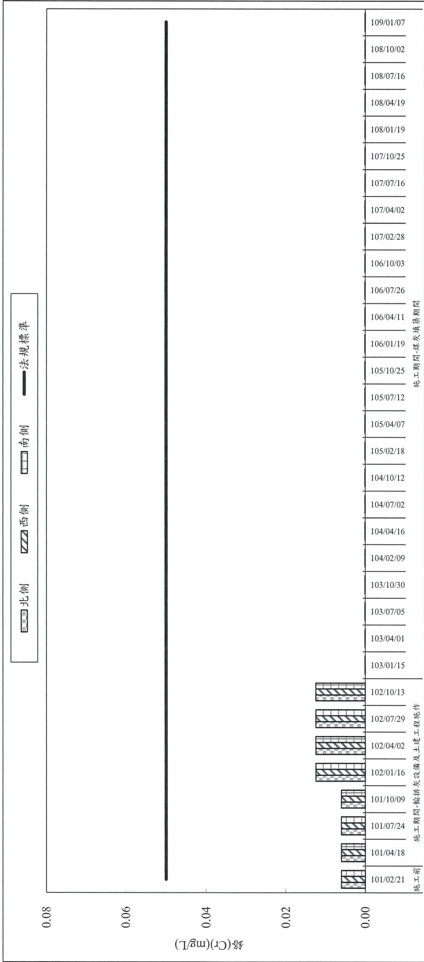
圖 2.2-12 歷季各測站鉻(Cr)監測成果彙整
