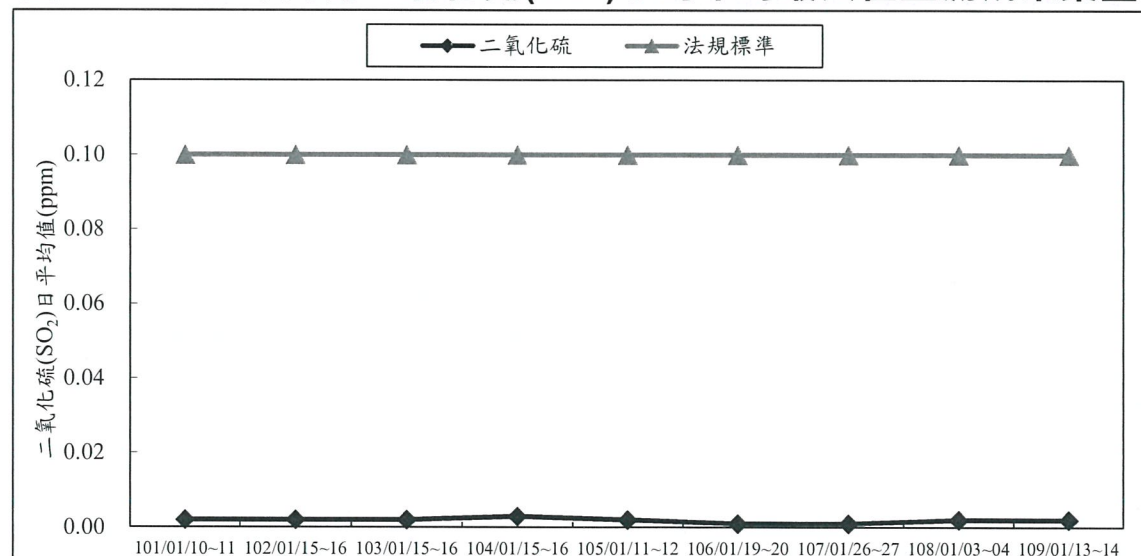
圖 3.1-5 歷年同期二氧化硫( \text{SO}_2 )日平均值監測成果彙整
