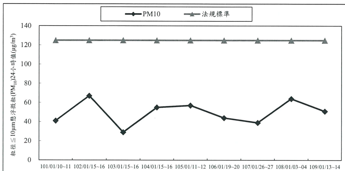
圖 3.1-3 歷年同期粒徑 \leq 10\mu\text{m} 之懸浮微粒( \text{PM}_{10} )日平均值監測成果彙整
