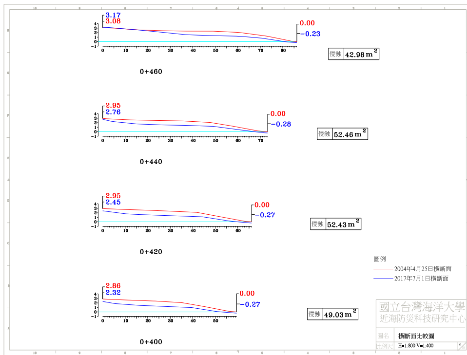
圖 4-4(e) 2017 年 7 月 1 日 A 監測區橫斷面比較圖
