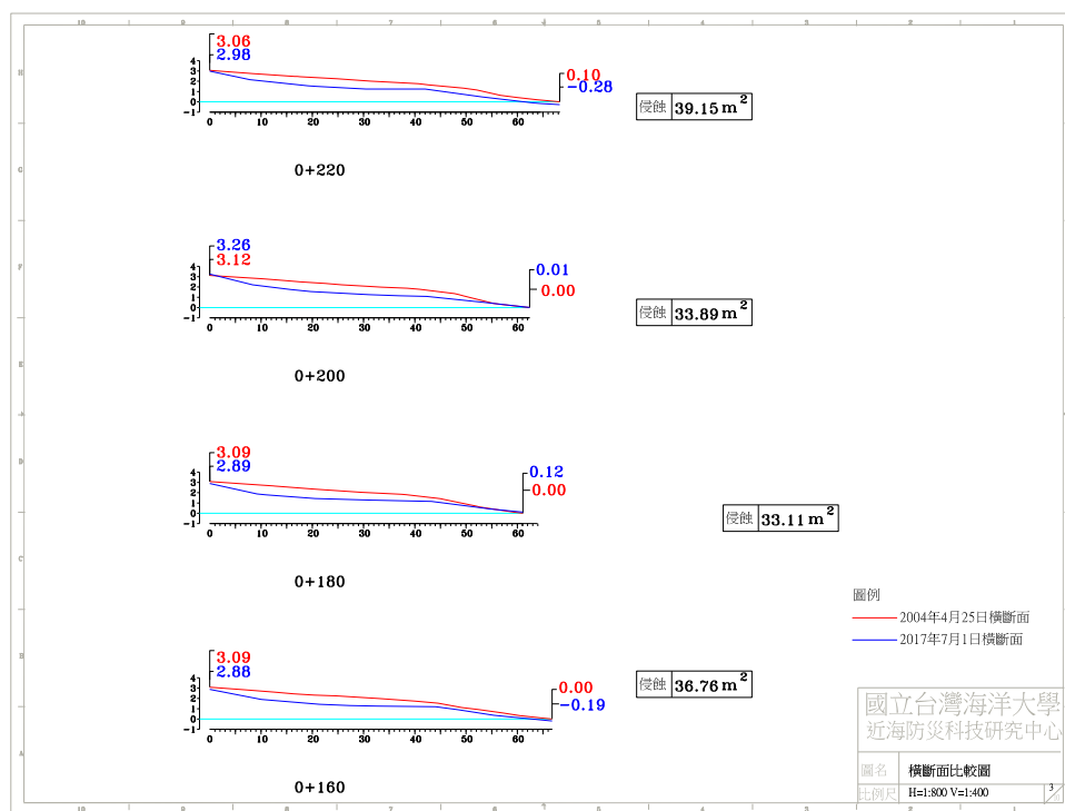
圖 4-4(h) 2017 年 7 月 1 日 A 監測區橫斷面比較圖
