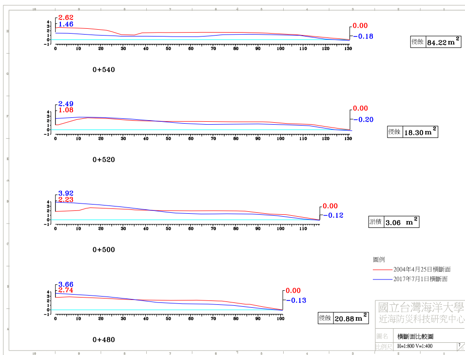
圖 4-4(d) 2017 年 7 月 1 日 A 監測區橫斷面比較圖
