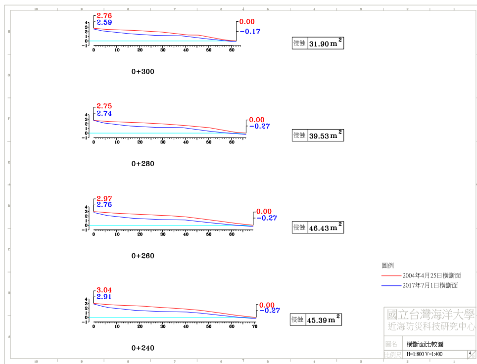
圖 4-4(g) 2017 年 7 月 1 日 A 監測區橫斷面比較圖
