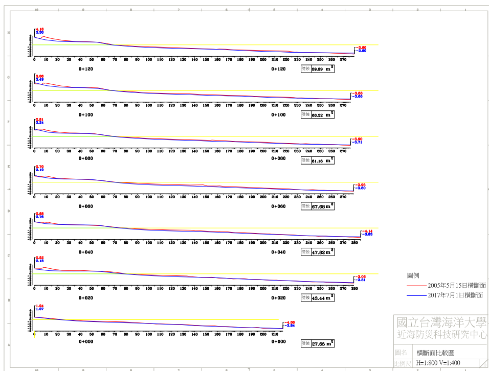
圖 4-5(f) 2017 年 7 月 1 日 B 監測區橫斷面比較圖
