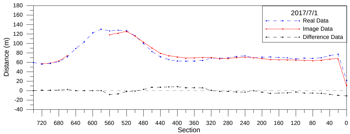
圖 3-23 海岸線分析比較圖(2017/7/1)
