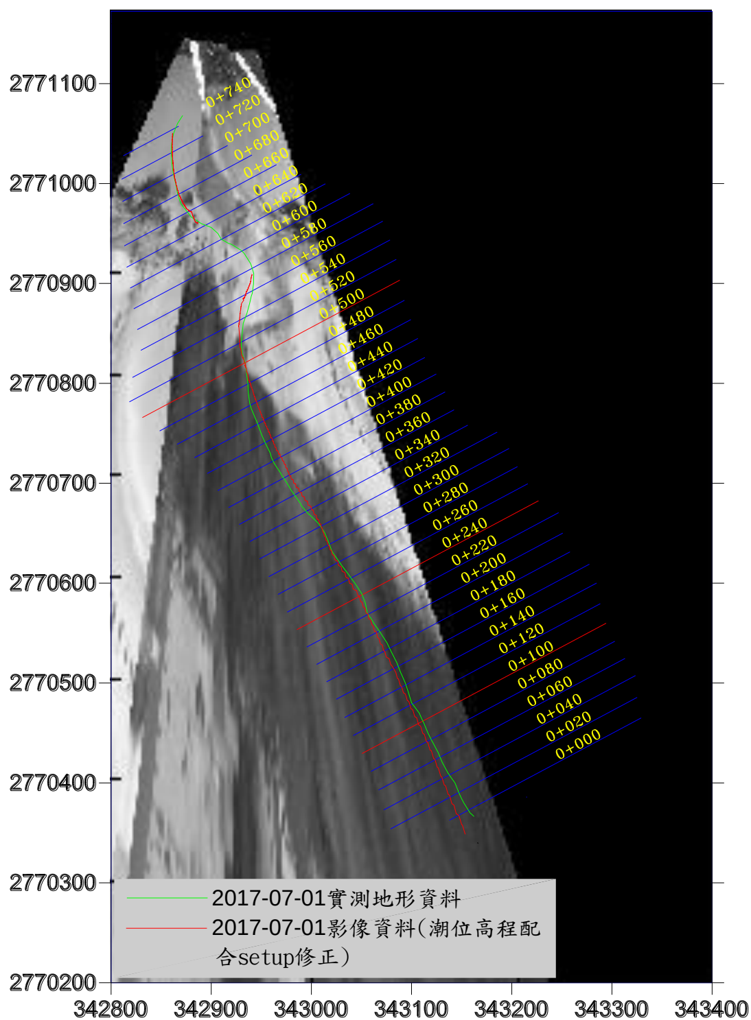
圖 3-22 水位線分析結果圖(2017/7/1)
