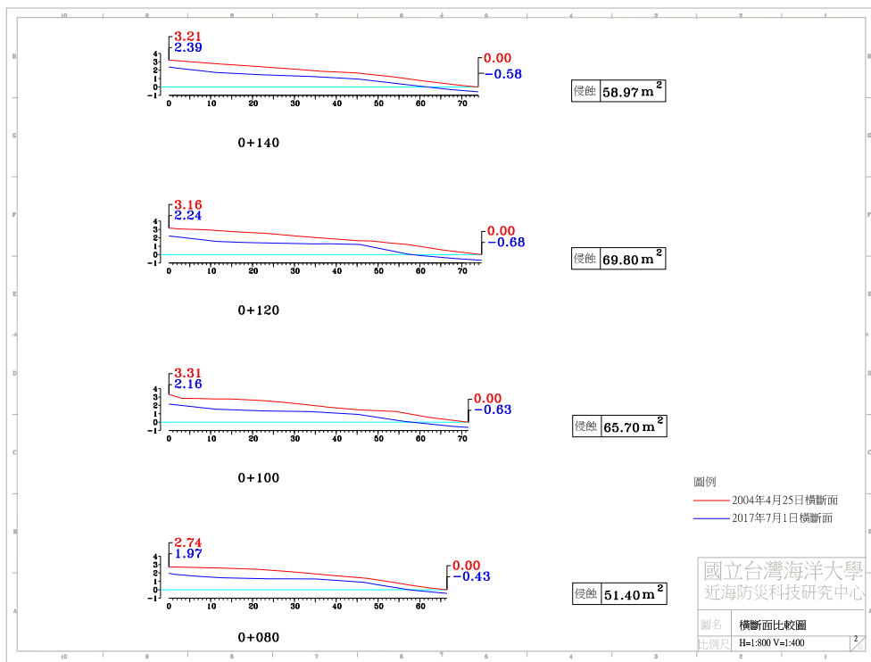
圖 4-4(i) 2017 年 7 月 1 日 A 監測區橫斷面比較圖
