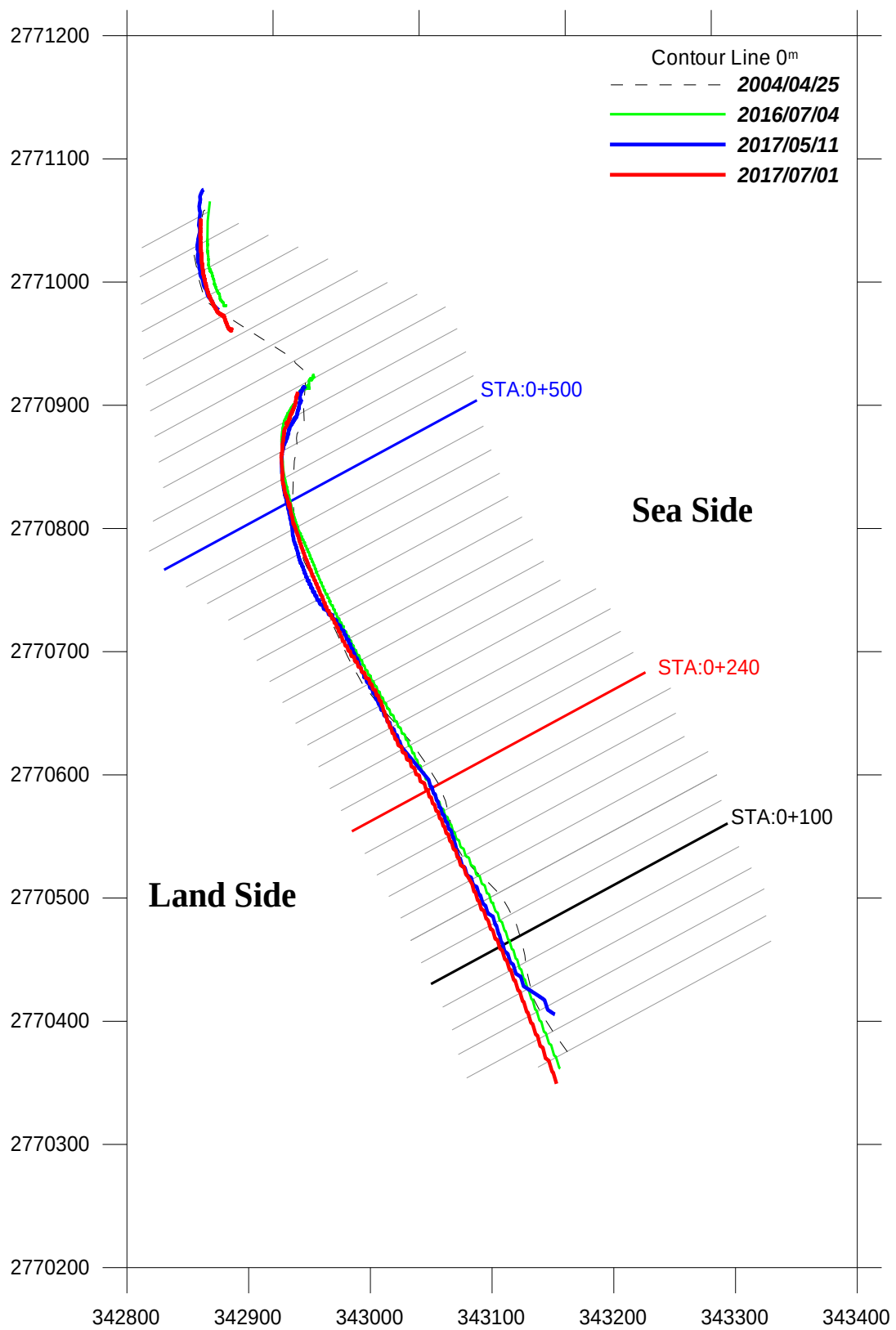
圖 4-20 鹽寮海岸線變遷分析比較圖
