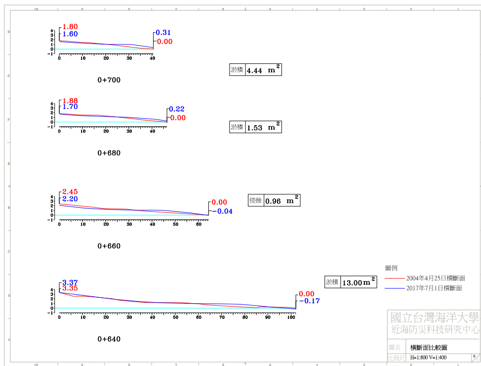
圖 4-4(b) 2017 年 7 月 1 日 A 監測區橫斷面比較圖
