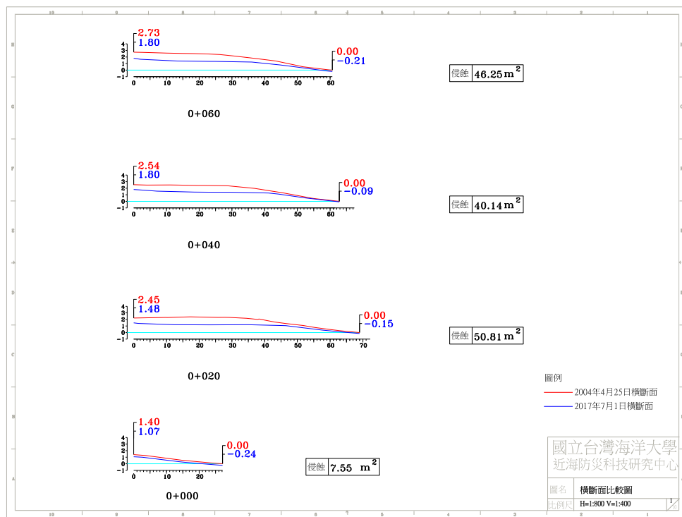
圖 4-4(j) 2017 年 7 月 1 日 A 監測區橫斷面比較圖
