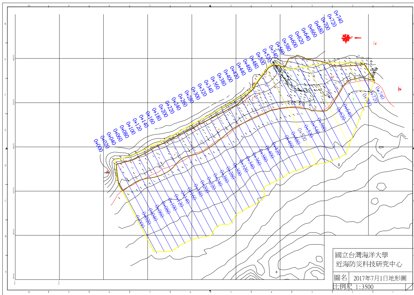
圖 4-1 2017 年 7 月 1 日監測地形圖
