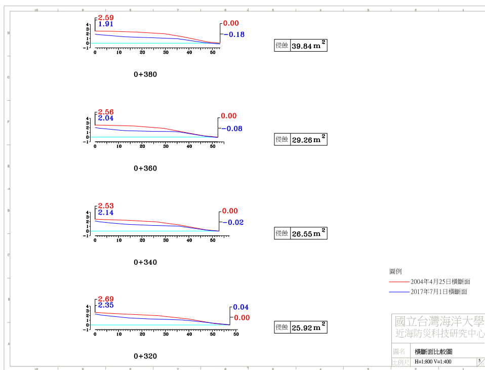
圖 4-4(f) 2017 年 7 月 1 日 A 監測區橫斷面比較圖
