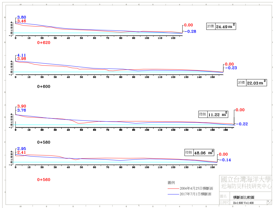
圖 4-4(c) 2017 年 7 月 1 日 A 監測區橫斷面比較圖
