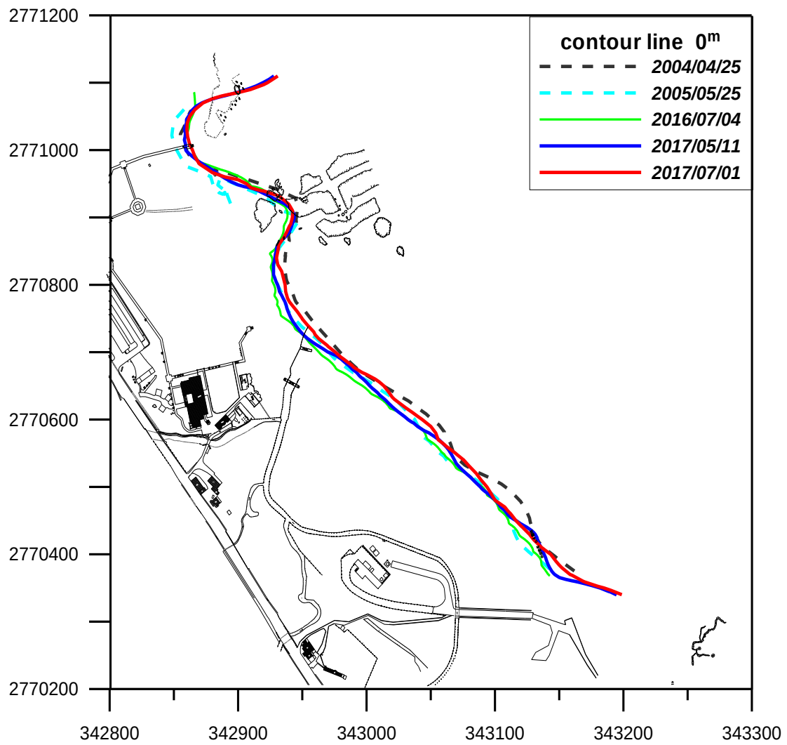
圖 4-2 監測區 0 m 等高線變化比較圖
