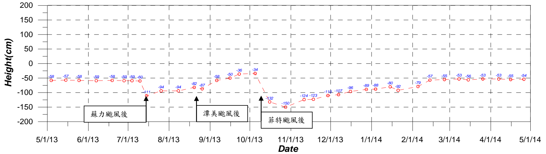
監測區 #04 樁觀測紀錄圖
