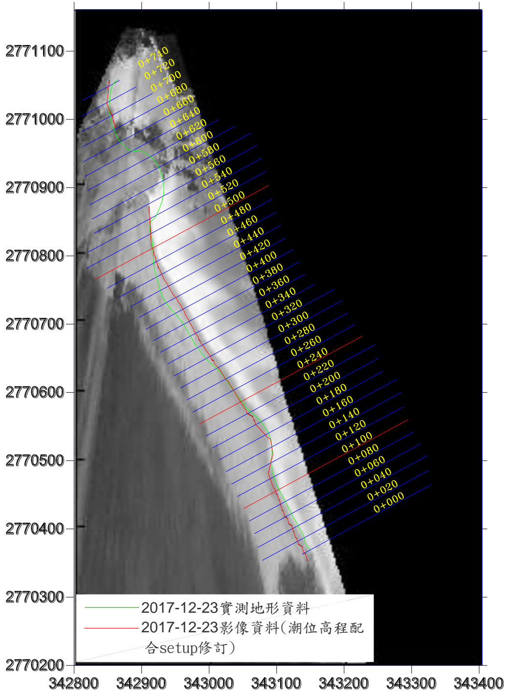
圖 3-22 水位線分析結果圖(2017/12/23)
