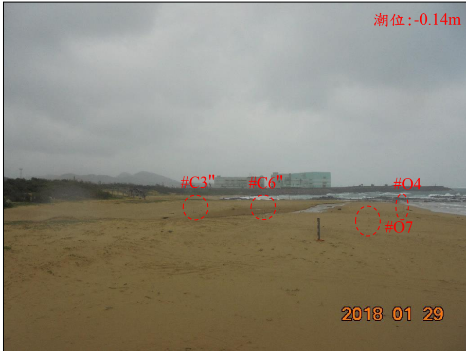
圖 3-8 小舞台前輔助觀測樁位置圖(2018/01/29)
