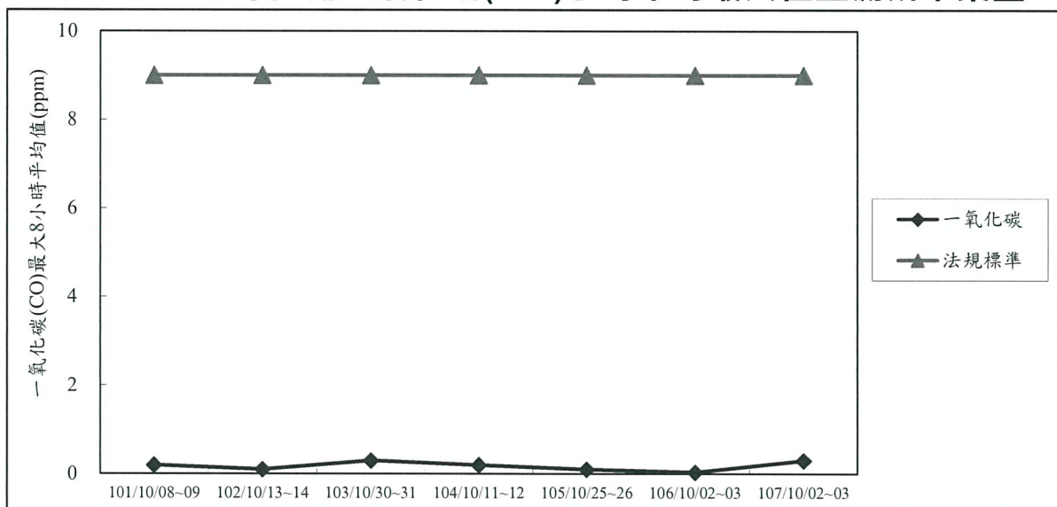
圖 3.1-7 歷年同期一氧化碳(CO)最大 8 小時平均值監測成果彙整
