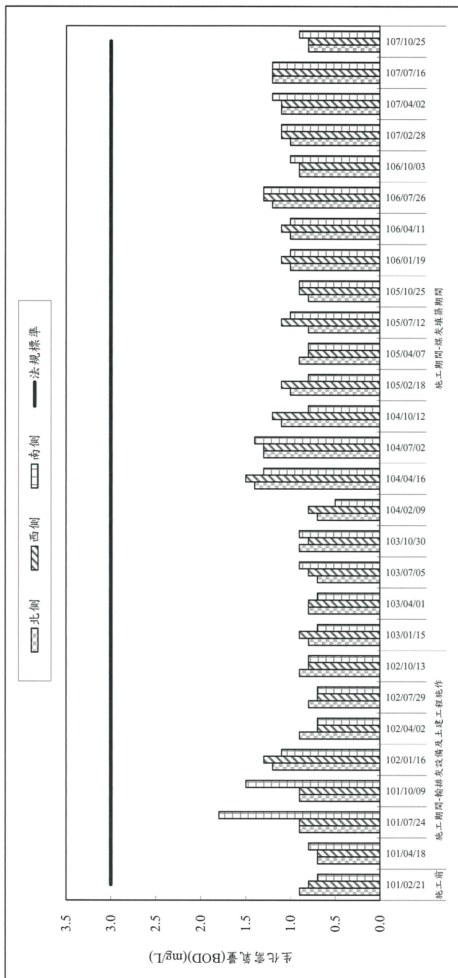
圖 2.2-5 歷季各測站生化需氧量(BOD)監測成果彙整
