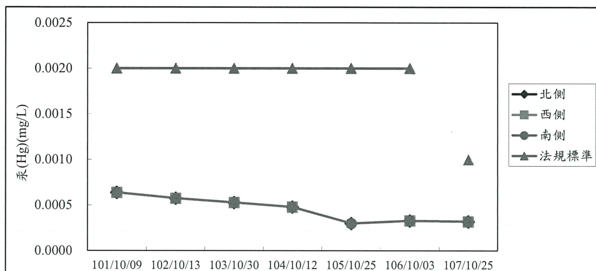
圖 3.1-21 歷年同期各測站汞(Hg)監測成果彙整
