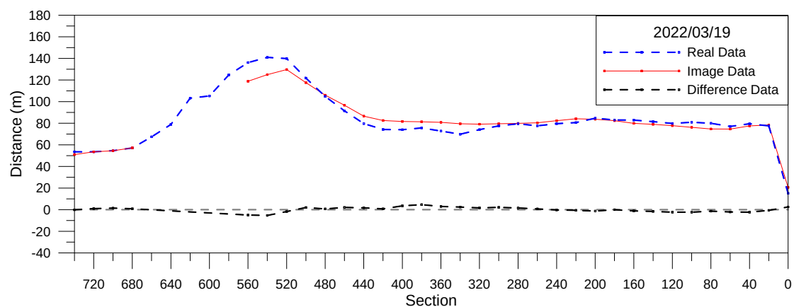
圖 3-23 海岸線分析比較圖(2022/03/19)
