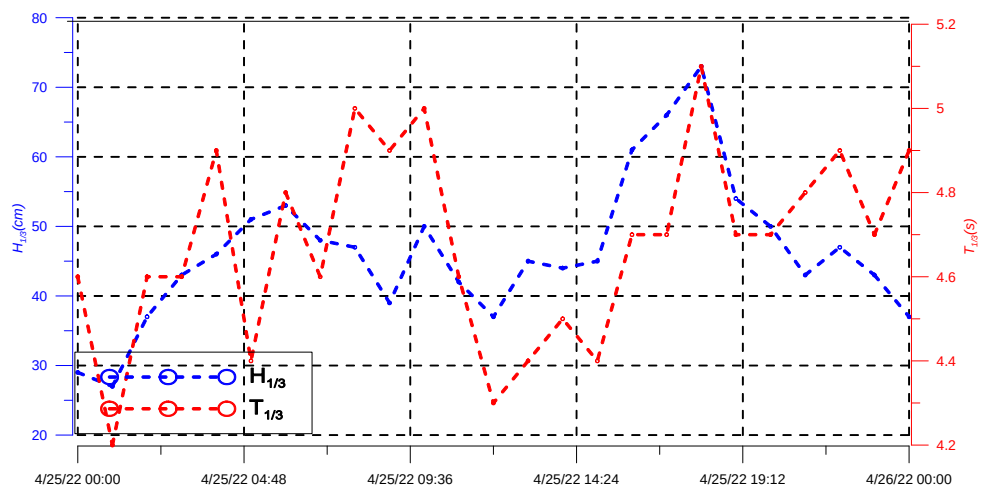
圖 2-3 波浪時序列變化圖
