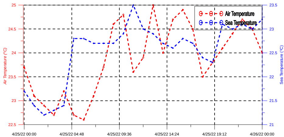
圖 2-4 溫度時序列變化圖
