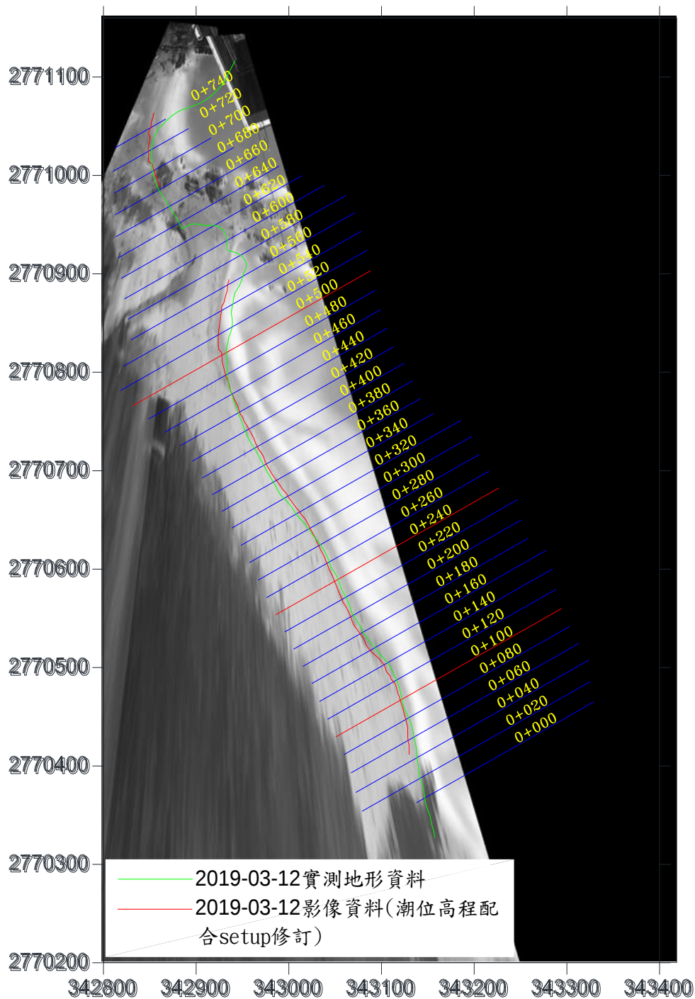
圖 3-22 水位線分析結果圖(2019/03/12)
