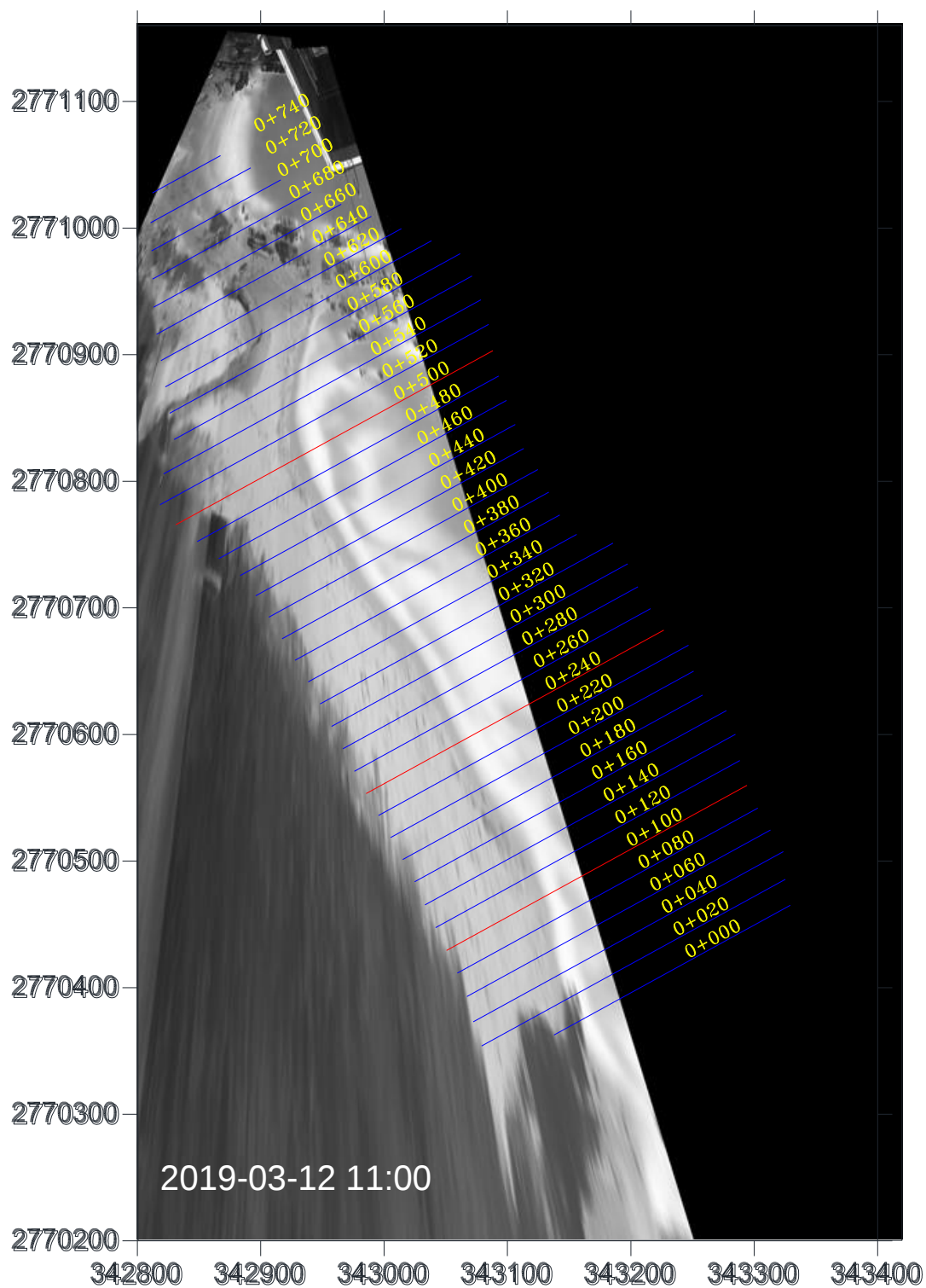
圖 4-19 鹽寮海岸地形影像全景圖(2019/3/12 11:00)
