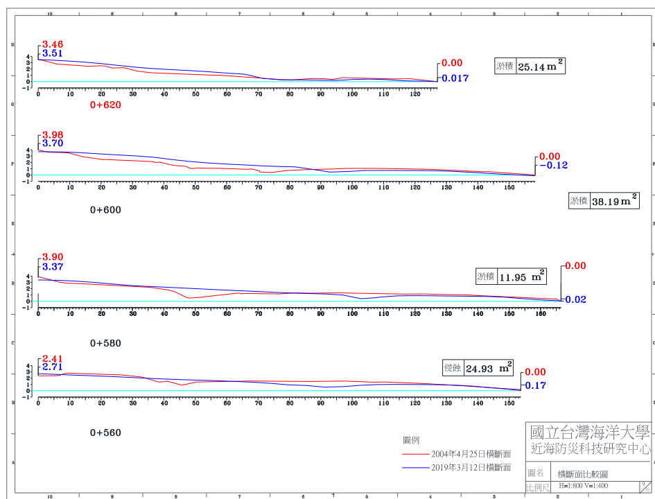
圖 4-4(c) 2019 年 3 月 12 日 A 監測區橫斷面比較圖
