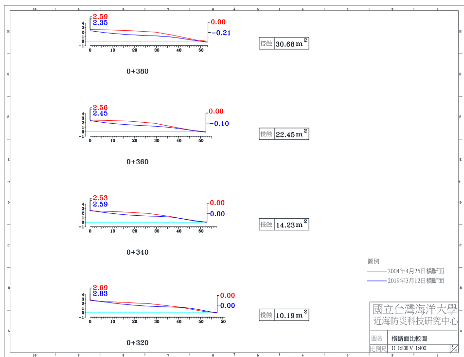
圖 4-4(f) 2019 年 3 月 12 日 A 監測區橫斷面比較圖
