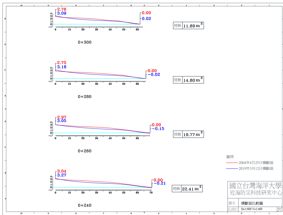
圖 4-4(g) 2019 年 3 月 12 日 A 監測區橫斷面比較圖
