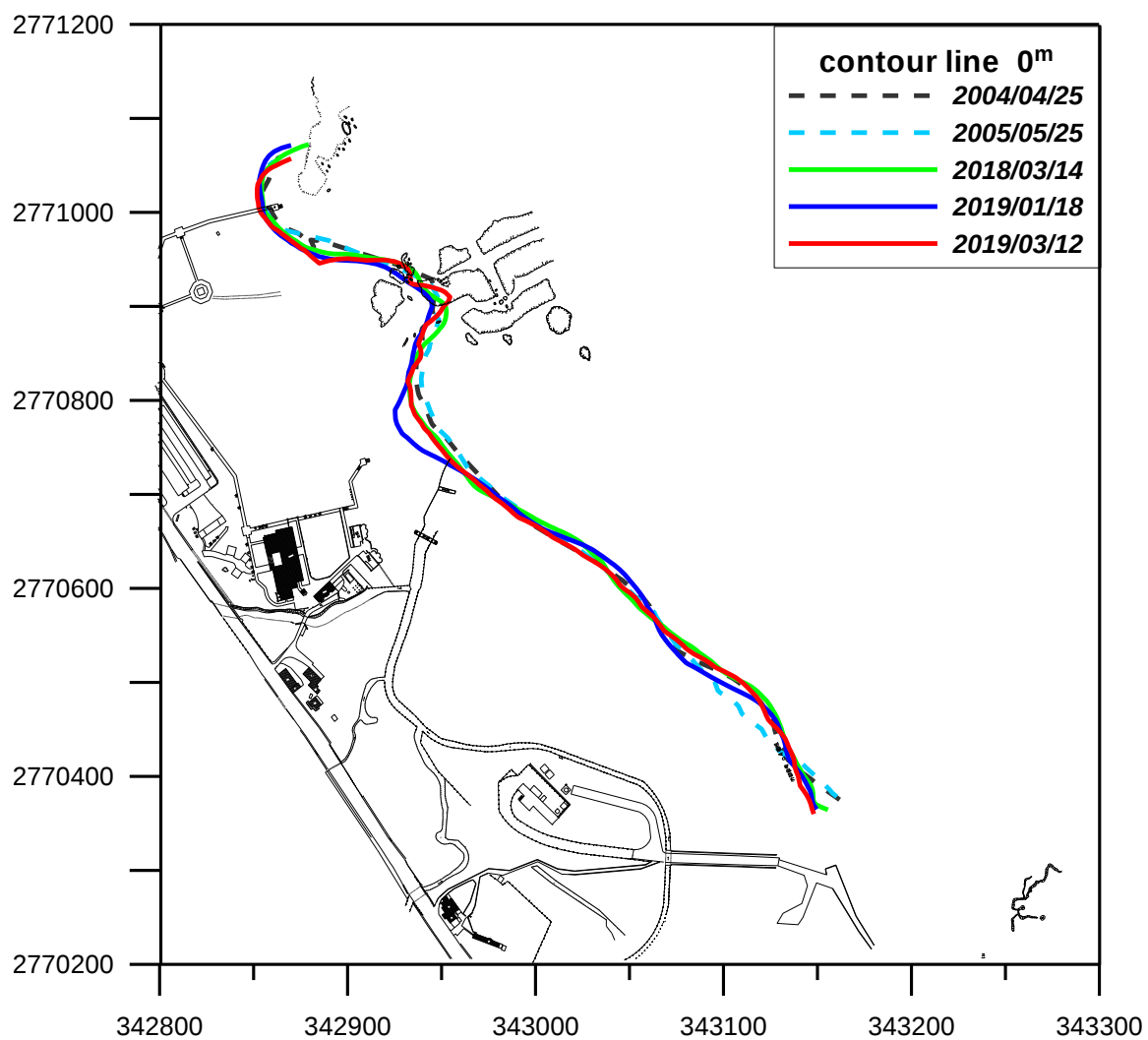
圖 4-2 監測區 0 m 等高線變化比較圖
