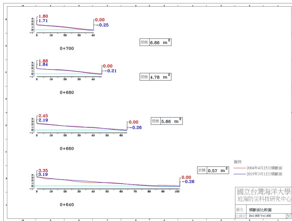
圖 4-4(b) 2019 年 3 月 12 日 A 監測區橫斷面比較圖
