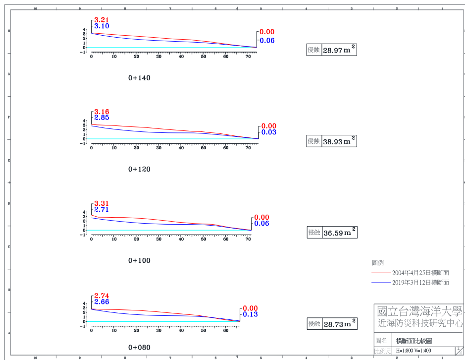
圖 4-4(i) 2019 年 3 月 12 日 A 監測區橫斷面比較圖
