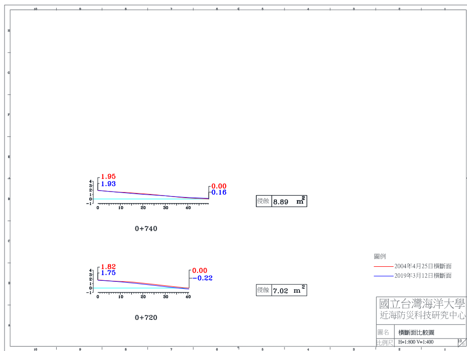
圖 4-4(a) 2019 年 3 月 12 日 A 監測區橫斷面比較圖
