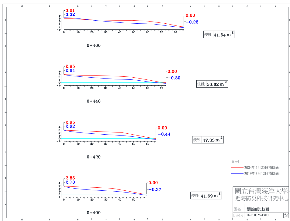
圖 4-4(e) 2019 年 3 月 12 日 A 監測區橫斷面比較圖
