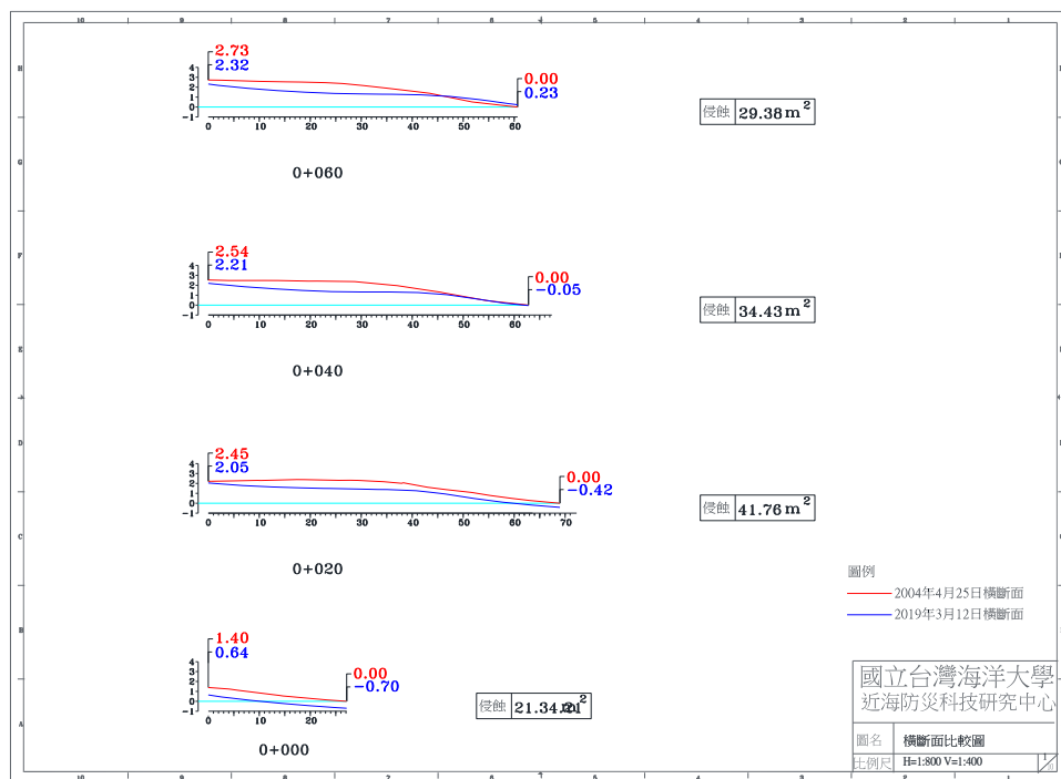
圖 4-4(j) 2019 年 3 月 12 日 A 監測區橫斷面比較圖
