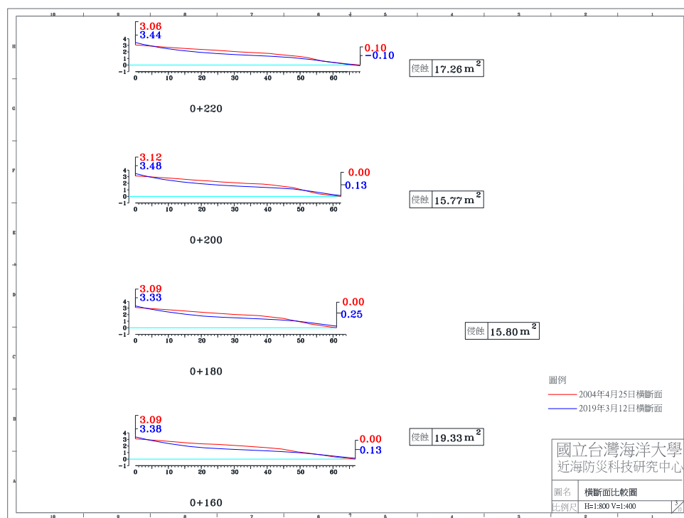
圖 4-4(h) 2019 年 3 月 12 日 A 監測區橫斷面比較圖
