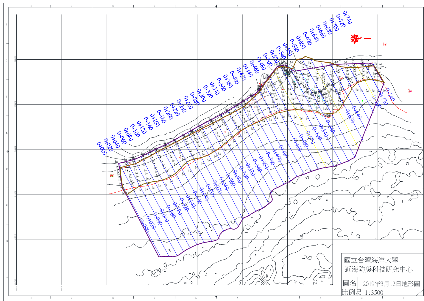
圖 4-1 2019 年 3 月 12 日監測地形圖
