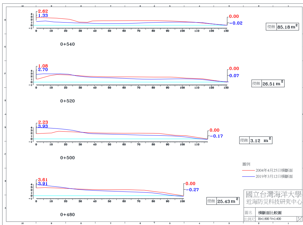
圖 4-4(d) 2019 年 3 月 12 日 A 監測區橫斷面比較圖
