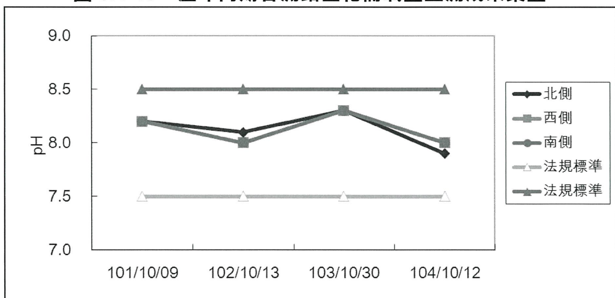
圖 3.1-14 歷年同期各測站 pH 監測成果彙整
