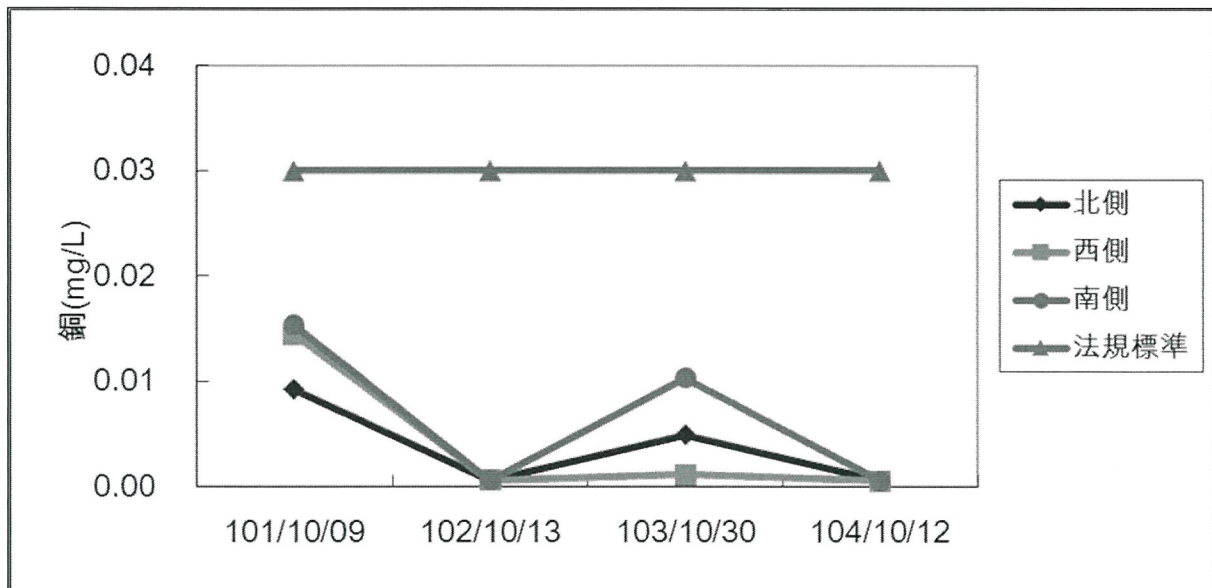
圖 3.1-15 歷年同期各測站銅監測成果彙整
