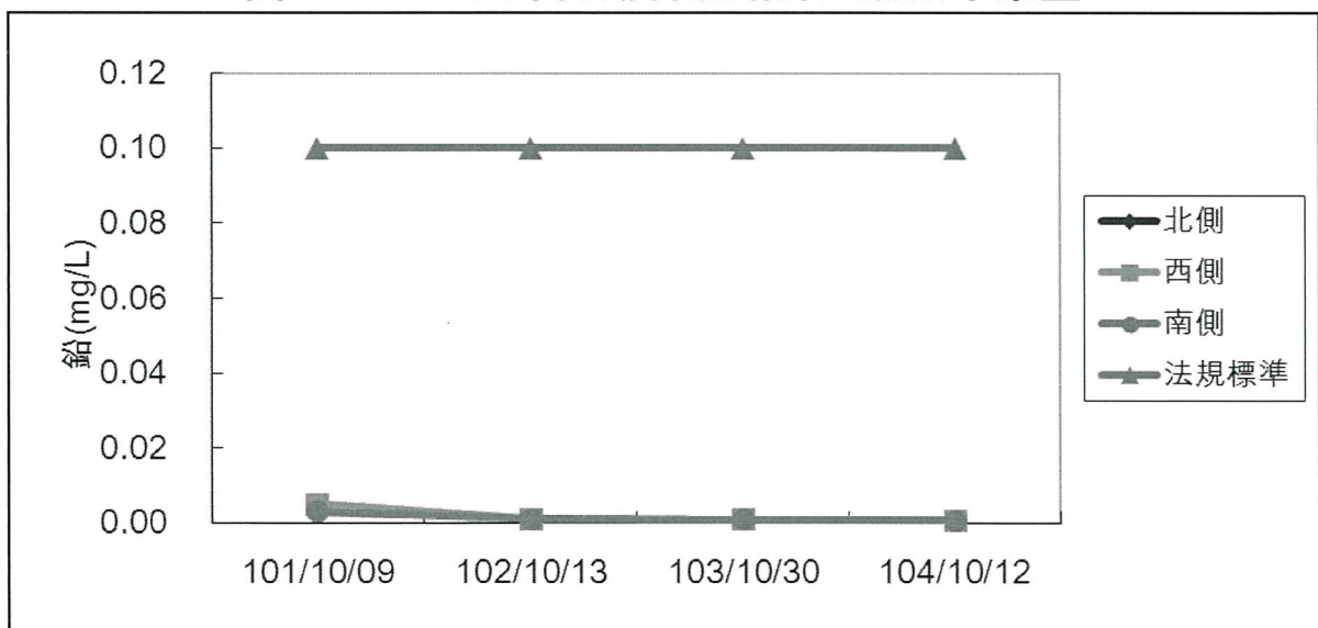
圖 3.1-17 歷年同期各測站鉛監測成果彙整
