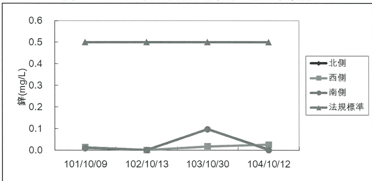
圖 3.1-16 歷年同期各測站鋅監測成果彙整
