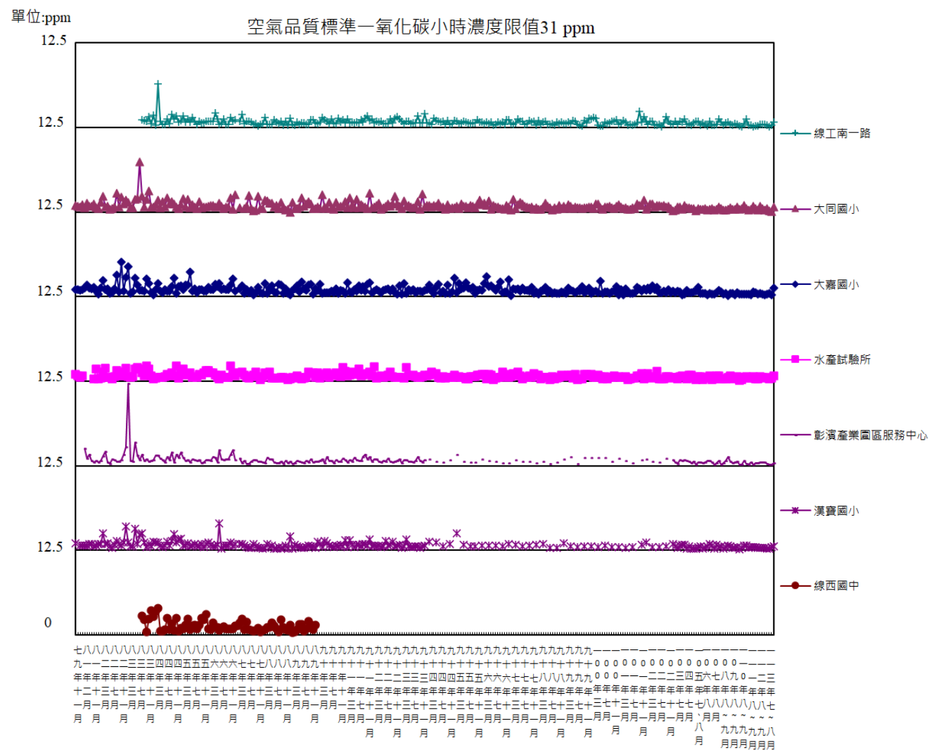
圖3.1.1-1 彰濱地區歷年一氧化碳(CO)最高小時值監測結果分析圖
