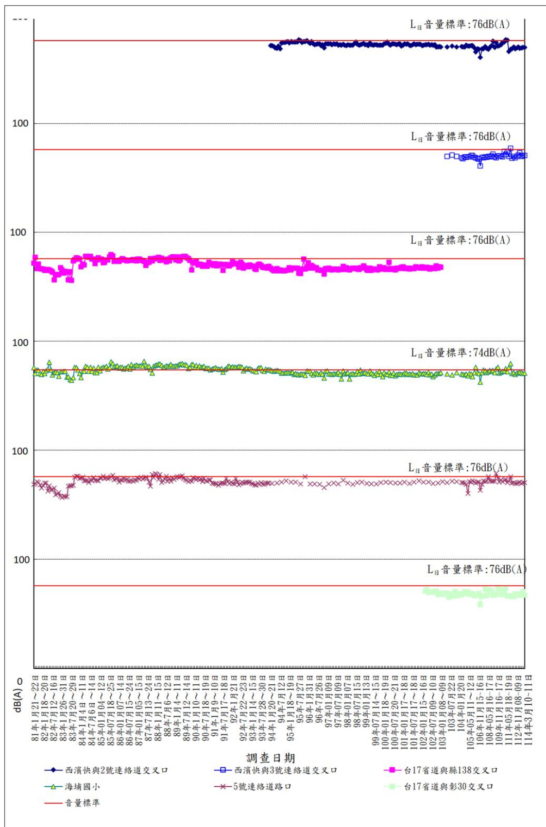
圖 3.1.2-3 彰濱地區歷次噪音 L_{夜} 監測結果
