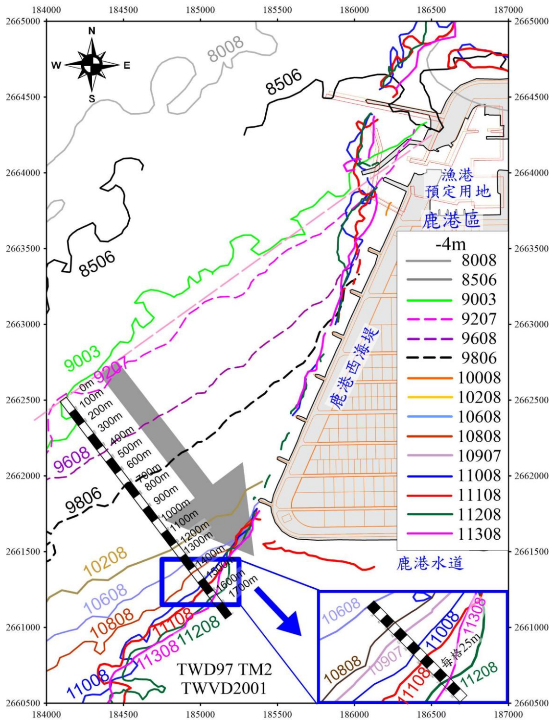
圖 2.11-7 鹿港區西海堤突堤群-4m 等深線位置比較
