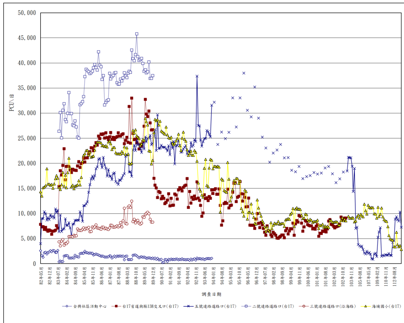
圖 3.1.4-1 彰濱地區歷次交通流量監測結果(1/2)
