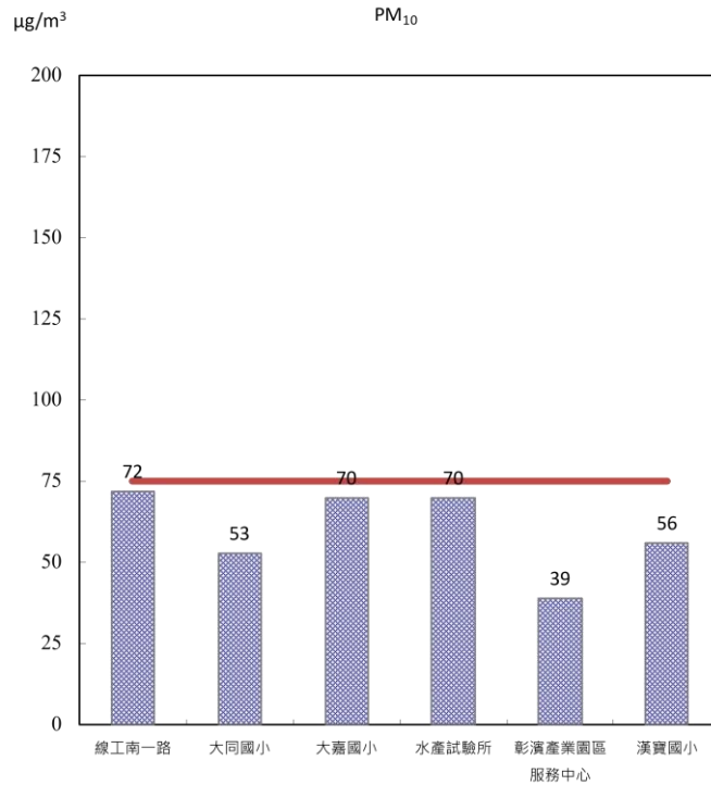
圖 2.1-9 本季各測站 PM 10 日平均值監測結果比較分析圖
