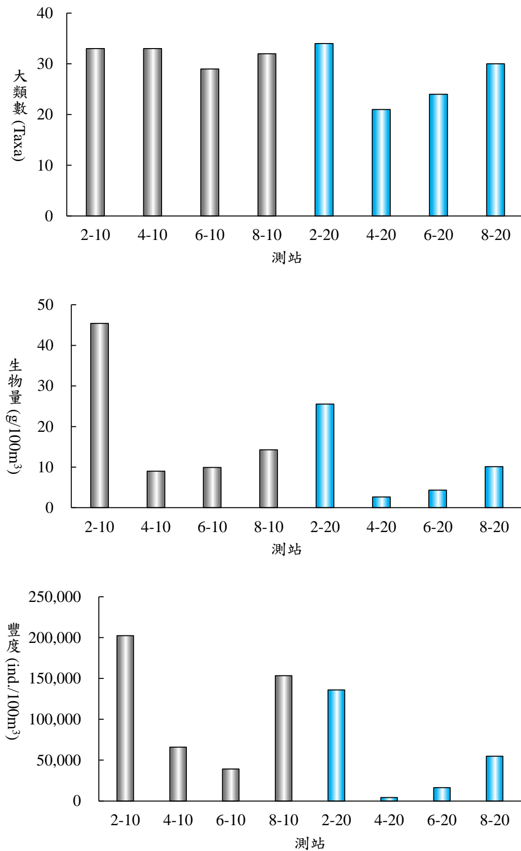
圖 2.10-2 民國 114 年 3 月彰化濱海產業區附近海域浮游動物豐度、生物量(濕重 g)及大類(Taxa)分布圖
