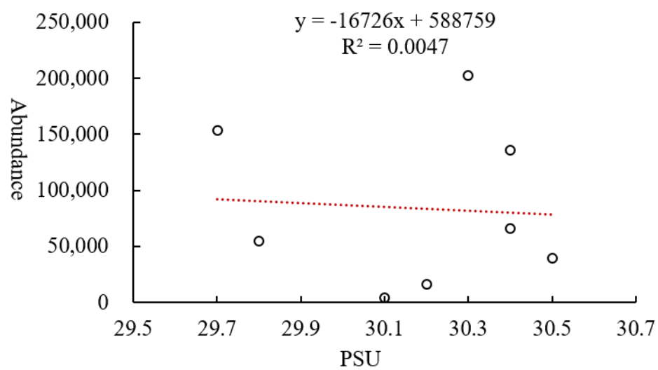
圖 2.10-6 民國 114 年 3 月彰濱產業園區附近海域各測站浮游動物豐度與溫度及鹽度之相關係數圖
