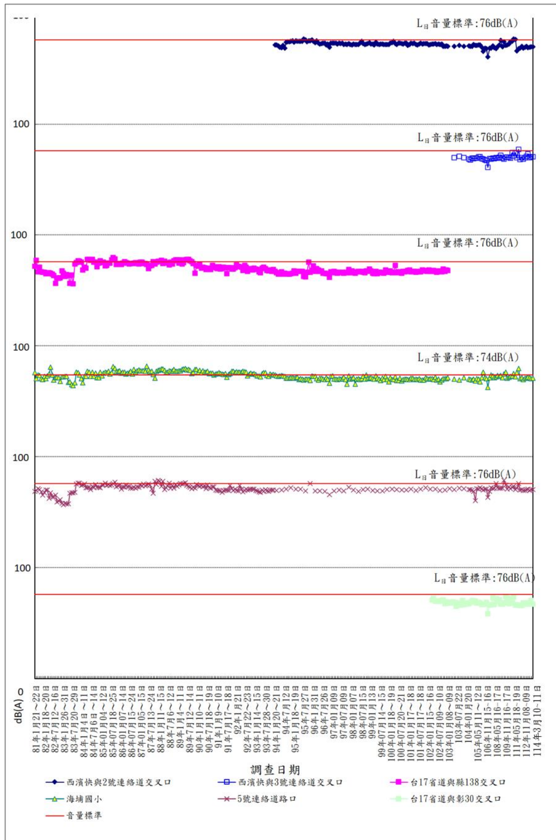
圖 3.1.2-1 彰濱地區歷次噪音 L d 監測結果
