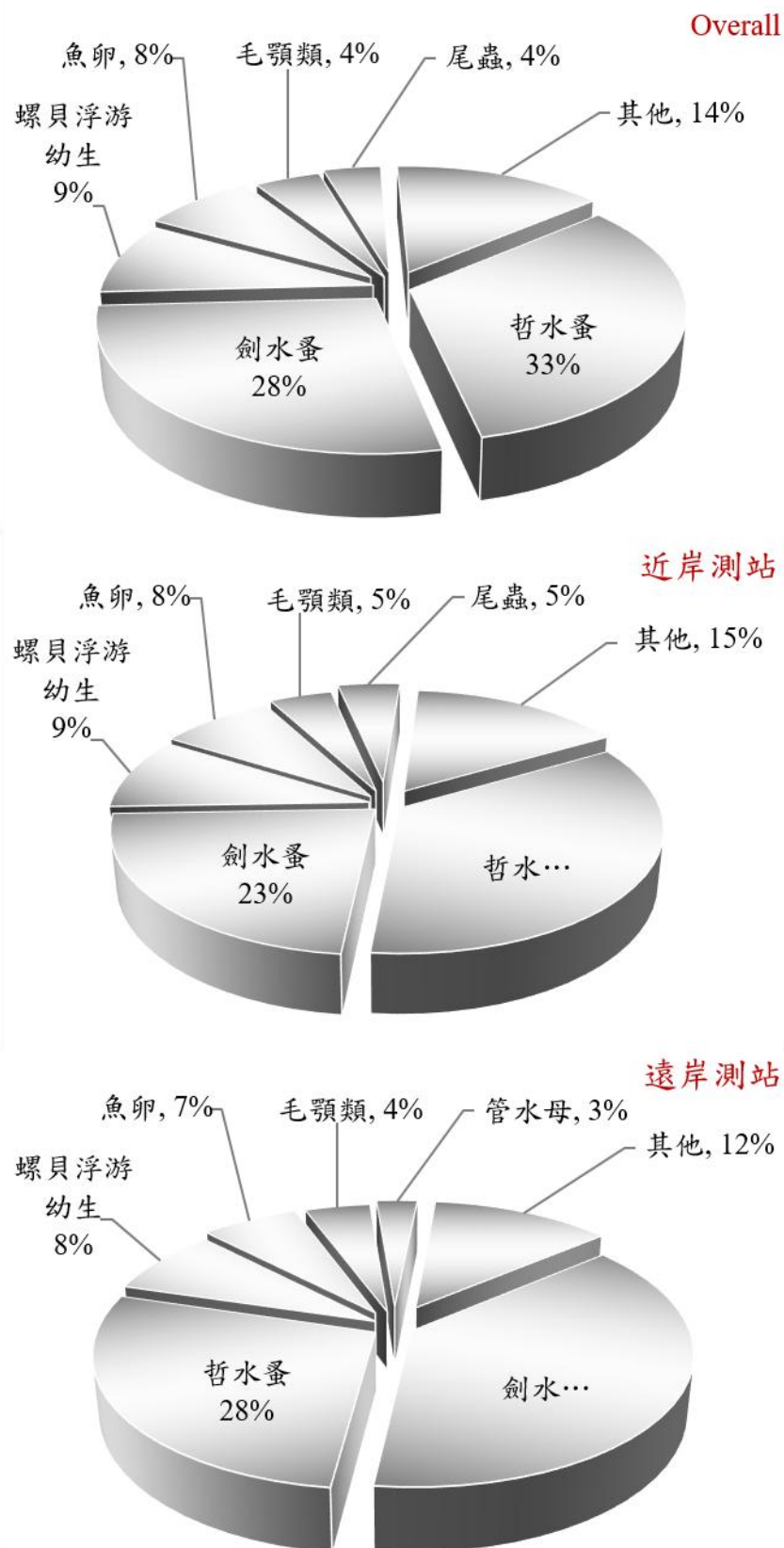
圖 2.10-3 民國 114 年 3 月彰化濱海產業園區附近海域浮游動物主要優勢類群之豐度百分比分布圖
