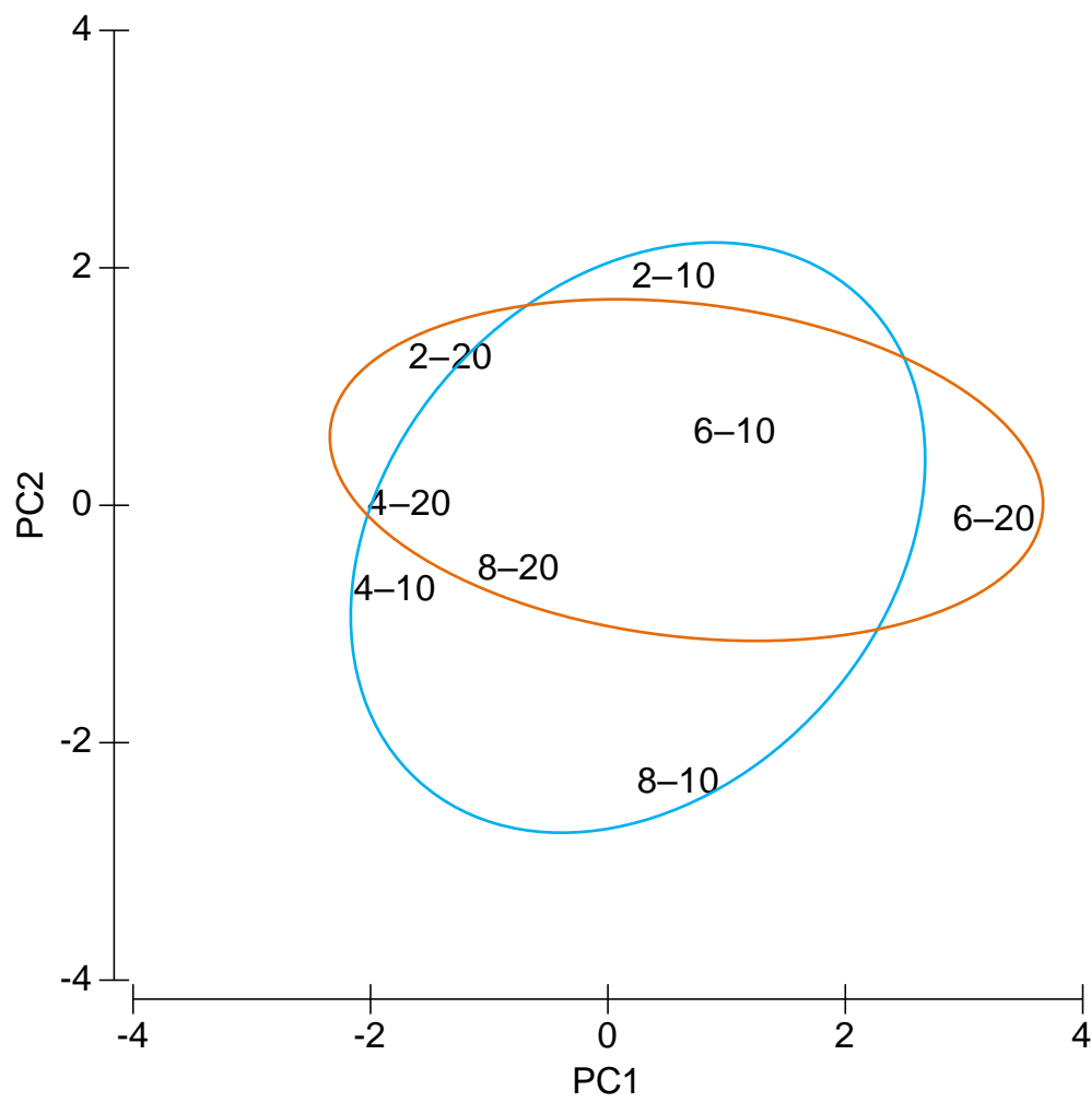
圖 2.10-5 民國 114 年 3 月彰濱產業園區附近海域各測站浮游動物群聚分析圖(圖中第一個數字代表測站，第二個數字代表深度)
