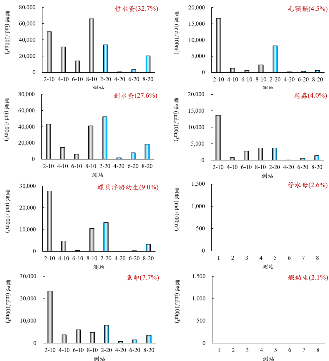
圖 2.10-4 民國 114 年 3 月彰化濱海產業園區附近海域浮游動物主要優勢類群豐度之測站變化圖
