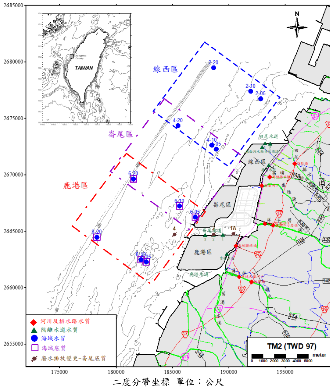
圖 1.4-11 彰濱產業園區河川及排水路、隔離水道與海域水質(含底質)監測點位示意圖
