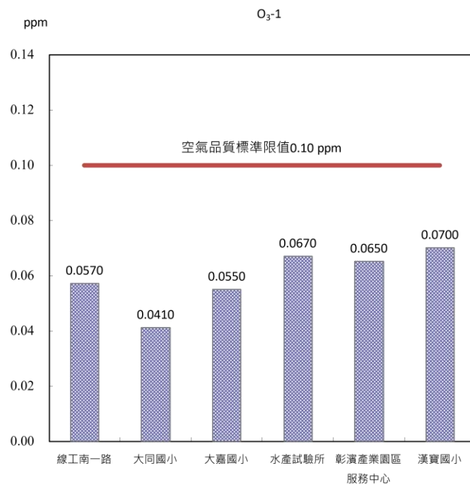
圖 2.1-7 本季各測站 O 3 最高小時值監測結果比較分析圖
