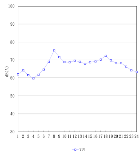
圖 2.2-6 海埔國小本季噪音測值逐時變化圖
