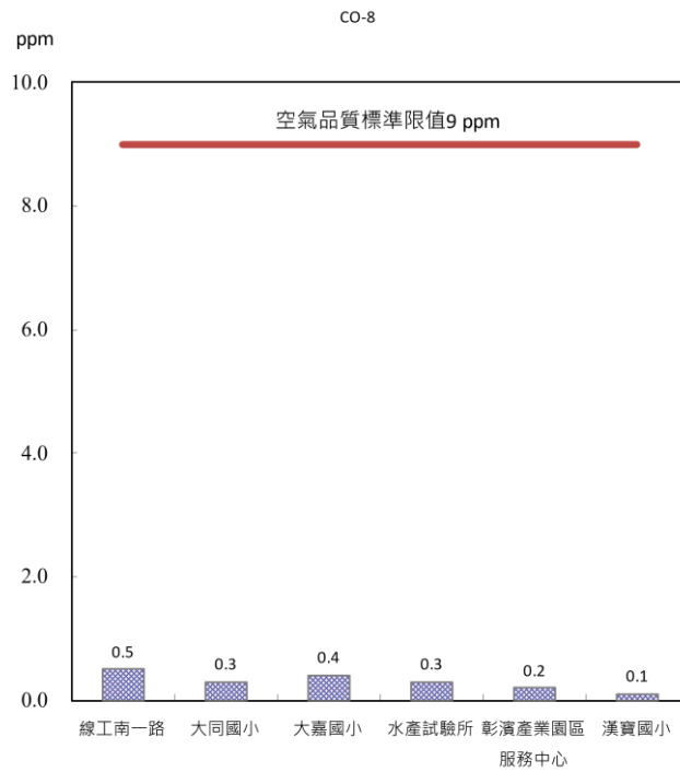
圖 2.1-1 本季各測站 CO 最高 8 小時平均值監測結果比較分析圖
