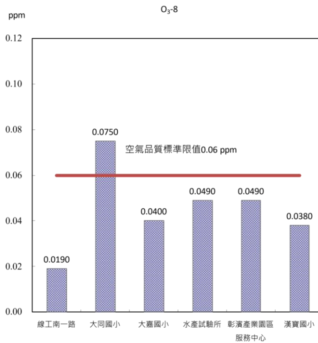
圖 2.1-6 本季各測站 O 3 最高 8 小時平均值監測結果比較分析圖
