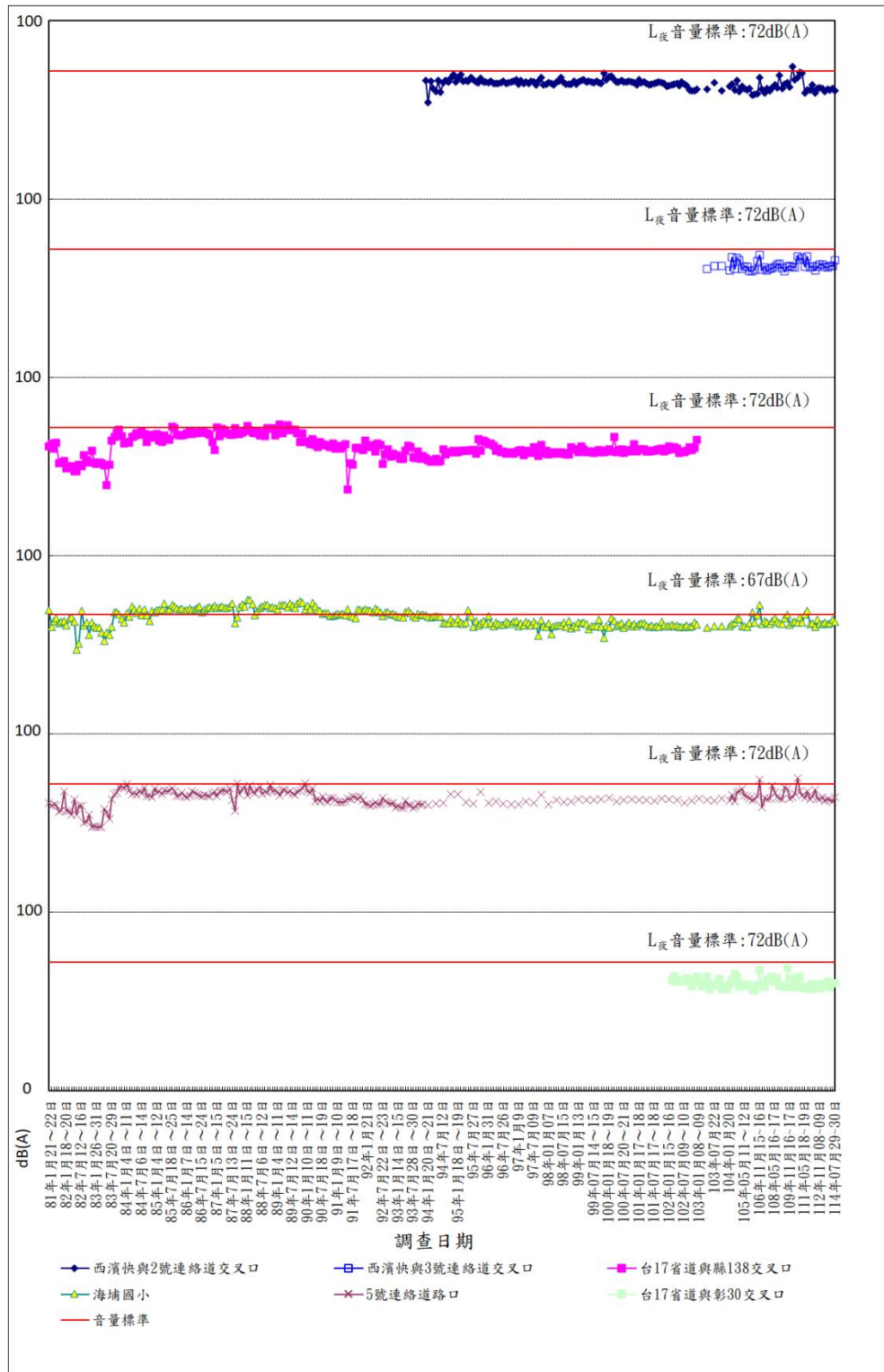
圖 3.1.2-3 彰濱地區歷次噪音 L 夜 監測結果
