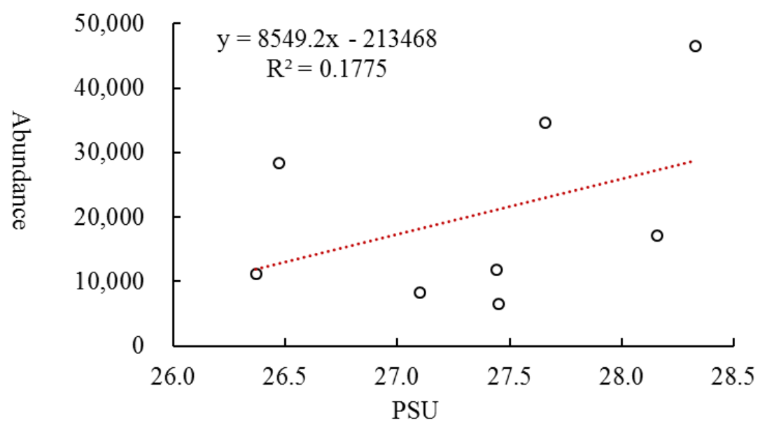
圖 2.10-6 民國 114 年 8 月彰濱產業園區附近海域各測站浮游動物豐度與溫度及鹽度之相關係數圖
