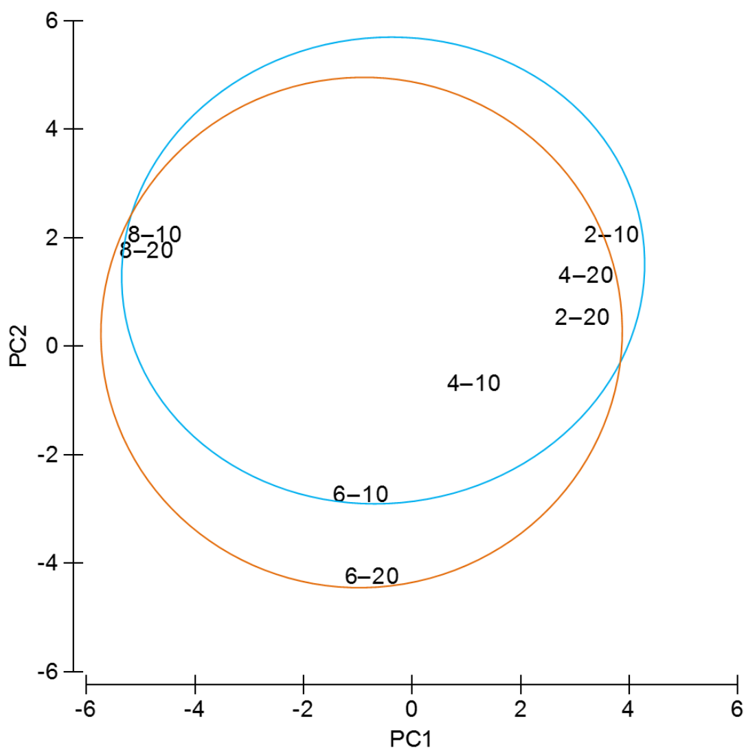
圖 2.10-5 民國 114 年 8 月彰濱產業園區附近海域各測站浮游動物群聚分析圖(圖中第一個數字代表測站，第二個數字代表深度)
