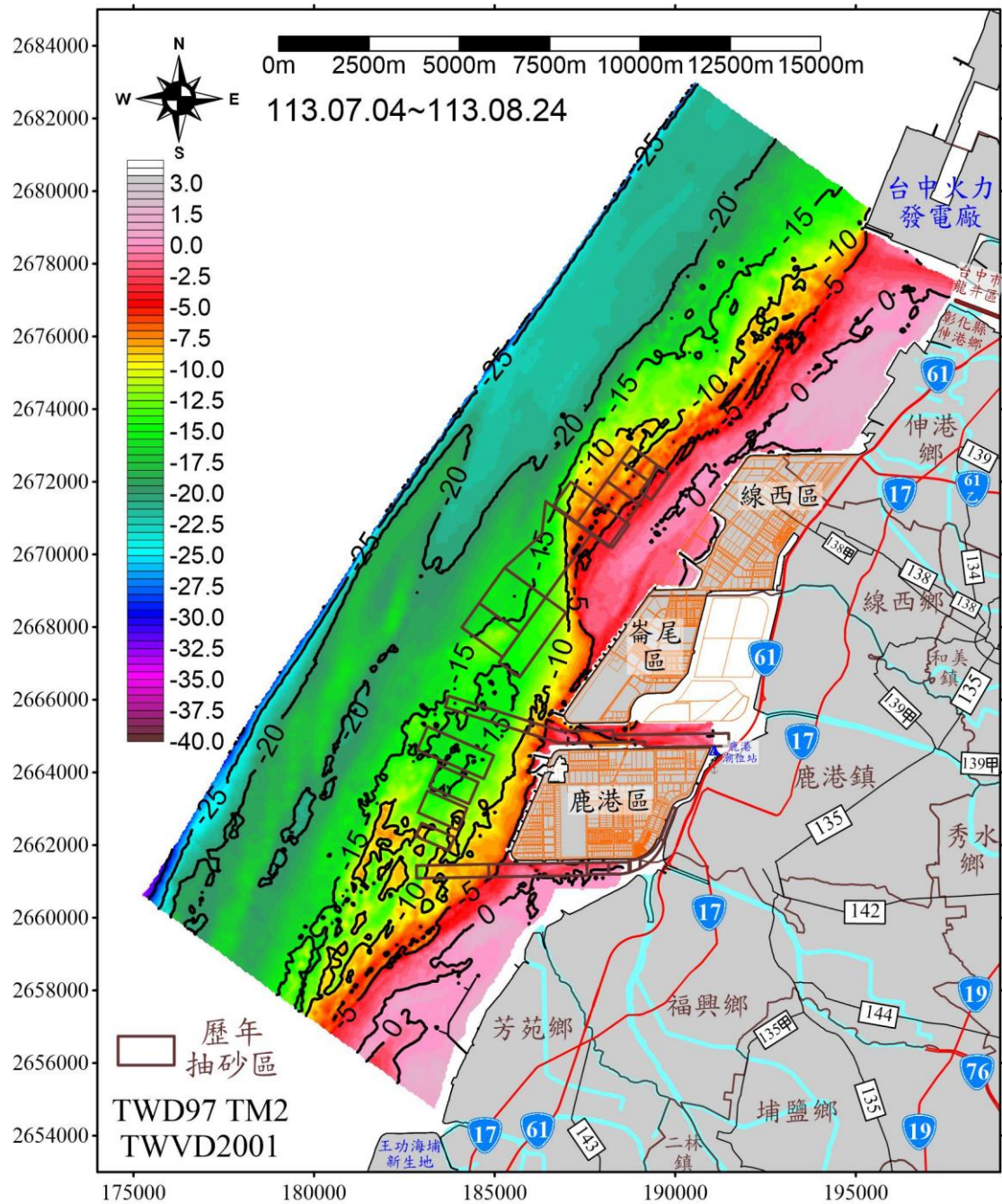
圖 2.11-1 113 年 7 月~9 月海底地形影像圖
