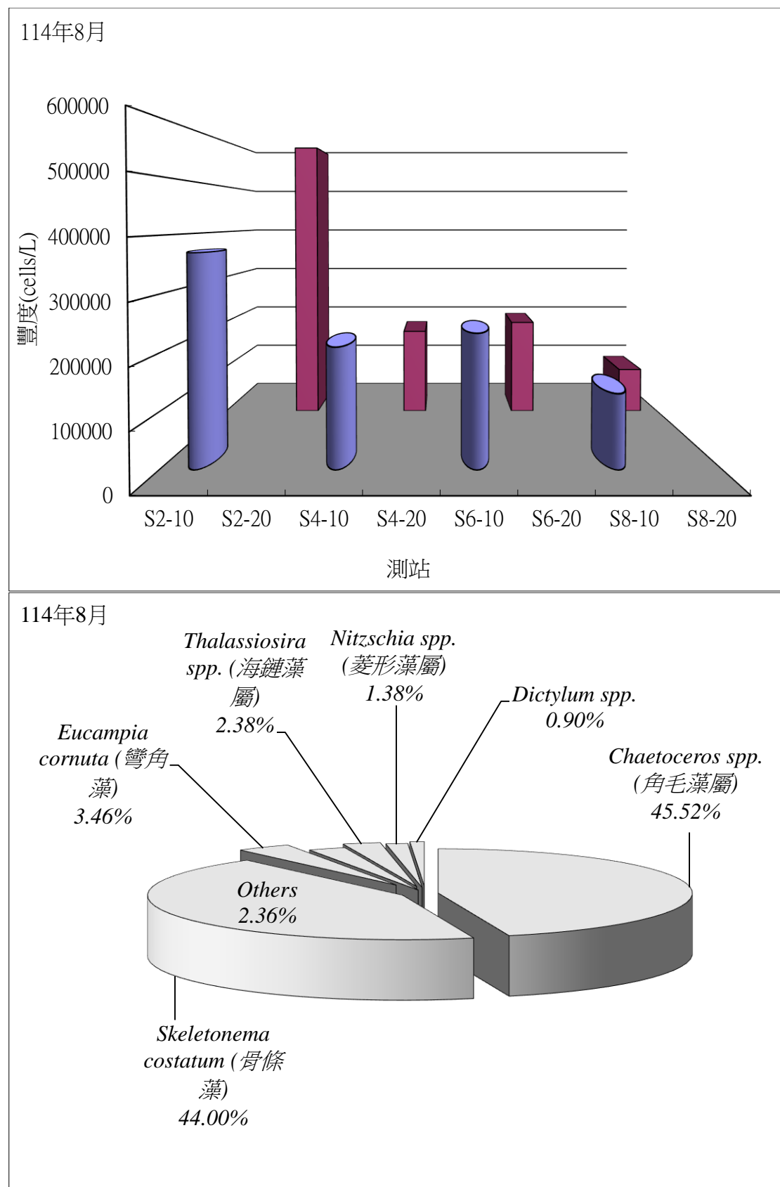
圖 2.10-1 民國 114 年 8 月於彰化濱海產業園區附近海域各測站之浮游植物豐度分析圖
