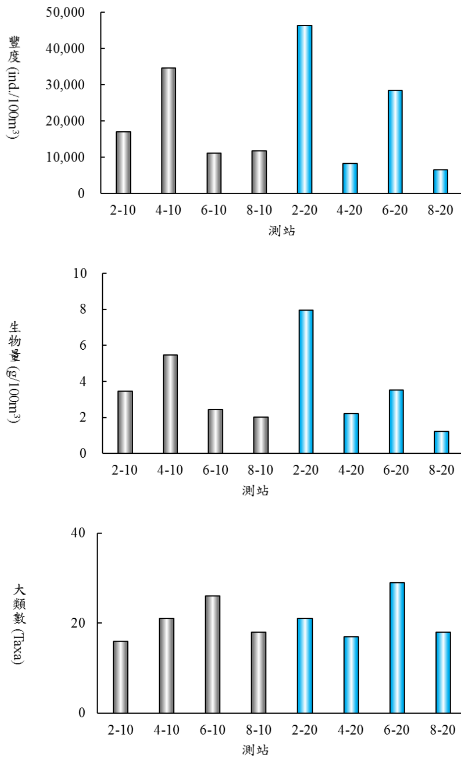
圖 2.10-2 民國 114 年 8 月彰化濱海產業區附近海域浮游動物豐度、生物量(濕重 g)及大類(Taxa)分布圖
