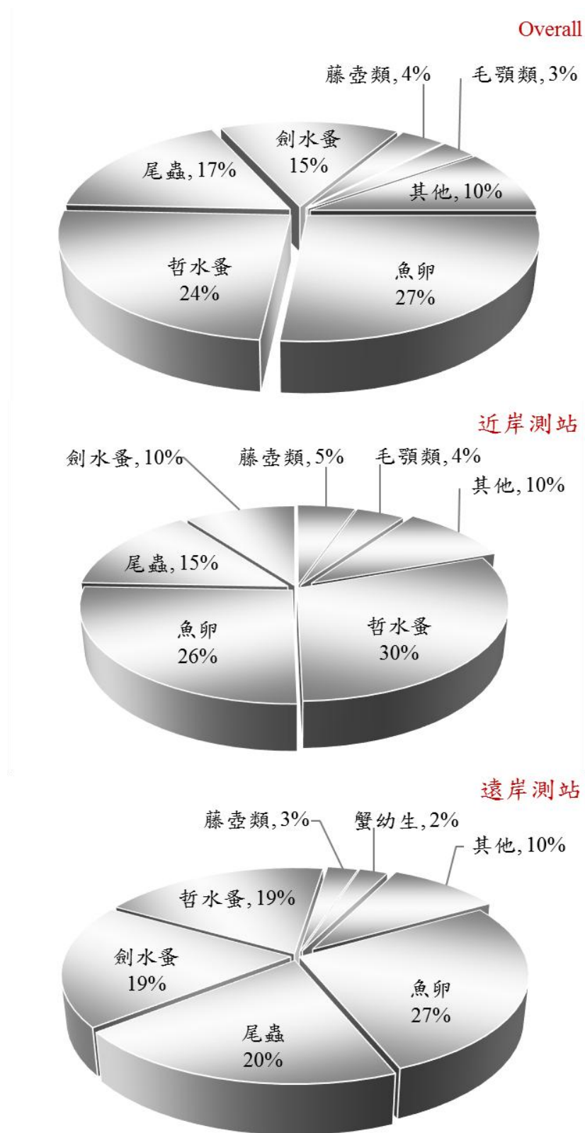
圖 2.10-3 民國 114 年 8 月彰化濱海產業園區附近海域浮游動物主要優勢類群之豐度百分比分布圖
