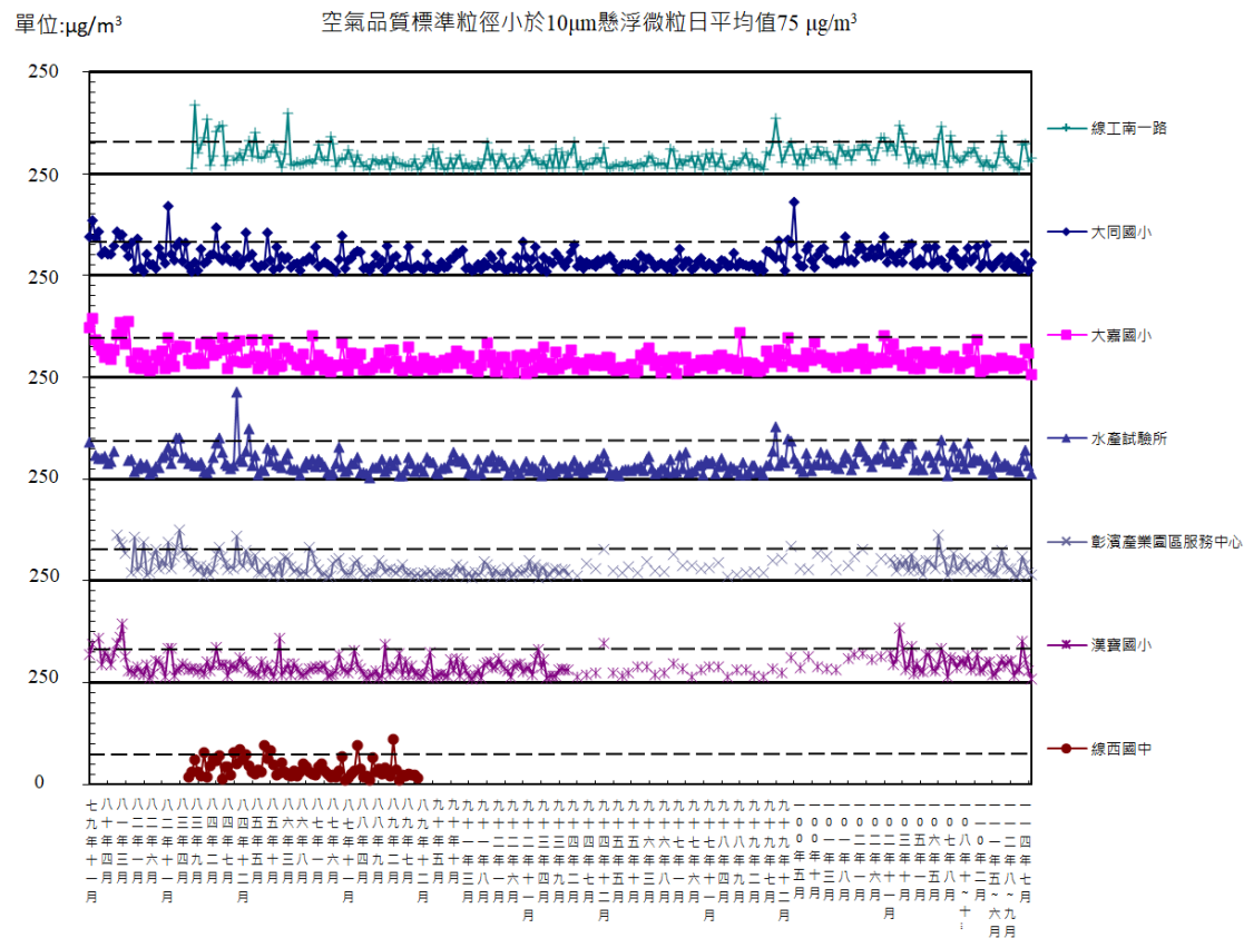
圖 3.1.1-7 彰濱地區歷年粒徑小於 10 \mu m 之懸浮微粒 (PM 10 ) 日平均值監測結果分析圖
