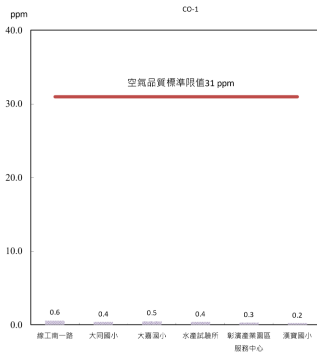
圖 2.1-2 本季各測站 CO 最高小時值監測結果比較分析圖
