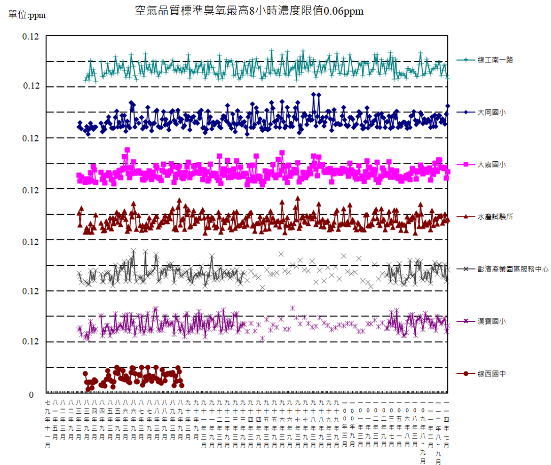
圖 3.1.1-5 彰濱地區歷年臭氧最高 8 小時平均值監測結果分析圖
