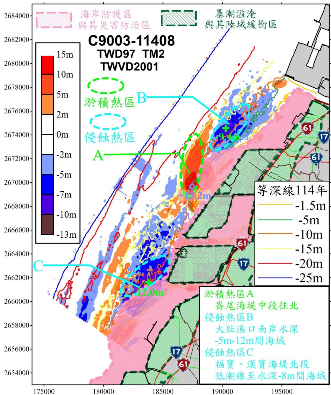
圖2.11-5 彰濱海域長期(24年期間)侵淤熱區區位圖
