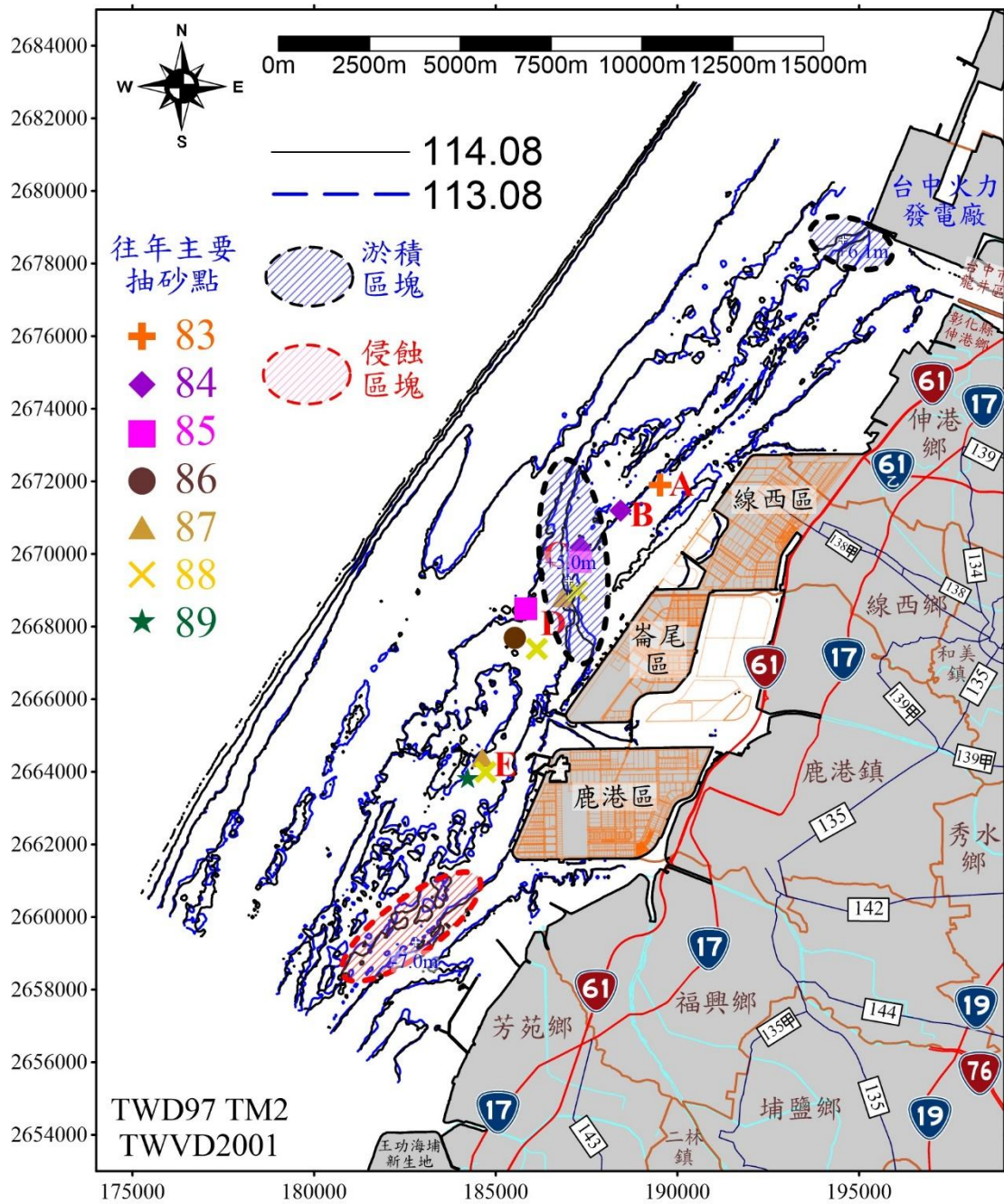
圖 2.11-3 113 年 8 月與 114 年 8 月兩次施測地形等深線比較圖
