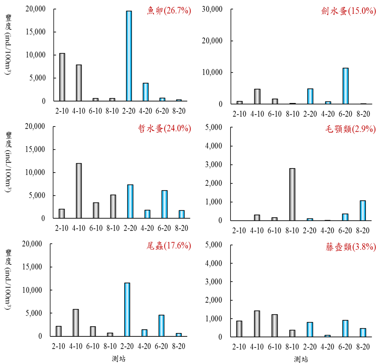
圖 2.10-4 民國 114 年 8 月彰化濱海產業園區附近海域浮游動物主要優勢類群豐度之測站變化圖
