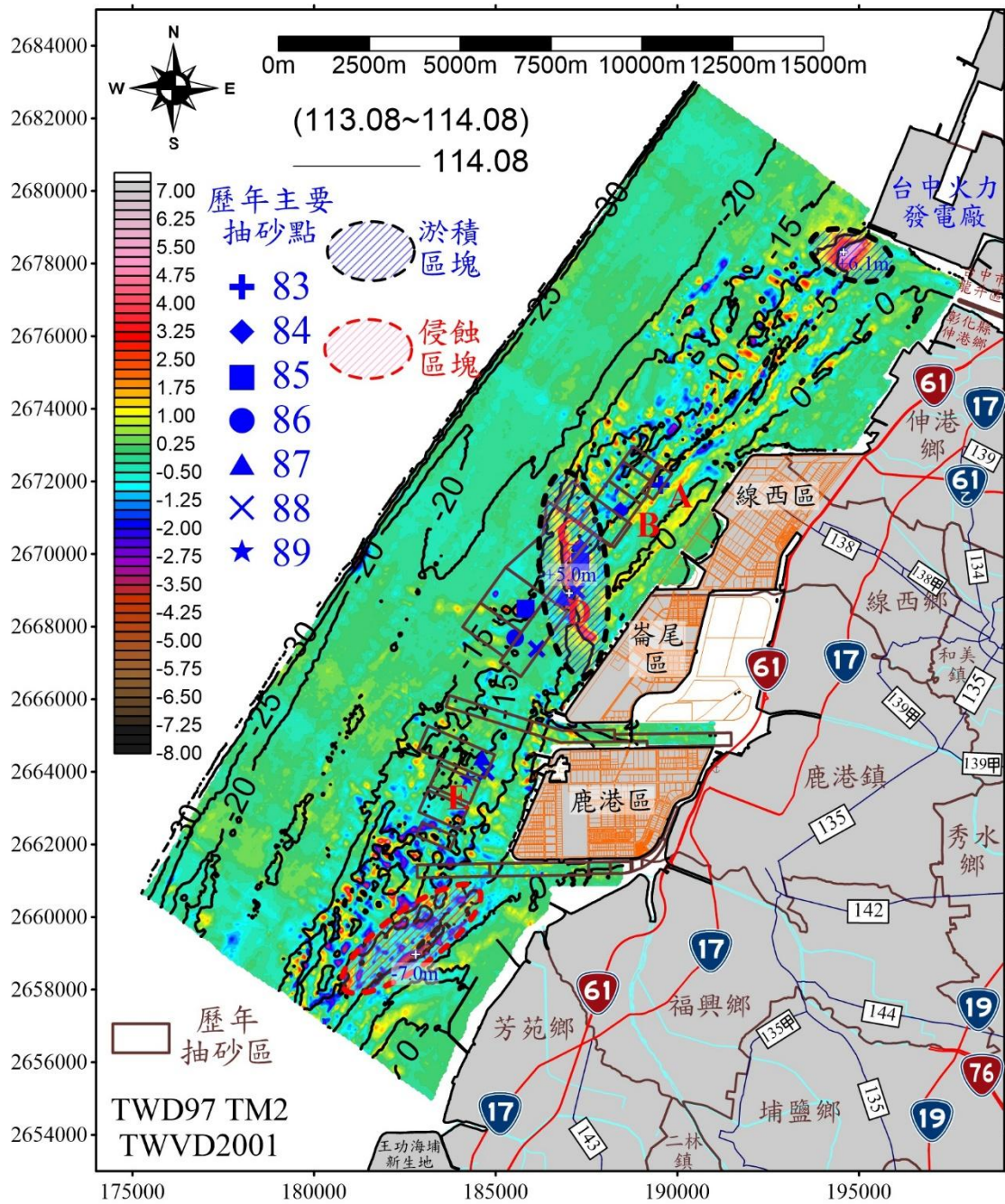
圖 2.11-4 113 年 8 月與 114 年 8 月海底地形侵淤圖
