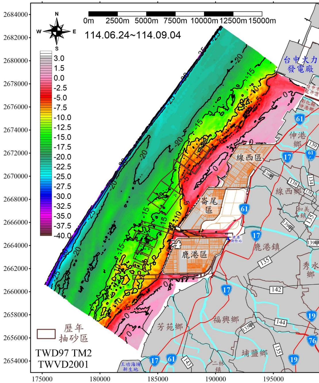
圖 2.11-2 114 年 6 月~9 月海底地形影像圖
